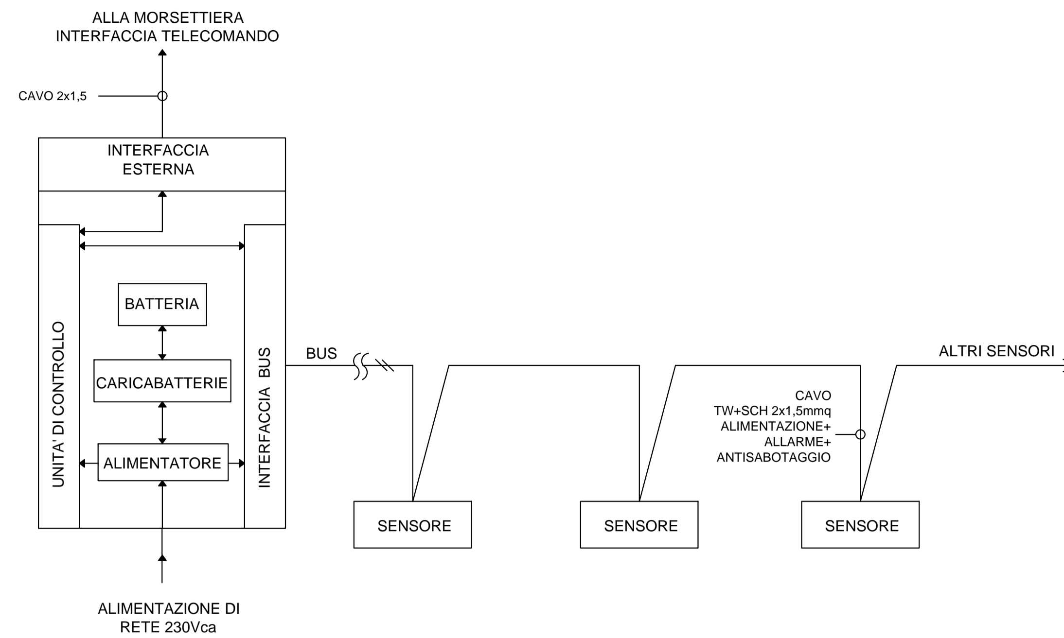
SCHEMA DI PRINCIPIO
