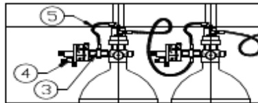
Figura 2 – Dettaglio Valvola di scarica e collettore pneumatico
