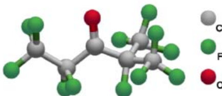
Figura 1: Struttura Chimica del Fluido FK-5-1-12
