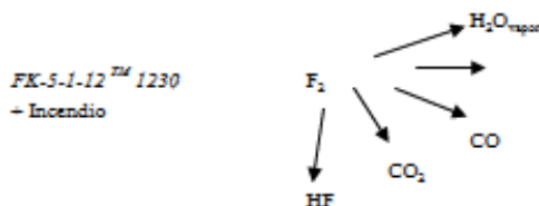
Figure 2: Decomposizione termica del Fluido FK-5-1-12 nella zona della reazione
