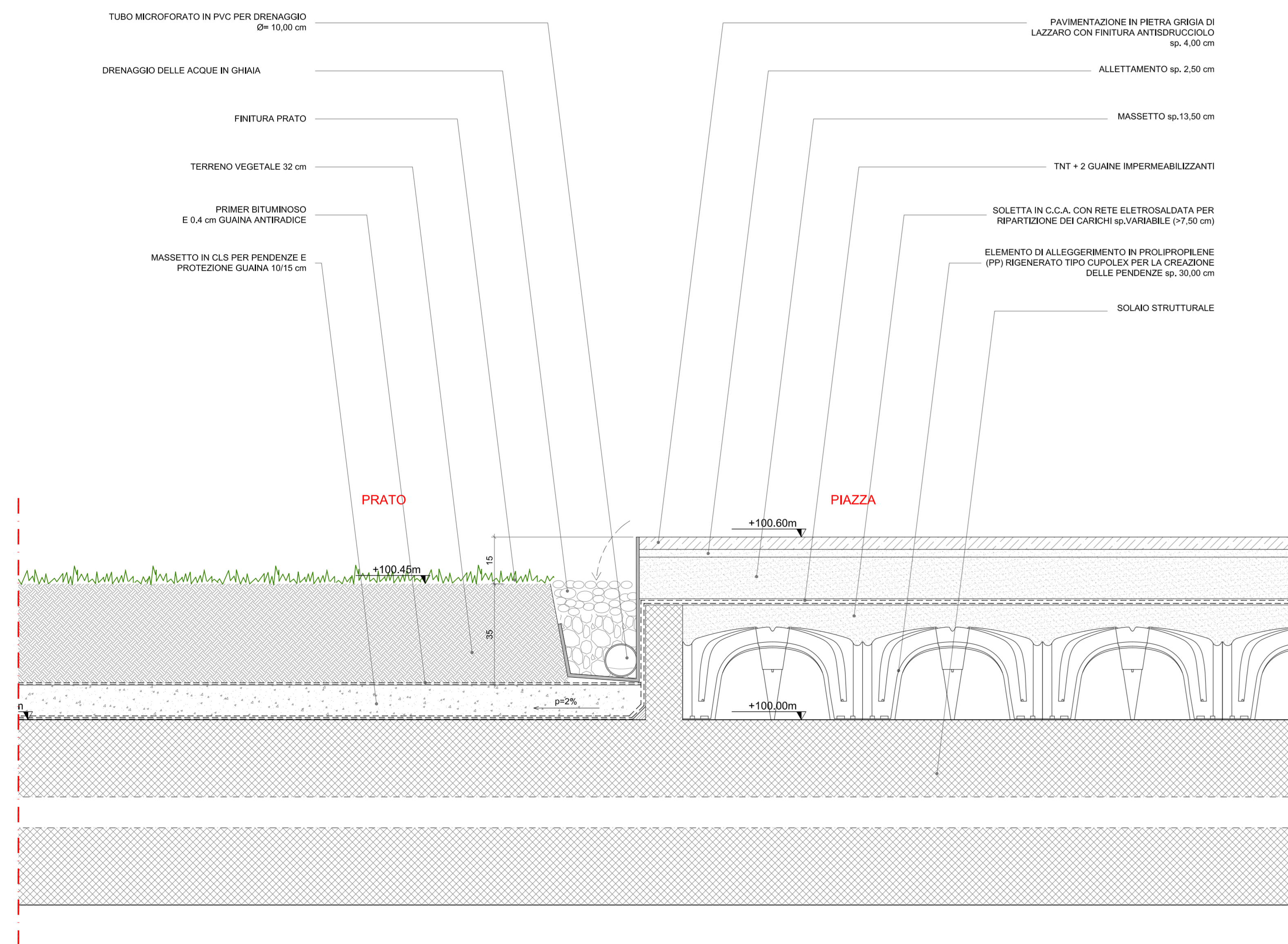
03 PARTICOLARE PAVIMENTAZIONE PIAZZA - PRATO 1:10
