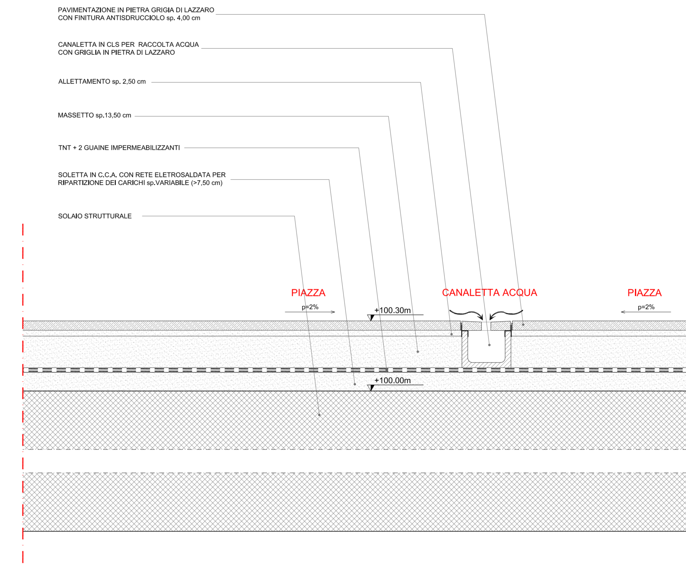
02 PARTICOLARE PAVIMENTAZIONE PIAZZA - CANALETTA ACQUA 1:10
