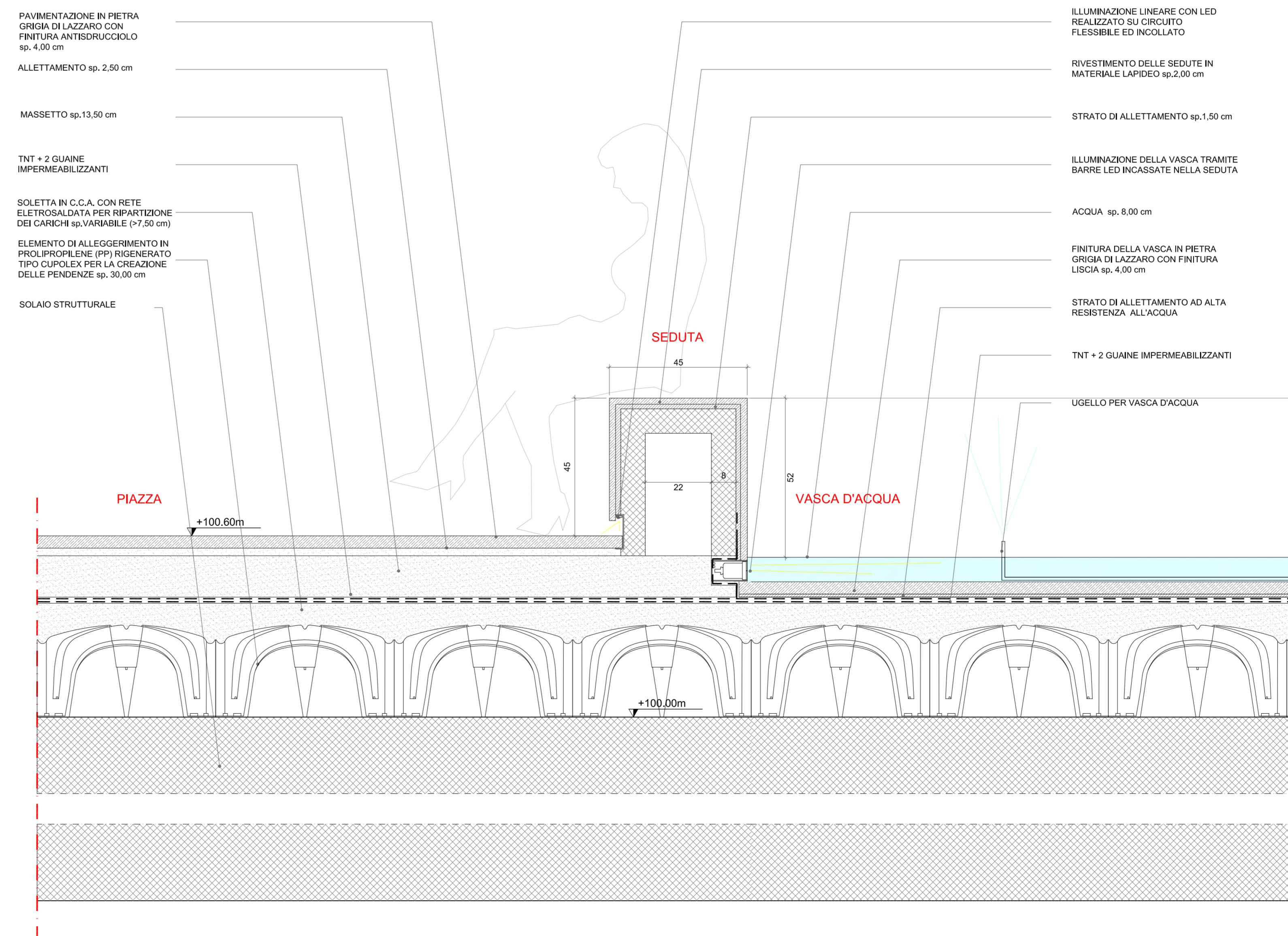
04 PARTICOLARE PAVIMENTAZIONE PIAZZA - VASCA D'ACQUA 1:10
