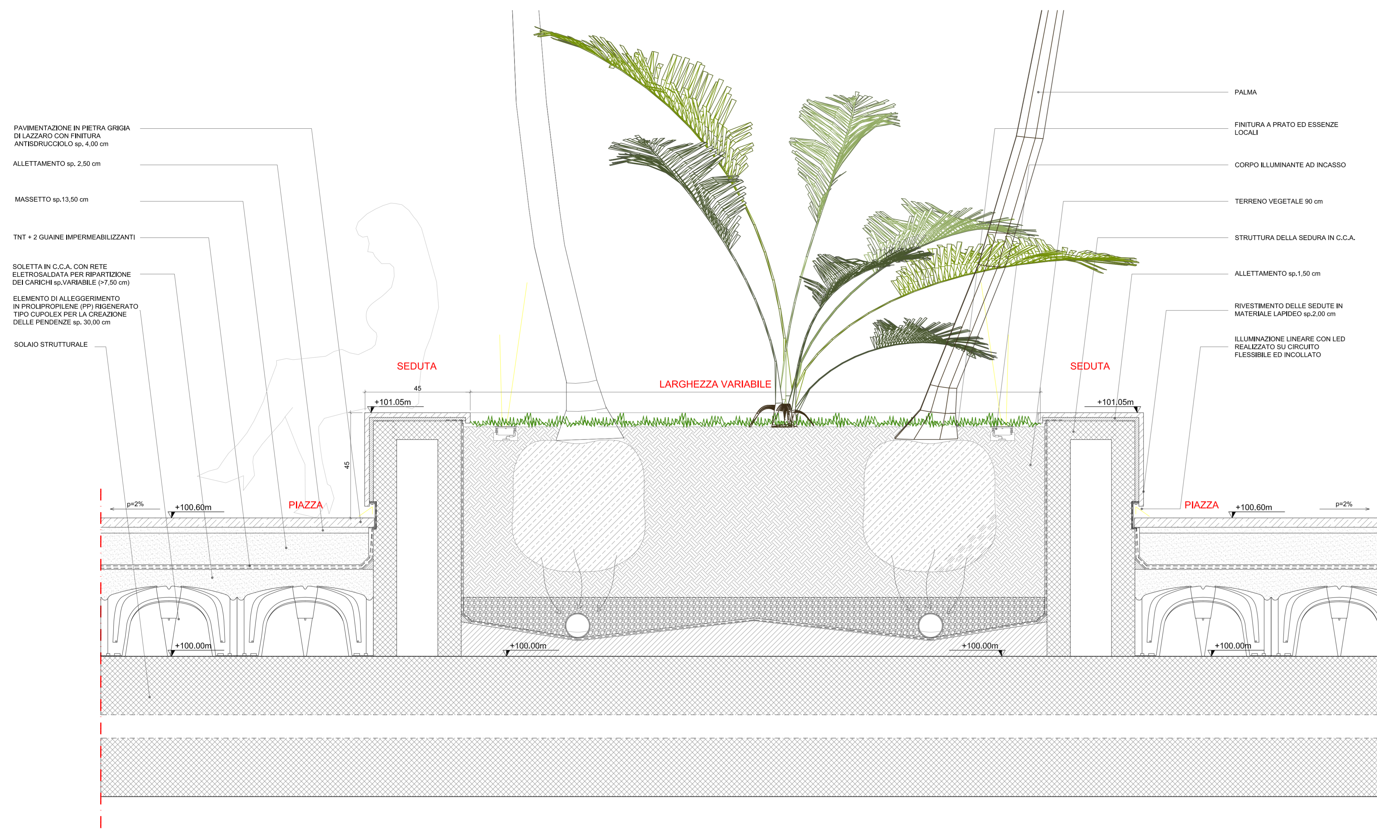
01 PARTICOLARE PAVIMENTAZIONE PIAZZA - FIORIERA 1:10
