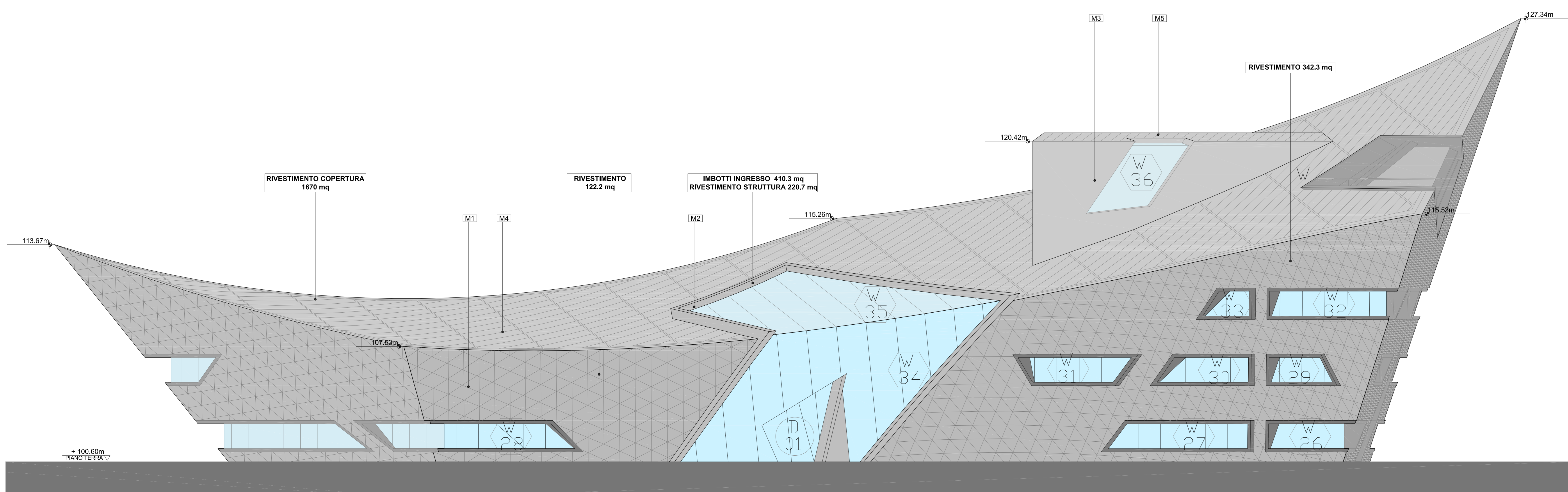
01 PROSPETTO NORD SCALA 1:100
