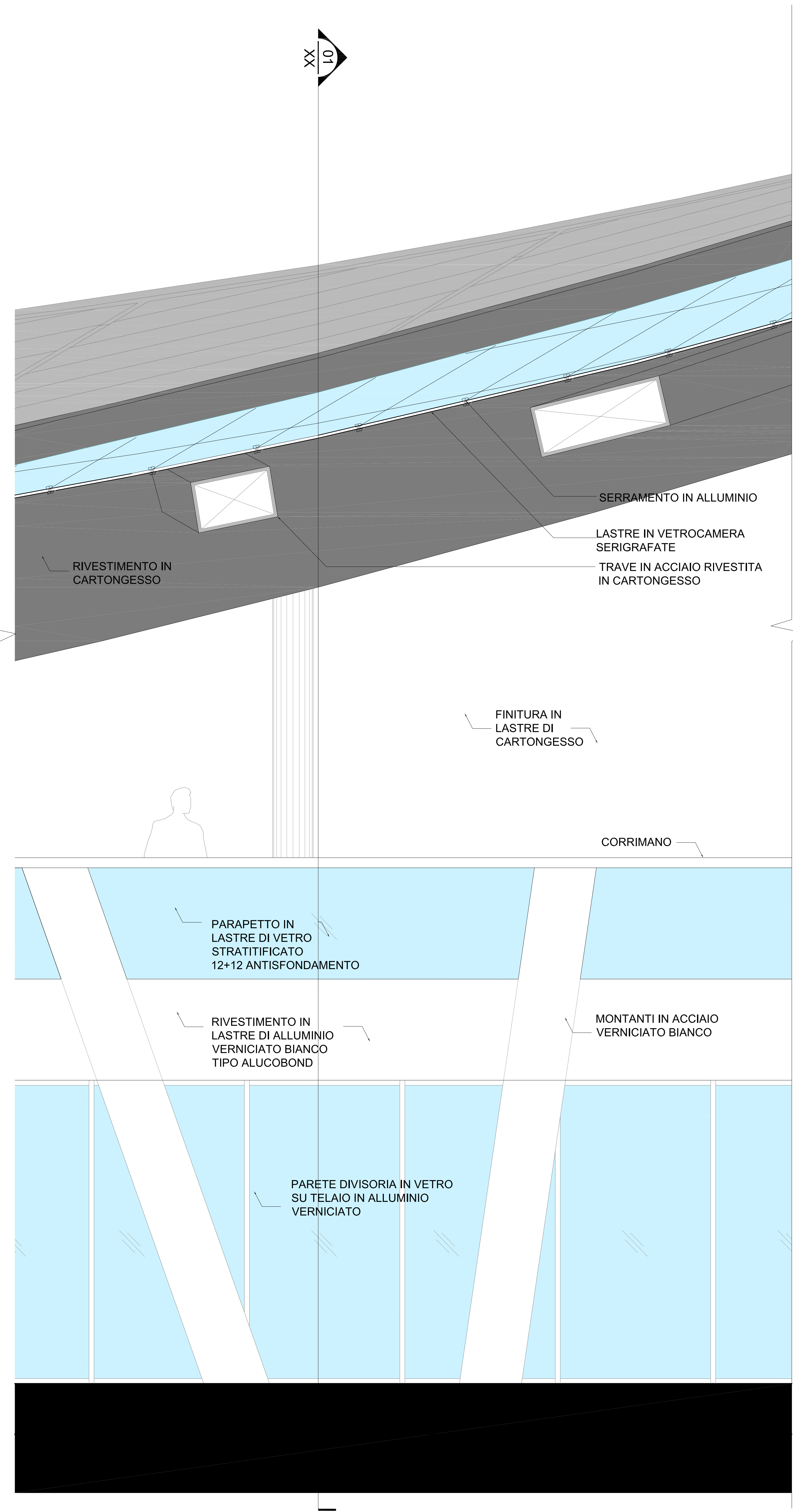
02 PROSPETTO OVEST SCALA 1:20
