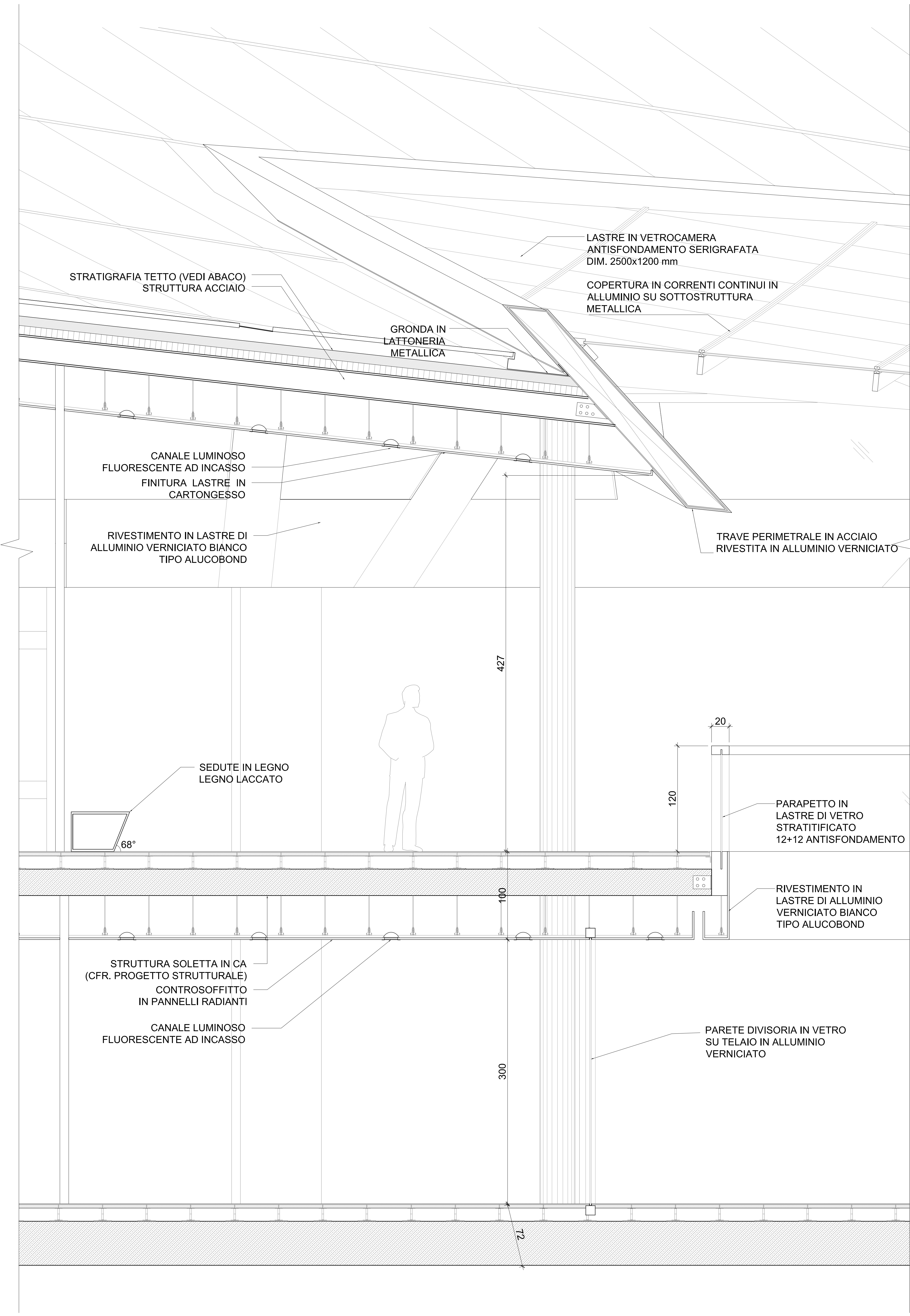
01 SEZIONE DETTAGLIATA LOBBY SCALA 1:20
