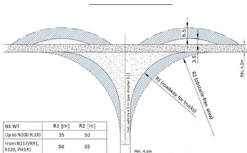
Figura 5 - Raggi minimi di curvatura ed ingombri da assicurare per il transito dei mezzi eccezionali sulla viabilità interna al parco
