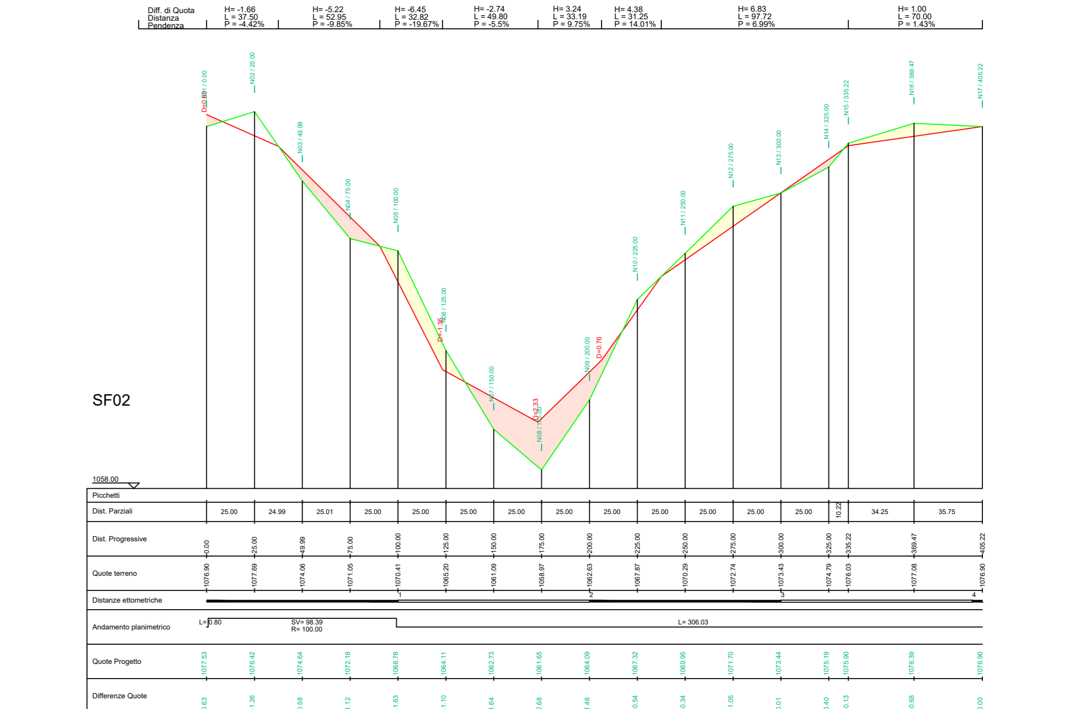
Profilo Longitudinale Scala altezza 1:200 Scala lunghezza 1:2000
