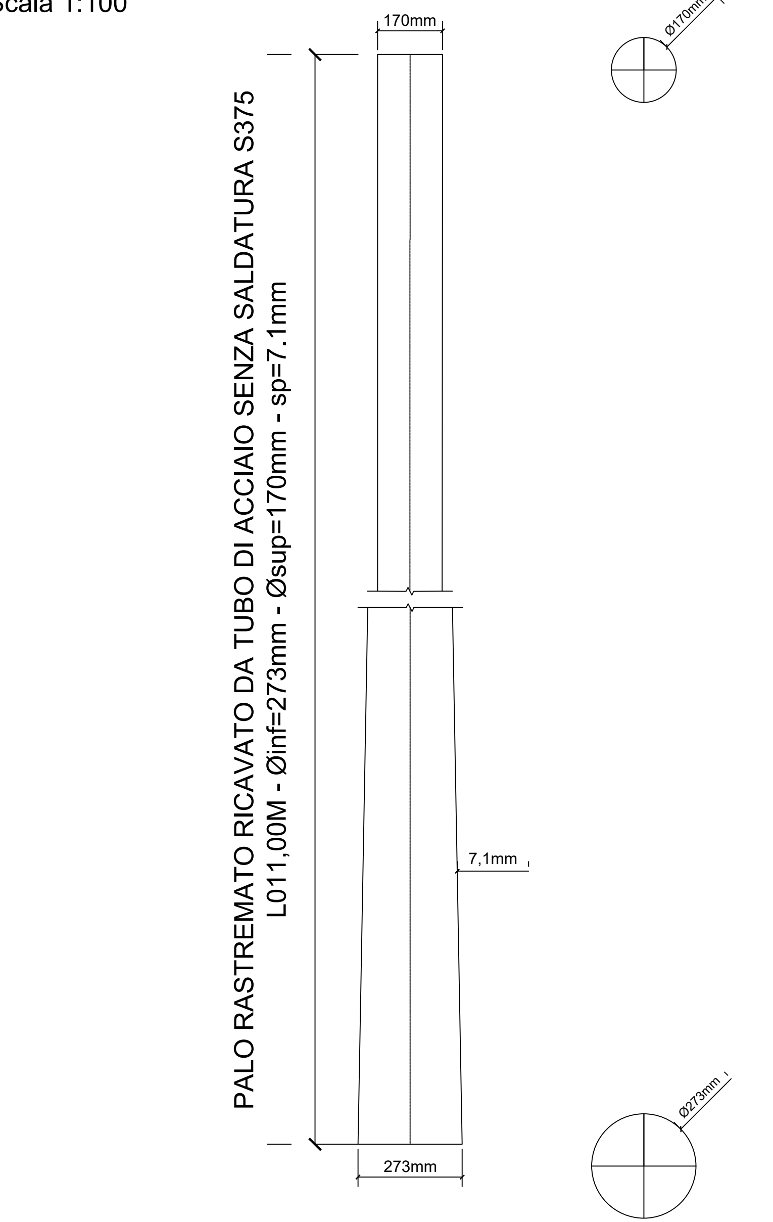
Particolare supporto antenna Scala 1:100
