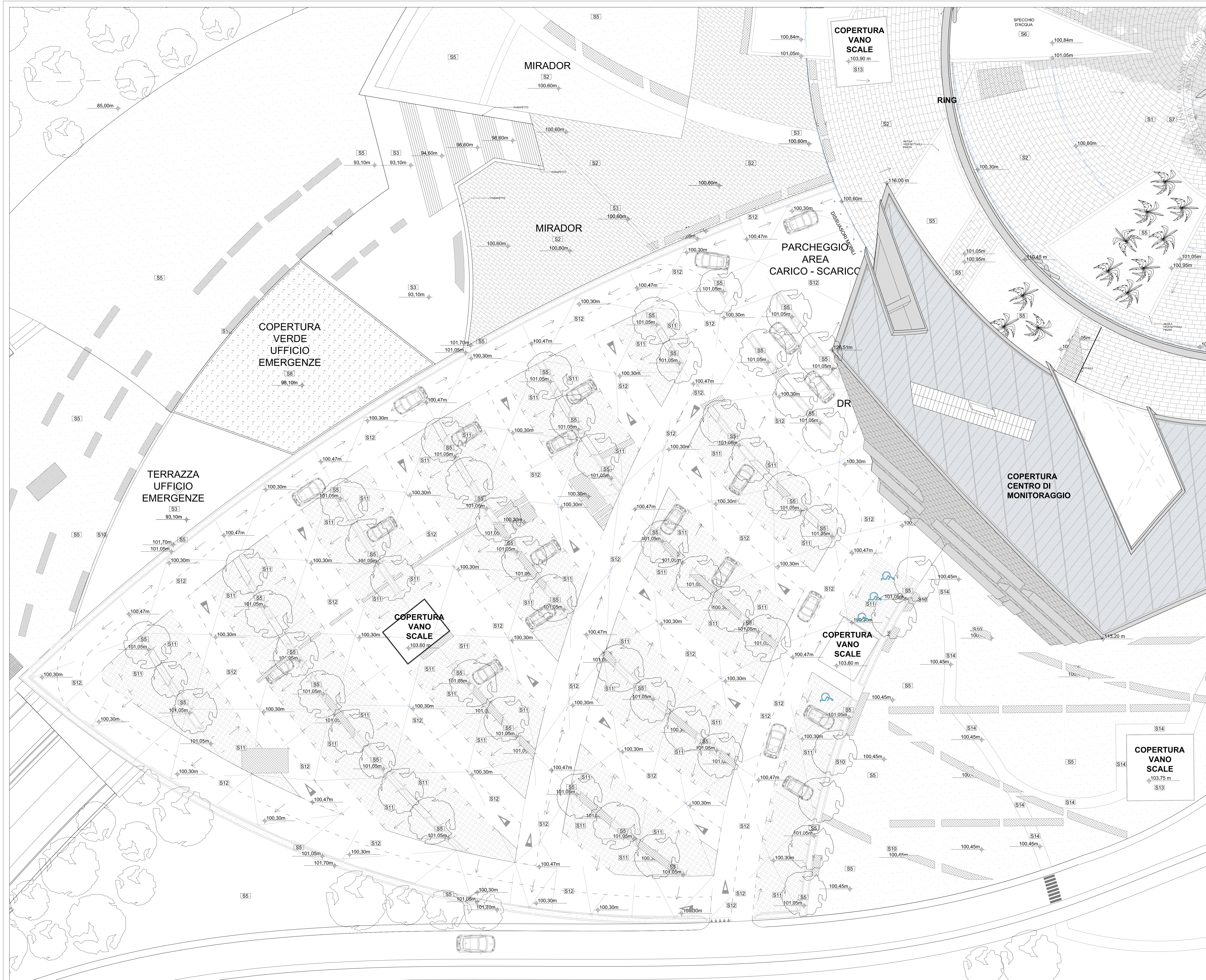
01 PARCHEGGIO A RASO : PIANTA COPERTURE (quota +120.60) 1:200
