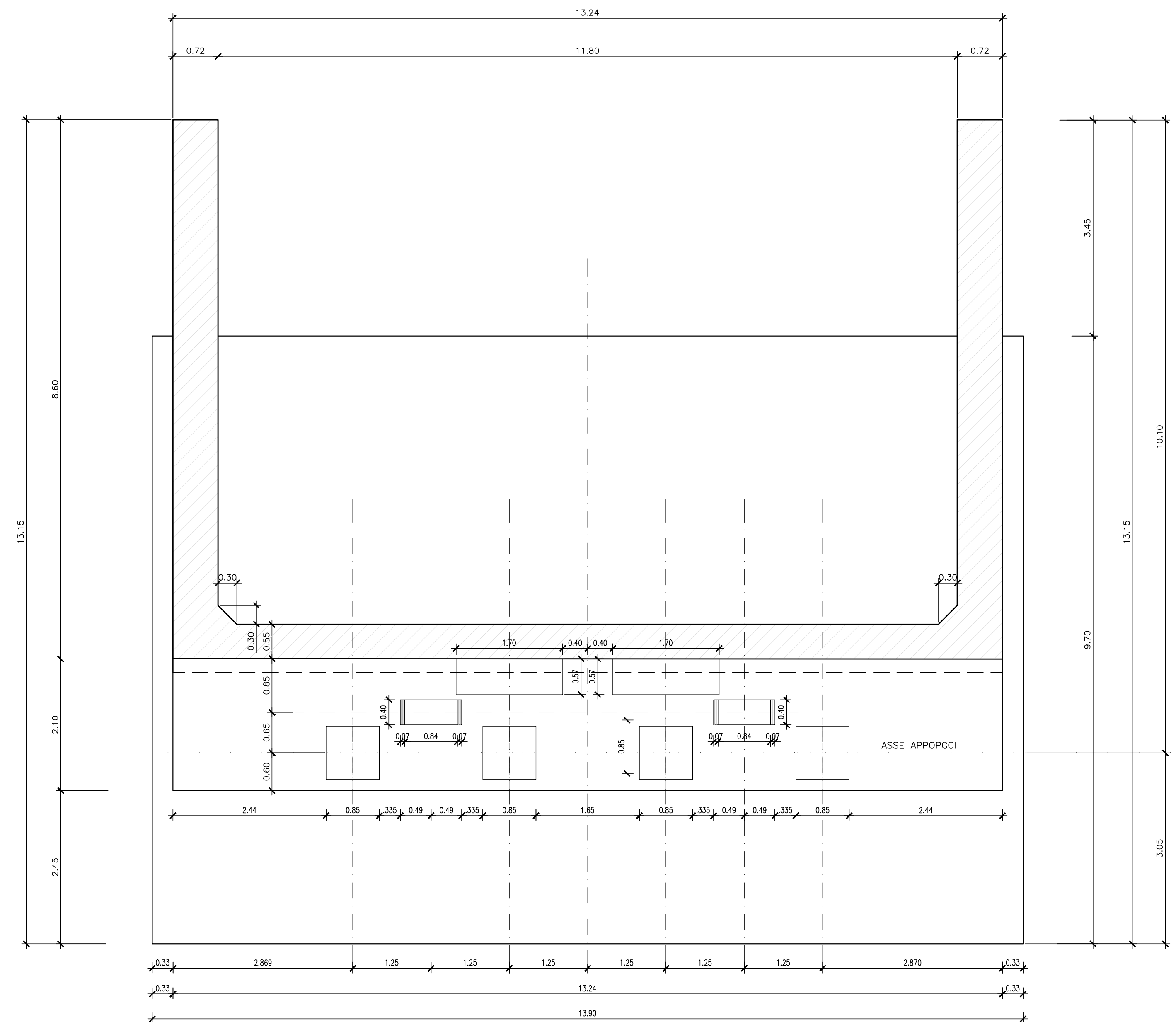
PIANTA A QUOTA APPOGGI SCALA 1:50
