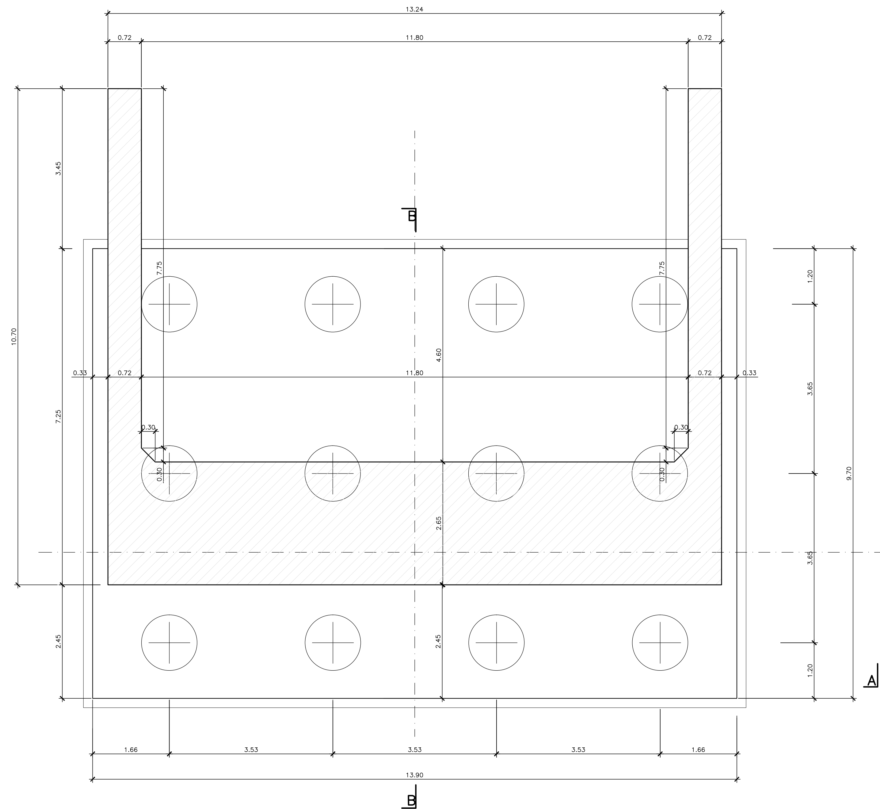
PIANTA FONDAZIONI E SPICCATO SCALA 1:50
