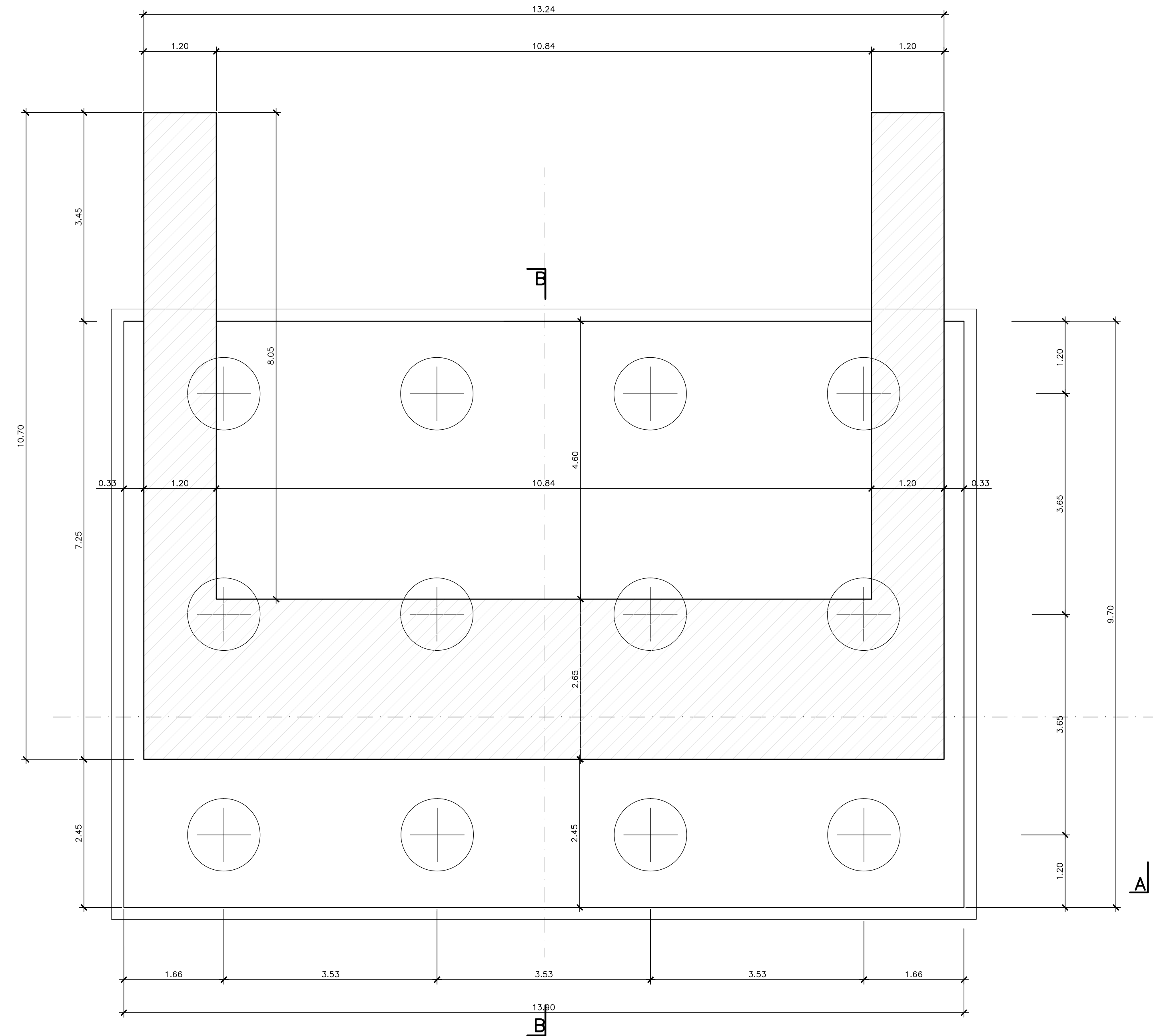
PIANTA FONDAZIONI E SPICCATO SCALA 1:50
