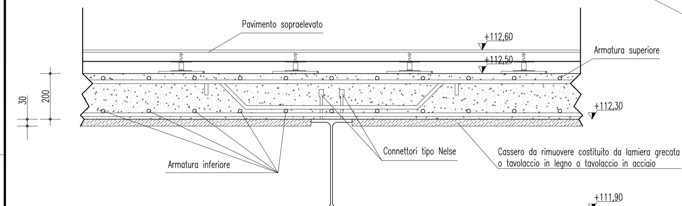
PARTICOLARE SOLAIO SCALA 1:10
