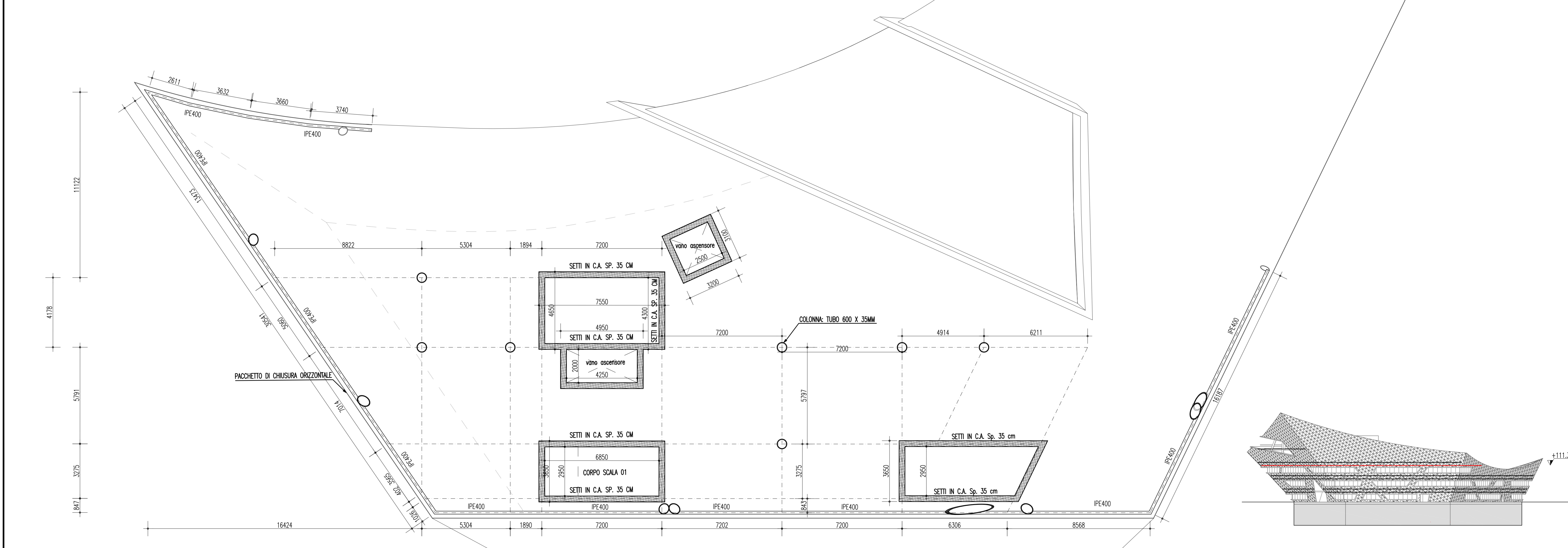
PIANTA CARPENTERIE QUOTA 111,37 S.L.M.
