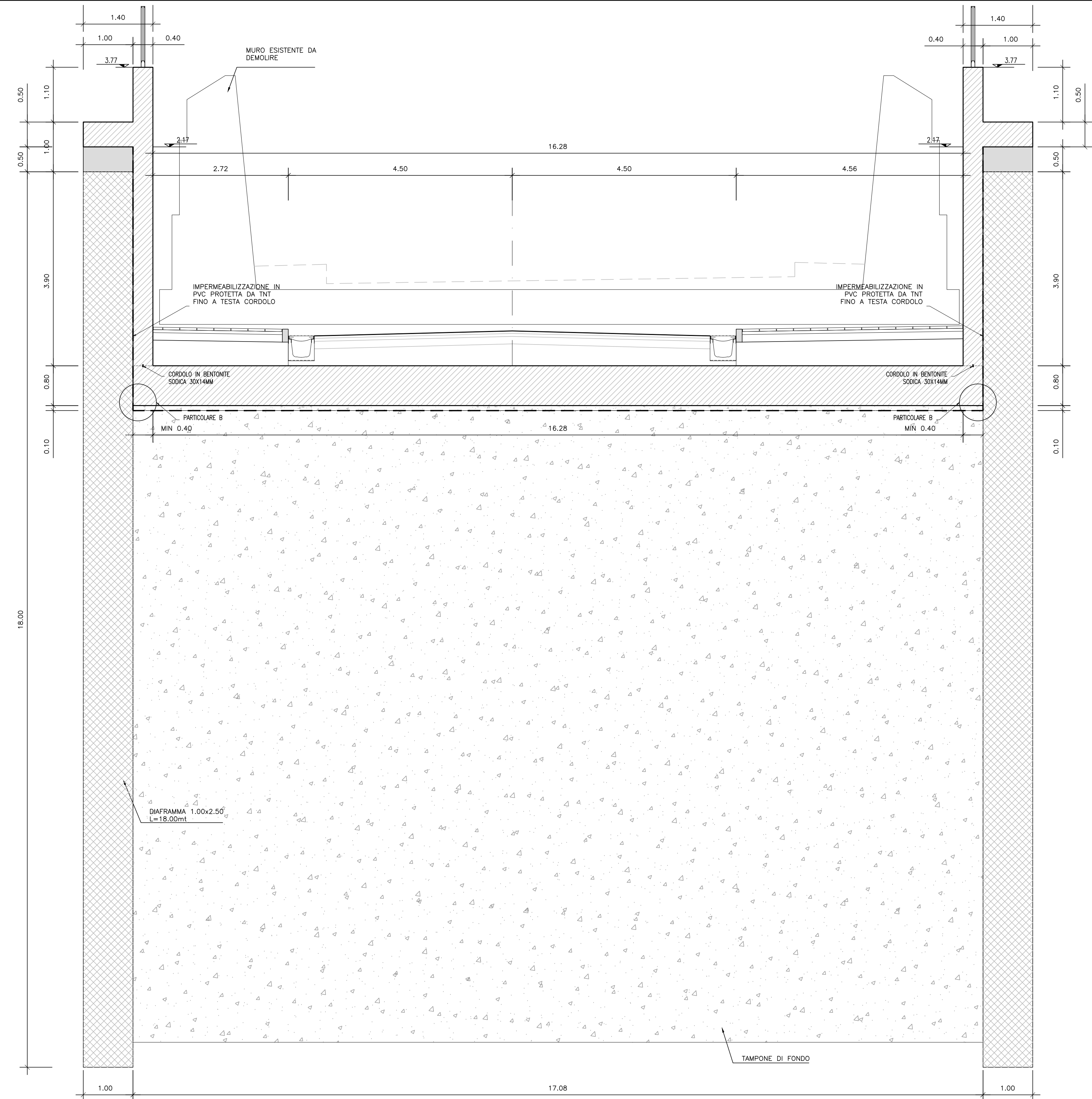
TRATTO "A" SEZIONE A-A SCALA 1:100
