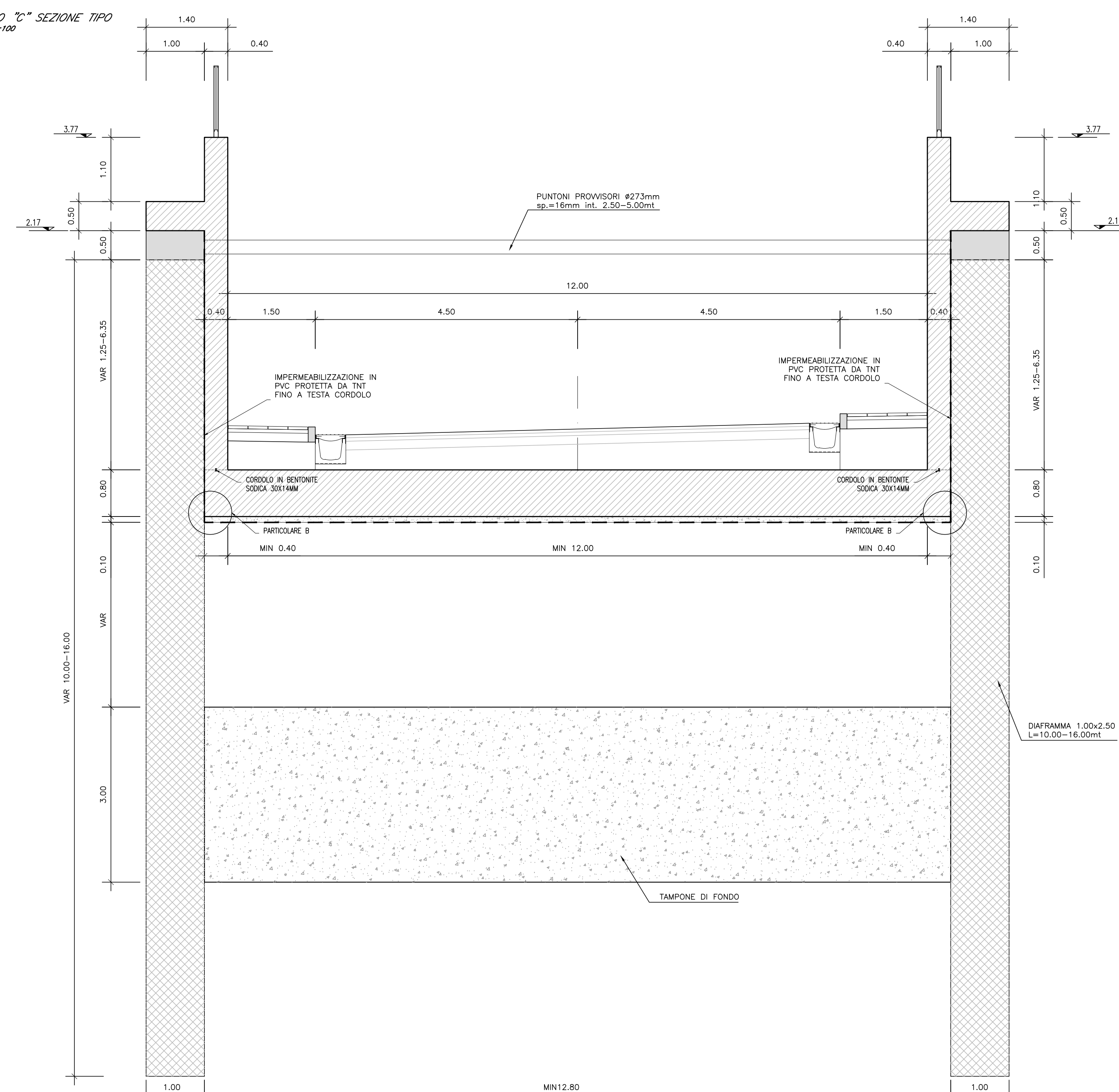
TRATTO "C" SEZIONE TIPO SCALA 1:100
