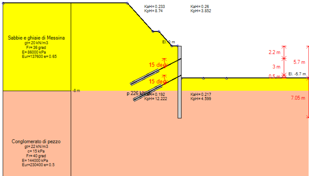
Stage 4 – Inserimento tirante a quota -5.20 m
