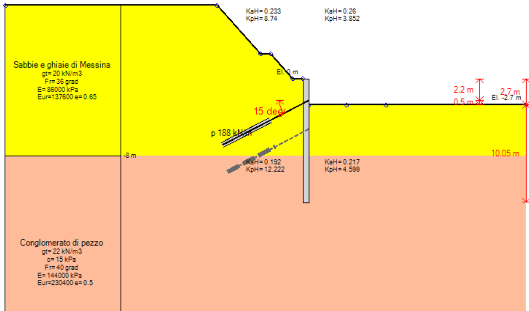
Stage 2 – Inserimento tirante a quota -2.20 m
