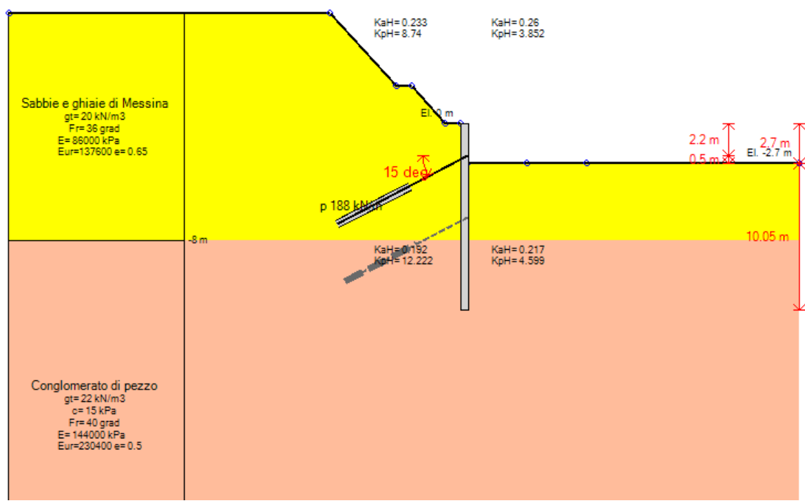
Stage 2 – Inserimento tirante a quota -2.20 m
