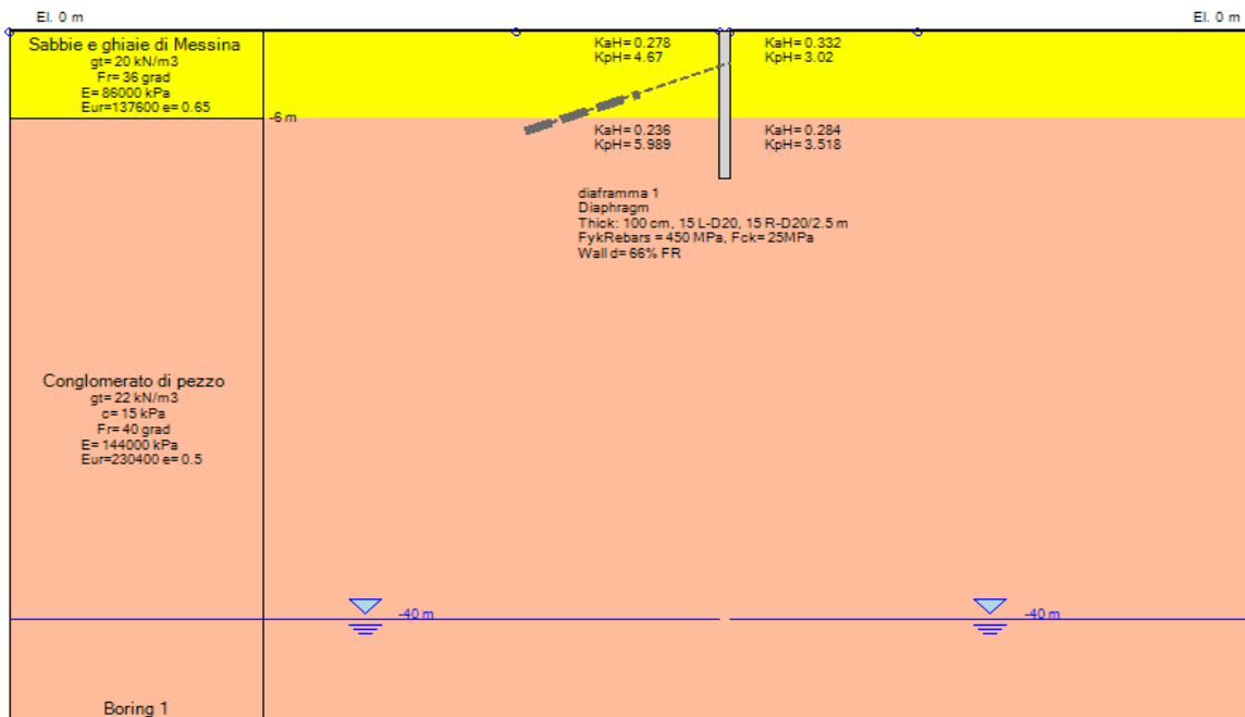
Stage 0 – condizioni iniziali
