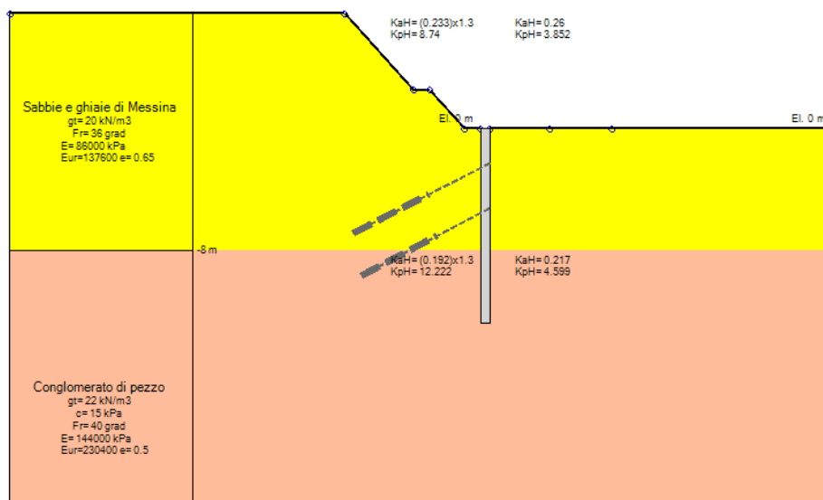
Stage 0 – condizioni iniziali
