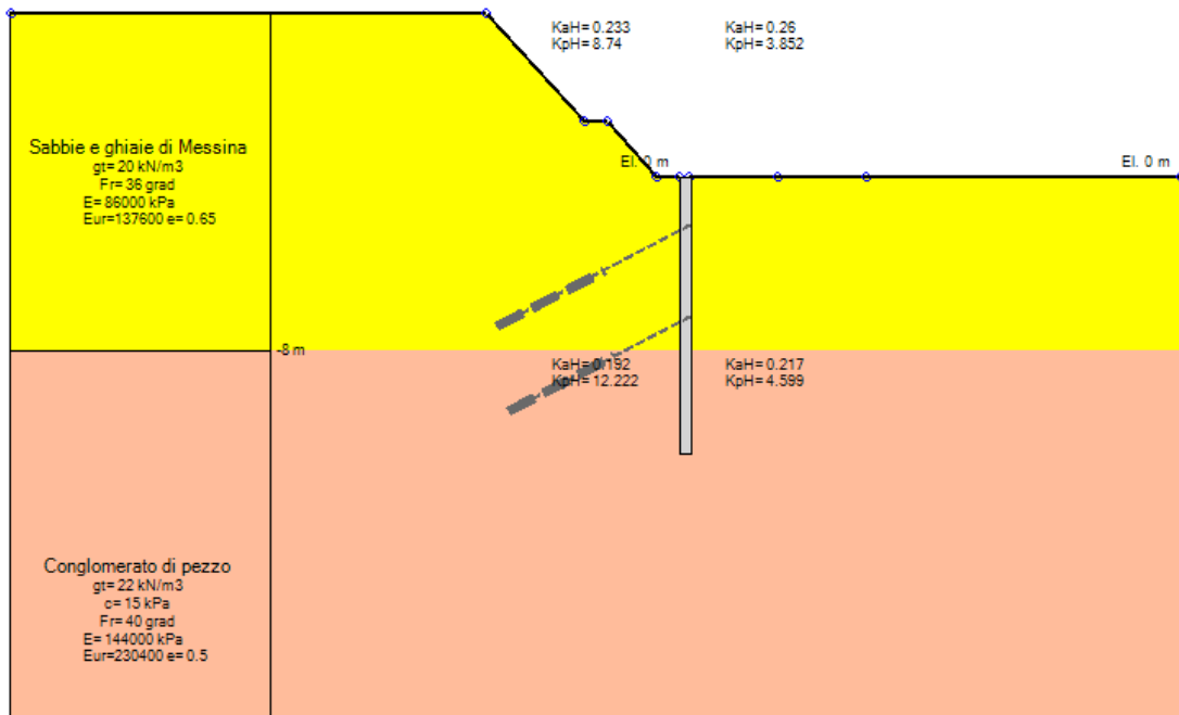
Stage 0 – condizioni iniziali
