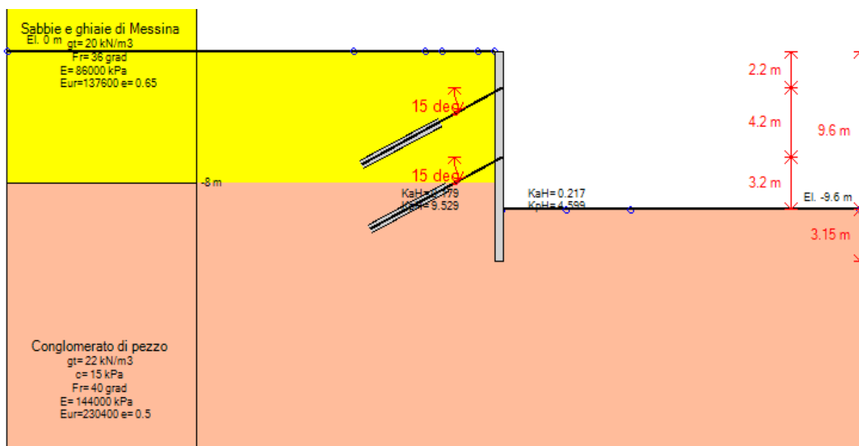
Stage 9 – Scavo a monte quota +0.00 m per realizzazione solettone G.A. asse 1-2
