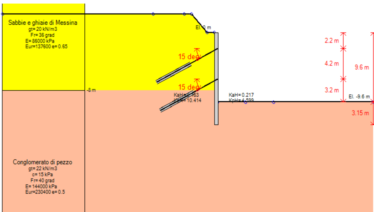
Stage 8 – Scavo a monte quota +2.55 m per realizzazione solettone G.A. asse 1-2
