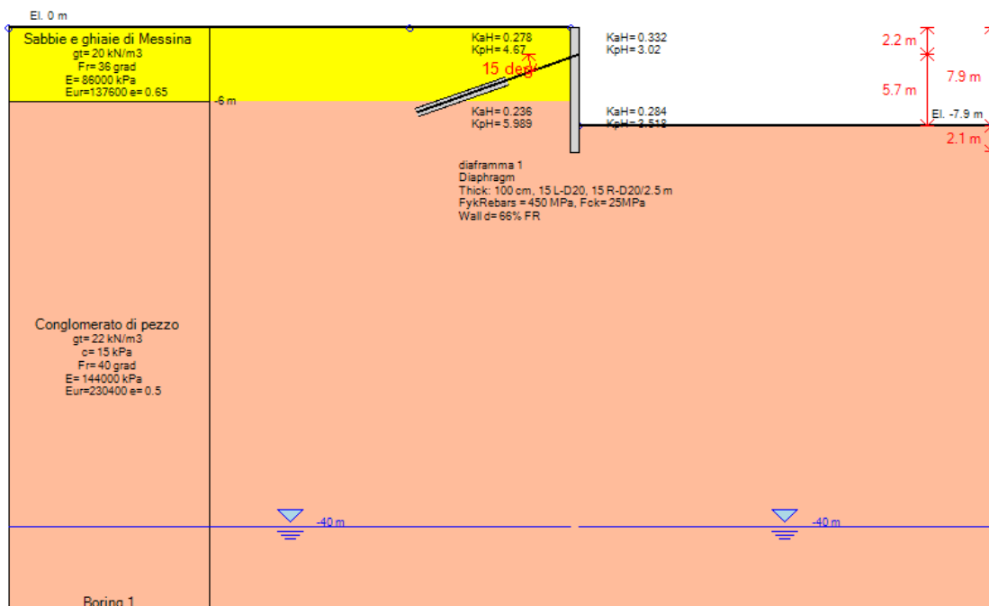
Stage 3 – Scavo fino alla quota 7.90 m
