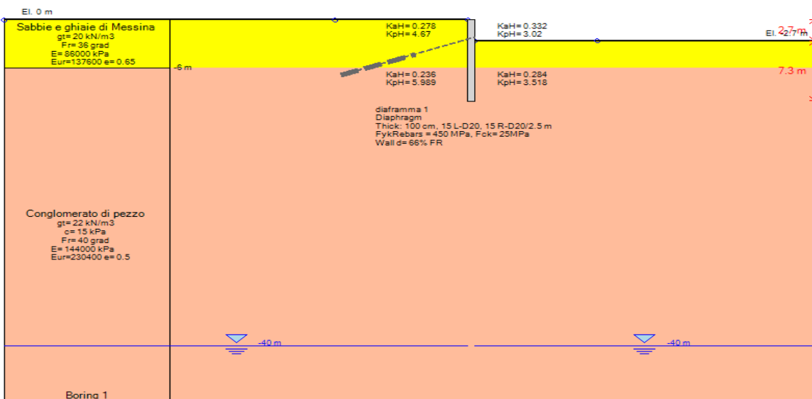
Stage 1 – Scavo fino alla quota 2.70 m
