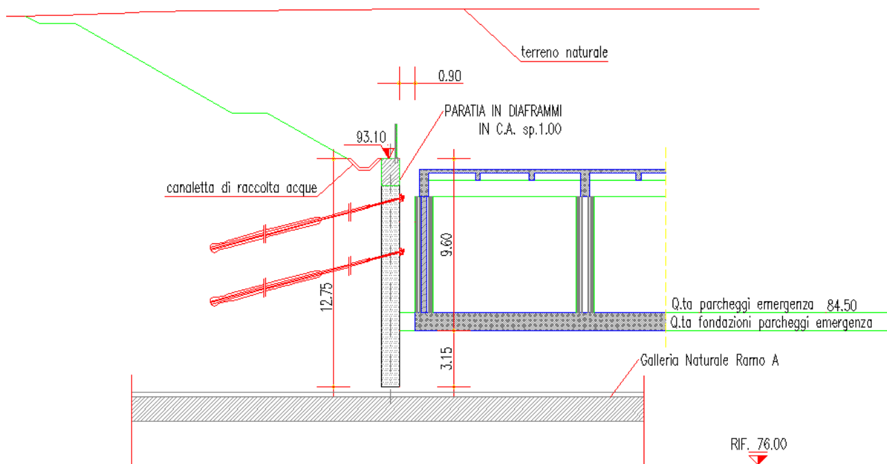
Figura 4.2: Sezione tipo della paratia
