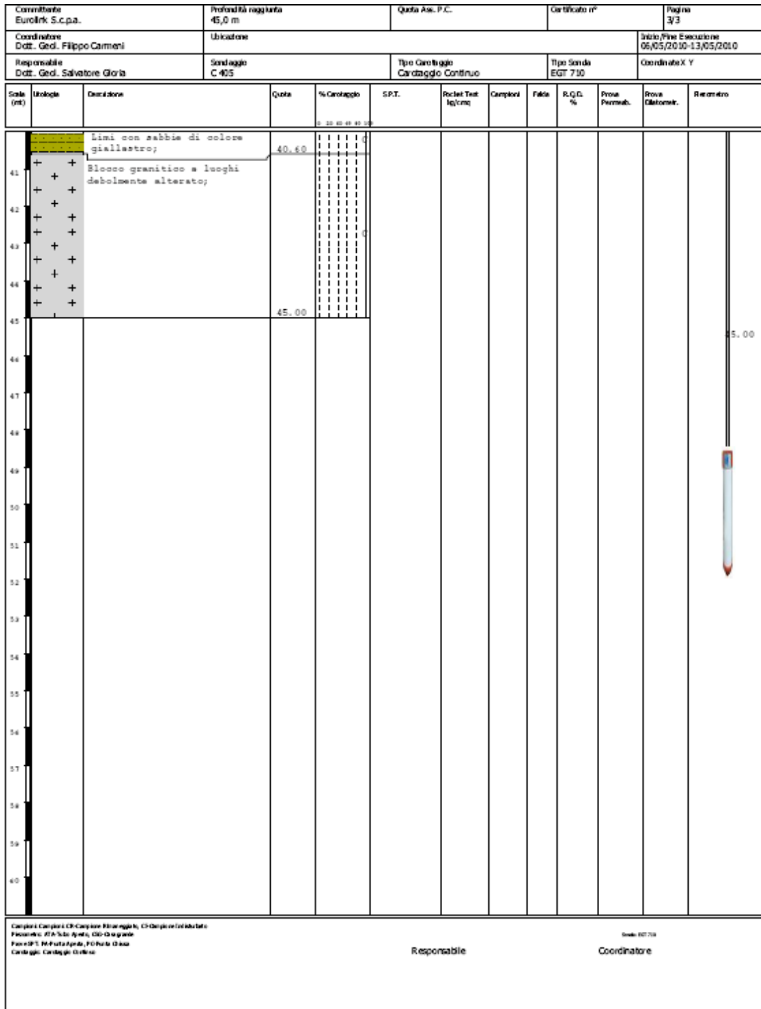
Figura 5.2: Sondaggio C405
