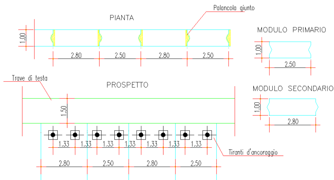
Figura 4.1: Dettaglio pannelli
