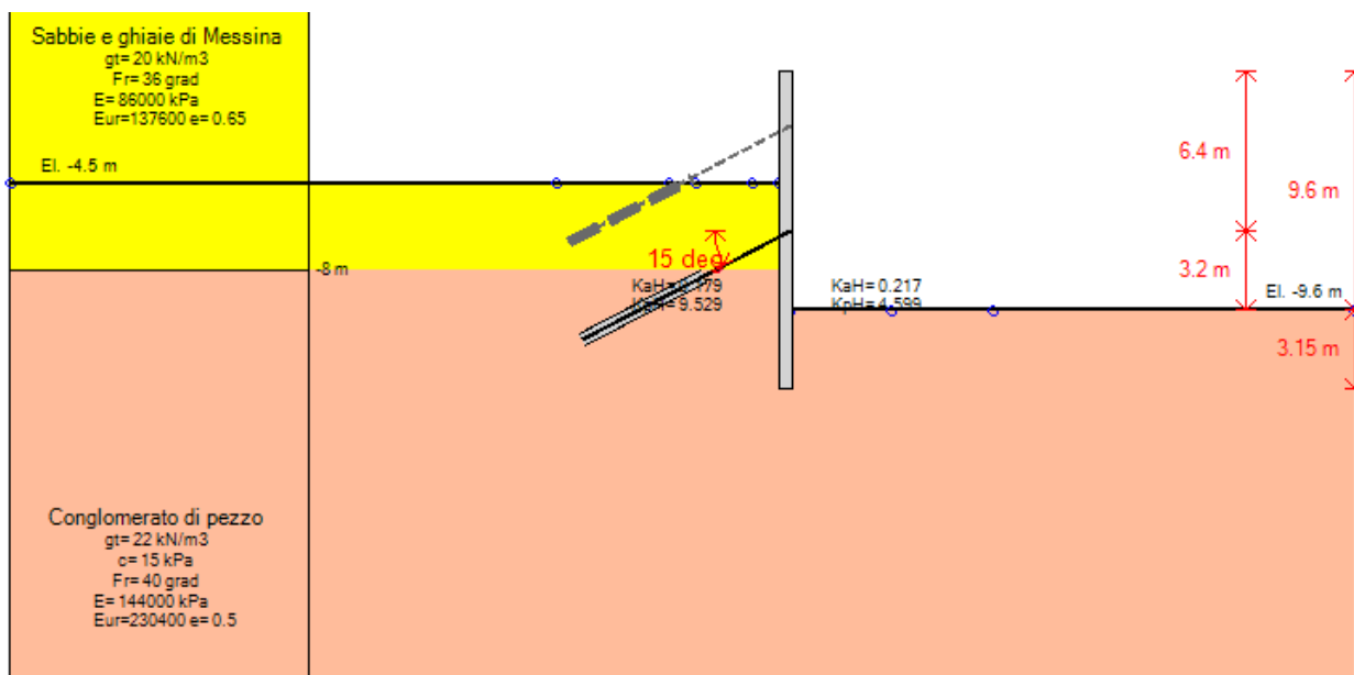
Stage 10 – Scavo finale a monte quota -4.50 m per realizzazione solettone G.A. asse 1-2 ed eliminazione primo ordine di tiranti
