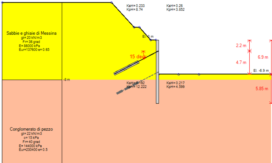
Stage 4 – Scavo a quota -6.90 m
