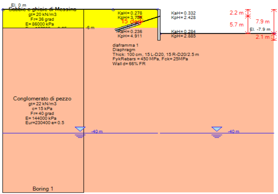
Stage 4 –Azione del sisma
