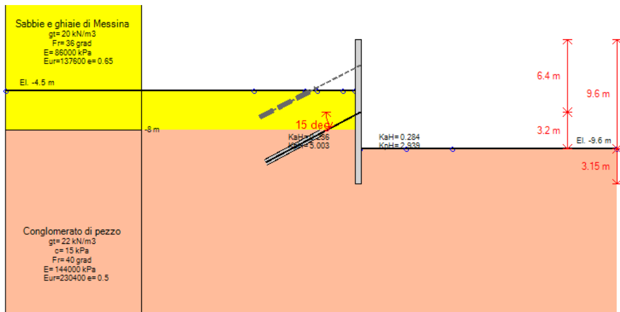
Stage 11 – Azione del sisma
