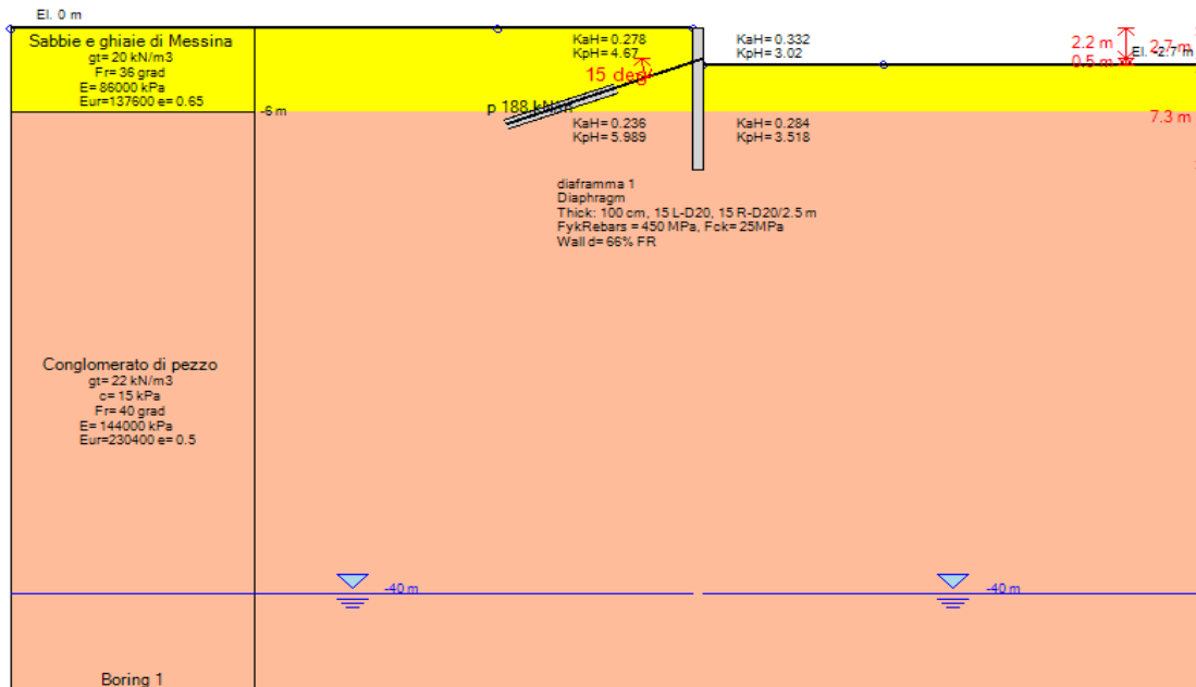
Stage 2 – Inserimento tirante a quota -2.20 m
