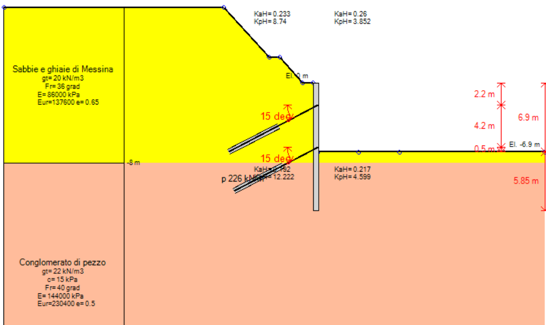
Stage 5 – Inserimento tirante a quota -6.40 m
