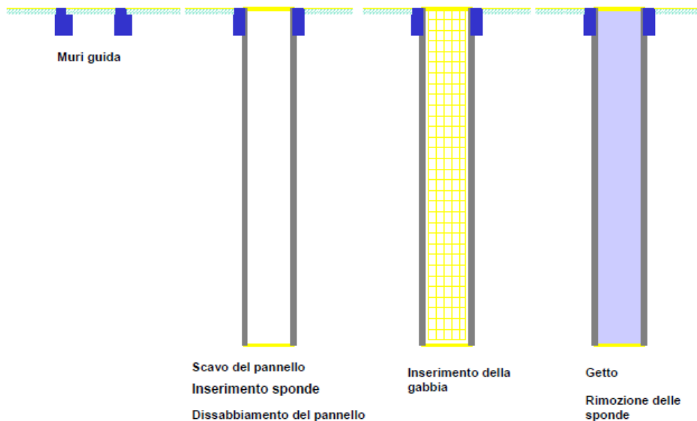
Figura 6.2: Fasi costruttive dei diaframmi
