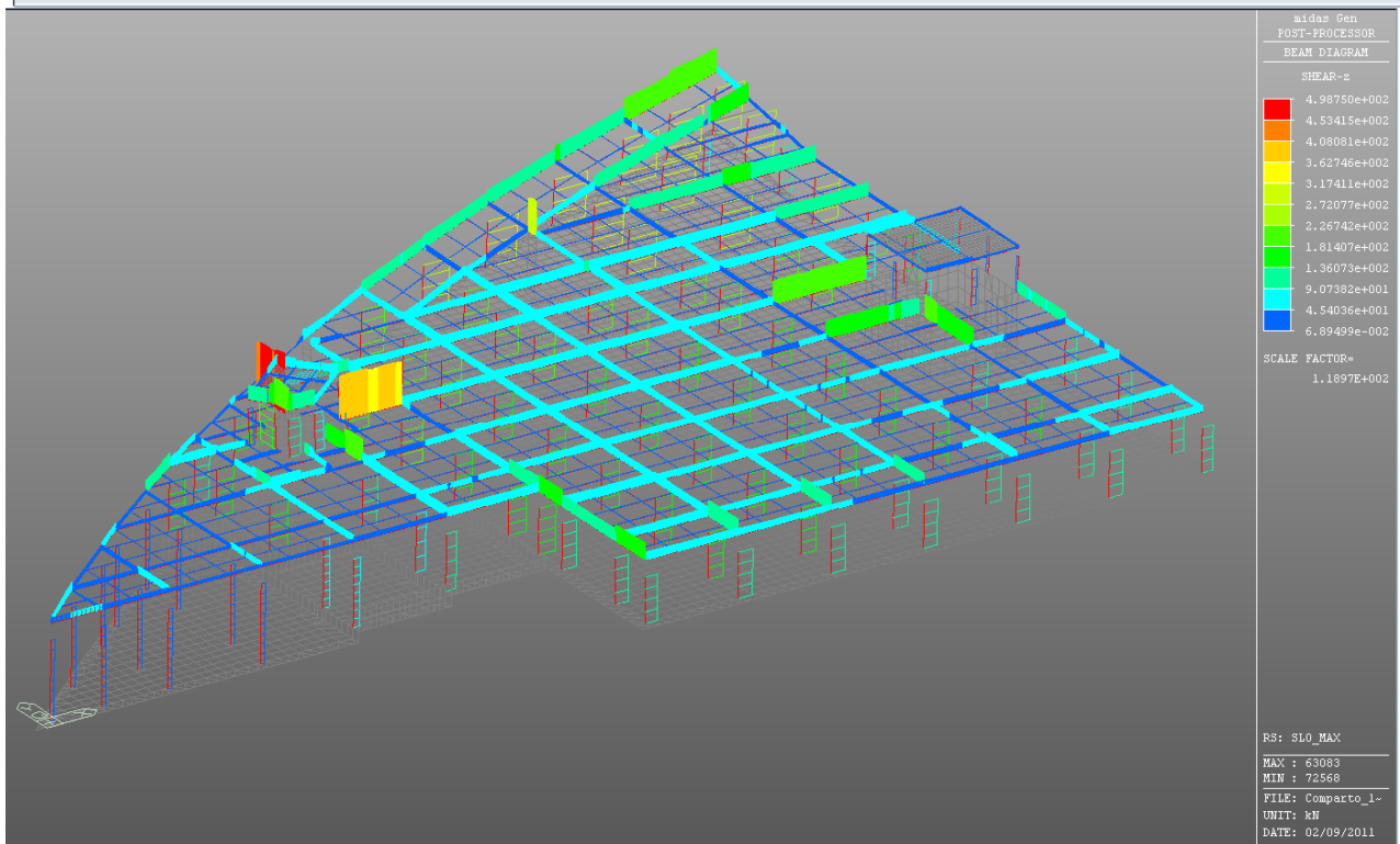
Figura 6.30: SLO max – Valore del taglio
