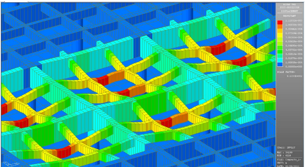
Figura 6.5: Deformate per effetto dei carico mobile in dir. Y – Q1 (inviol. max e min spostamenti)
