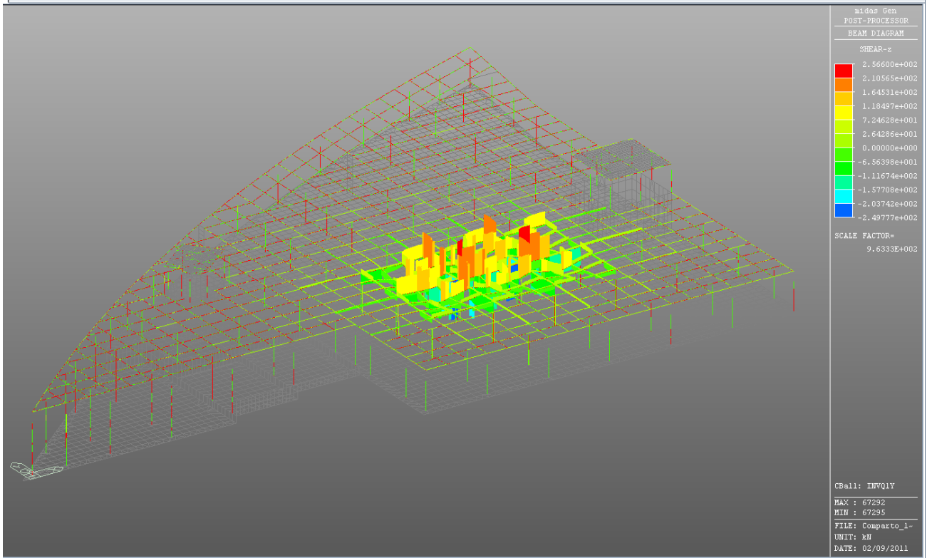
Figura 6.26: Caso di carico Q1 (traffico) in dir Y – Valore del taglio
