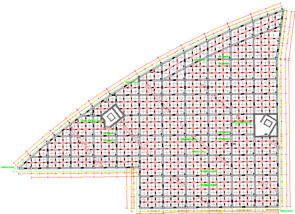
Figura 4.1: Carpenteria del primo impalcato del corpo n. 7
