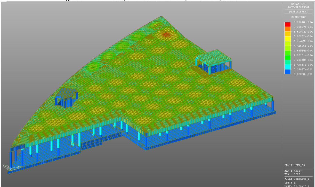
Figura 6.3: Deformate per effetto dei carico della folla compatta – Q5 (invil. max e min spostamenti)
