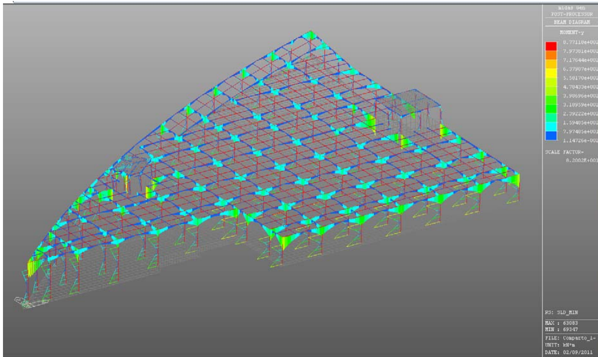
Figura 6.16: SLD min – Valore del momento flettente
