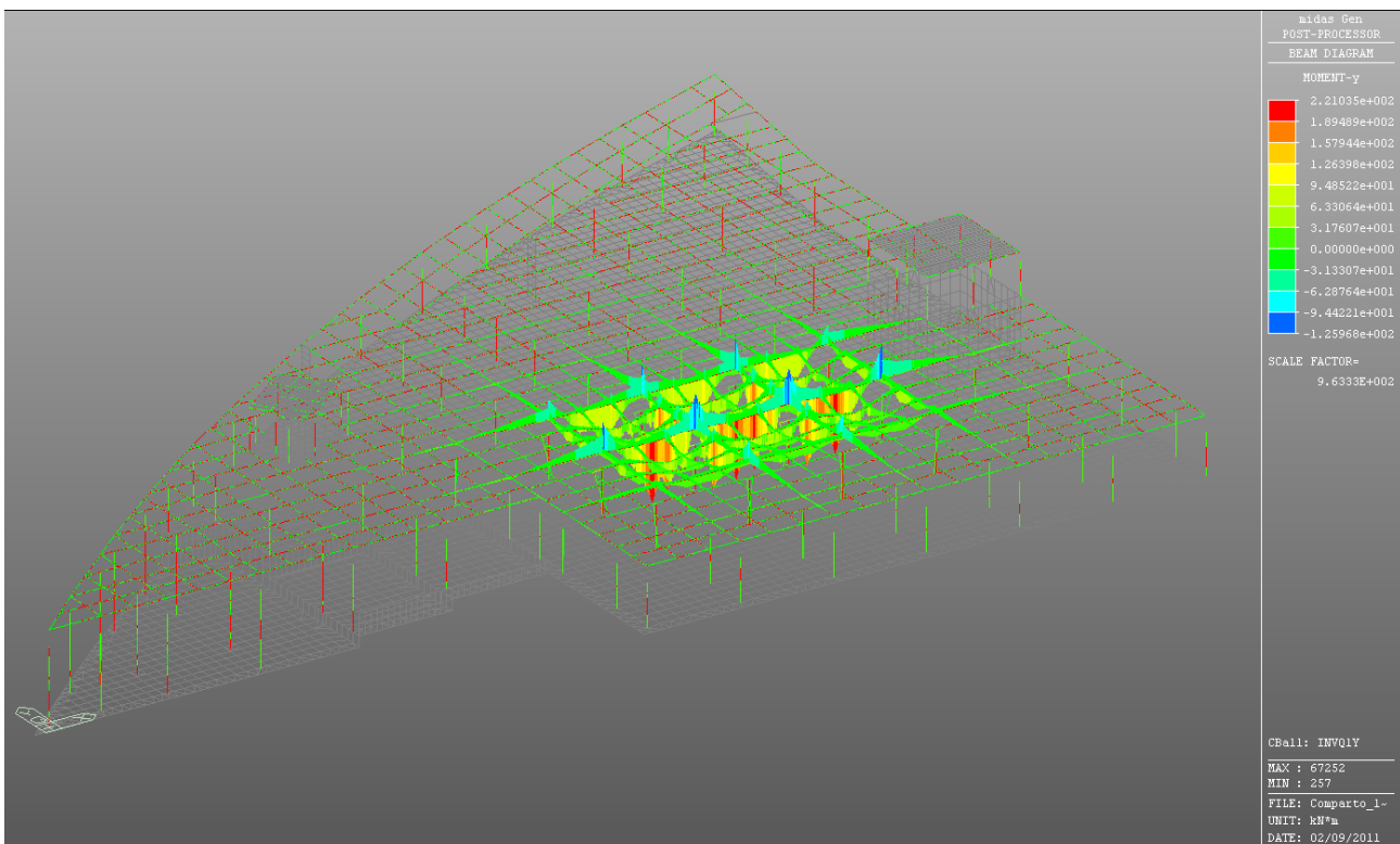
Figura 6.13: Caso di carico Q1 (traffico) in dir Y – Valore del momento flettente
