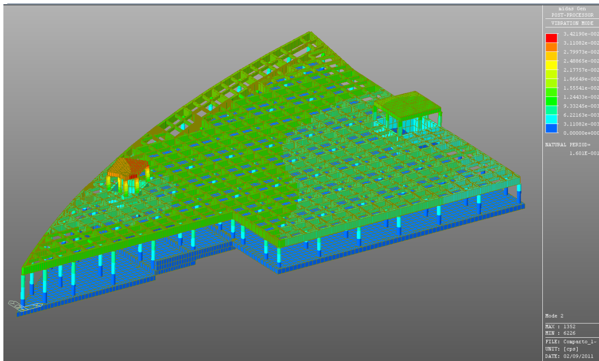
Figura 6.7: Modo di vibrare n. 2
