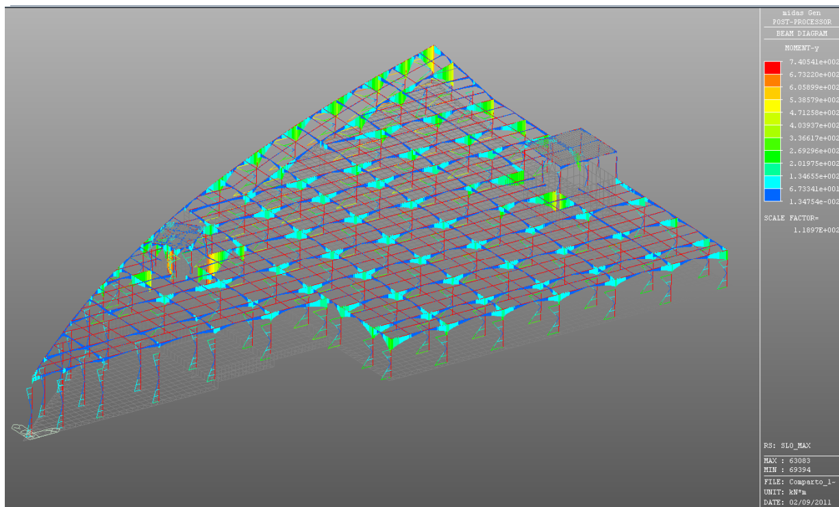
Figura 6.17: SLO max – Valore del momento flettente
