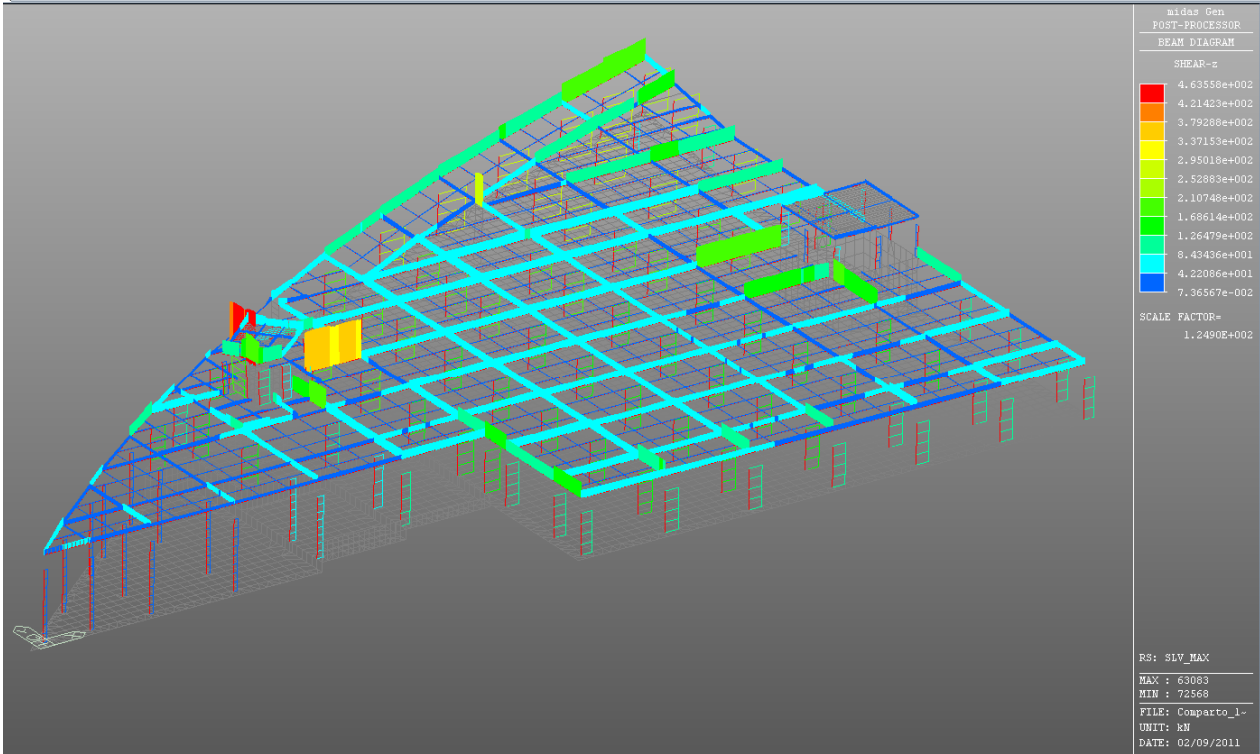
Figura 6.32: SLV max – Valore del taglio
