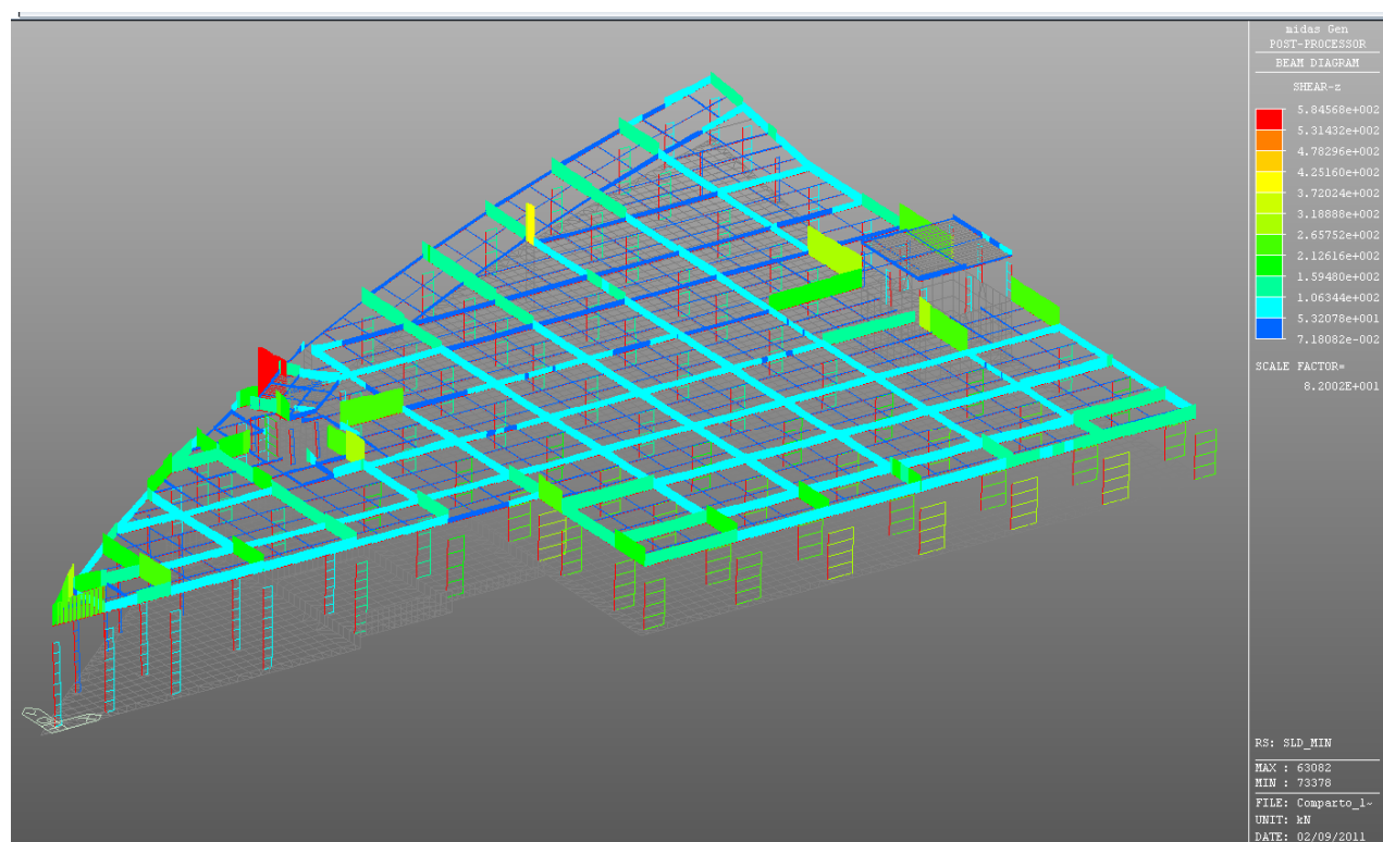
Figura 6.29: SLD min – Valore del taglio
