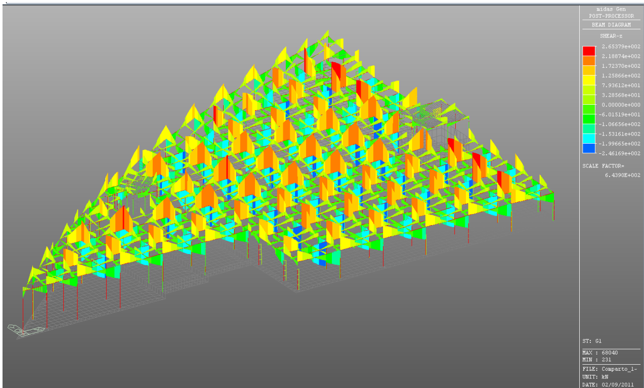
Figura 6.23: Caso di carico G1 – Valore del taglio
