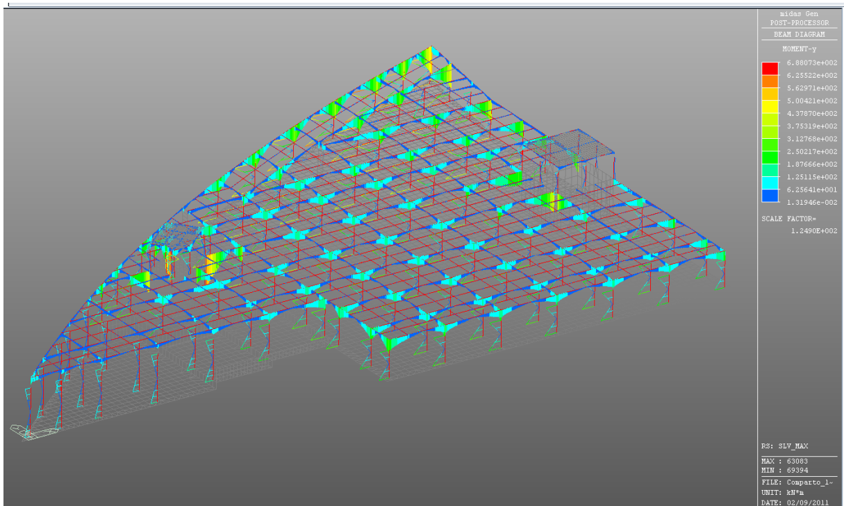
Figura 6.19: SLV max – Valore del momento flettente
