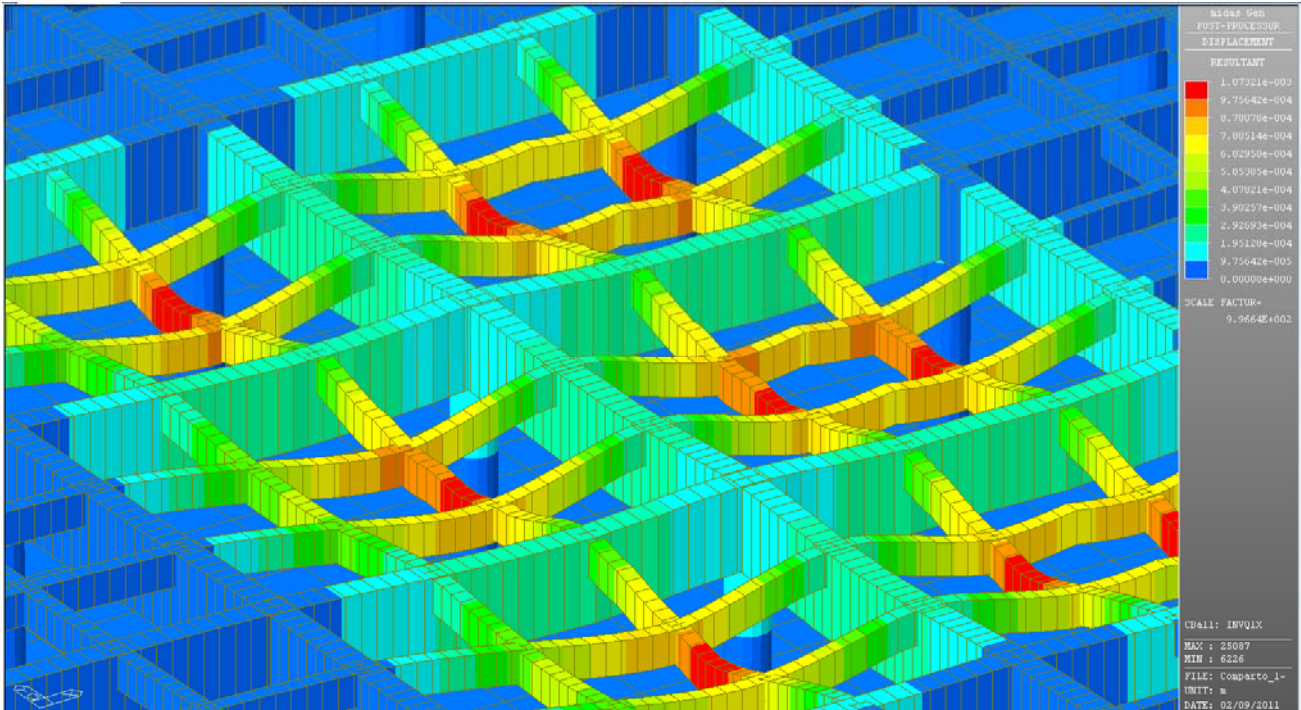
Figura 6.4: Deformate per effetto dei carico mobile in dir. X – Q1 (inviol. max e min spostamenti)
