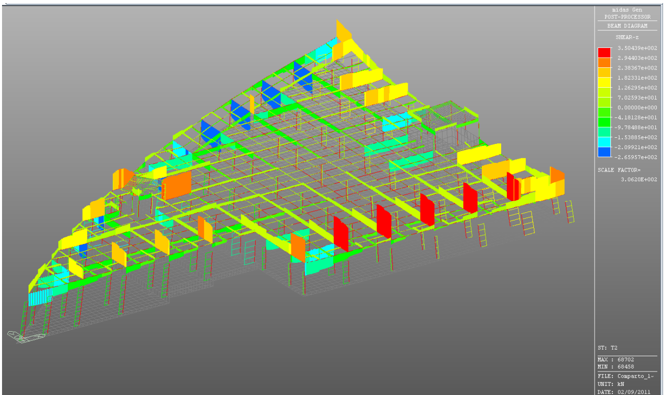
Figura 6.35: Caso di carico T2 (termico) – Valore del taglio
