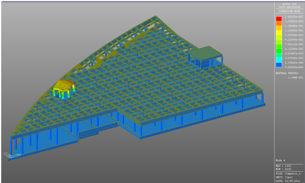
Figura 6.9: Modo di vibrare n. 4
