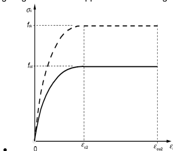
• Figura 3.1 – Legame costitutivo del calcestruzzo
