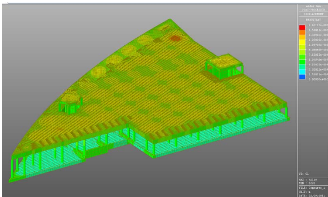
Figura 6.1: Deformate per effetto dei pesi propri strutturali – G1
