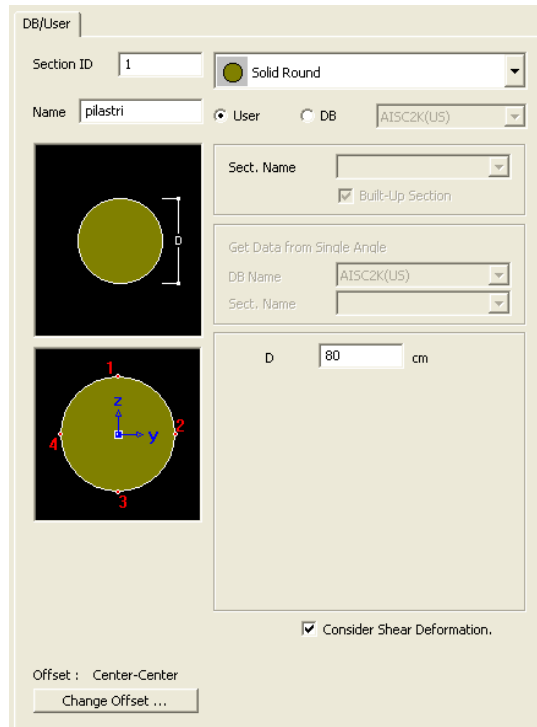
Figura 4.18:Caratteristiche geometriche delle sezioni trasversali dei pilastri
