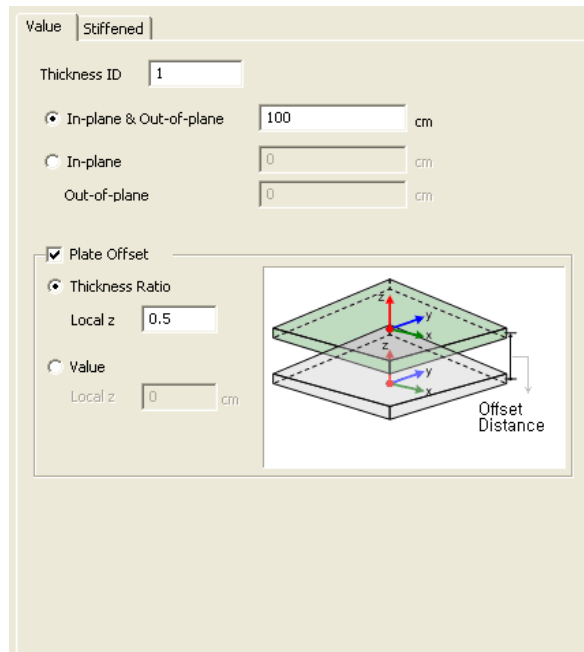
Figura 4.20: Caratteristiche geometriche delle solette
