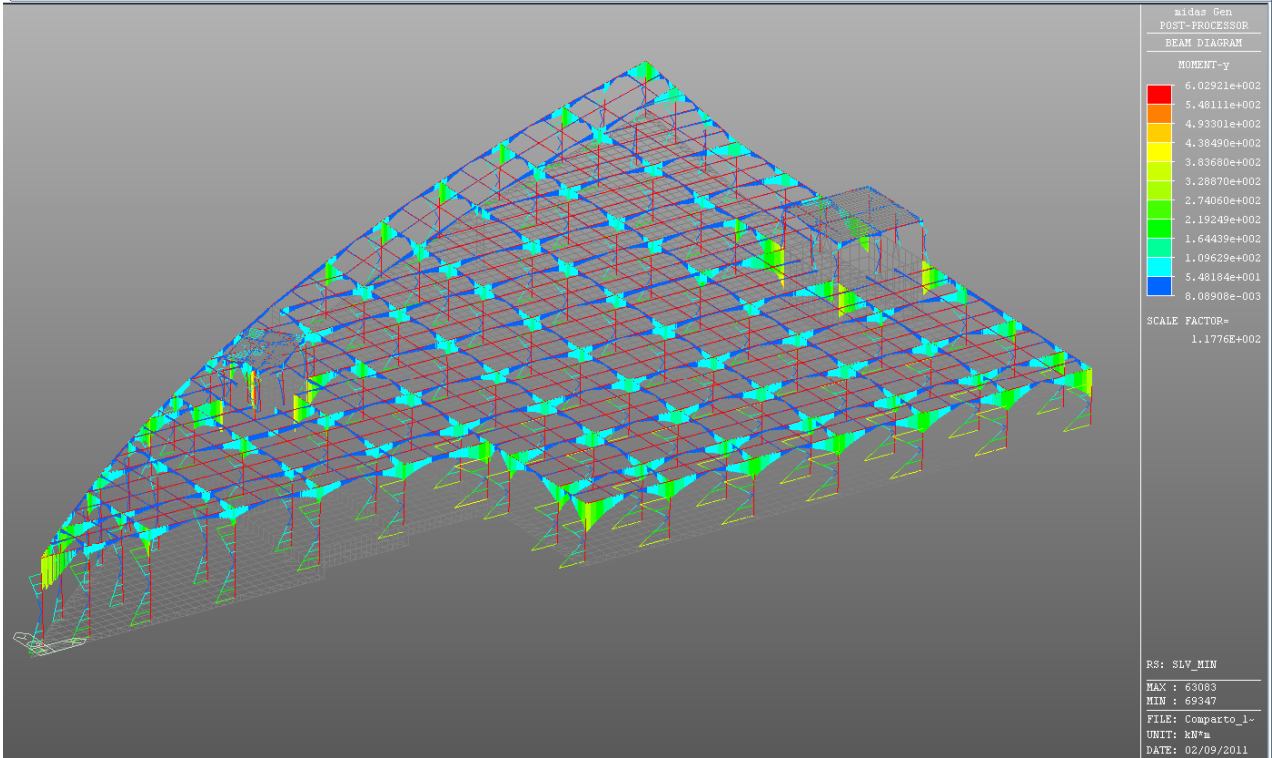
Figura 6.20: SLV min – Valore del momento flettente
