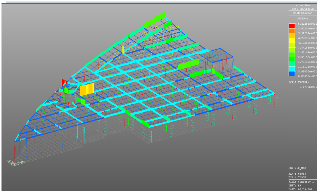
Figura 6.28: SLD max – Valore del taglio
