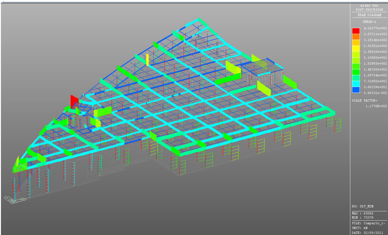
Figura 6.33: SLV min – Valore del taglio
