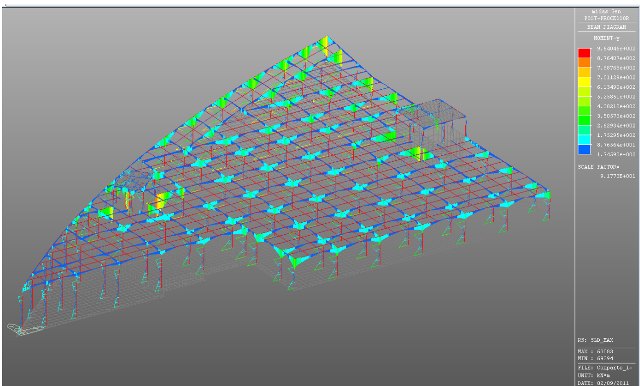
Figura 6.15: SLD max – Valore del momento flettente
