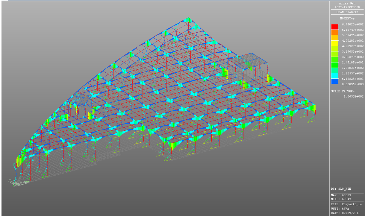
Figura 6.18: SLO min – Valore del momento flettente
