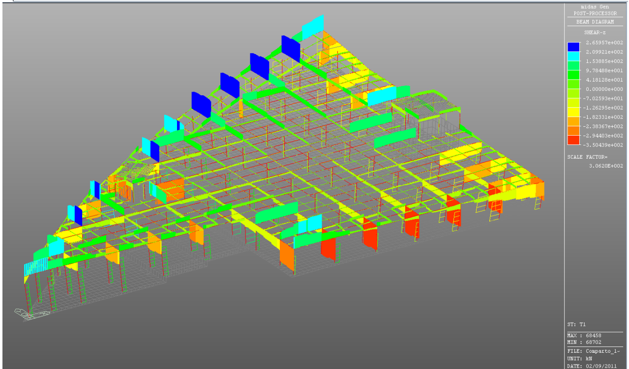
Figura 6.34: Caso di carico T1 (termico) – Valore del taglio
