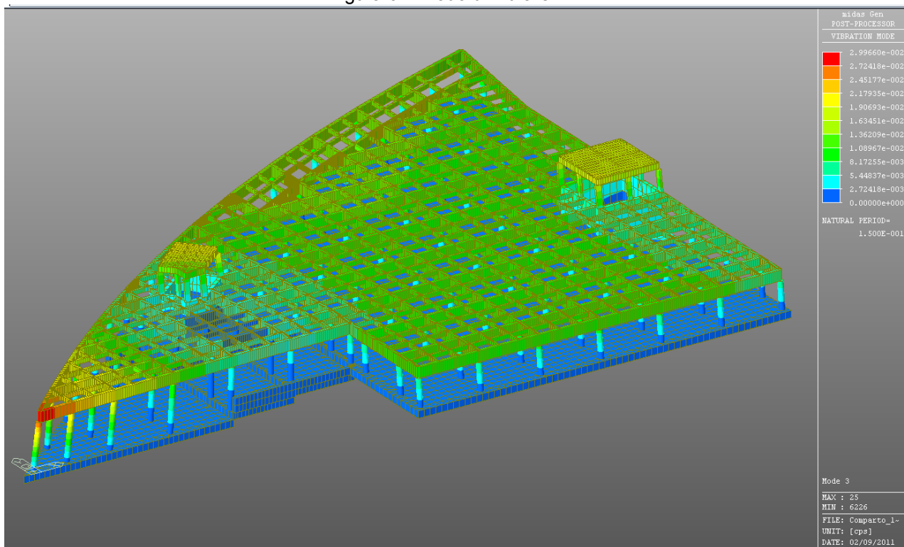
Figura 6.8: Modo di vibrare n. 3
