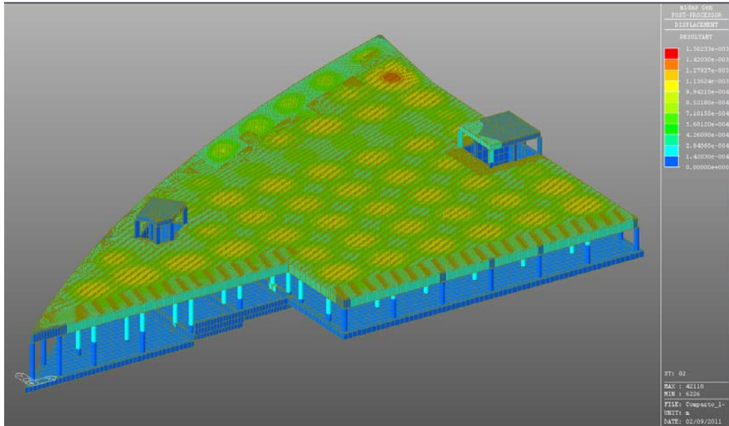
Figura 6.2: Deformate per effetto dei carichi permanenti portati – G2
