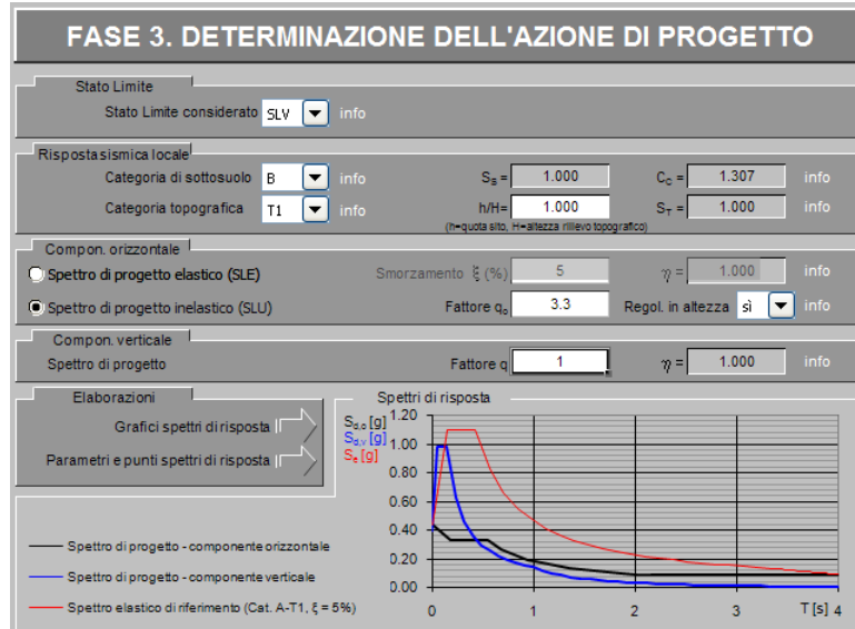
Figura 4.11: Determinazione dello spettro di progetto relativo allo SLV
