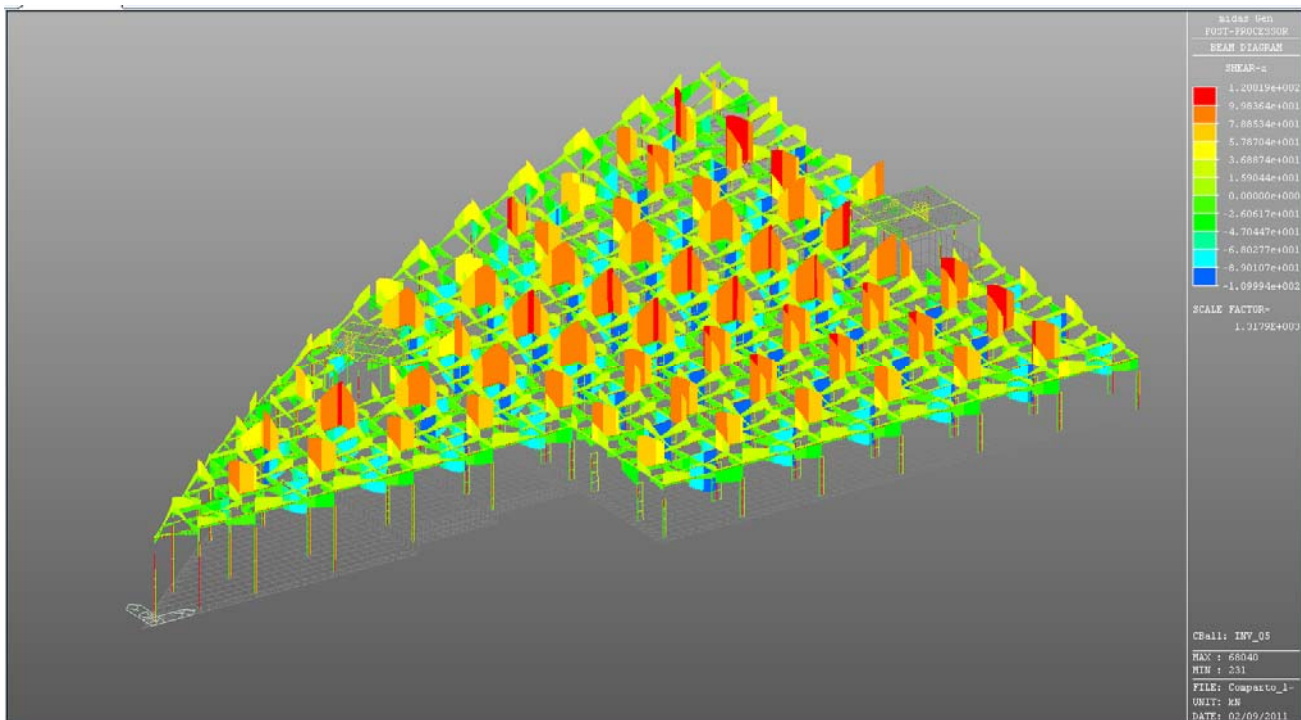
Figura 6.27: Involuppo del carico Q5 (folla) – valore del taglio
