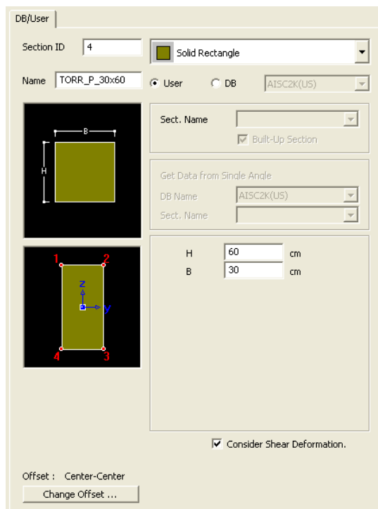
Figura 4.19:Caratteristiche geometriche delle sezioni trasversali dei pilastri del torrino
