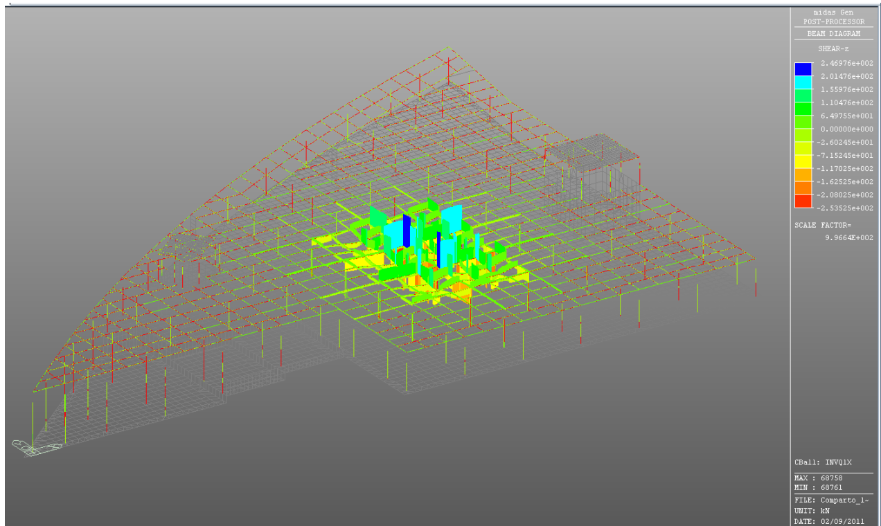
Figura 6.25: Caso di carico Q1 (traffico) in dir X – Valore del taglio
