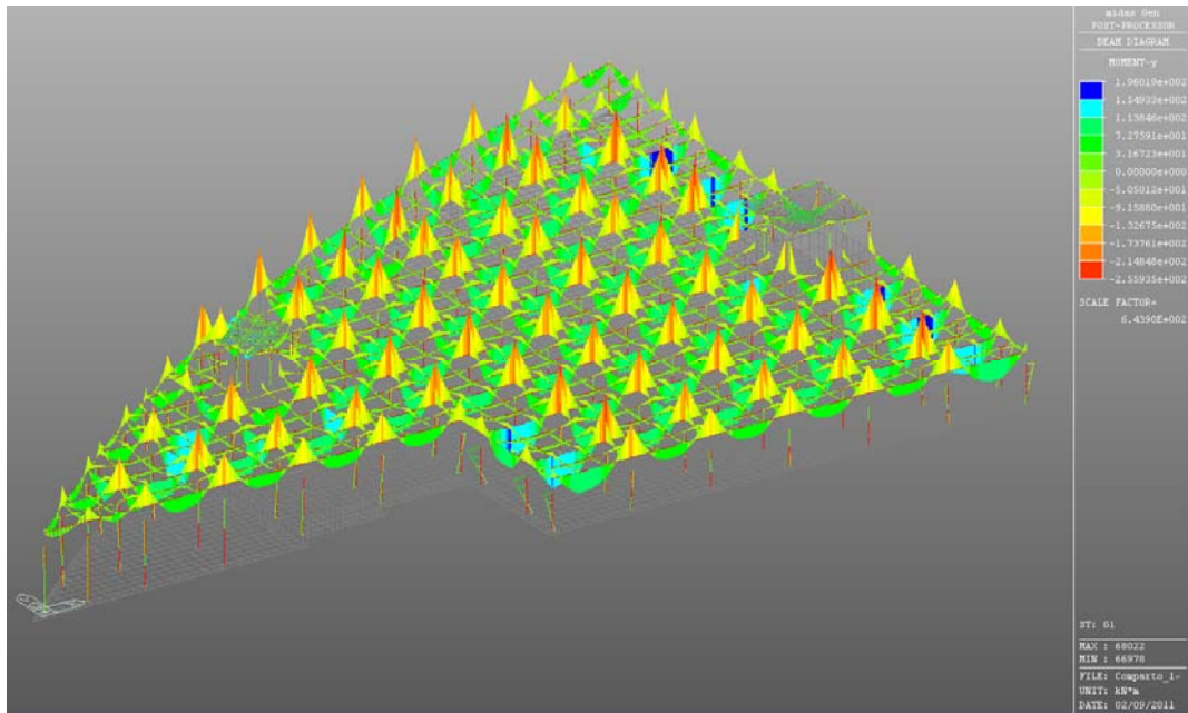
Figura 6.10: Caso di carico G1 – Valore del momento flettente
