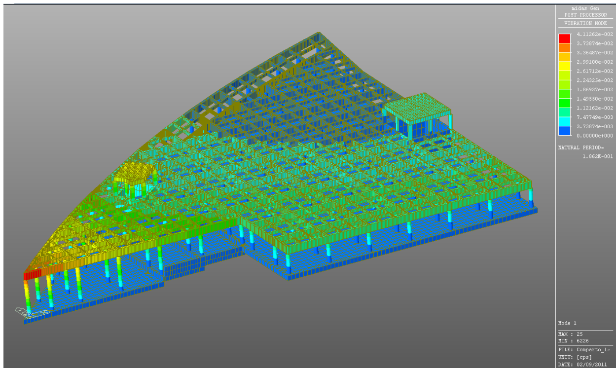
Figura 6.6: Modo di vibrare n. 1
