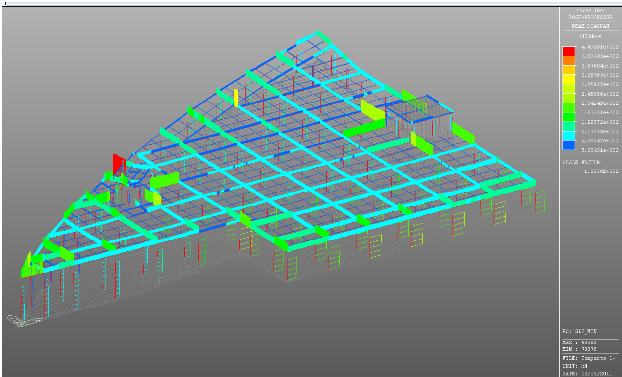
Figura 6.31: SLO min – Valore del taglio
