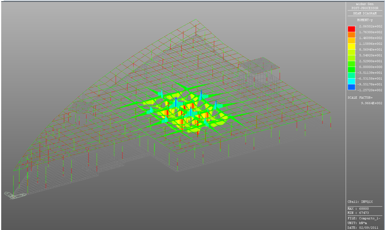
Figura 6.12: Caso di carico Q1 (traffico) in dir X – Valore del momento flettente
