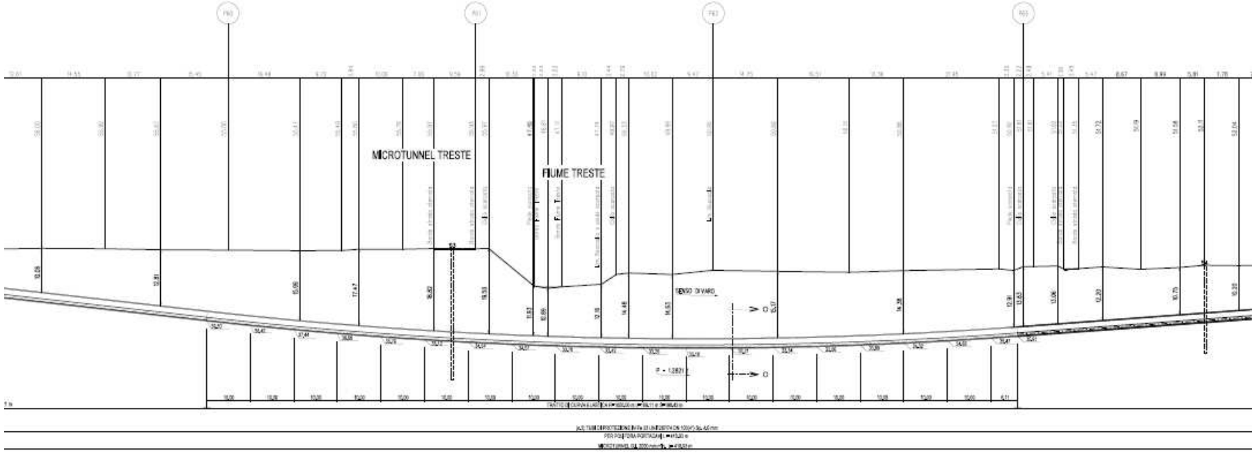
Figura 5: attraversamento Fiume Treste - Sezione schematica di progetto
