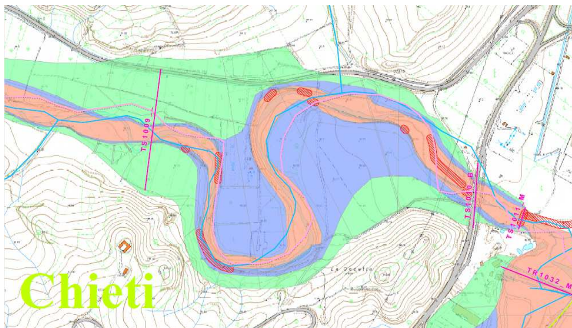
Figura 2: stralcio cartografia PAI con evidenziate le sezioni ove sono state calcolate le portate di riferimento. Nel caso di interesse l'attraversamento in progetto cade tra le sezioni TS1009 e TS1010
