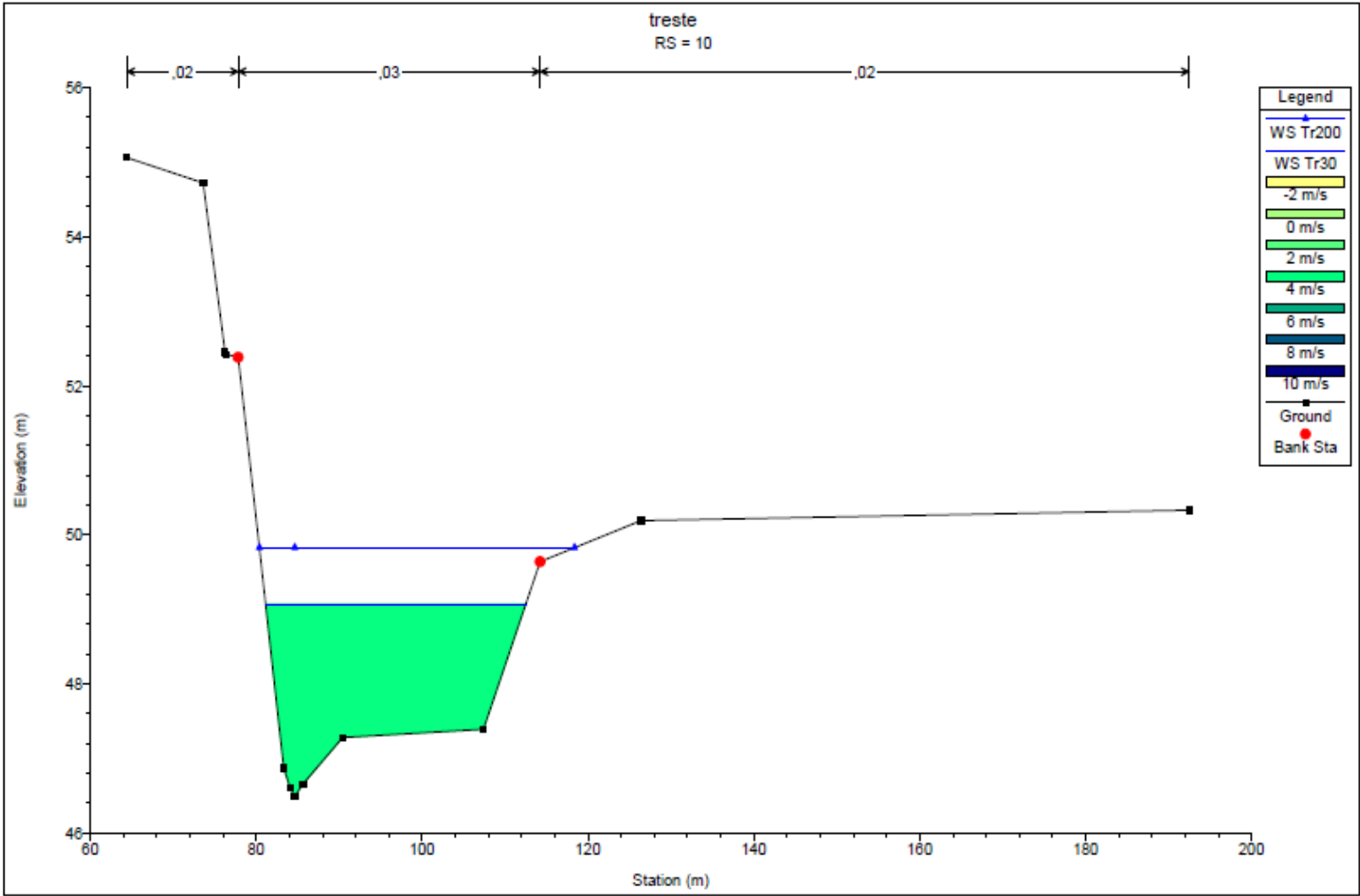
Figura 6.5: sezione trasversale 10 al termine del tratto modellato – stato di fatto e di progetto
