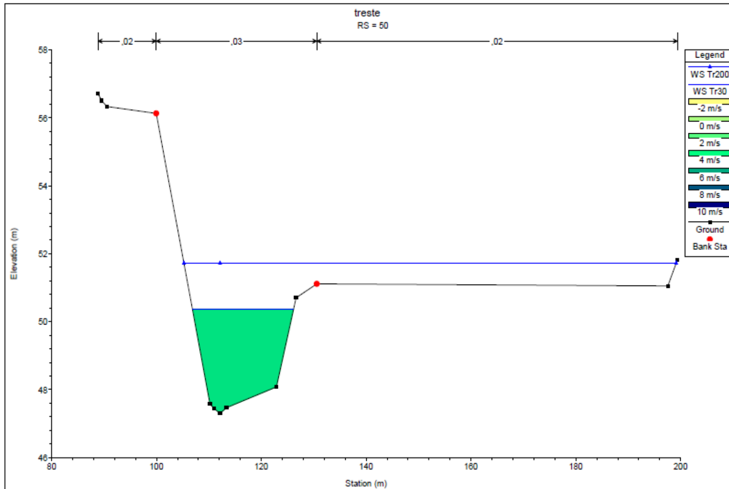
Figura 6.1: sezione trasversale 50 all'inizio del tratto modellato – stato di fatto e di progetto
