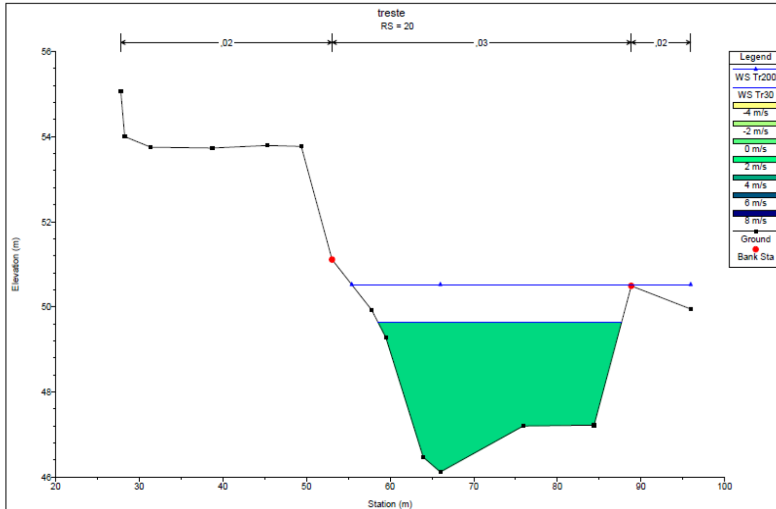
Figura 6.4: sezione trasversale 20 a valle dell'attraversamento in progetto – stato di fatto e di progetto
