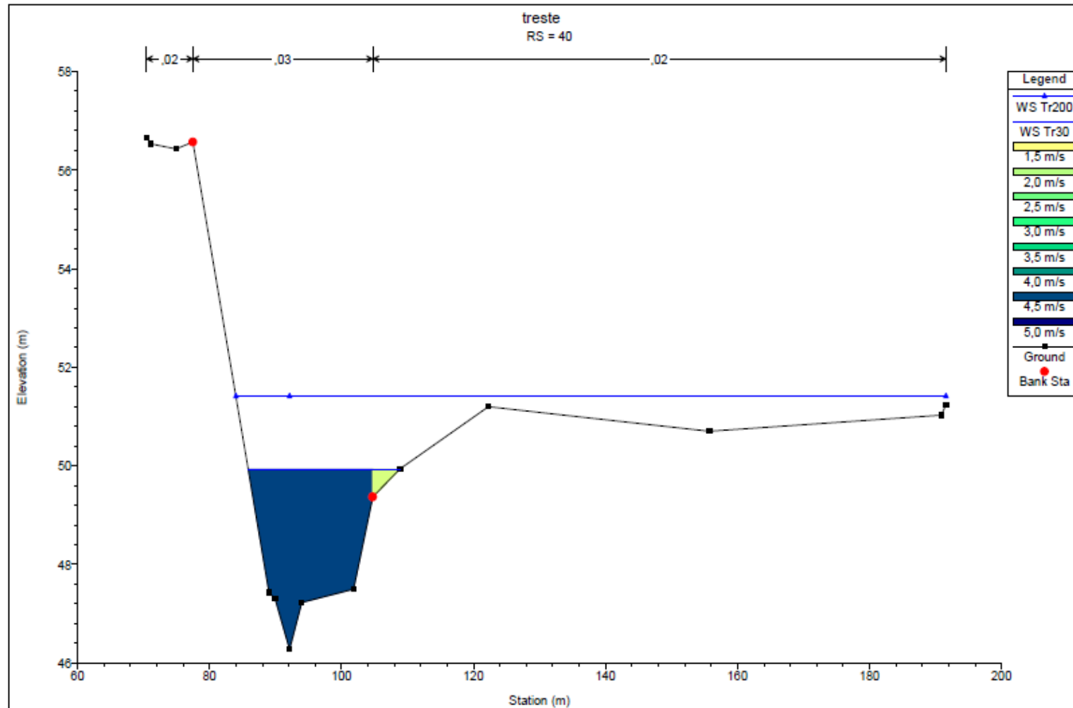
Figura 6.2: sezione trasversale 40 a monte dell'attraversamento – stato di fatto e di progetto
