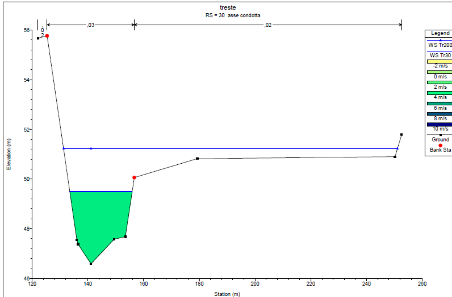
Figura 6.3: sezione trasversale 30 in corrispondenza dell'attraversamento in progetto – stato di fatto e di progetto
