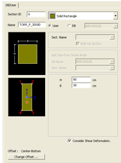
Figura 4.19:Caratteristiche geometriche delle sezioni trasversali delle travi (torrino)
