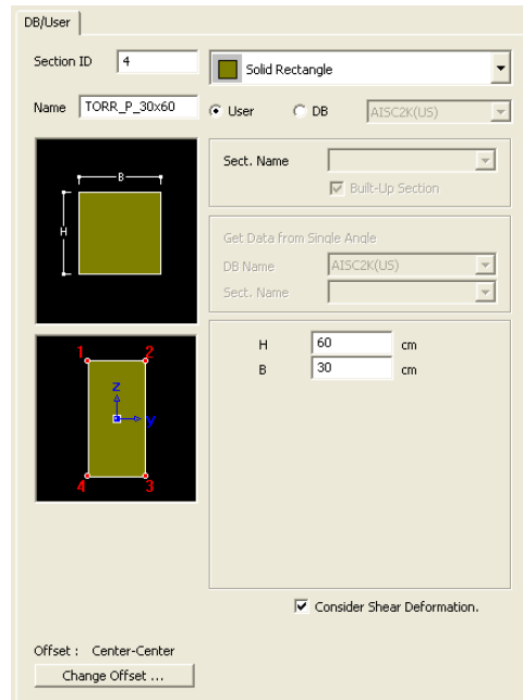
Figura 4.21:Caratteristiche geometriche delle sezioni trasversali dei pilastri del torrino
