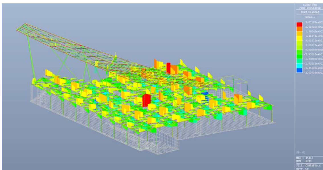
Figura 6.26: Caso di carico G2 – Valore del taglio
