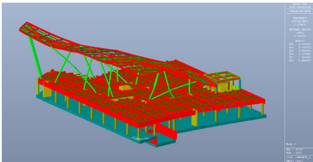
Figura 6.7: Modo di vibrare n. 2
