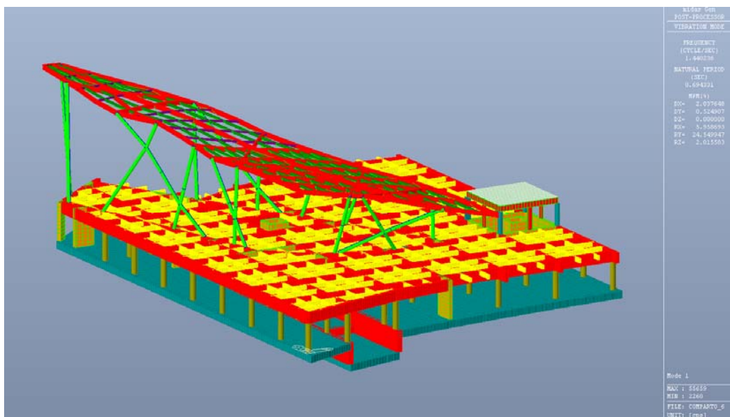
Figura 6.6: Modo di vibrare n. 1
