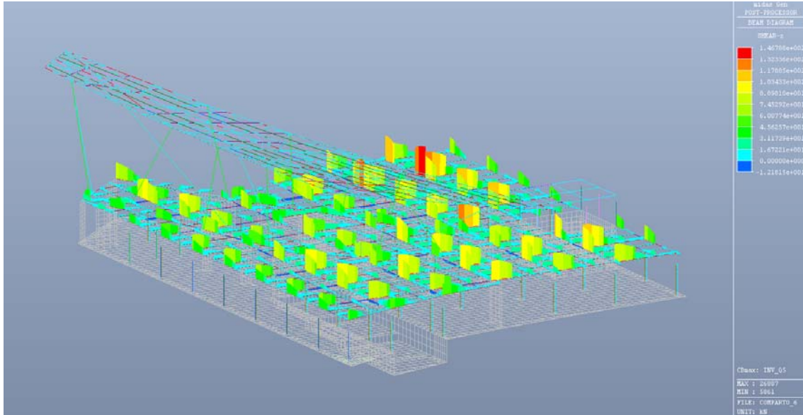
Figura 6.29: Involuppo del carico Q5 (folla) – valore del taglio
