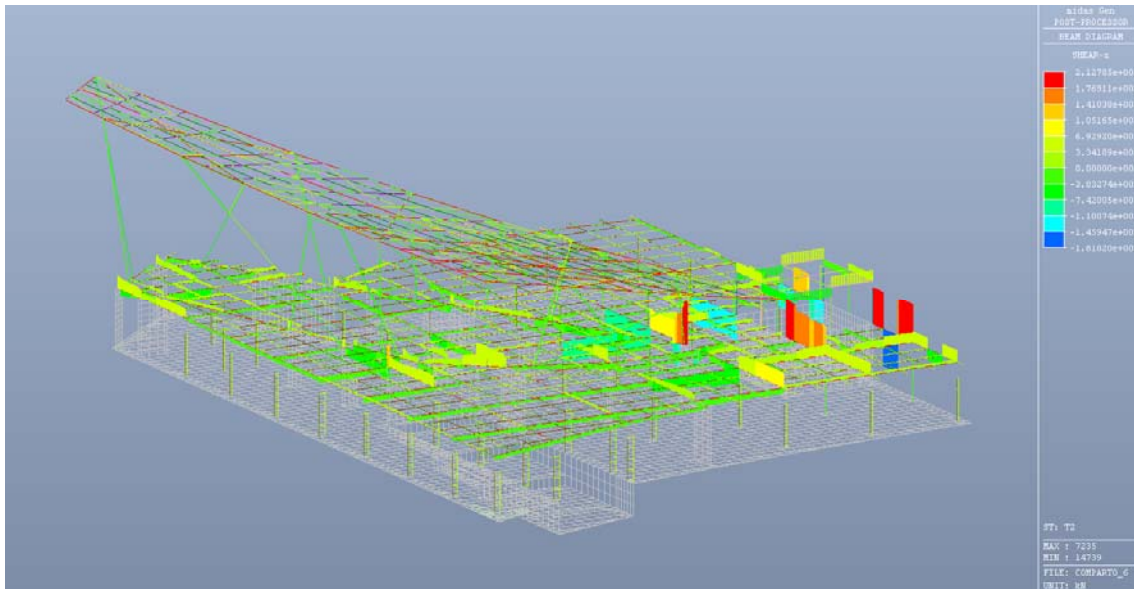
Figura 6.37: Caso di carico T2 (termico) – Valore del taglio
