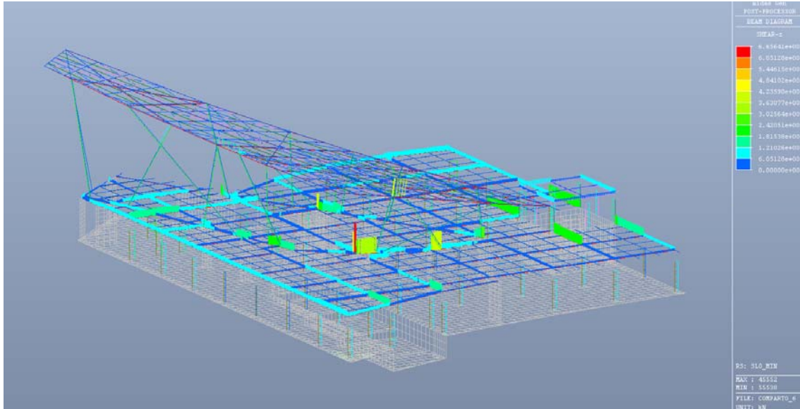
Figura 6.33: SLO min – Valore del taglio
