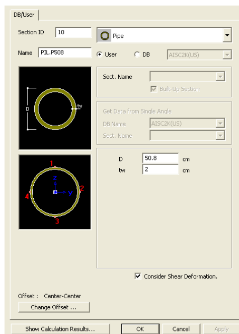
Figura 4.24:Caratteristiche geometriche pilastri arcade
