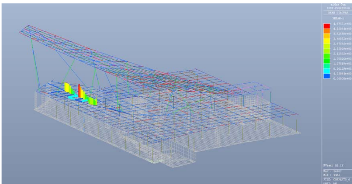
Figura 6.28: Caso di carico Q1 (traffico) in dir Y (travi principali) – Valore del taglio
