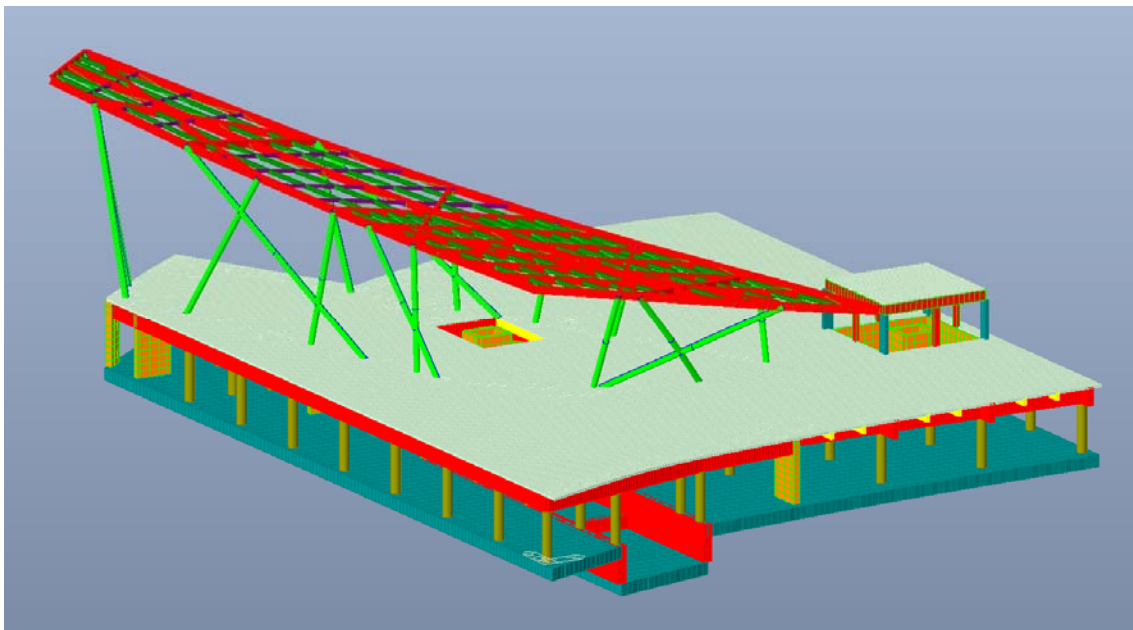
Figura 4.14: Vista assonometrica del modello di calcolo
