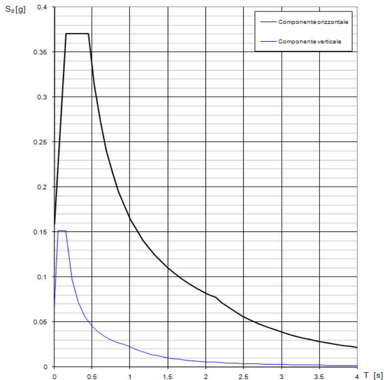
Figura 4.10: Spettro di progetto relativo allo SLO
