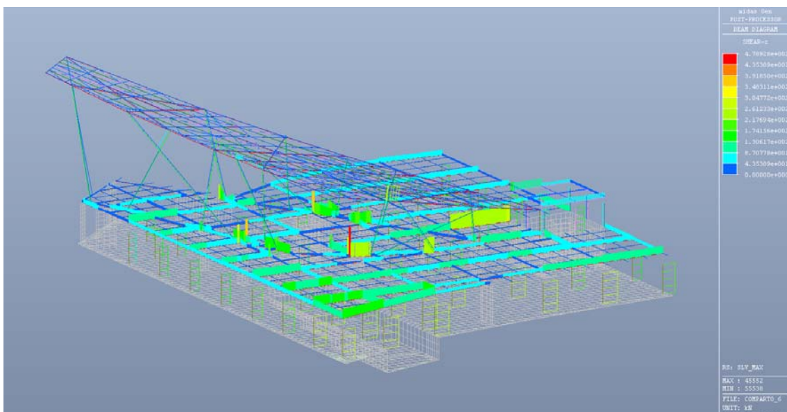
Figura 6.34: SLV max – Valore del taglio
