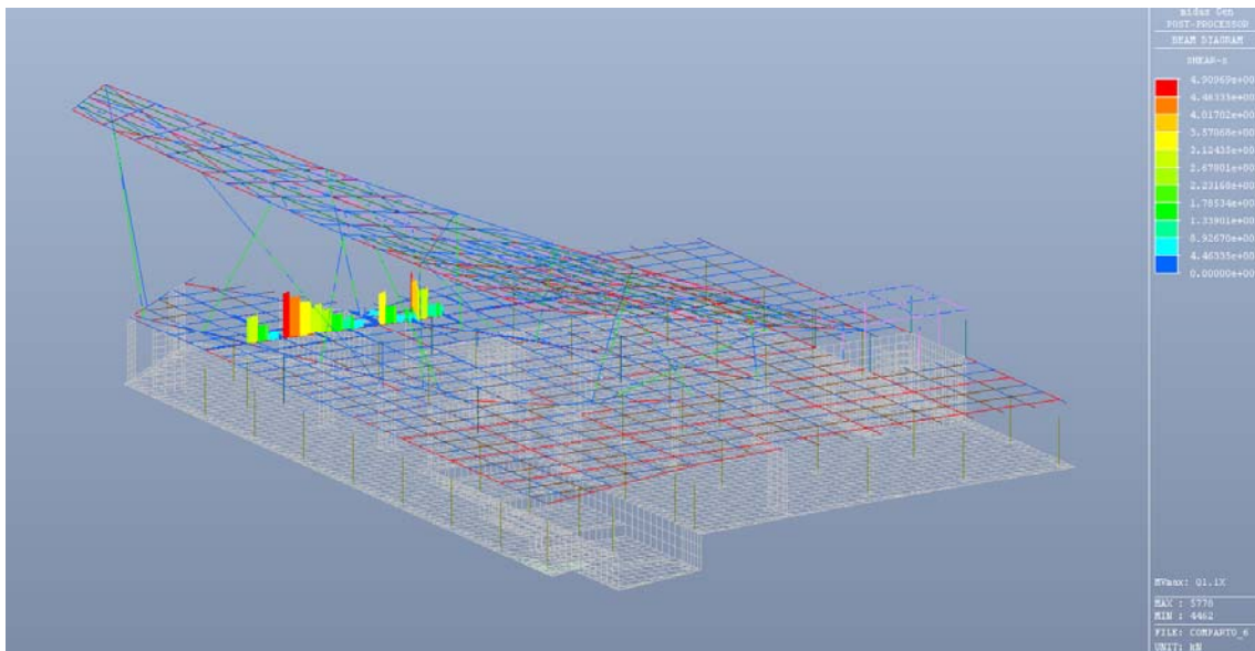
Figura 6.27: Caso di carico Q1 (traffico) in dir X (travi principali) – Valore del taglio
