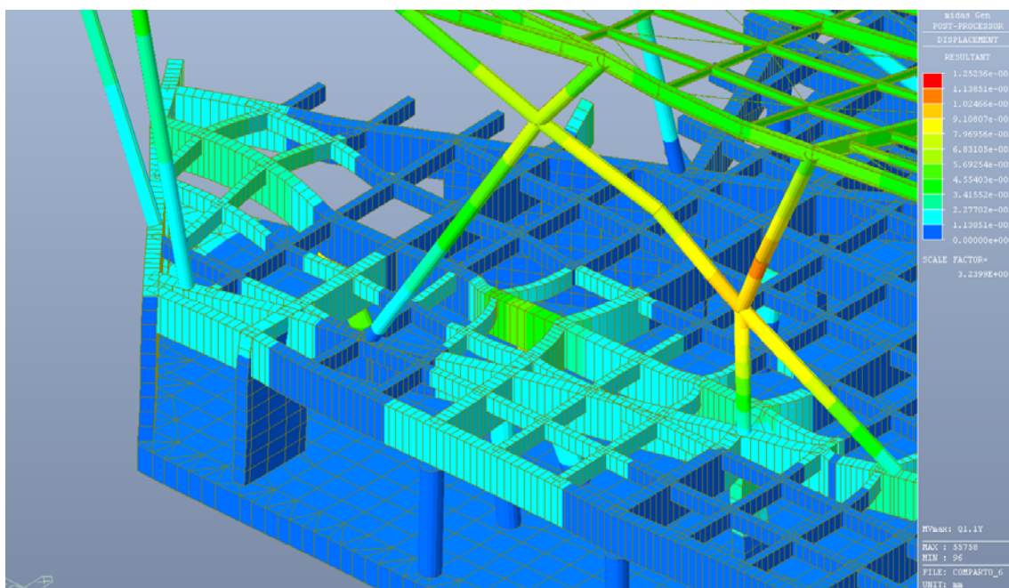
Figura 6.5: Deformate per effetto dei carico mobile in dir. Y – Q1 (inviol. max e min spostamenti)
