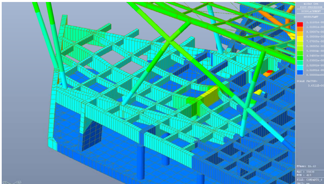
Figura 6.4: Deformate per effetto dei carico mobile in dir. X – Q1 (inviol. max e min spostamenti)
