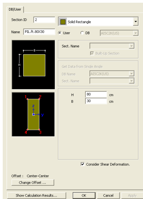
Figura 4.22:Caratteristiche geometriche delle sezioni trasversali dei pilastri del torrino
