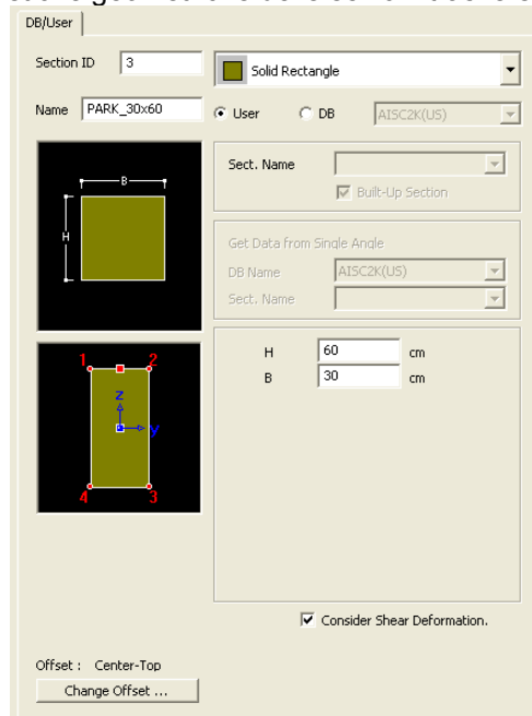
Figura 4.18:Caratteristiche geometriche delle sezioni trasversali delle travi secondarie
