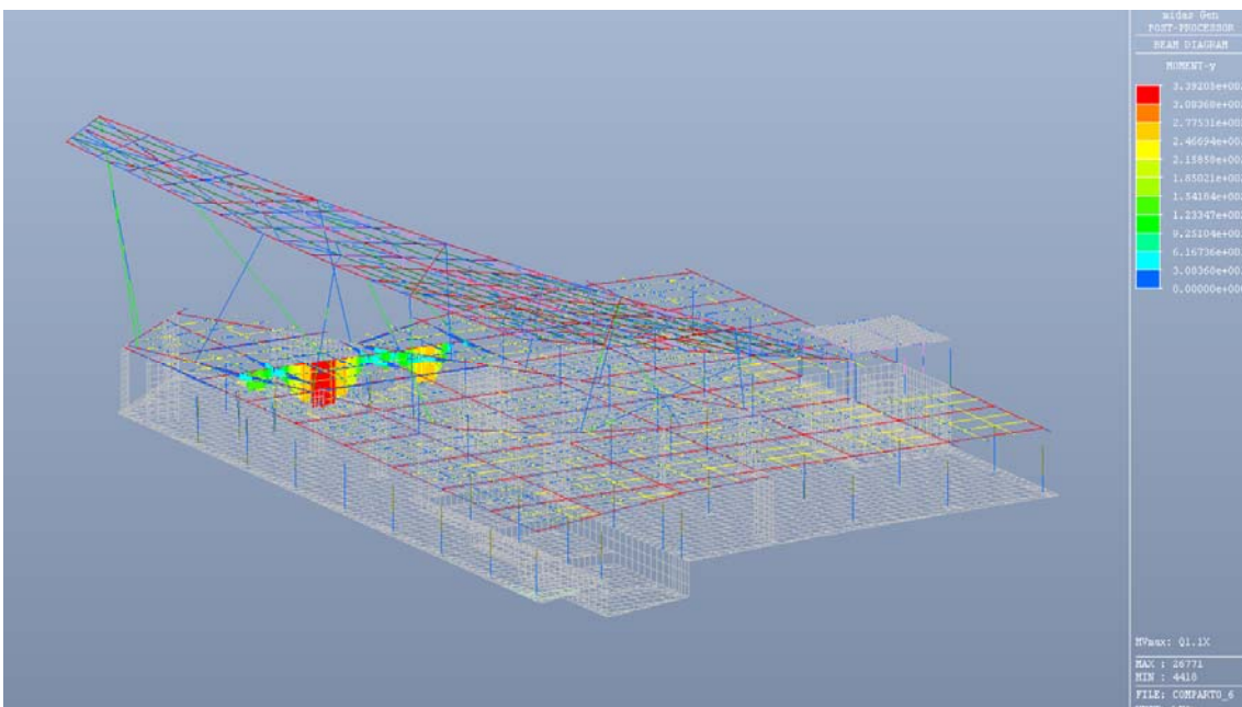
Figura 6.12: Caso di carico Q1 (traffico) in dir X (travi principali) – Valore del momento flettente
