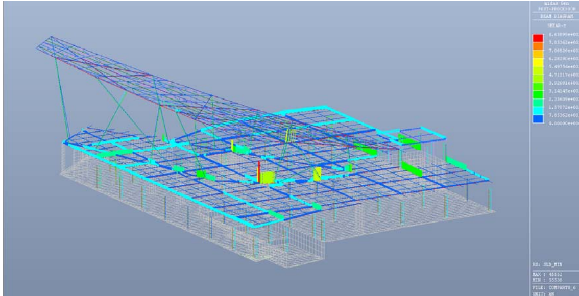
Figura 6.31: SLD min – Valore del taglio
