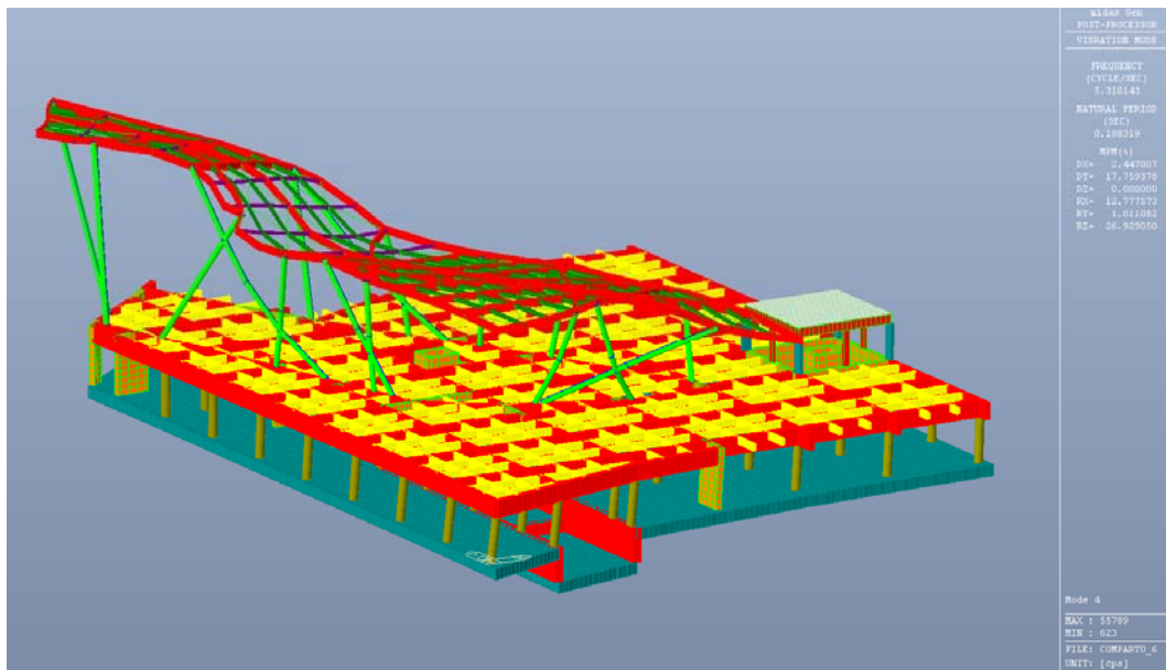
Figura 6.9: Modo di vibrare n. 4
