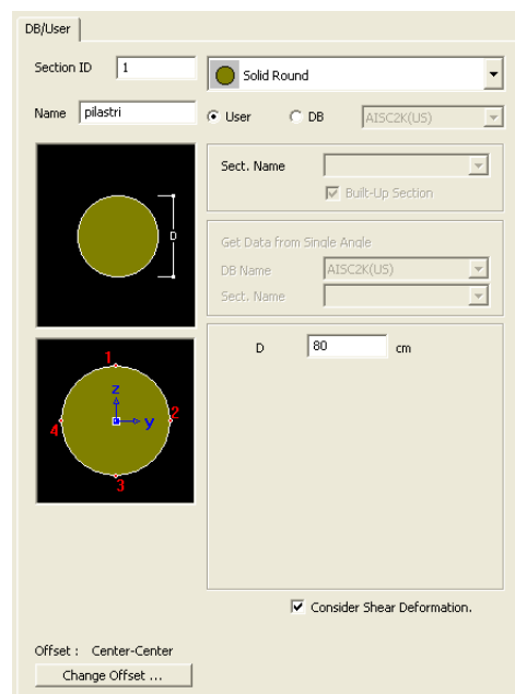
Figura 4.20:Caratteristiche geometriche delle sezioni trasversali dei pilastri
