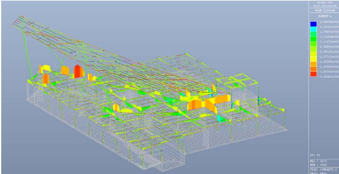
Figura 6.21: Caso di carico T1 (termico) – Valore del momento flettente
