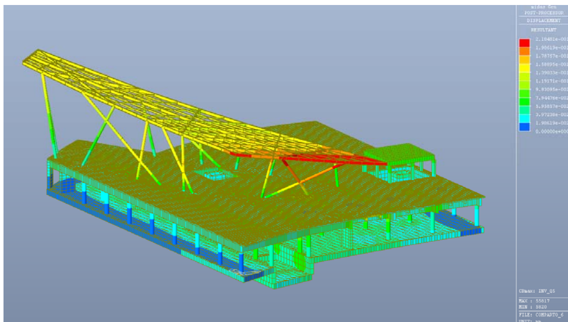
Figura 6.3: Deformate per effetto dei carico della folla compatta – Q5 (invil. max e min spostamenti)
