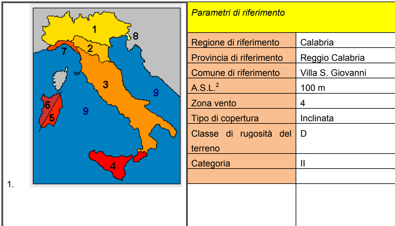
Fig. 4.5 – Determinazione dell'azione del vento
