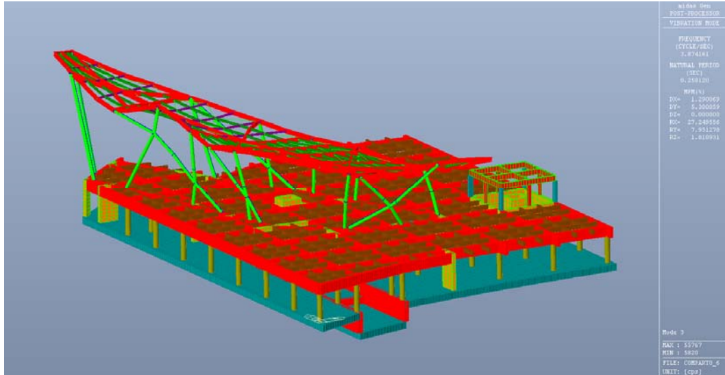
Figura 6.8: Modo di vibrare n. 3
