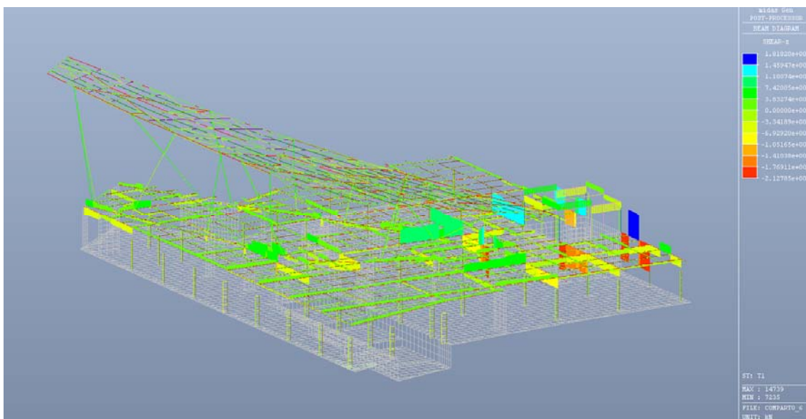
Figura 6.36: Caso di carico T1 (termico) – Valore del taglio
