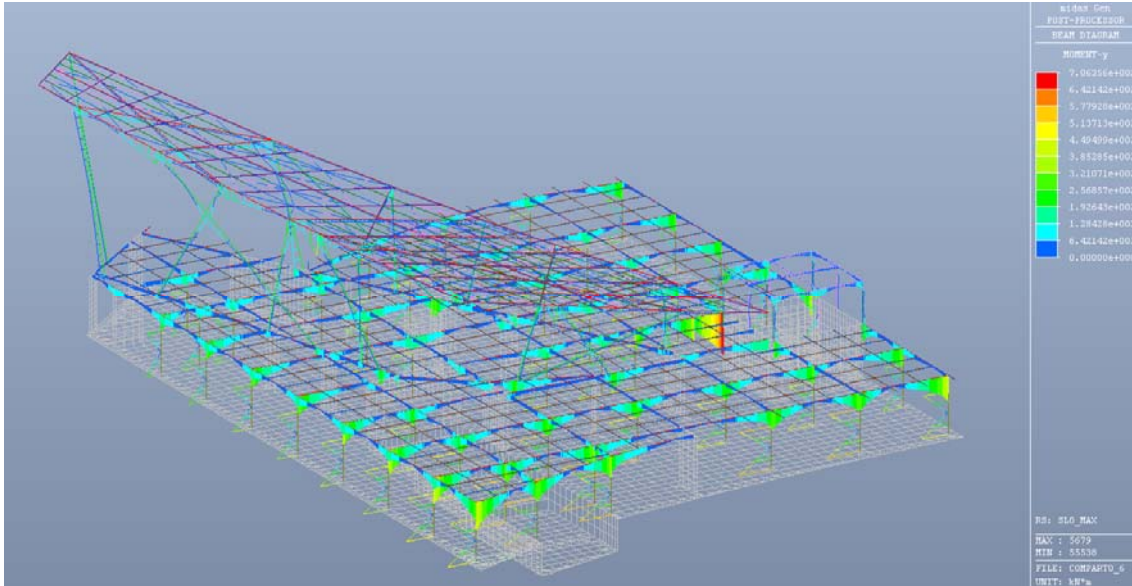
Figura 6.17: SLO max – Valore del momento flettente
