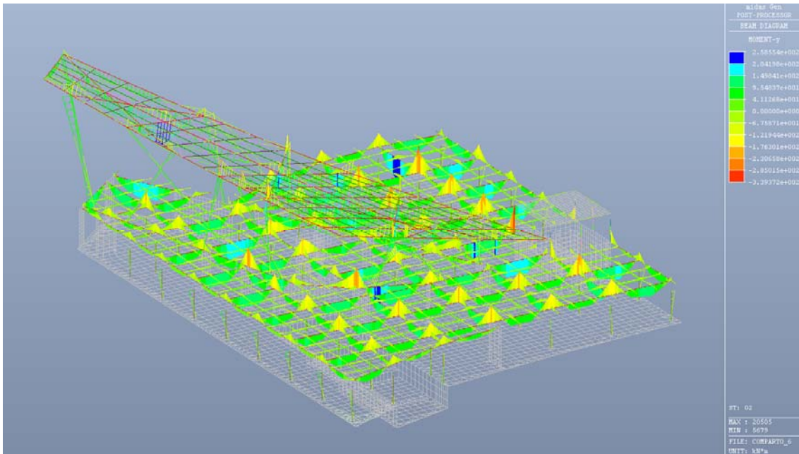
Figura 6.11: Caso di carico G2 – Valore del momento flettente
