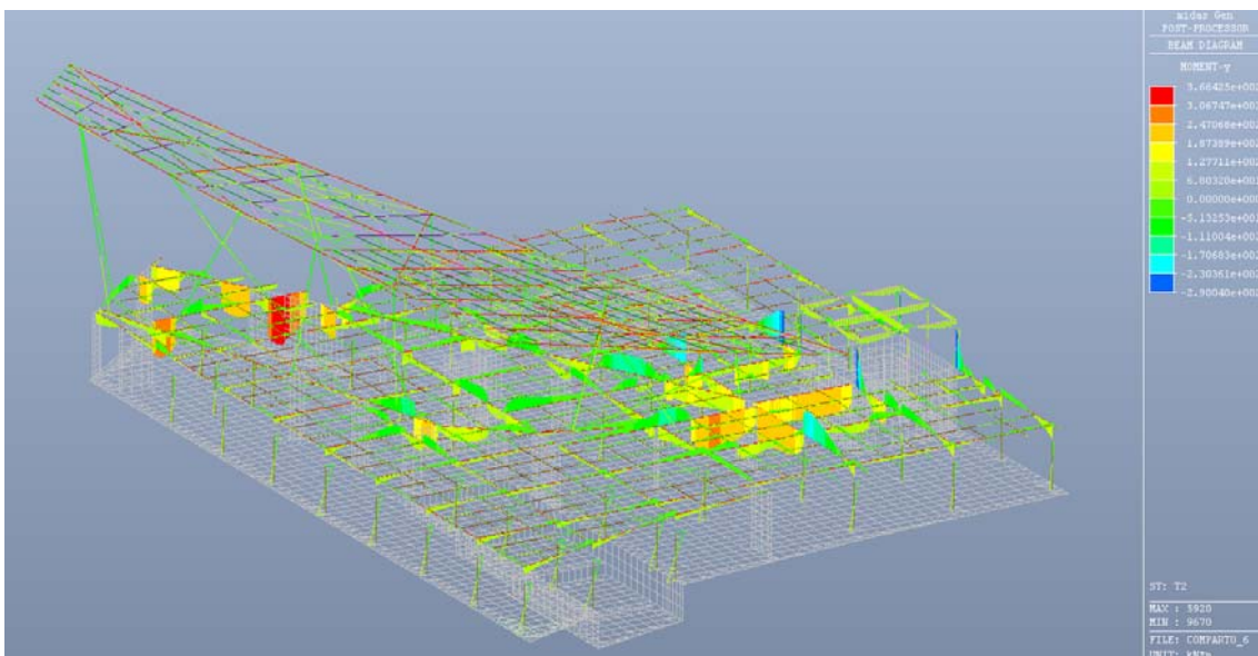
Figura 6.22: Caso di carico T2 (termico) – Valore del momento flettente
