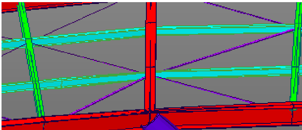
Figura 4.16 – Particolare del sistema di controventatura
