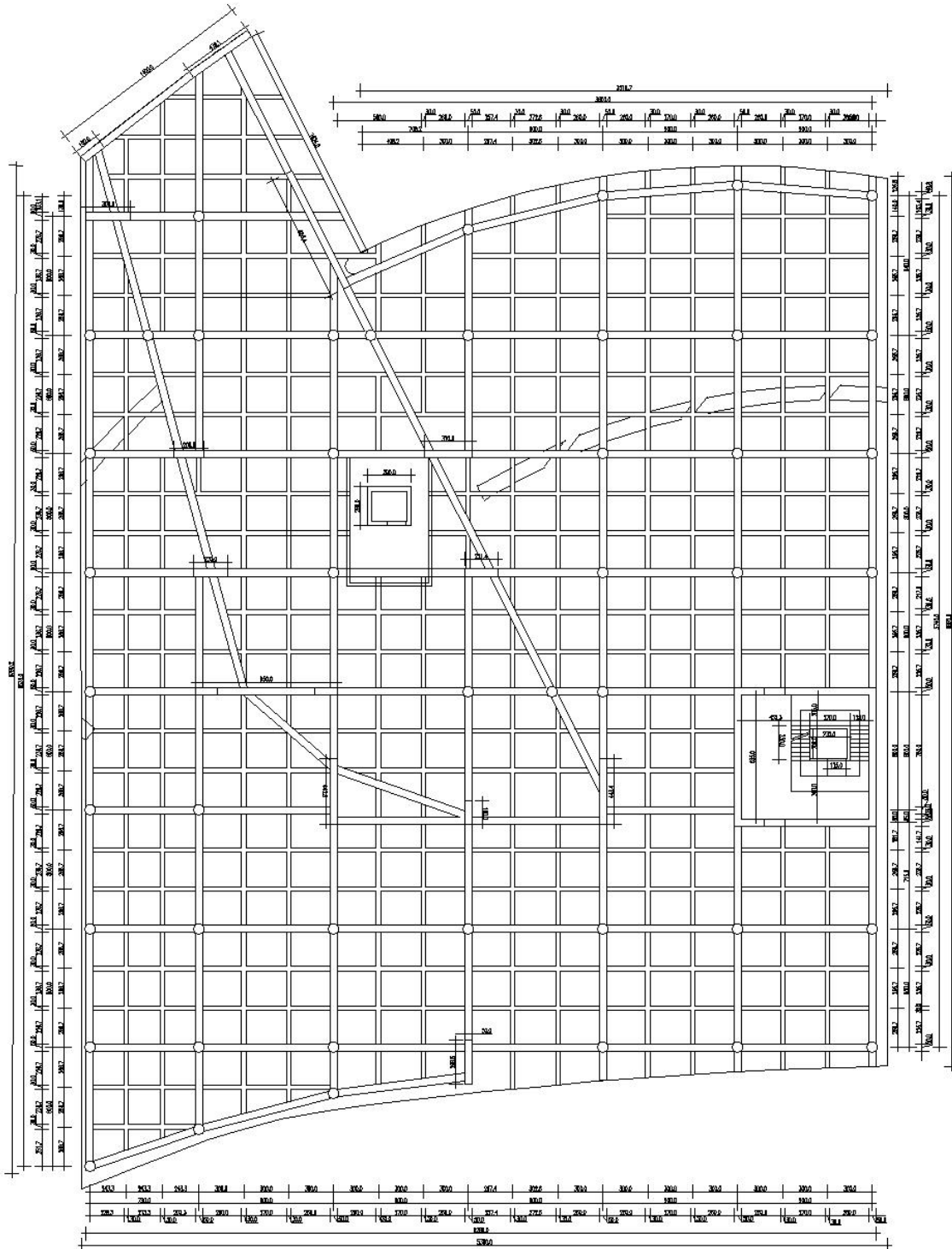
Figura 4.1: Carpenteria del primo impalcato del corpo n. 6
