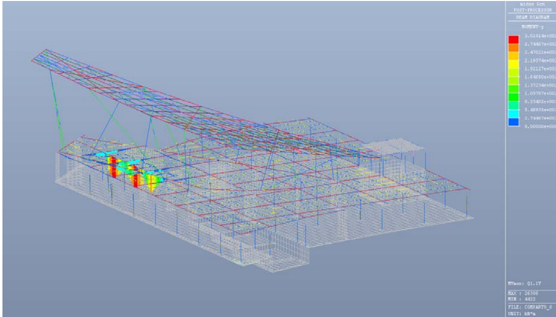
Figura 6.13: Caso di carico Q1 (traffico) in dir Y (travi principali) – Valore del momento flettente
