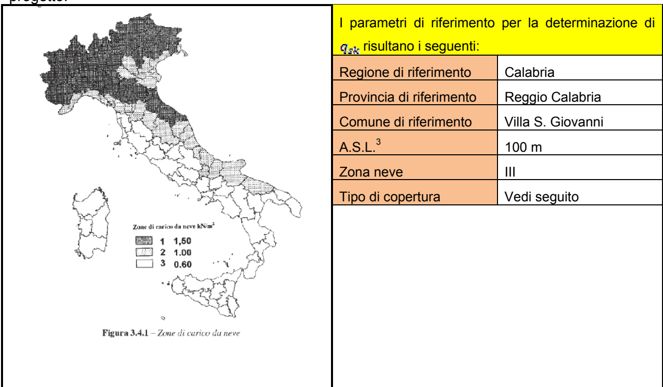
Fig. 4.6 – Parametri calcolo azione neve
