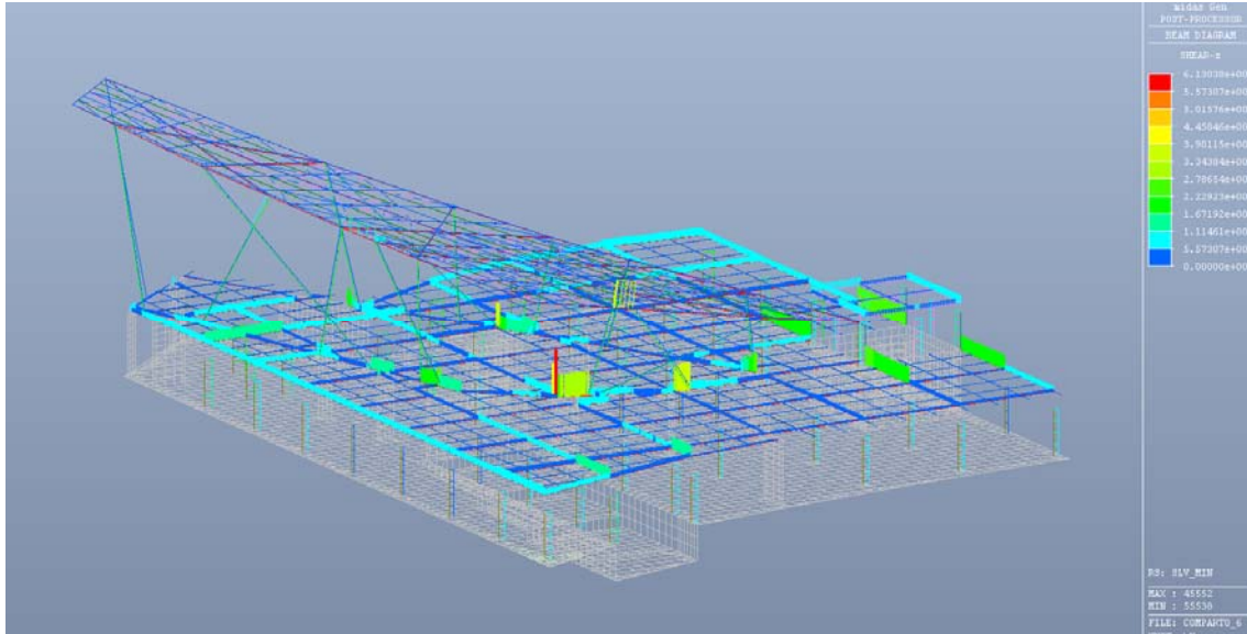
Figura 6.35: SLV min – Valore del taglio
