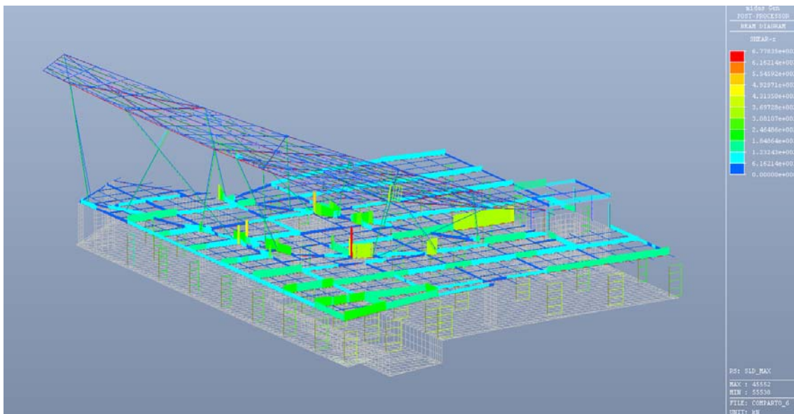
Figura 6.30: SLD max – Valore del taglio
