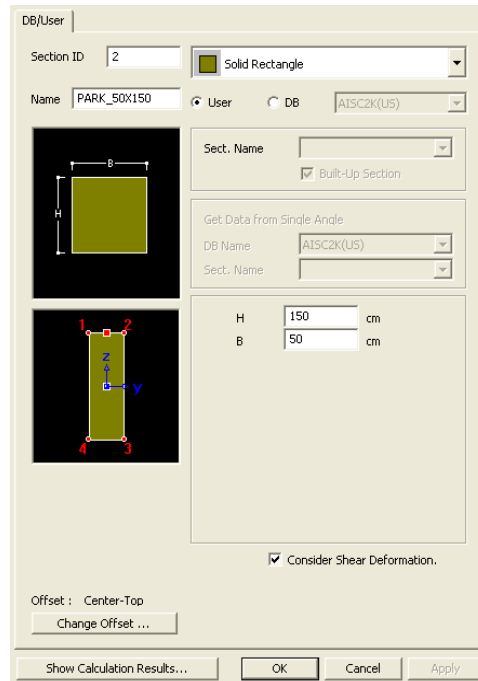
Figura 4.17:Caratteristiche geometriche delle sezioni trasversali delle travi principali
