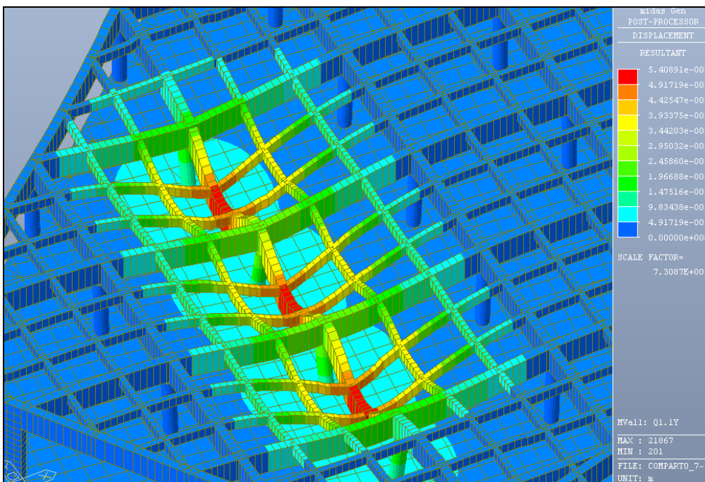
Figura 6.5: Deformate per effetto dei carico mobile in dir. Y – Q1 (inviol. max e min spostamenti)
