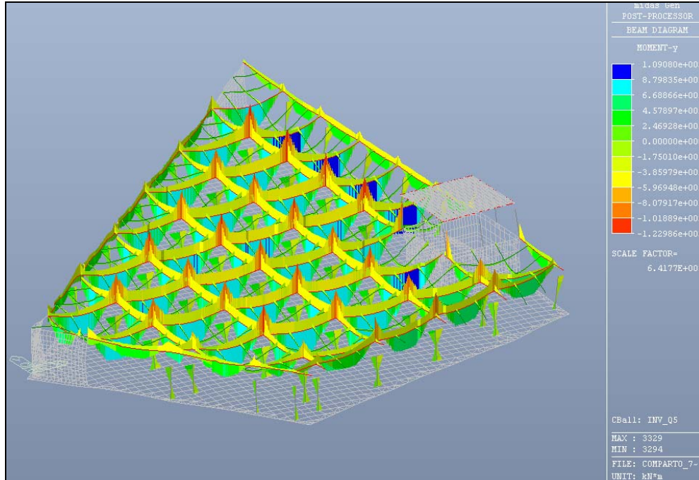
Figura 6.16: Involuppo del carico Q5 (folia) – valore del momento flettente
