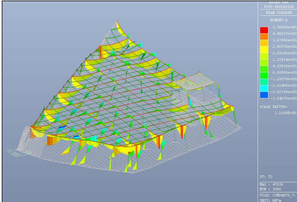
Figura 6.24: Caso di carico T2 (termico) – Valore del momento flettente
