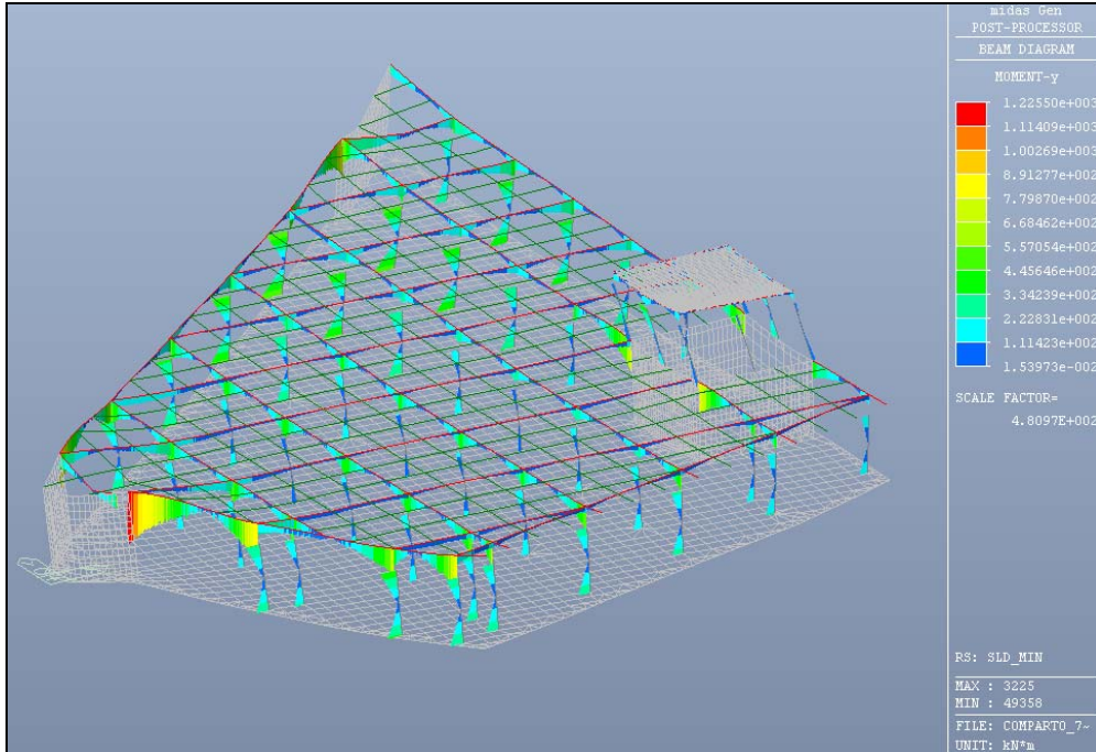
Figura 6.18: SLD min – Valore del momento flettente
