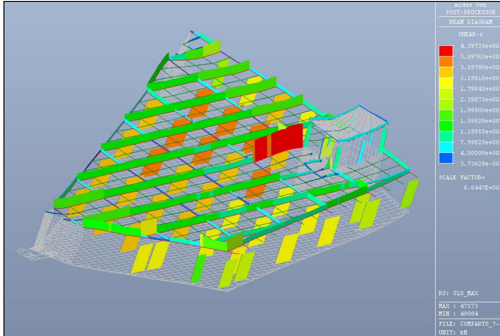
Figura 6.34: SLO max – Valore del taglio
