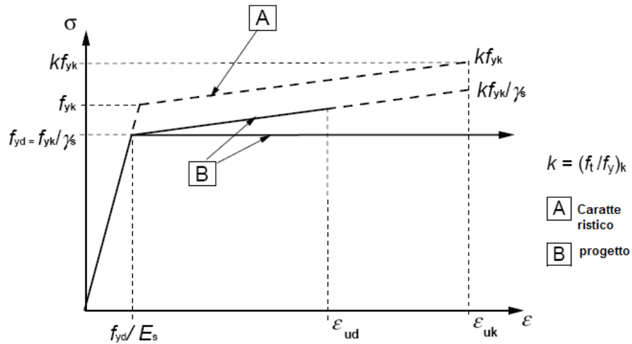
Figura 3.2: Legge costitutiva di progetto dell'acciaio
