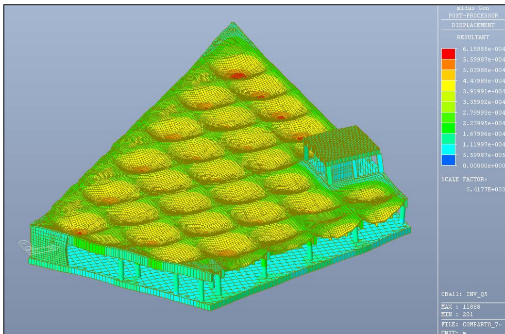
Figura 6.3: Deformate per effetto dei carico della folla compatta – Q5 (inviol. max e min spostamenti)
