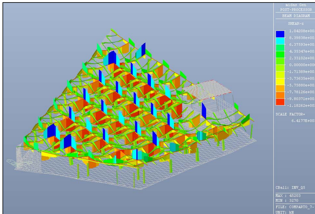
Figura 6.31: Involuppo del carico Q5 (folla) – valore del taglio
