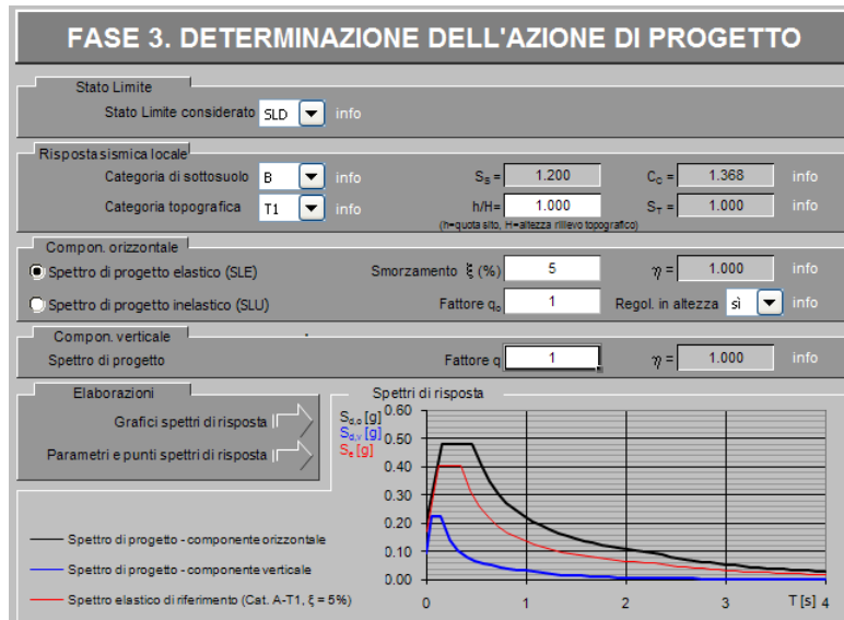
Figura 4.10: Determinazione dello spettro di progetto relativo allo SLD
