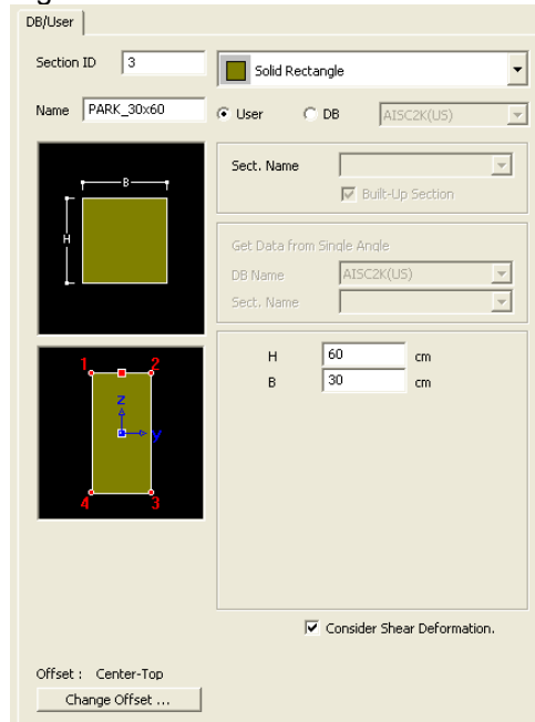
Figura 4.17:Caratteristiche geometriche delle sezioni trasversali delle travi secondarie (piazza)
