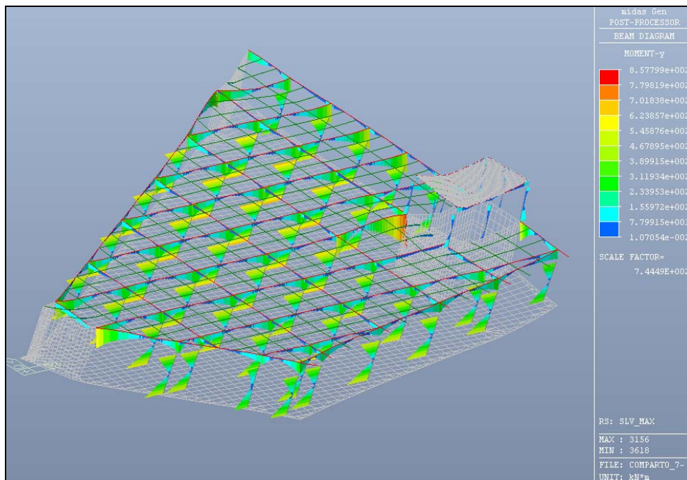
Figura 6.21: SLV max – Valore del momento flettente
