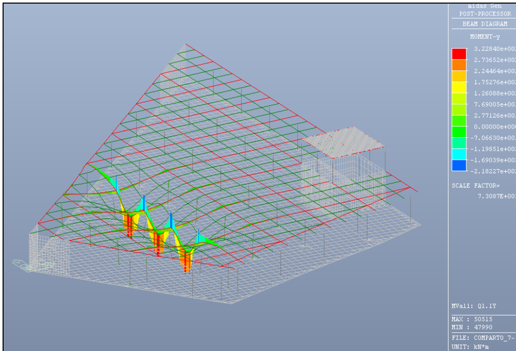
Figura 6.14: Caso di carico Q1 (traffico) in dir Y (travi principali) – Valore del momento flettente
