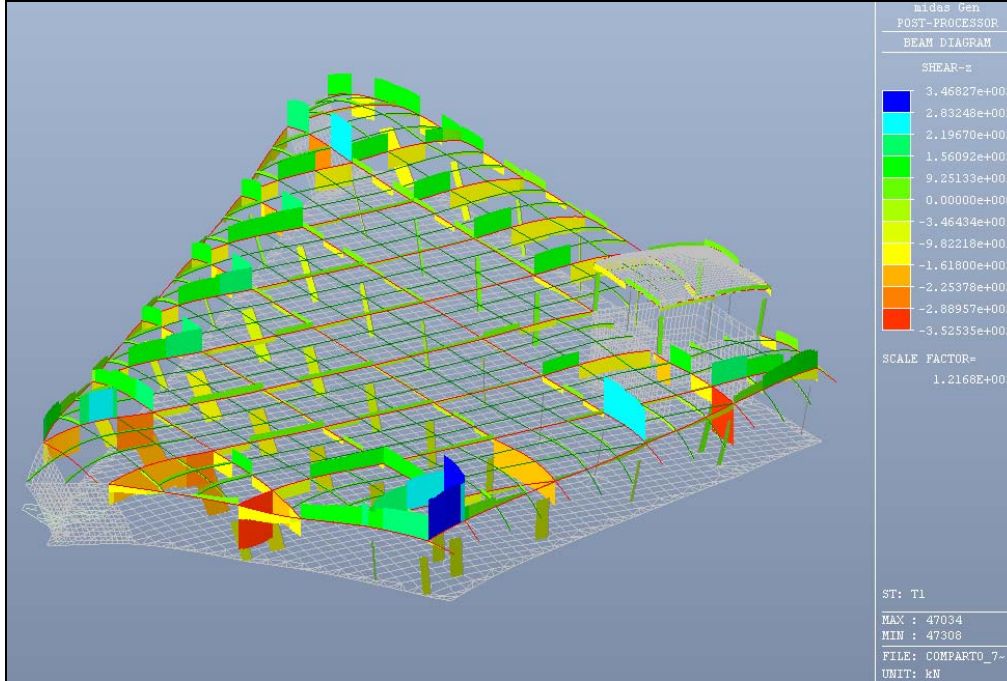
Figura 6.38: Caso di carico T1 (termico) – Valore del taglio
