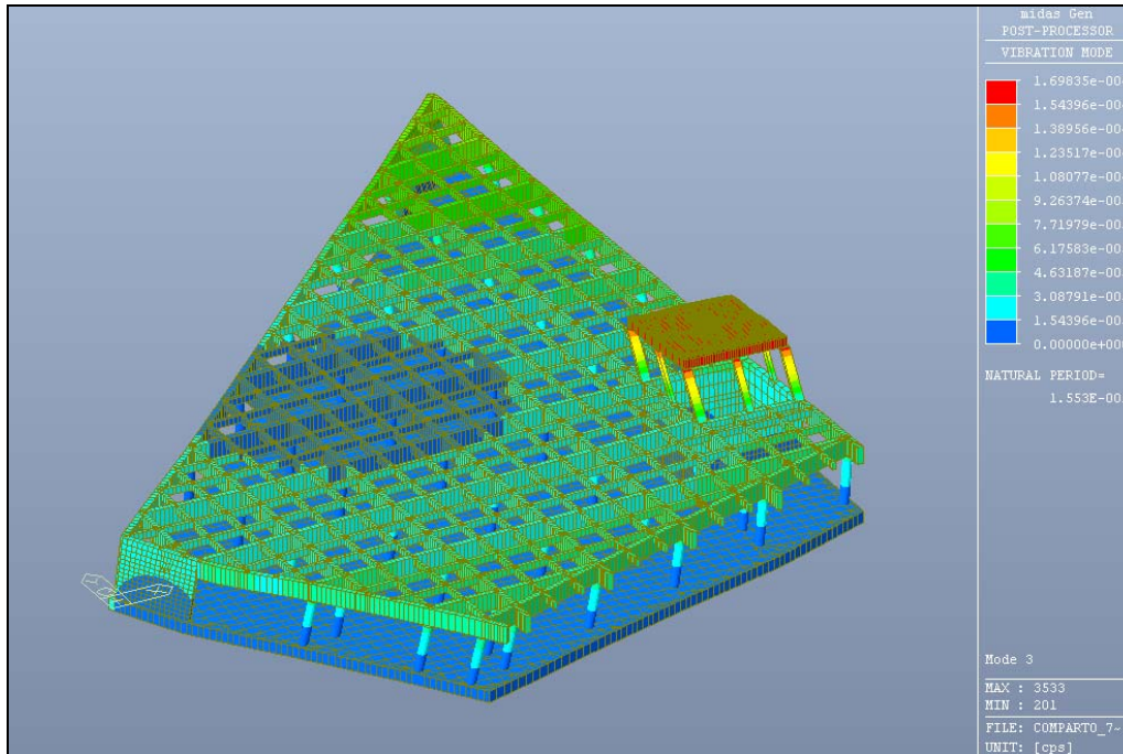
Figura 6.8: Modo di vibrare n. 3
