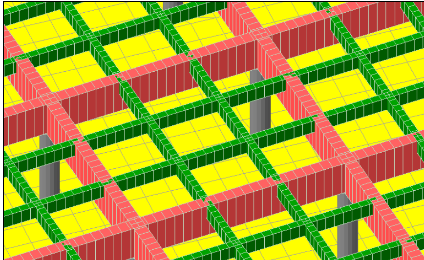
Figura 4.15: Particolare delle travi principali (in rosso) e delle travi secondarie (in verde)
