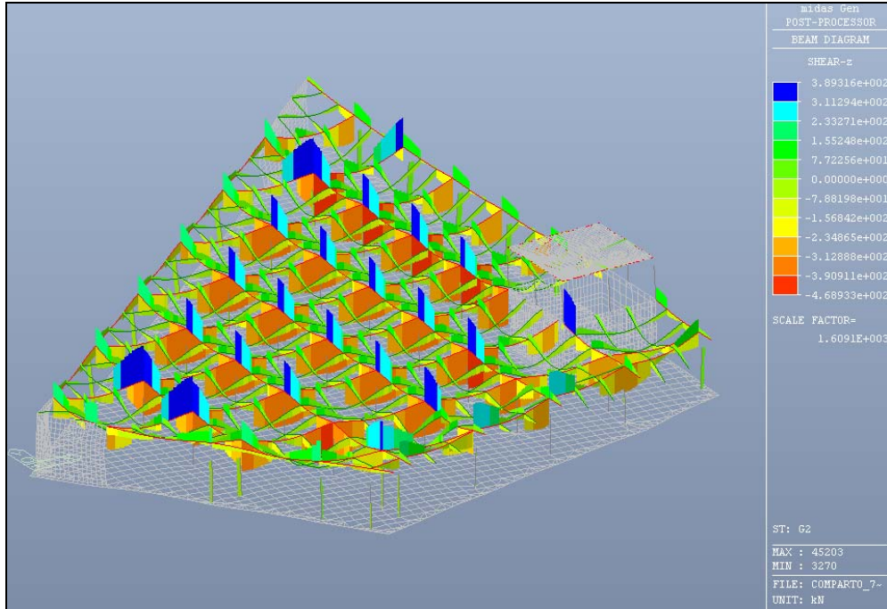
Figura 6.26: Caso di carico G2 – Valore del taglio
