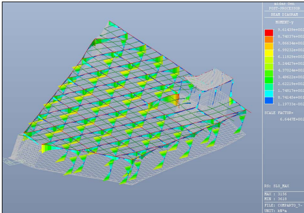
Figura 6.19: SLO max – Valore del momento flettente
