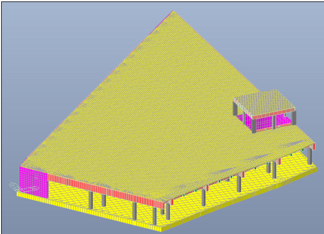
Figura 4.14: Vista assometrica del modello di calcolo
