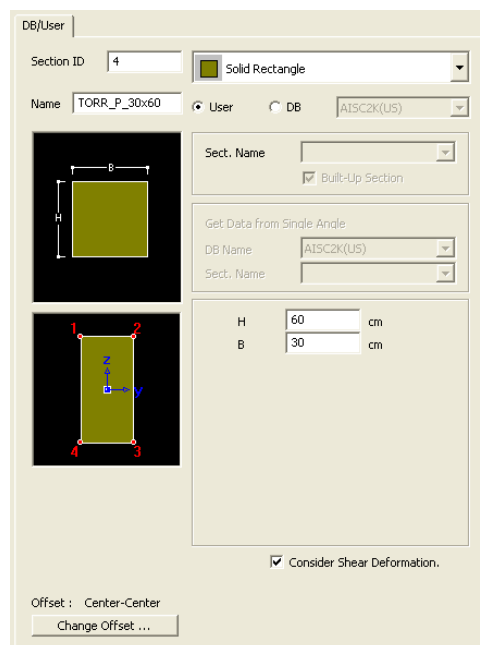
Figura 4.20:Caratteristiche geometriche delle sezioni trasversali dei pilastri del torrino
