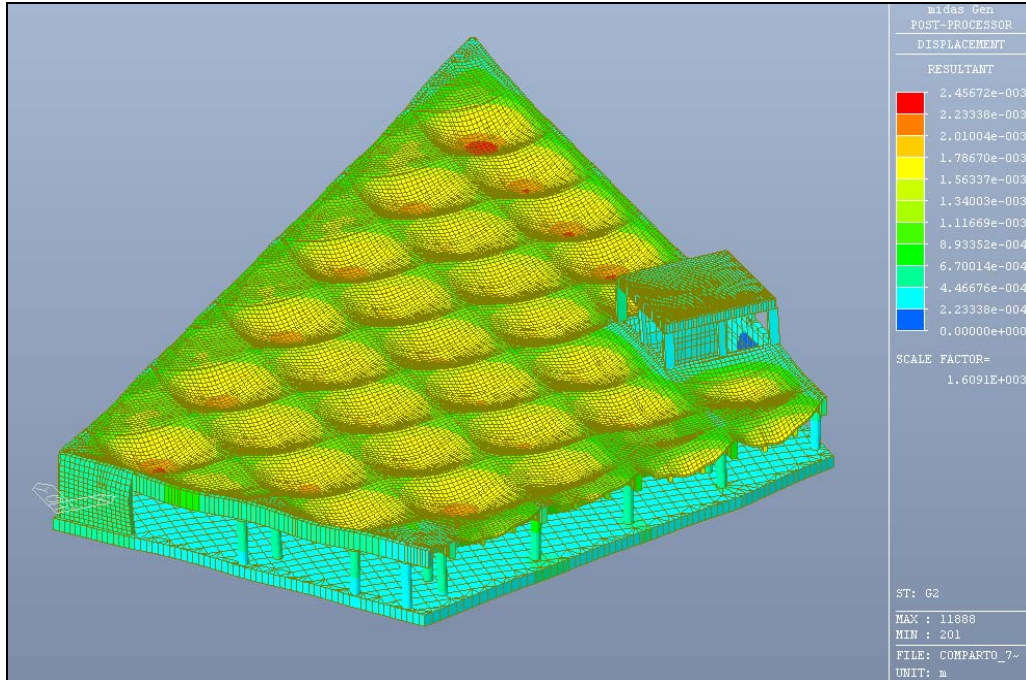
Figura 6.2: Deformate per effetto dei carichi permanenti portati – G2
