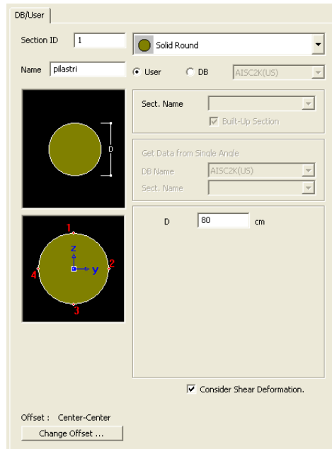
Figura 4.19:Caratteristiche geometriche delle sezioni trasversali dei pilastri
