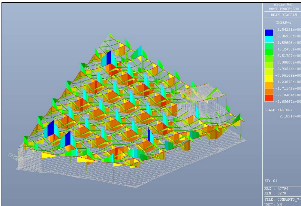
Figura 6.25: Caso di carico G1 – Valore del taglio
