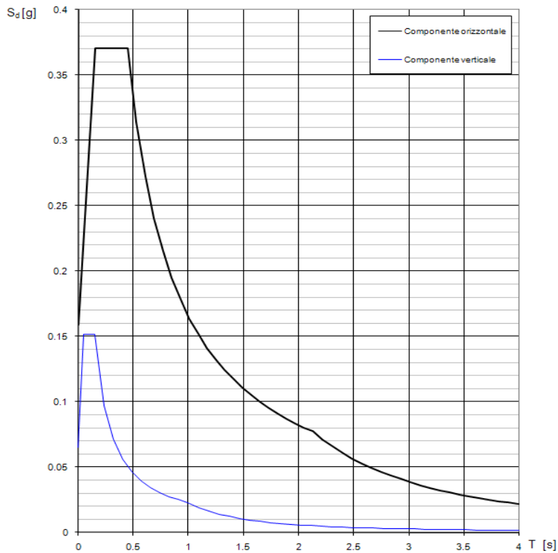
Figura 4.9: Spettro di progetto relativo allo SLO
