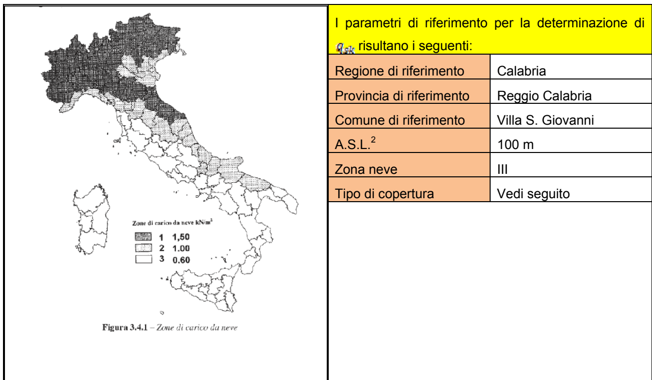
Figura 4.5: Parametri valutazione carico da neve
