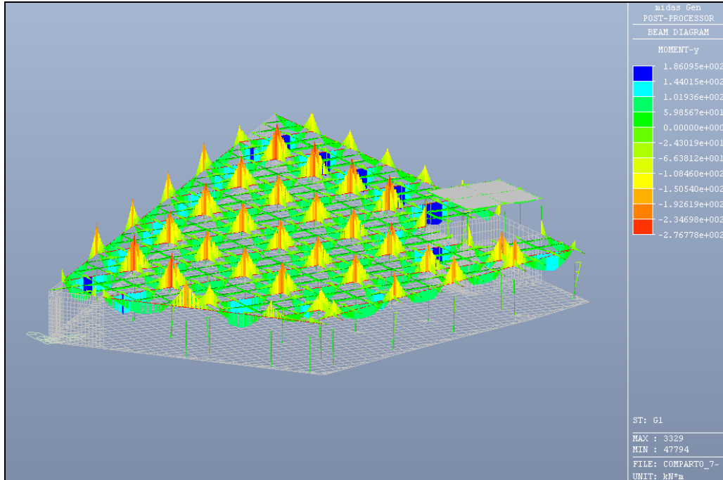
Figura 6.10: Caso di carico G1 – Valore del momento flettente
