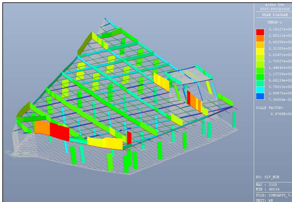
Figura 6.37: SLV min – Valore del taglio
