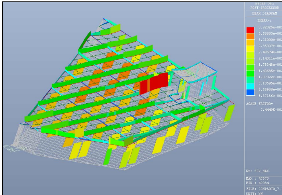
Figura 6.36: SLV max – Valore del taglio
