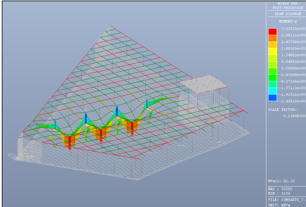
Figura 6.12: Caso di carico Q1 (traffico) in dir X (travi principali) – Valore del momento flettente
