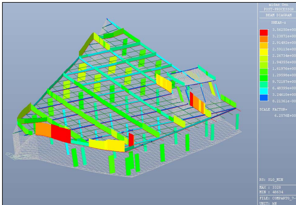
Figura 6.35: SLO min – Valore del taglio
