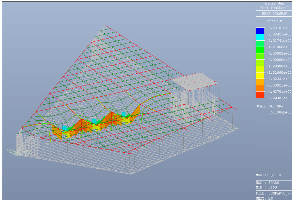
Figura 6.27: Caso di carico Q1 (traffico) in dir X (travi principali) – Valore del taglio
