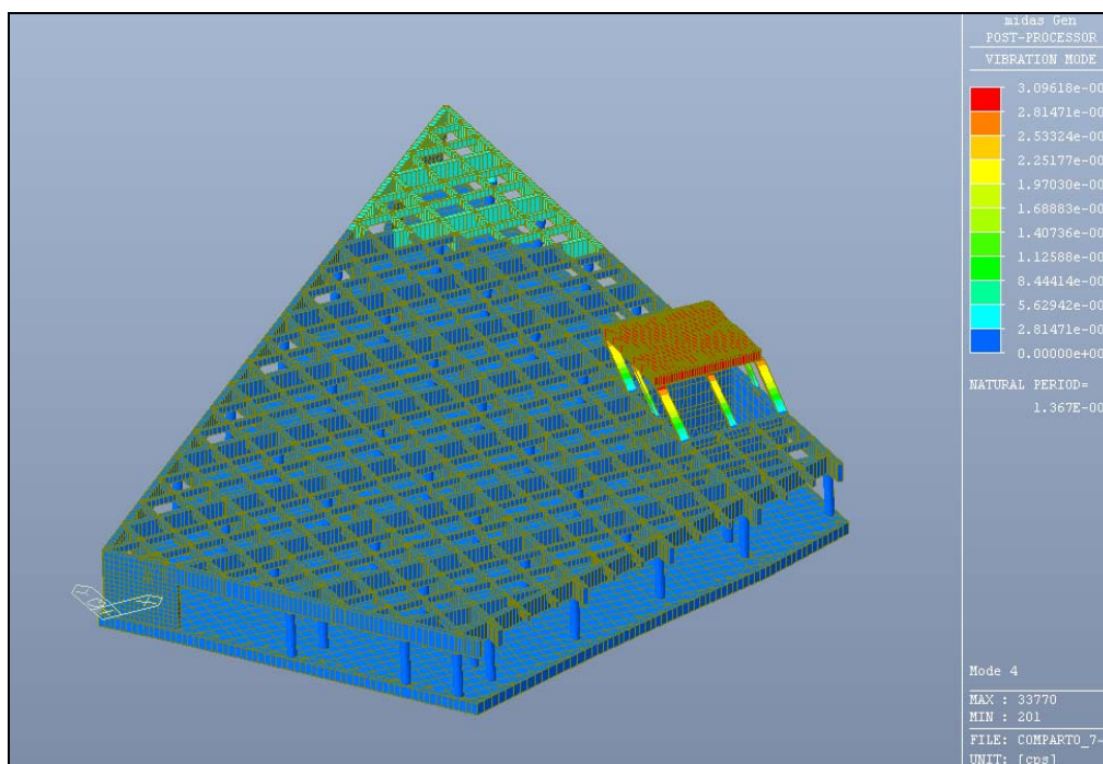
Figura 6.9: Modo di vibrare n. 4
