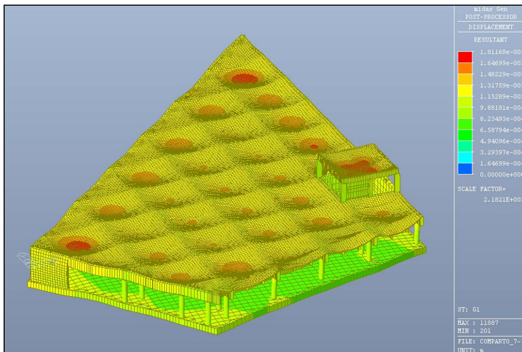
Figura 6.1: Deformate per effetto dei pesi propri strutturali – G1
