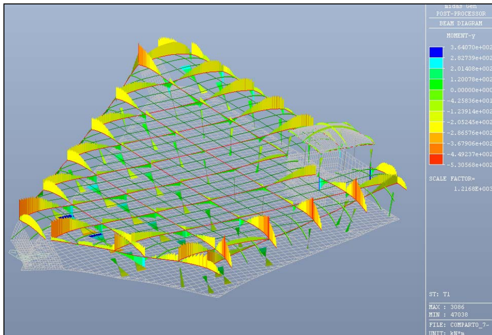
Figura 6.23: Caso di carico T1 (termico) – Valore del momento flettente
