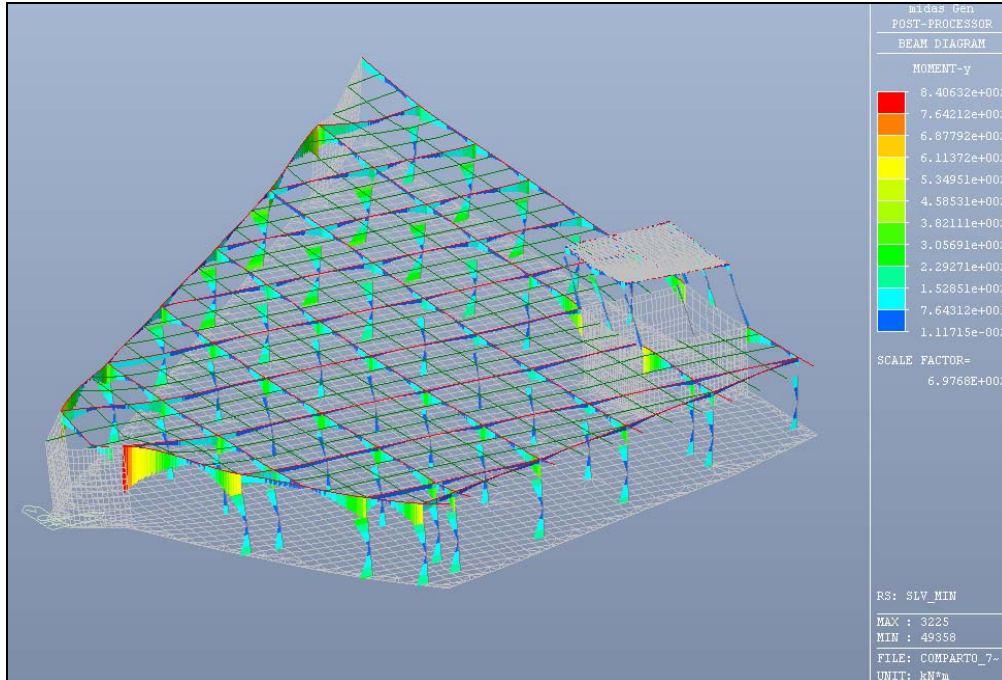
Figura 6.22: SLV min – Valore del momento flettente
