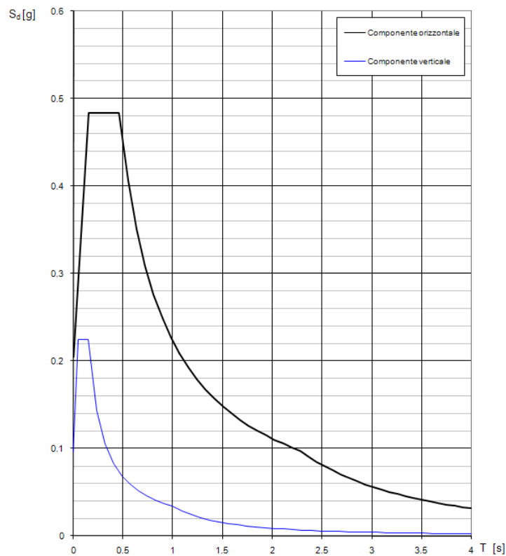
Figura 4.11: Spettro di progetto relativo allo SLD
