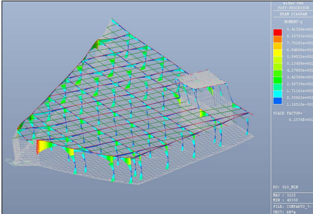
Figura 6.20: SLO min – Valore del momento flettente
