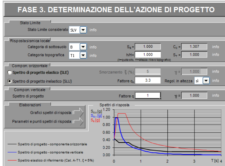
Figura 4.12: Determinazione dello spettro di progetto relativo allo SLV
