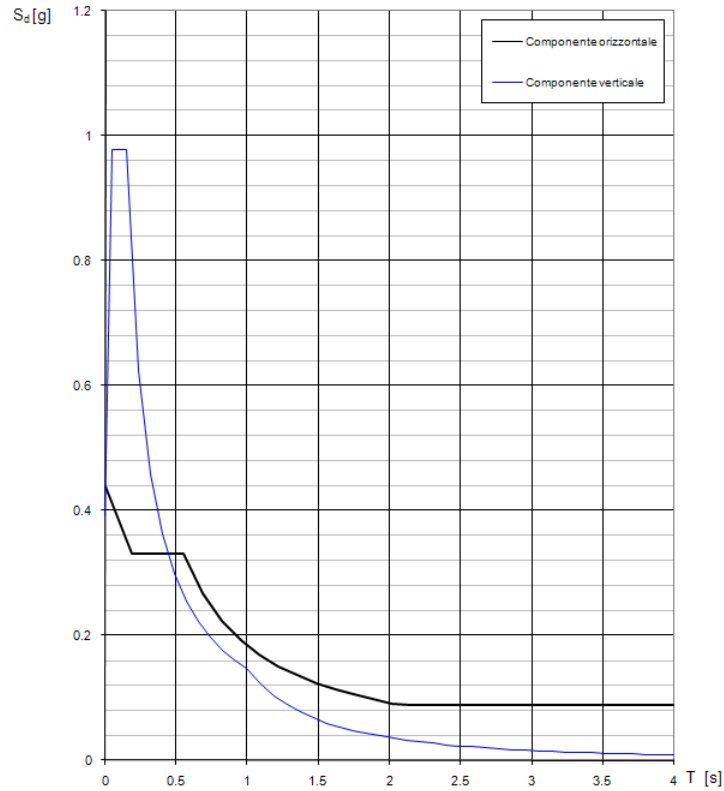
Figura 4.13: Spettro di progetto relativo allo SLV
