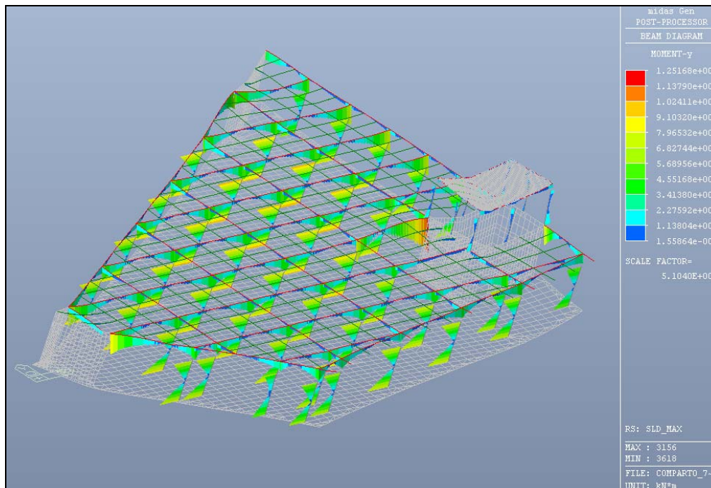
Figura 6.17: SLD max – Valore del momento flettente
