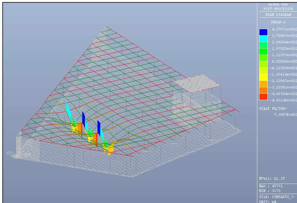
Figura 6.29: Caso di carico Q1 (traffico) in dir Y (travi principali) – Valore del taglio
