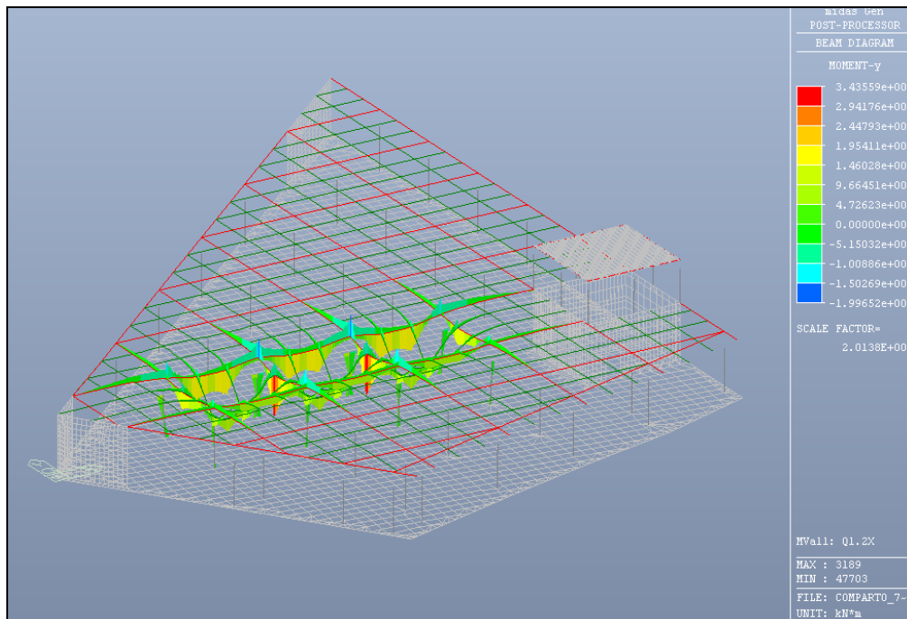
Figura 6.13: Caso di carico Q1 (traffico) in dir X (travi secondarie) – Valore del momento flettente
