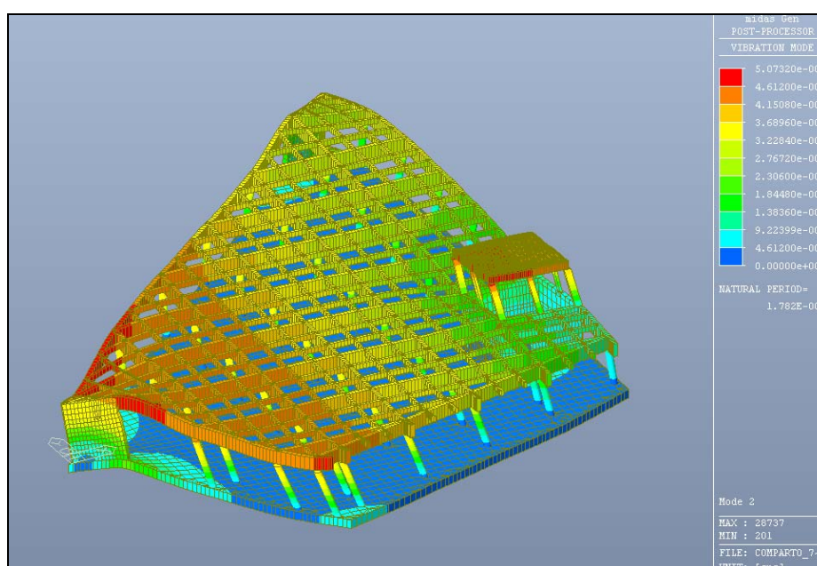
Figura 6.7: Modo di vibrare n. 2
