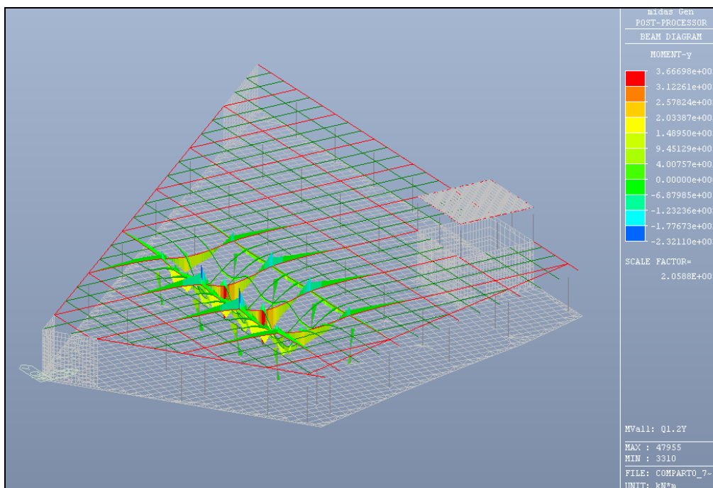
Figura 6.15: Caso di carico Q1 (traffico) in dir Y (travi secondarie) – Valore del momento flettente
