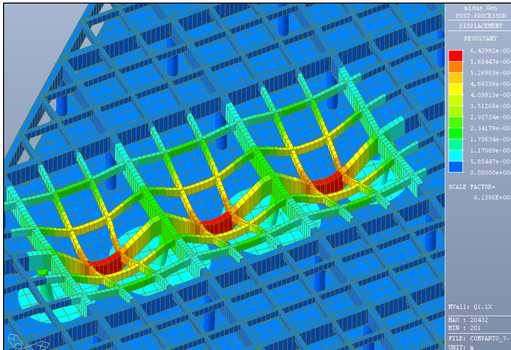
Figura 6.4: Deformate per effetto dei carico mobile in dir. X – Q1 (inviol. max e min spostamenti)
