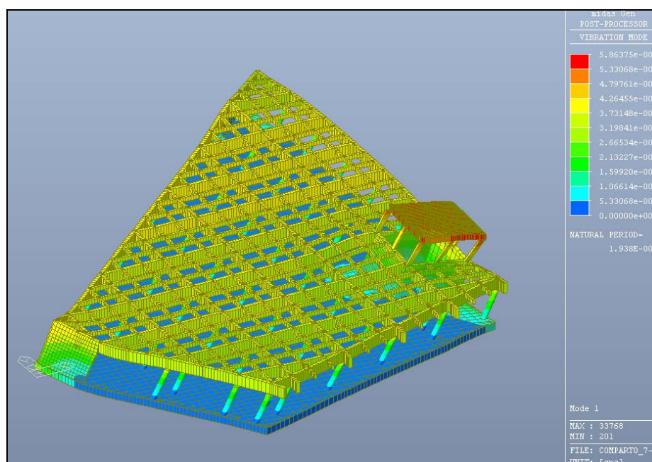
Figura 6.6: Modo di vibrare n. 1
