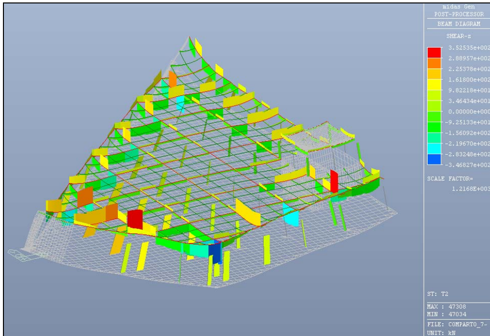
Figura 6.39: Caso di carico T2 (termico) – Valore del taglio
