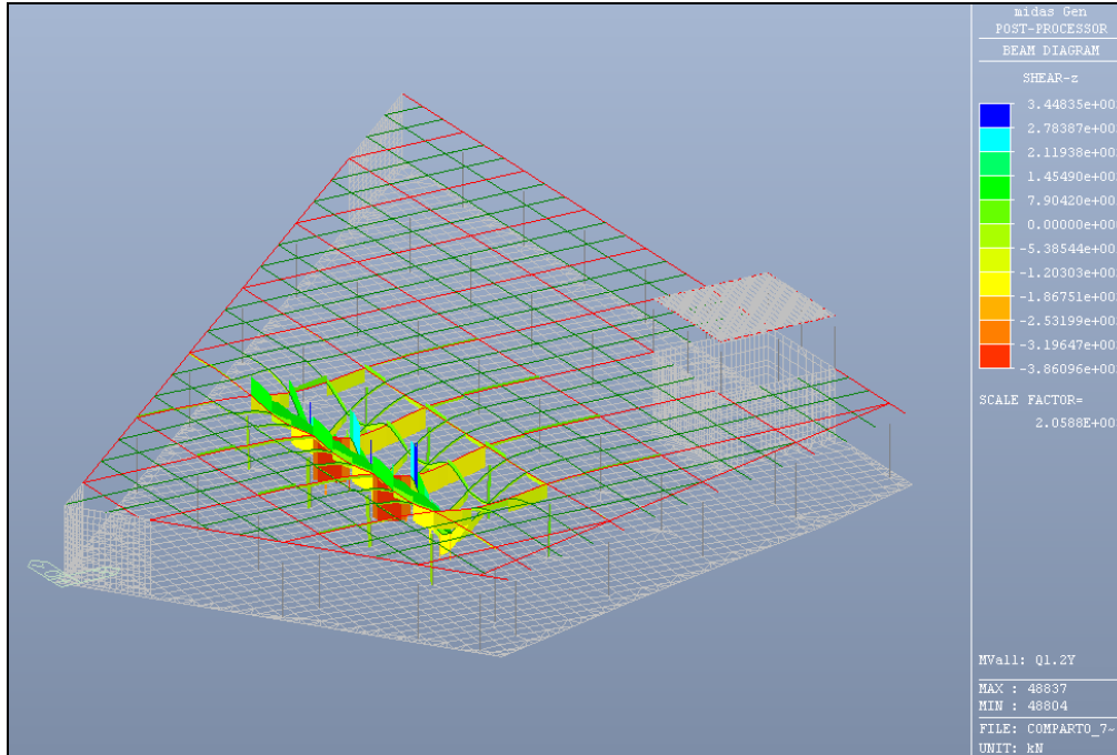
Figura 6.30: Caso di carico Q1 (traffico) in dir Y (travi secondarie) – Valore del taglio
