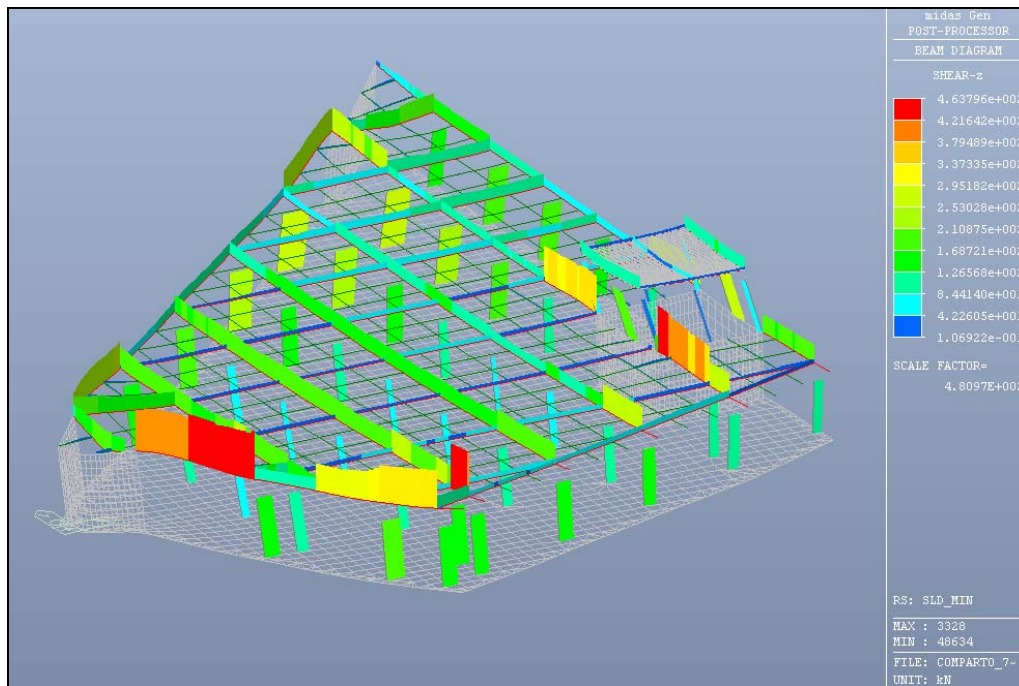
Figura 6.33: SLD min – Valore del taglio
