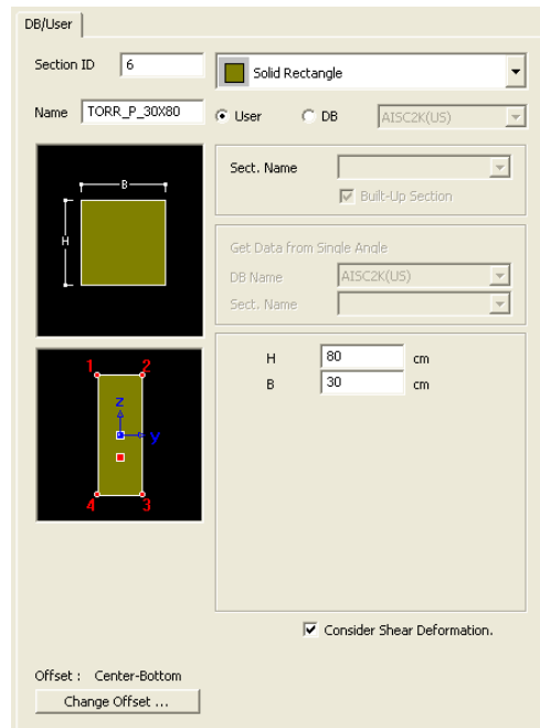
Figura 4.18: Caratteristiche geometriche delle sezioni trasversali delle travi (torrino)
