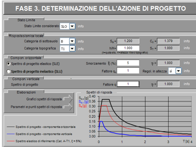
Figura 4.8: Determinazione dello spettro di progetto relativo allo SLO
