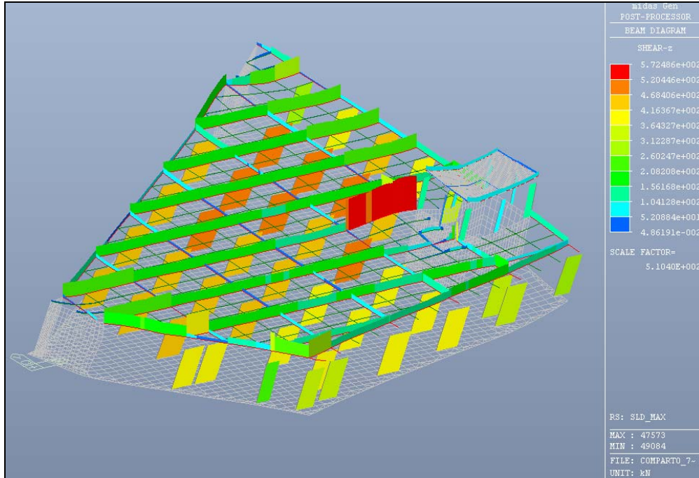
Figura 6.32: SLD max – Valore del taglio
