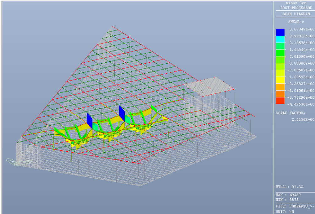
Figura 6.28: Caso di carico Q1 (traffico) in dir X (travi secondarie) – Valore del taglio
