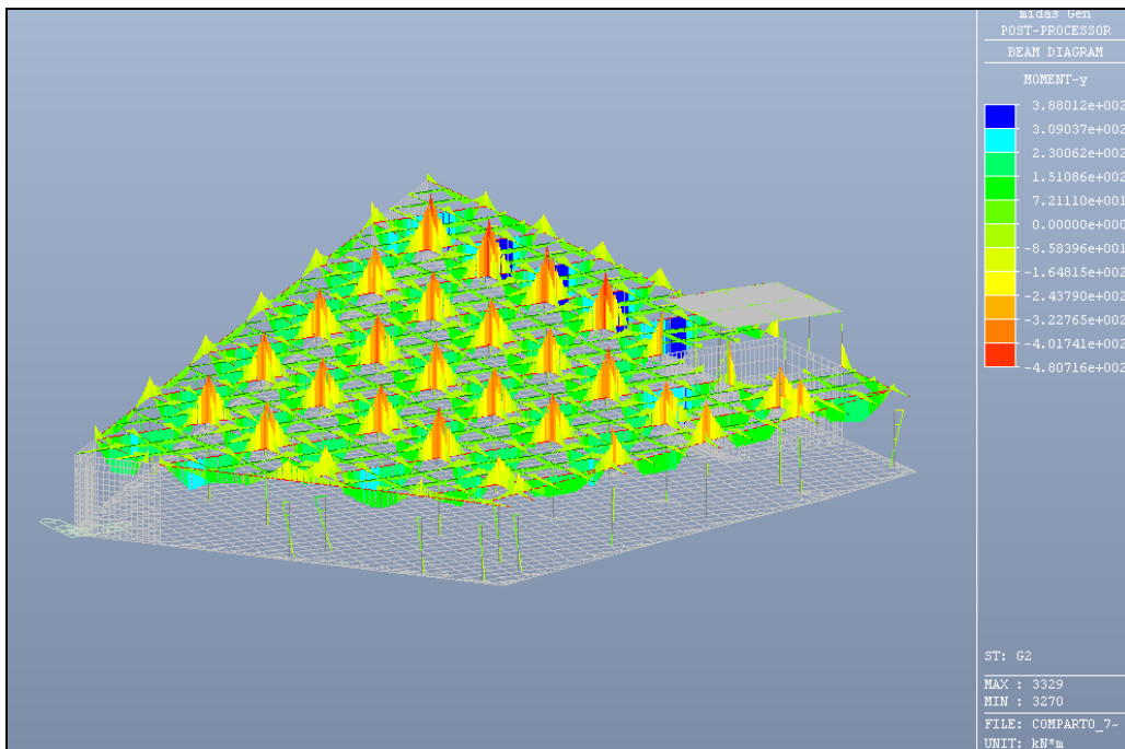
Figura 6.11: Caso di carico G2 – Valore del momento flettente
