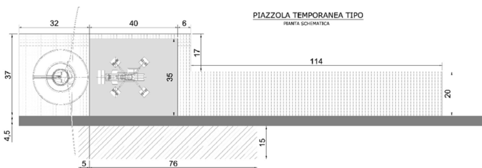
Piazzola temporanea tipo
