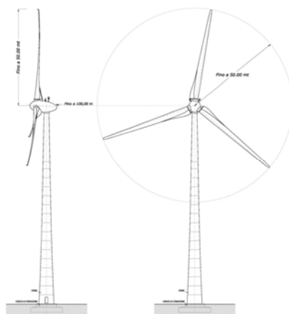
Caratteristiche aerogeneratore tipo
