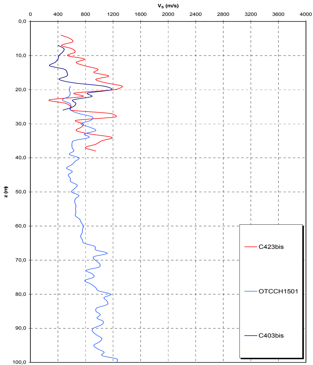
Andamento delle V_s nelle verticali indagate
