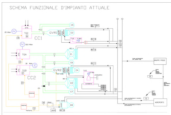
Immagine 1: Schema impianto attuale
