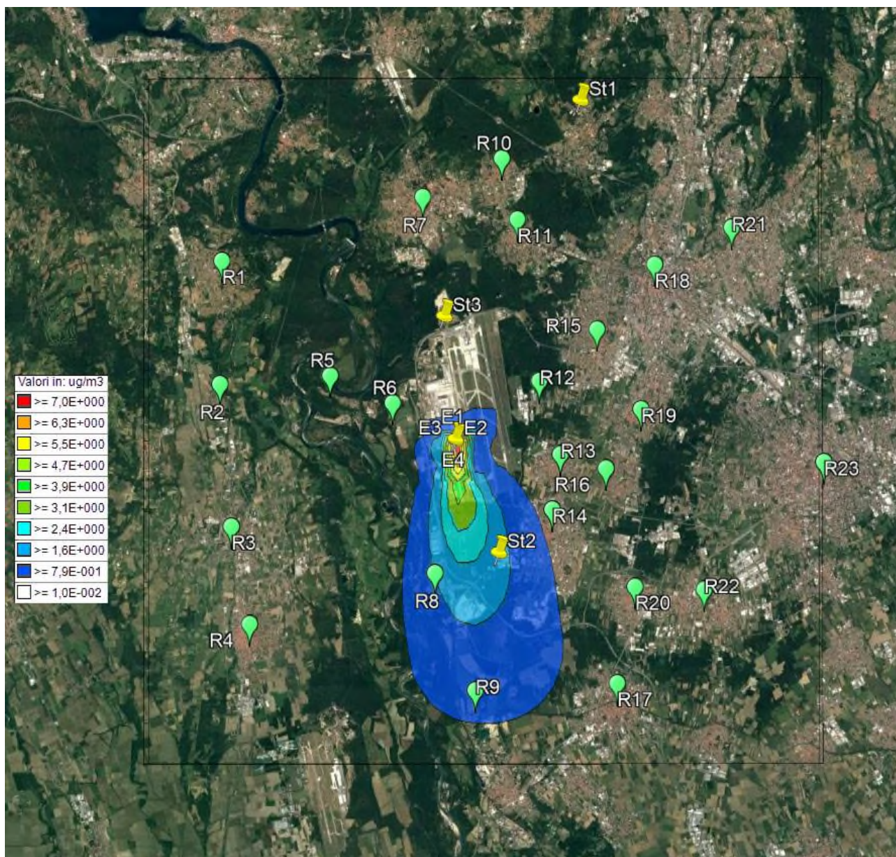
Immagine 9: - modellizzazione NOx espressi come NO 2 - valore medio 1h/anno ( \mu\text{g}/\text{m}^3 )
