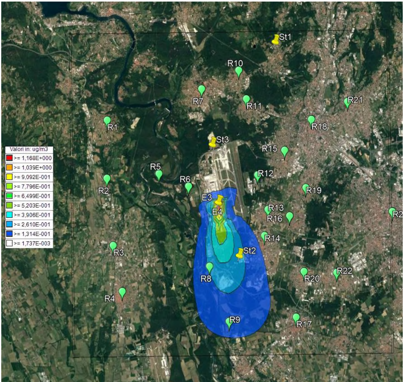
Immagine 11: - modellizzazione NO x espressi come NO 2 - valore medio 1h/anno (µg/m 3 )
