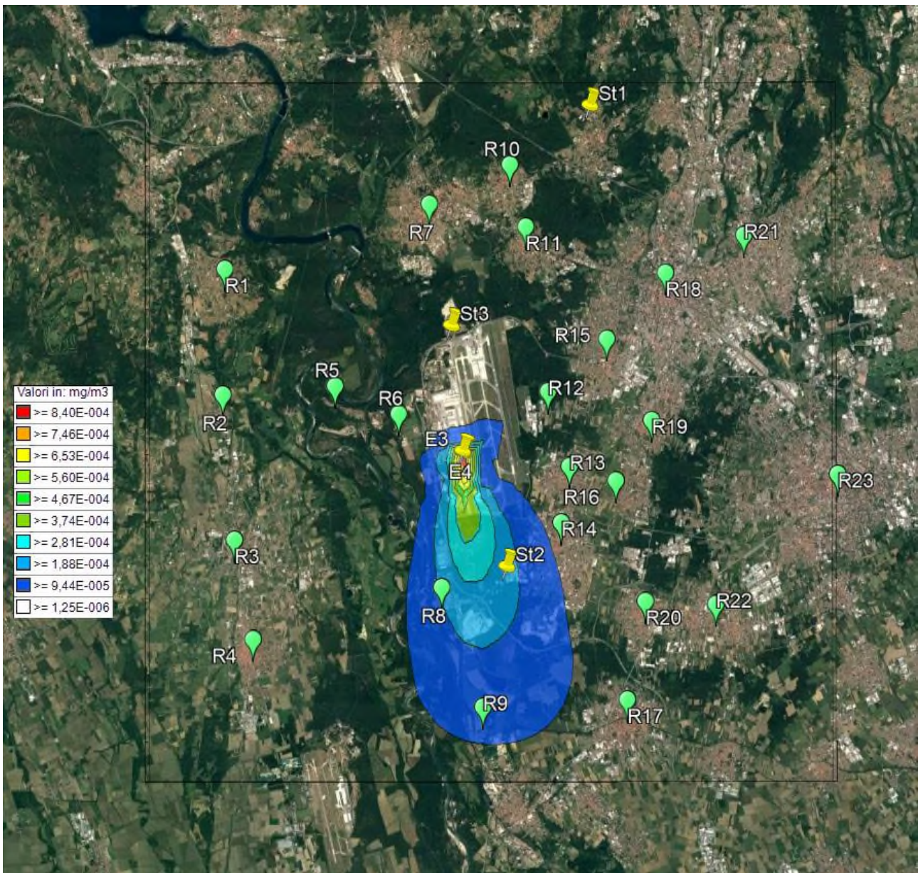
Immagine 12: - modellizzazione CO - valore medio 8h/anno (mg/m 3 )
