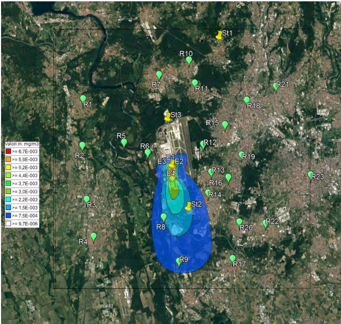
Immagine 10: - modellizzazione NOx espressi come CO - valore medio 8h/anno (mg/m³)
