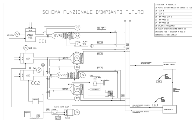
Immagine 2: Schema impianto futuro
