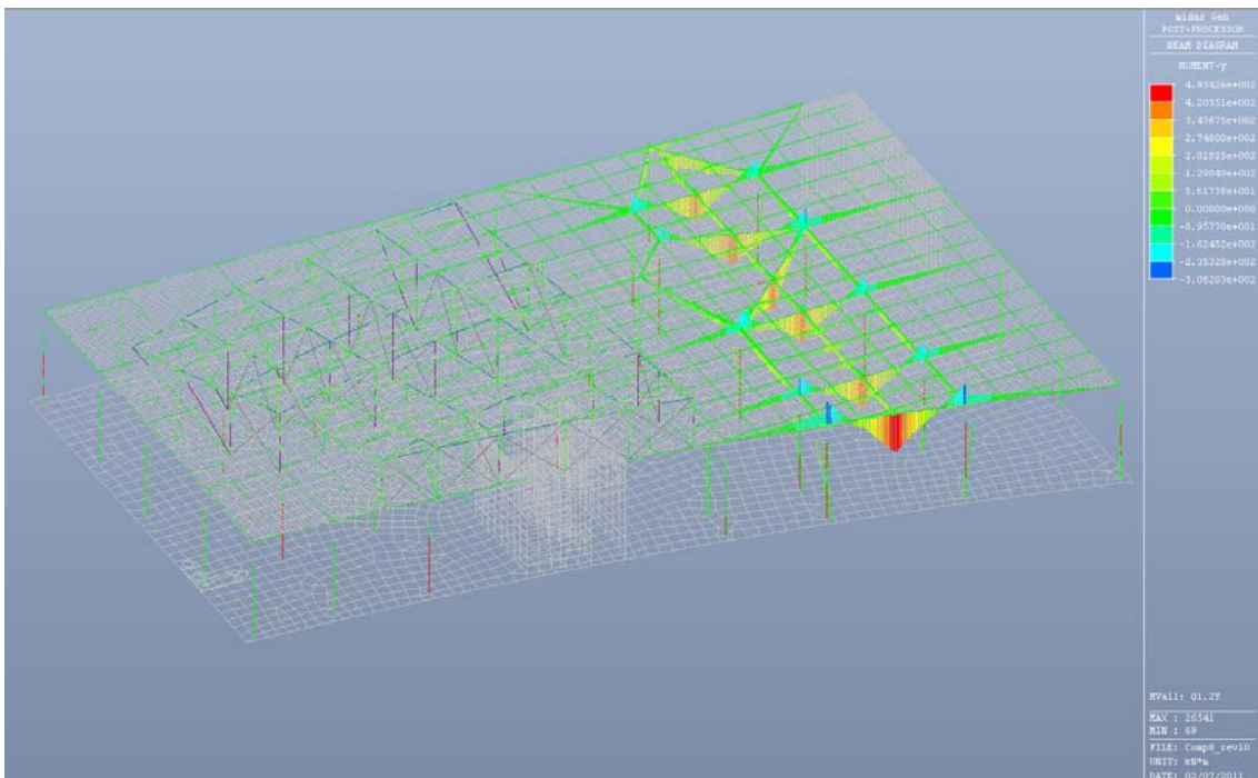
Fig. 6.16 – Momento flettente My - Condizione di carico Q1.2y
