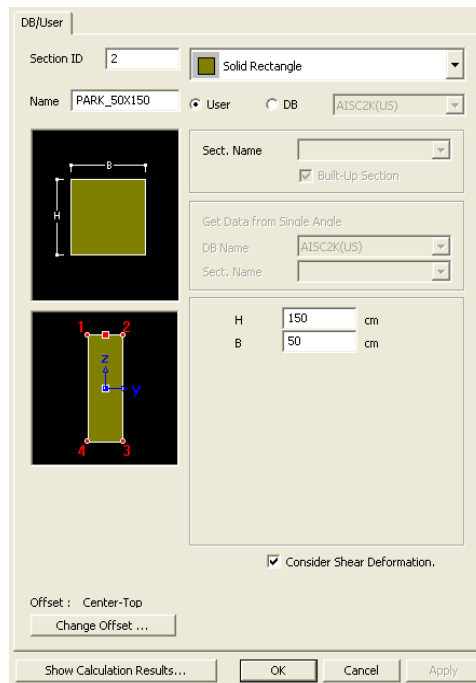
Fig. 4.17 – Caratteristiche geometriche delle sezioni trasversali delle travi principali (piazza)
