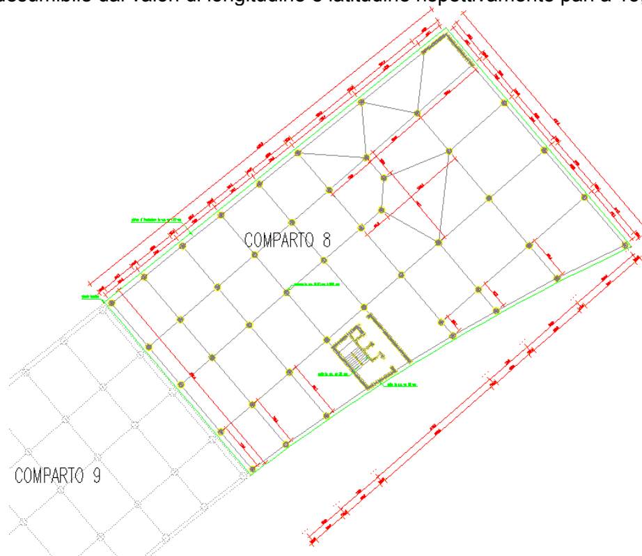
Fig. 4.1 – Carpenteria del primo impalcato del corpo n. 8
