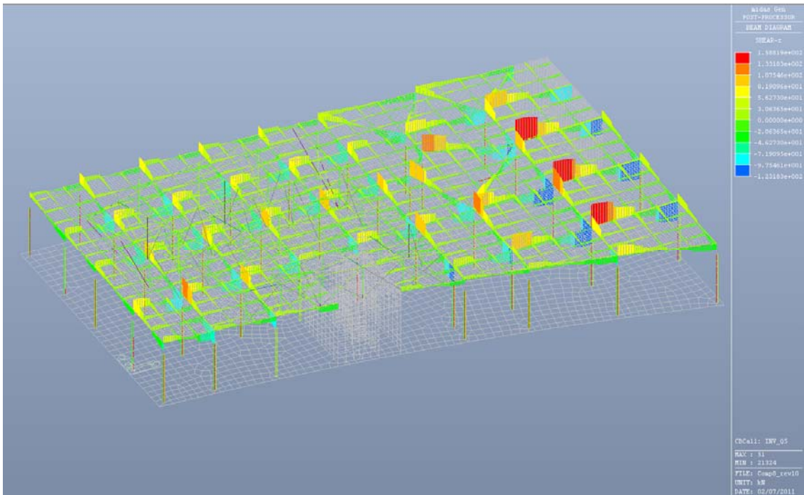
Fig. 6.29 – Taglio Fz - Condizione di carico Inv_Q5
