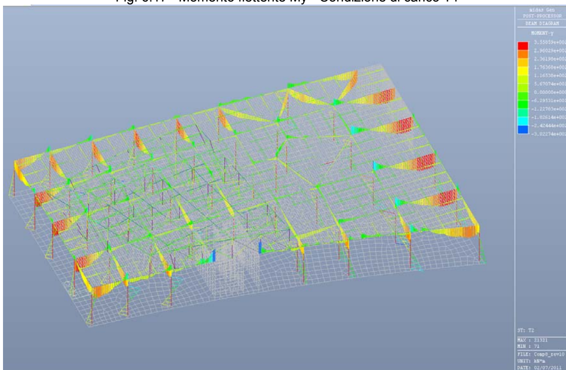
Fig. 6.18 – Momento flettente My - Condizione di carico T2
