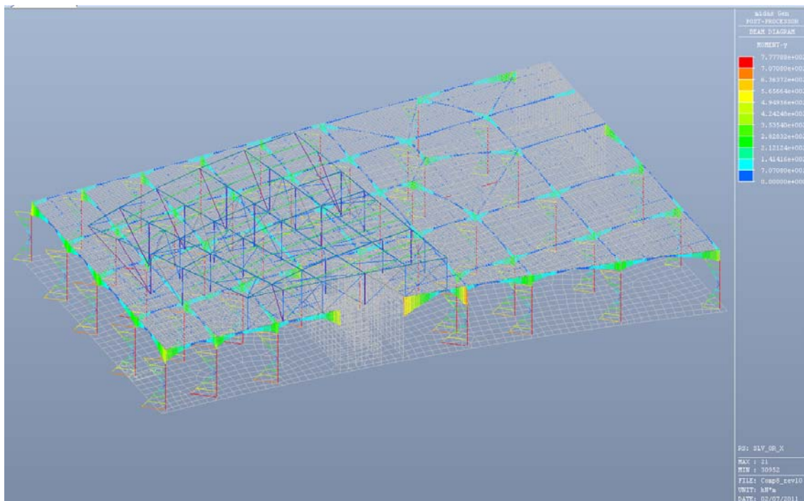
Fig. 6.23 – Momento flettente My - Condizione di carico SLV_Max
