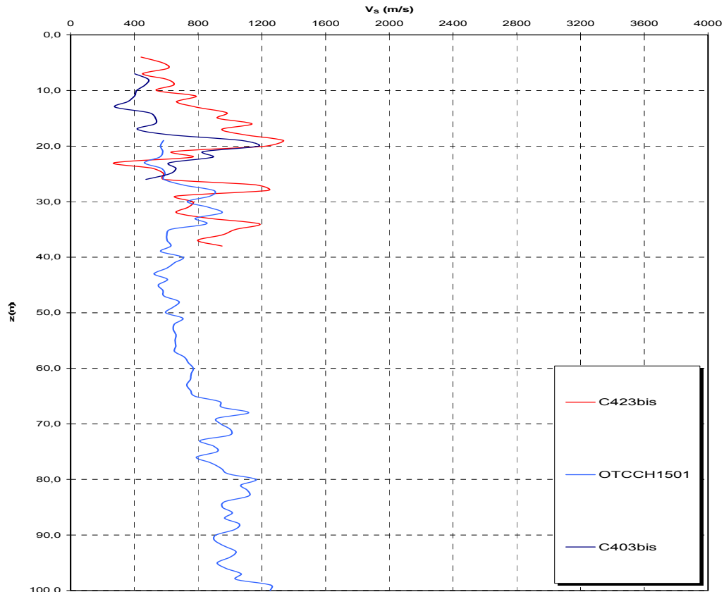
Figura 4.3: Andamento delle Vs nelle verticali indagate
