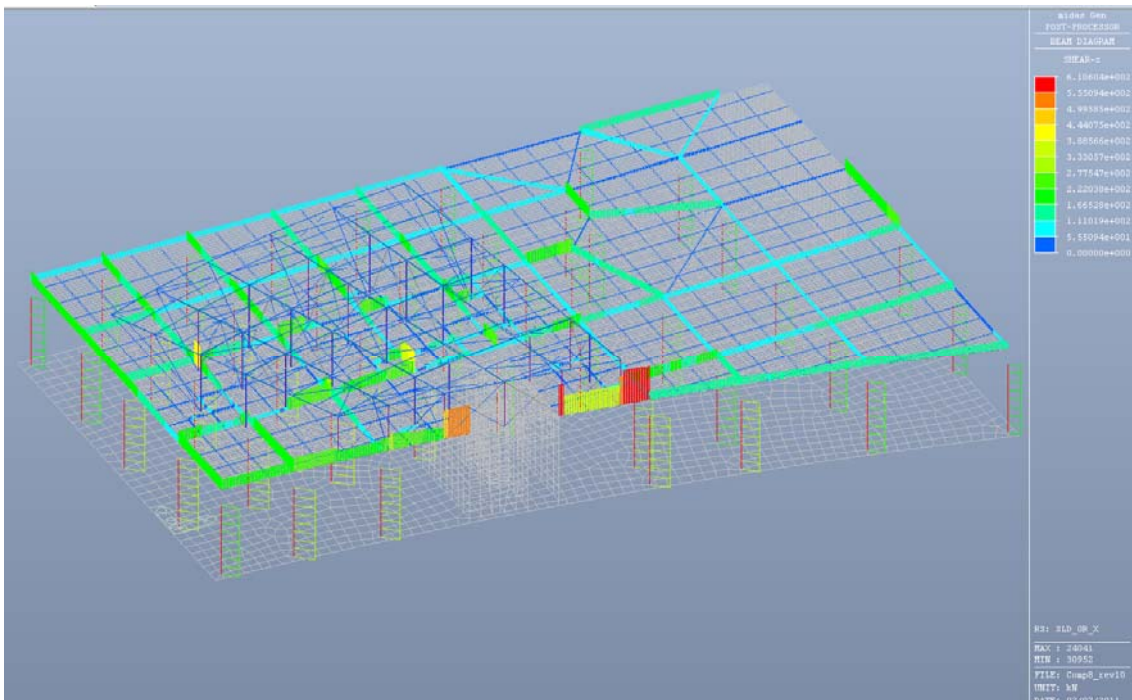
Fig. 6.34 – Taglio Fz - Condizione di carico SLD_Max
