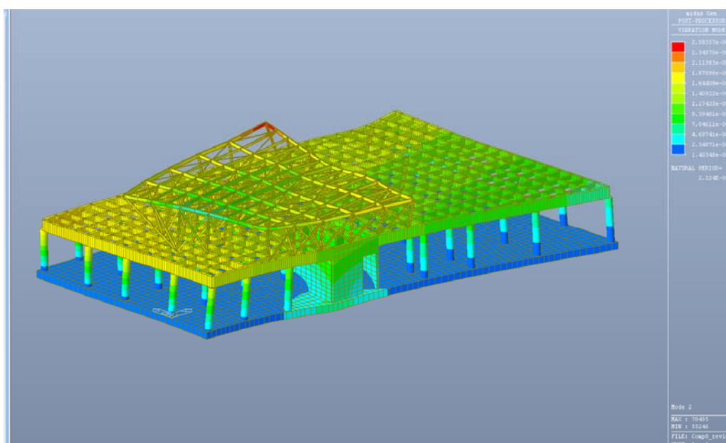
Fig. 6.7 – Modo di vibrare n. 2
