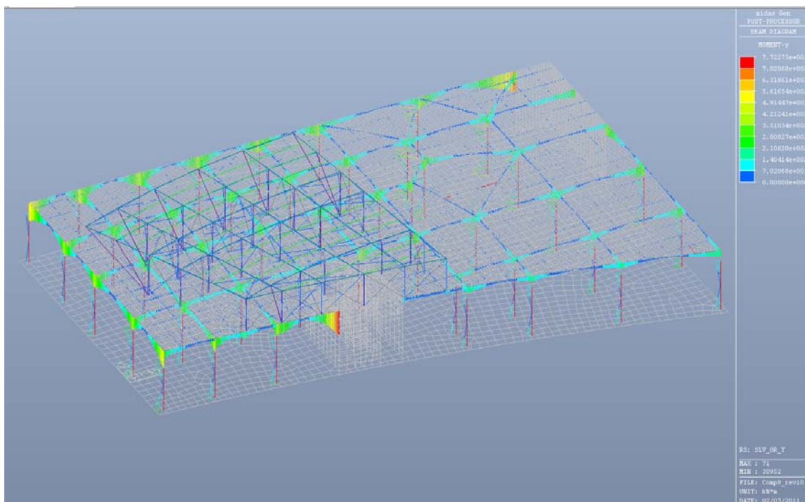
Fig. 6.24 – Momento flettente My - Condizione di carico SLV_Min
