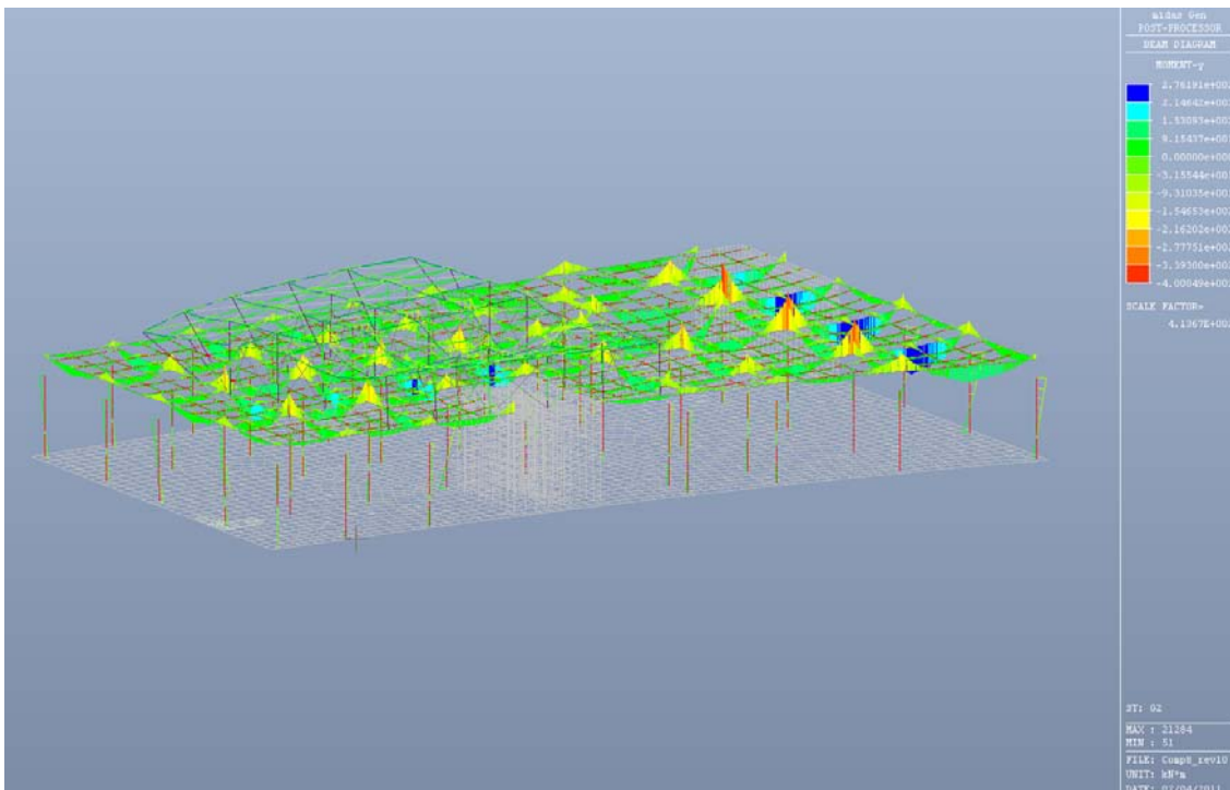
Fig. 6.11 – Momento flettente My - Condizione di carico G2
