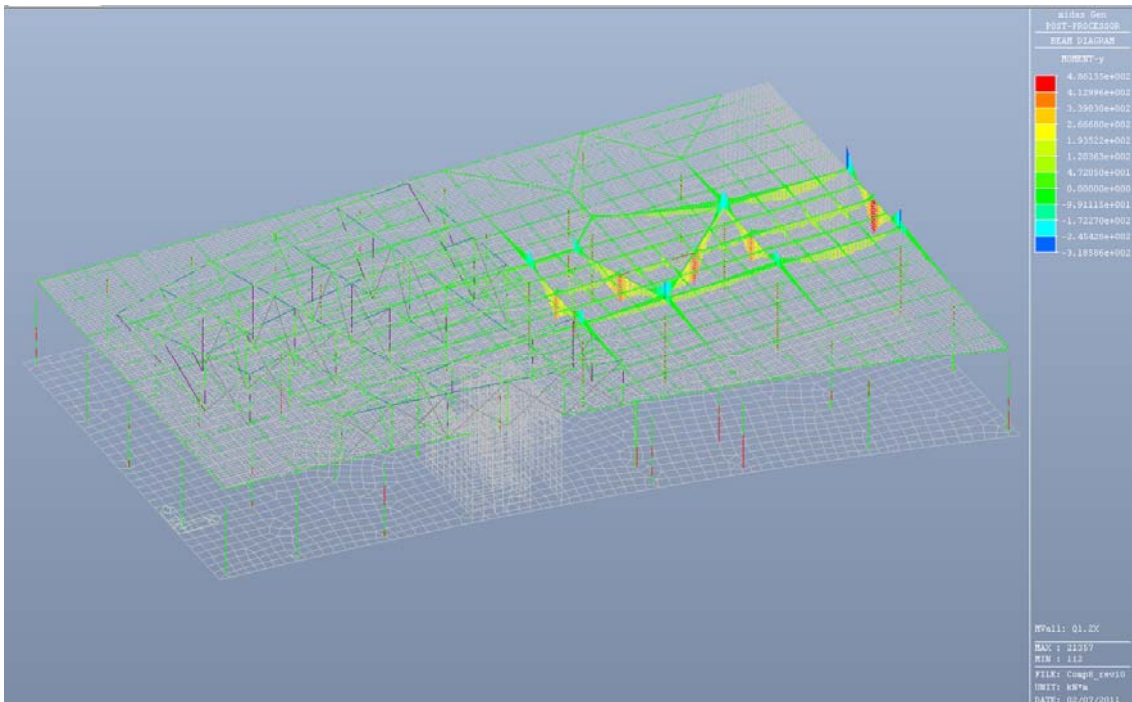
Fig. 6.14 – Momento flettente My - Condizione di carico Q1.2x
