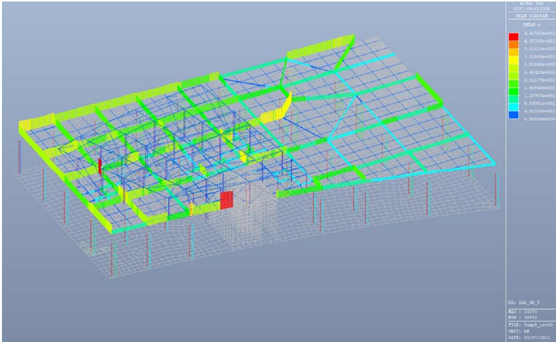
Fig. 6.35 – Taglio Fz - Condizione di carico SLD_Min
