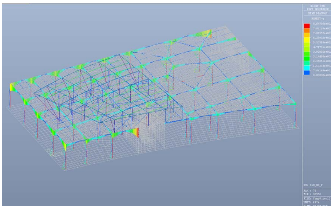
Fig. 6.22 – Momento flettente My - Condizione di carico SLO_Min
