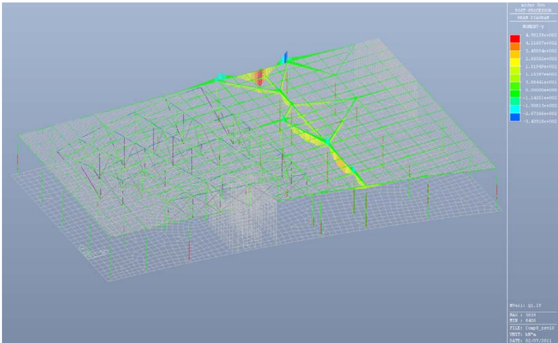
Fig. 6.15 – Momento flettente My - Condizione di carico Q1.1y
