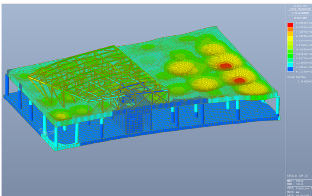
Fig. 6.3 – Deformate per effetto dei carico della folla compatta – Q5 (inviol. max e min spostamenti)
