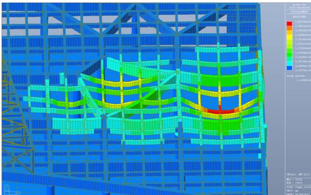
Fig. 6.4 – Deformate per effetto dei carico mobile in dir. X – Q1 (inviol. max e min spostamenti)
