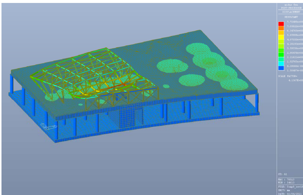
Fig. 6.2 – Deformate per effetto dei carichi permanenti portati – G2
