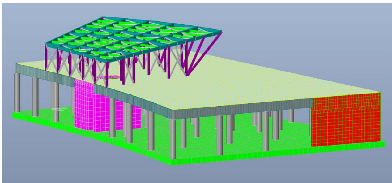
Fig. 4.15 – Vista assometrica del modello di calcolo
