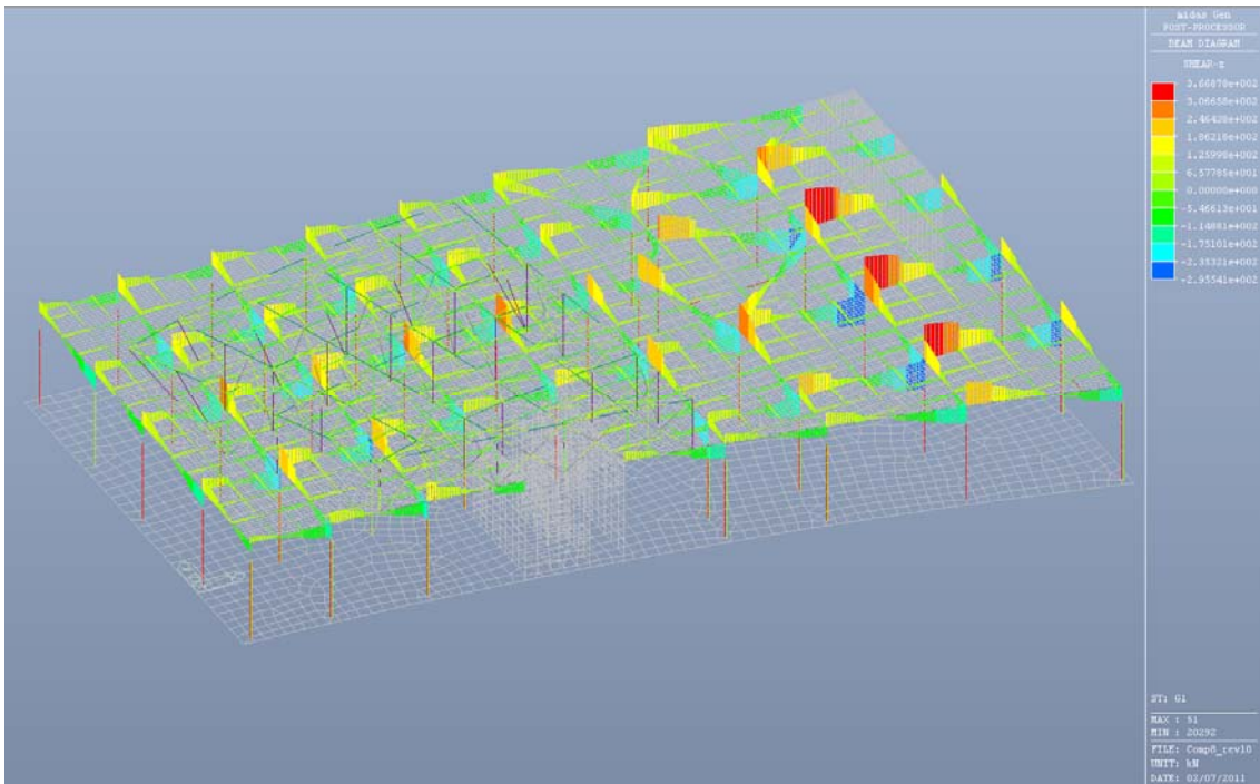
Fig. 6.25 – Taglio Fz - Condizione di carico G1
