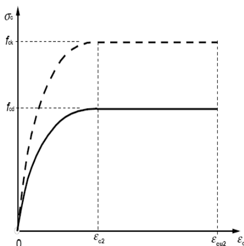
Figura 3.1 – Legame costitutivo del calcestruzzo
