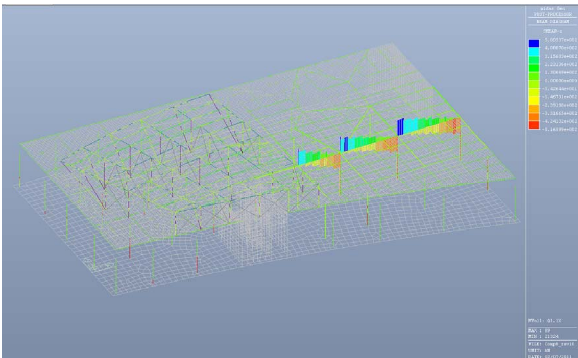
Fig. 6.30 – Taglio Fz - Condizione di carico Q1.1x
