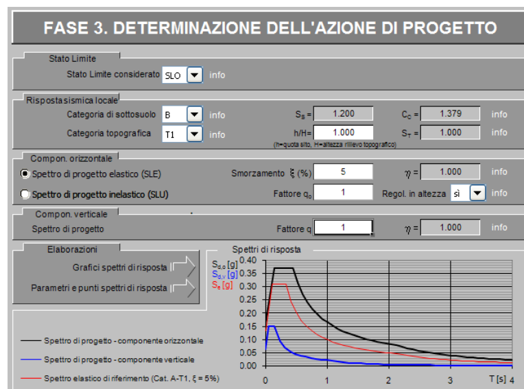
Fig. 4.9 – Determinazione dello spettro di progetto relativo allo SLO
