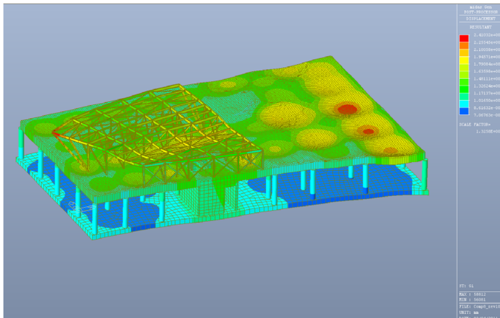
Fig. 6.1 – Deformate per effetto dei pesi propri strutturali – G1
