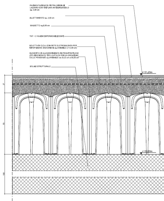
Fig. 1 – Sezione della soletta in elevazione
