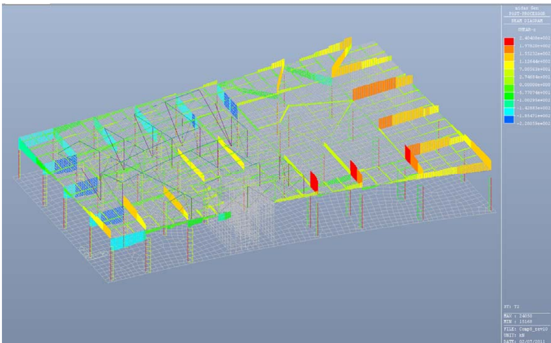
Fig. 6.28 – Taglio Fz - Condizione di carico T2
