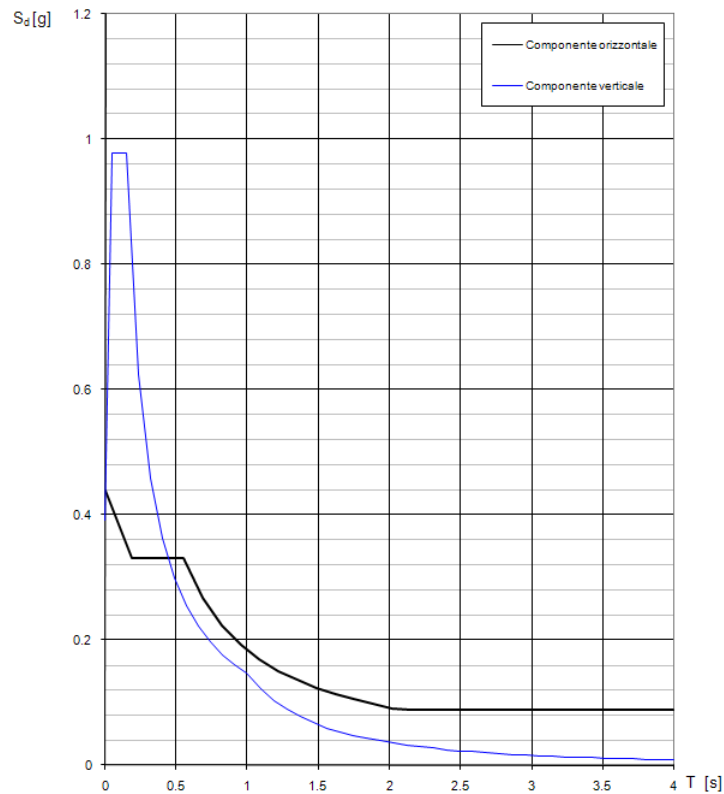
Fig. 4.14 – Spettro di progetto relativo allo SLV
