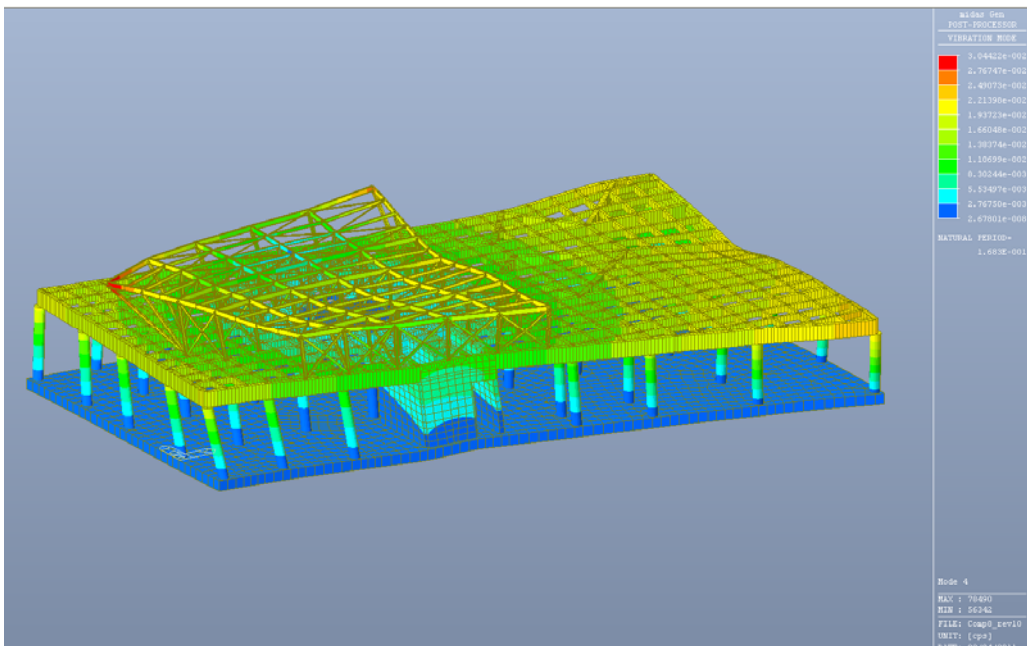
Fig. 6.9 – Modo di vibrare n. 4
