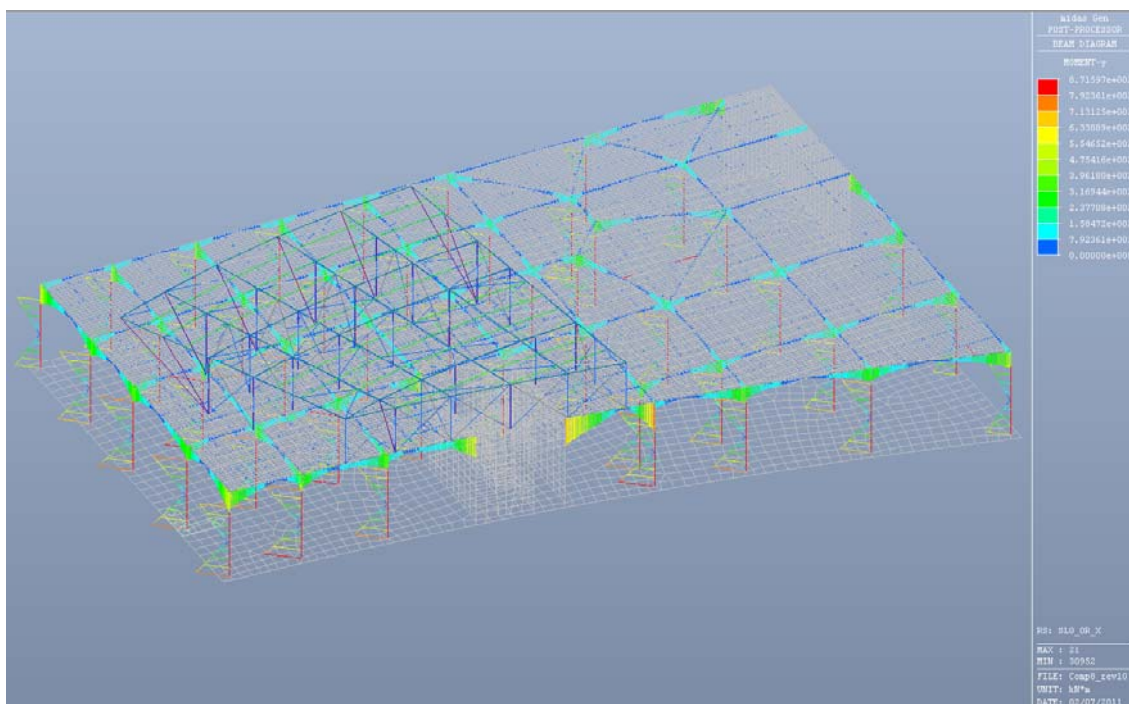
Fig. 6.21 – Momento flettente My - Condizione di carico SLO_Max
