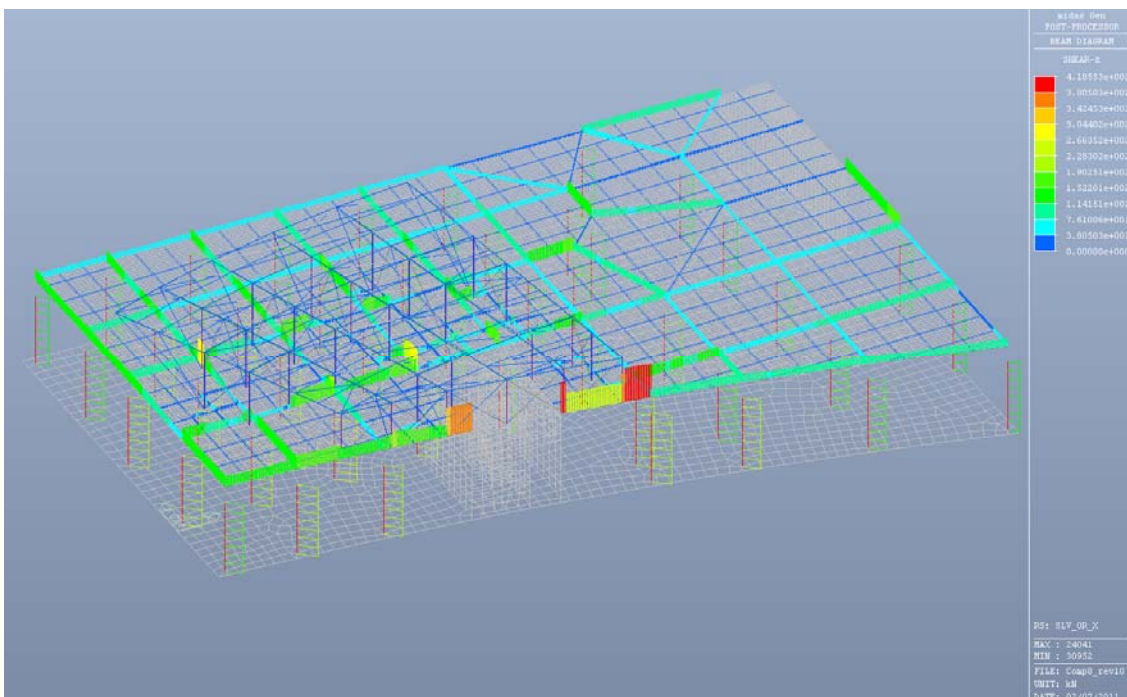
Fig. 6.38 – Taglio Fz - Condizione di carico SLV_Max
