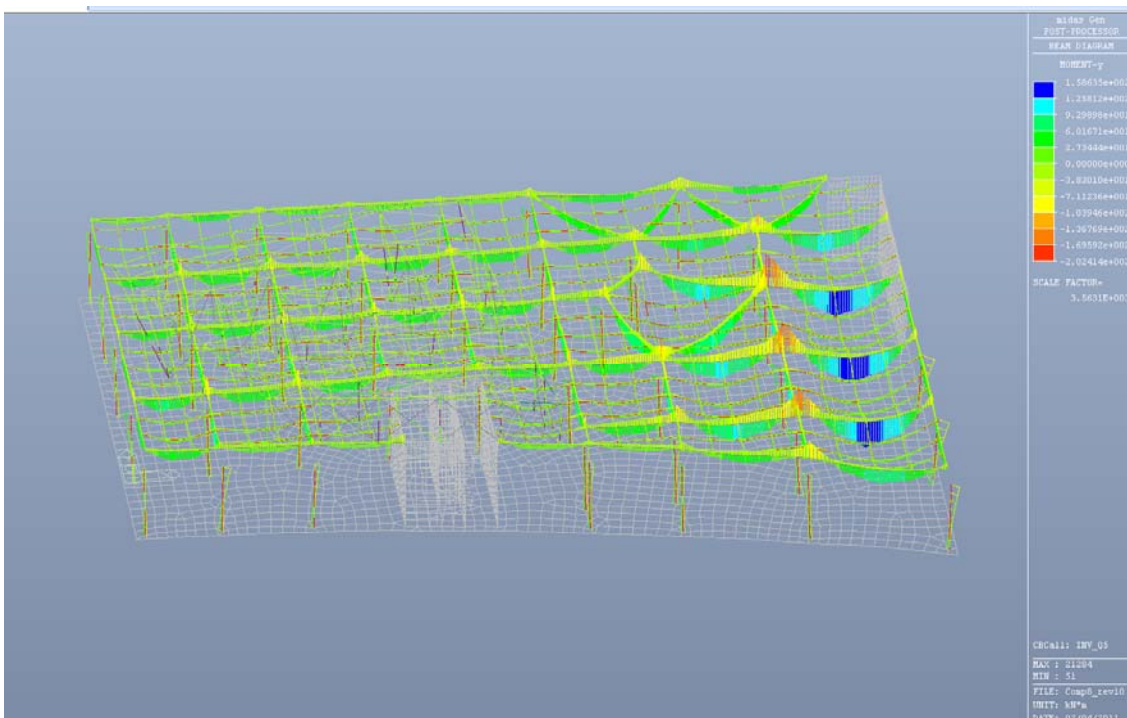
Fig. 6.12 – Momento flettente My - Condizione di carico Inv_Q5
