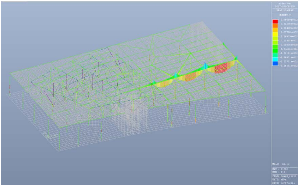
Fig. 6.13 – Momento flettente My - Condizione di carico Q1.1x
