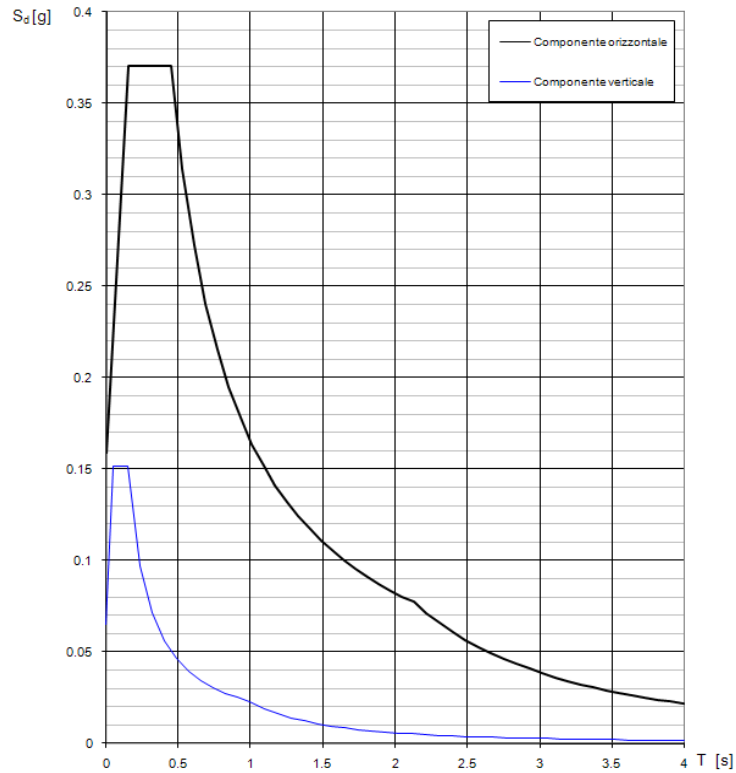
Fig. 4.10 – Spettro di progetto relativo allo SLO
