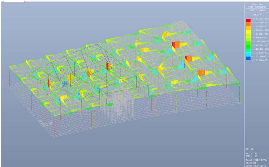
Fig. 6.26 – Taglio Fz - Condizione di carico G2
