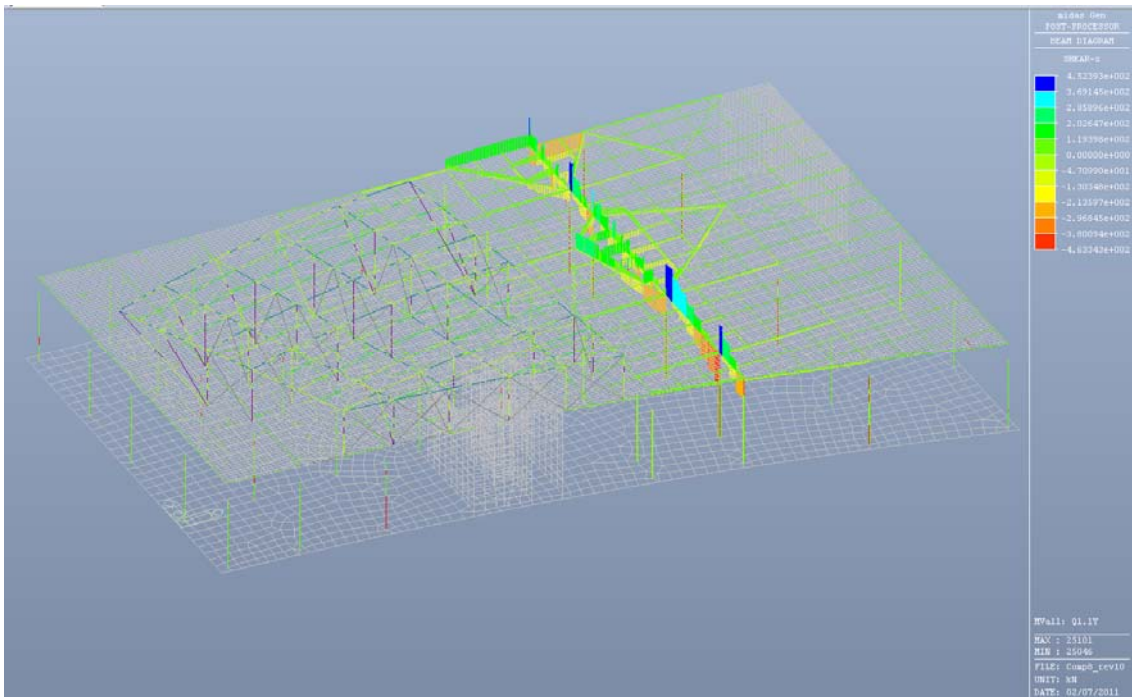
Fig. 6.32 – Taglio Fz - Condizione di carico Q1.1y
