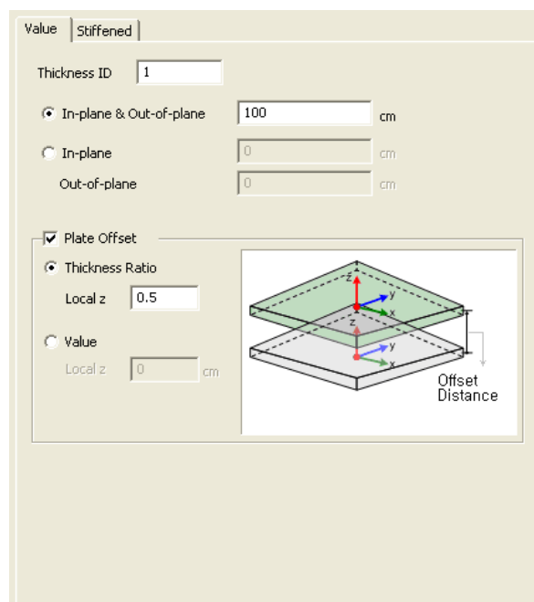
Fig. 4.25 – Caratteristiche geometriche delle solette
