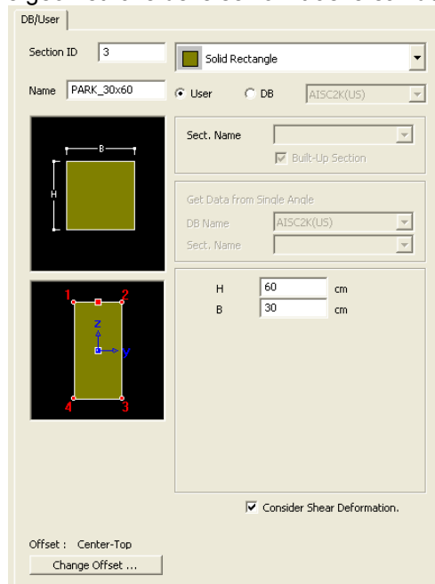
Fig. 4.18 – Caratteristiche geometriche delle sezioni trasversali delle travi secondarie (piazza)
