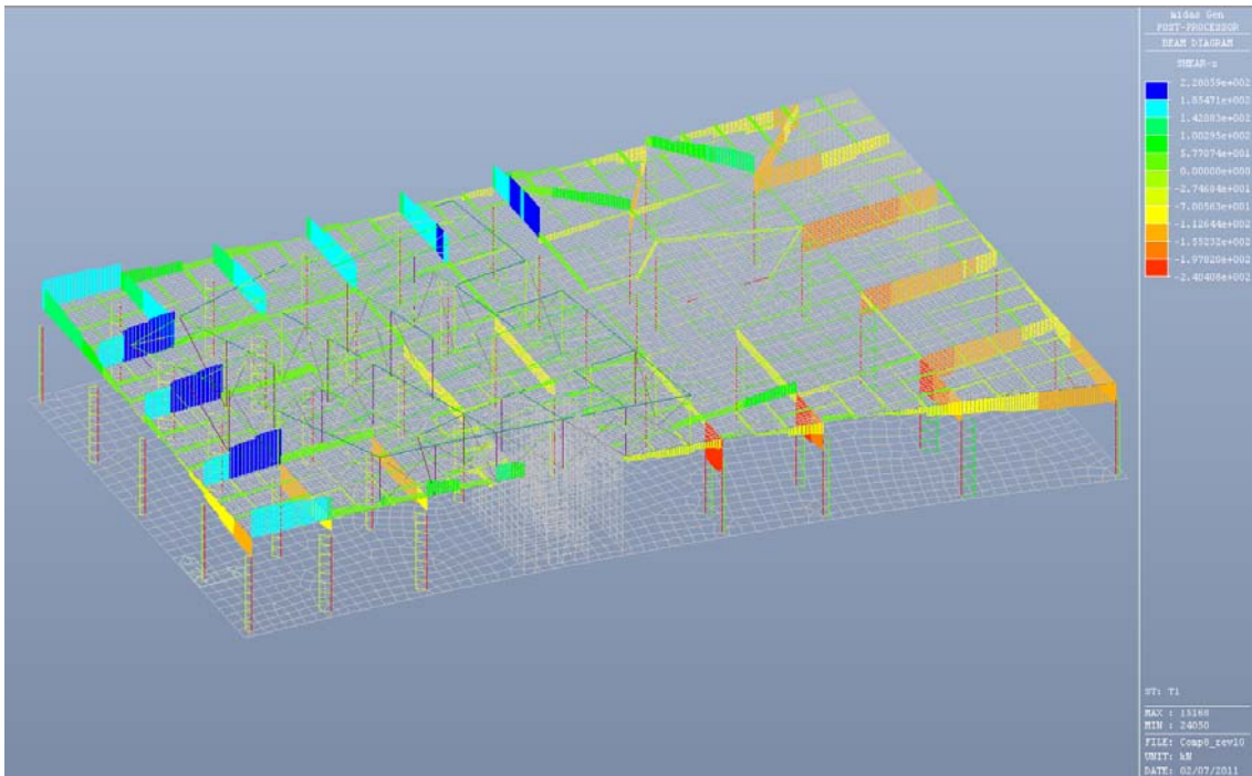
Fig. 6.27 – Taglio Fz - Condizione di carico T1
