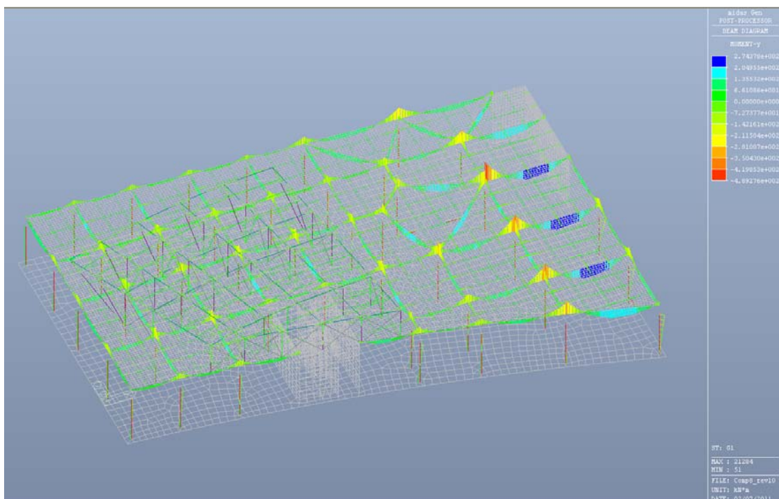
Fig. 6.10 -- Momento flettente My - Condizione di carico G1
