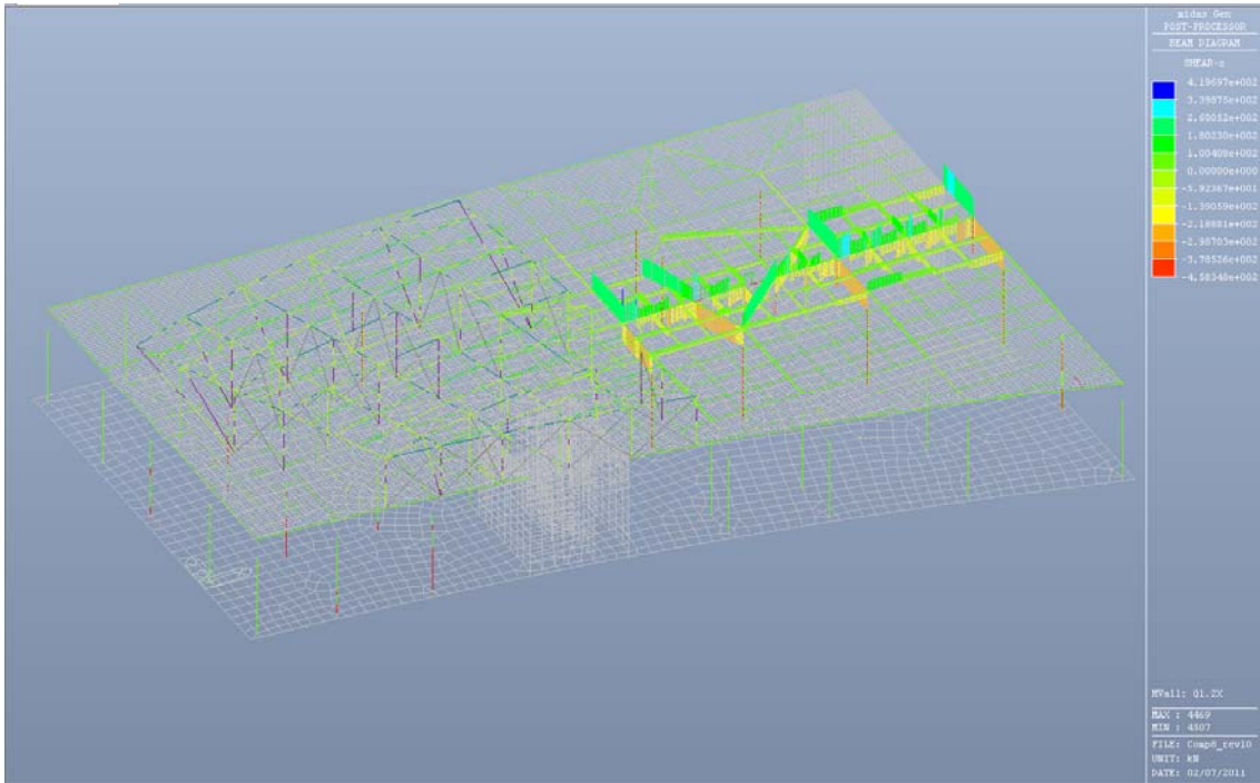
Fig. 6.31 – Taglio Fz - Condizione di carico Q1.2x
