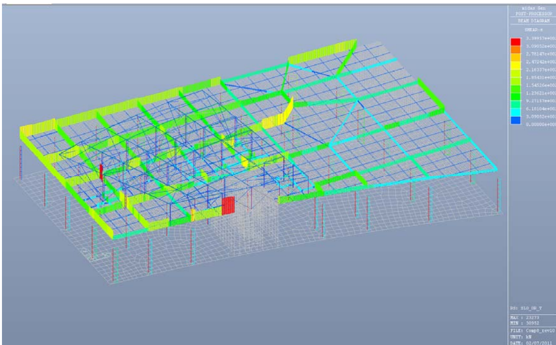
Fig. 6.37 – Taglio Fz - Condizione di carico SLO_Min
