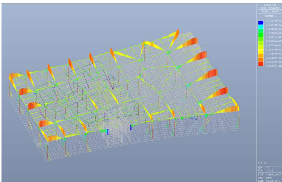
Fig. 6.17– Momento flettente My - Condizione di carico T1
