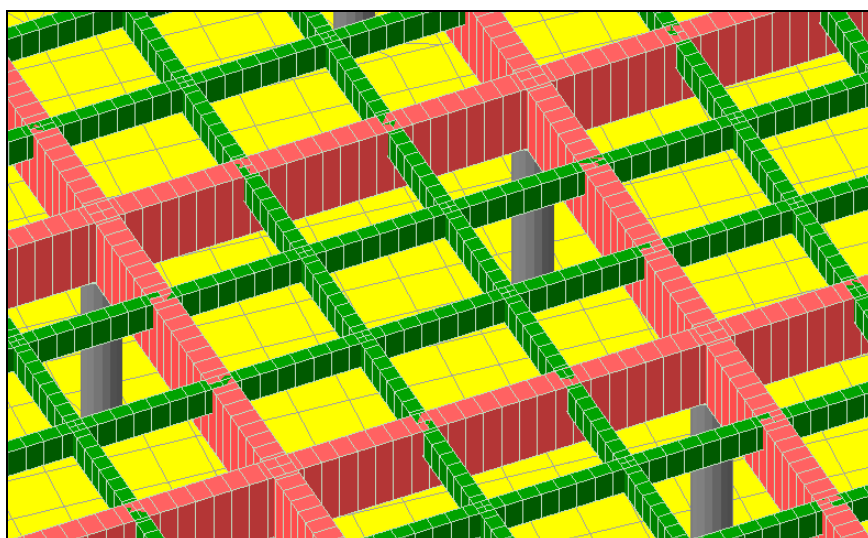
Fig. 4.16 – Particolare delle travi principali (in rosso) e delle travi secondarie (in verde)
