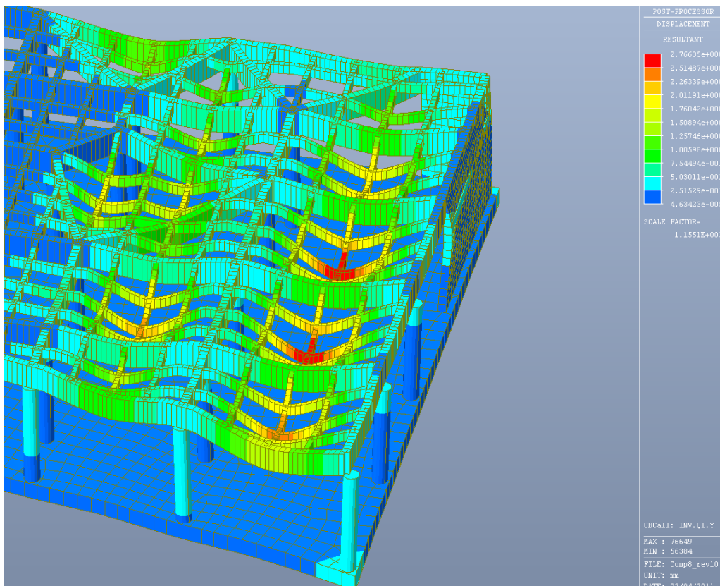
Fig. 6.5 – Deformate per effetto dei carico mobile in dir. Y – Q1 (inviol. max e min spostamenti)
