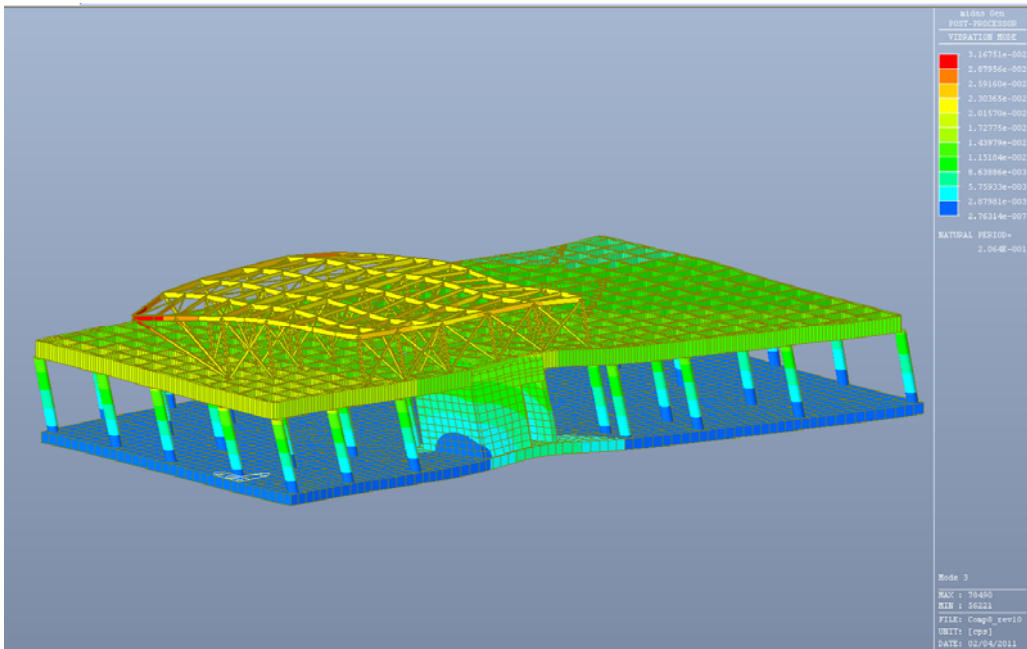
Fig. 6.8 – Modo di vibrare n. 3
