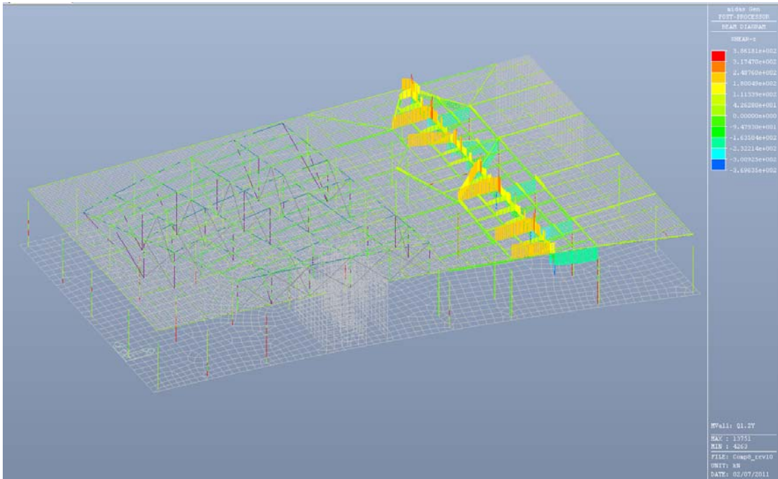
Fig. 6.33 – Taglio Fz - Condizione di carico Q1.2y
