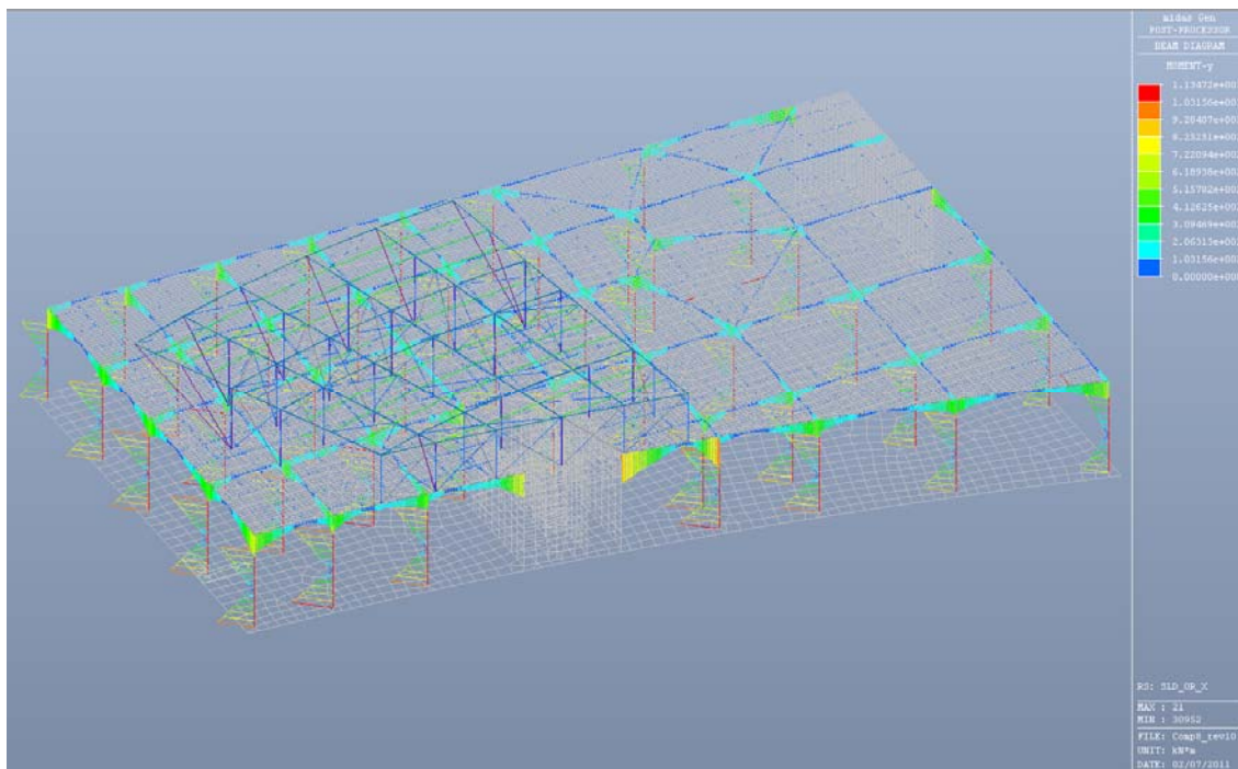
Fig. 6.19 – Momento flettente My - Condizione di carico SLD_Max
