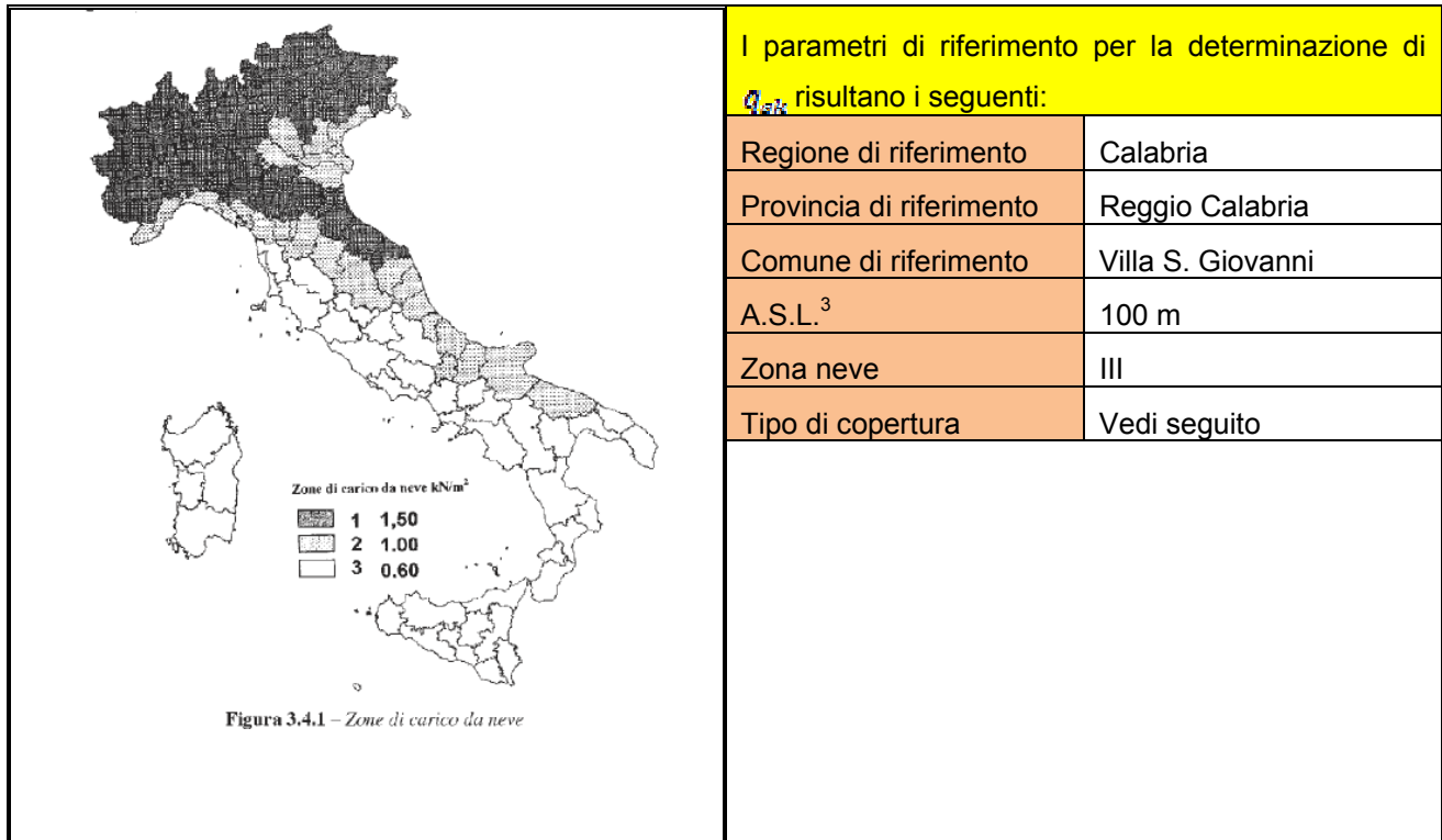
Fig. 4.6: Parametri valutazione azione da neve
