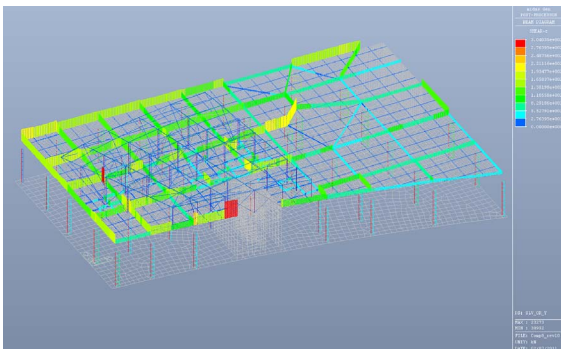
Fig. 6.39 – Taglio Fz - Condizione di carico SLV_Min
