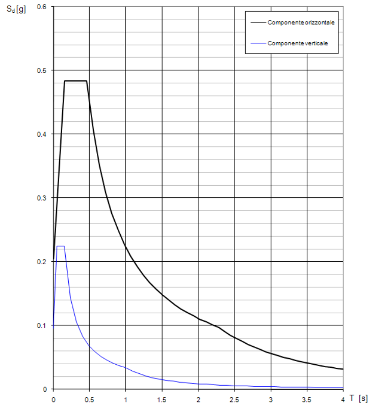
Fig. 4.12 – Spettro di progetto relativo allo SLD
