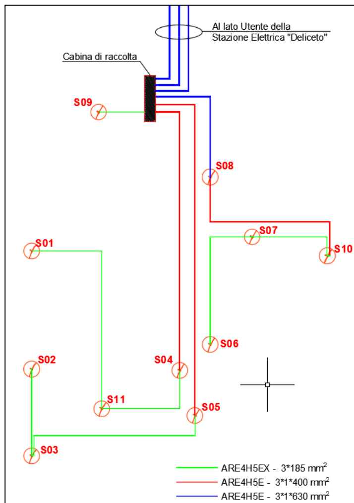
Figura 3 - Schema di connessione elettrica dell'impianto eolico in progetto
