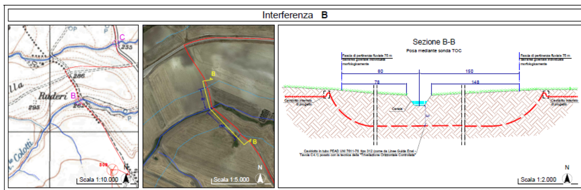
Figura 44--Stralcio studio degli attraversamenti - Fosso Tufara - VWS-CIV-PLN-017 – Studio degli attraversamenti
