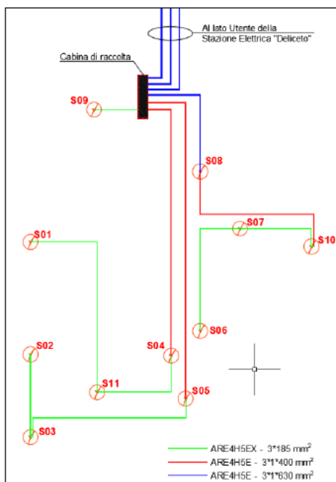
Figura 42 - Schema di connessione elettrica dell'impianto eolico in progetto
