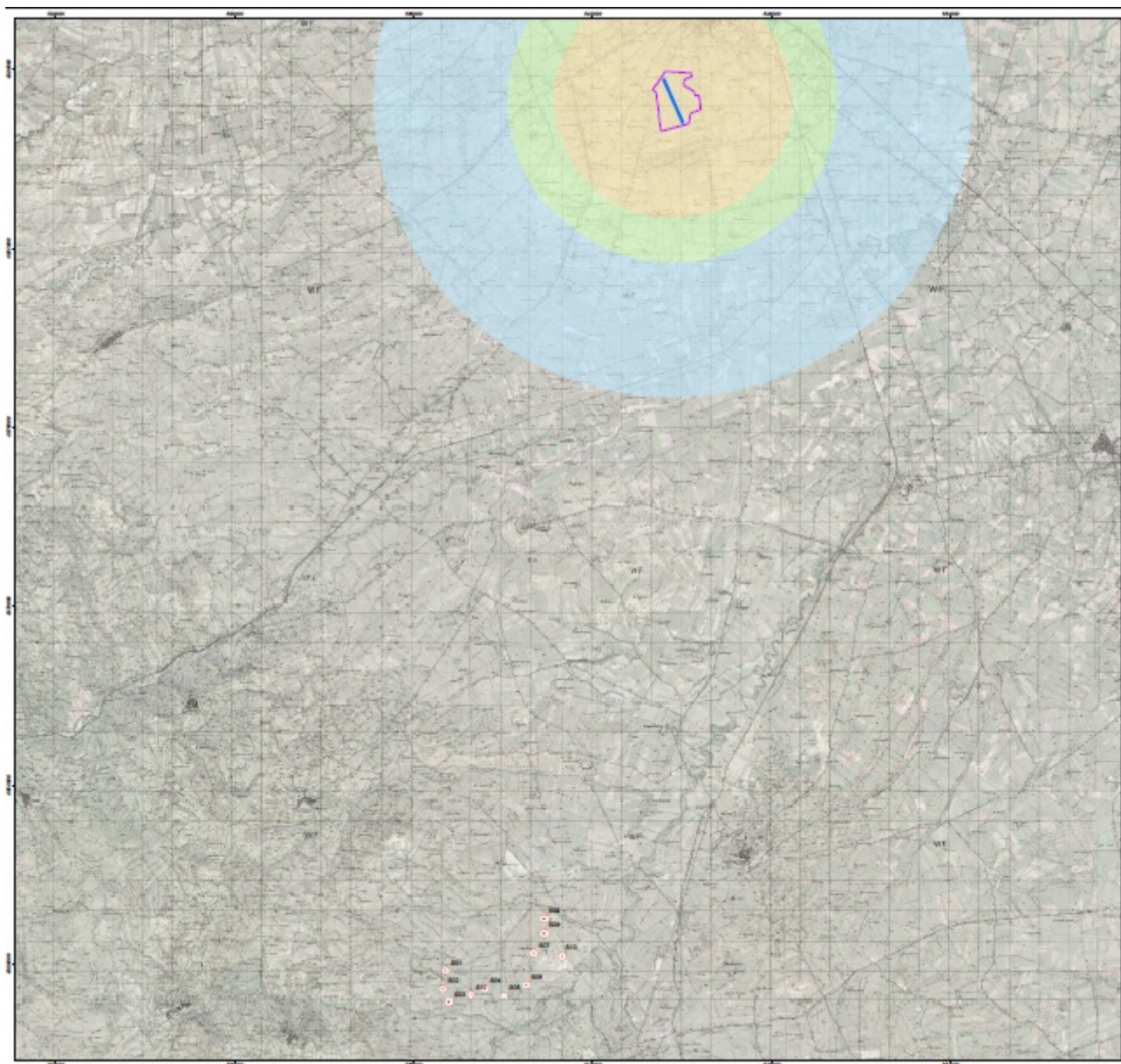
Figura 39 - Stralcio Planimetria Interferenza del Parco Eolico con le infrastrutture di volo
