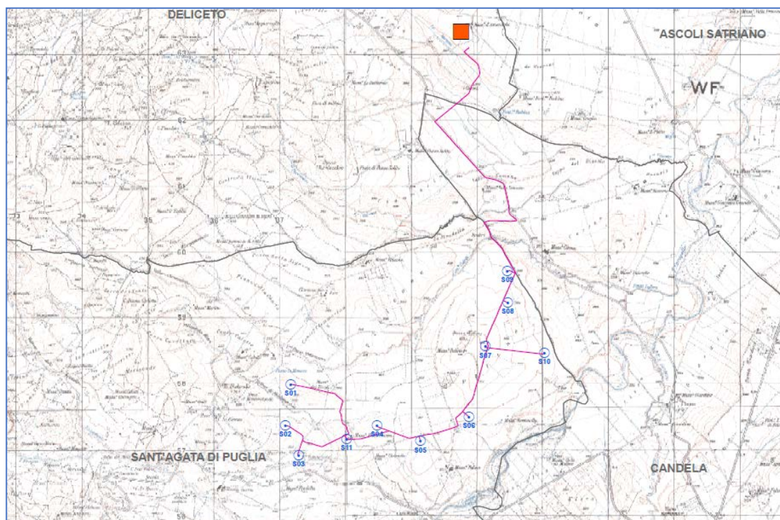
Figura 38 - layout impianto definitivo a n.11 aerogeneratori
