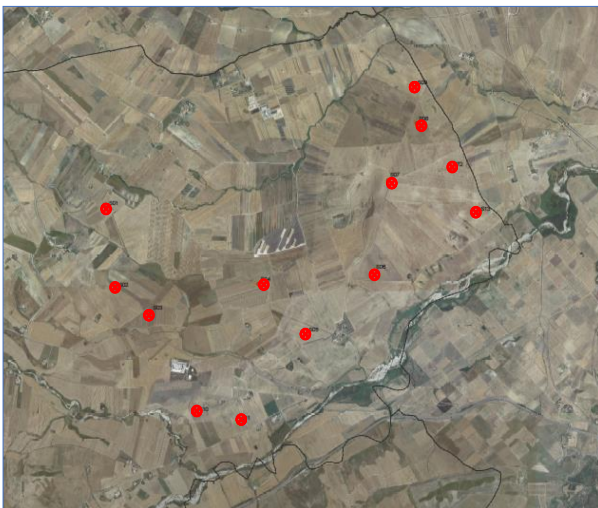
Figura 3 - Ipotesi di layout a 13 aerogeneratori
