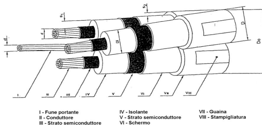
Figura 12 - Esempio di cavo
