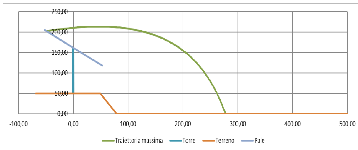
Figura 5 - Traiettoria del moto di un frammento di 10 m, a seguito di rottura
