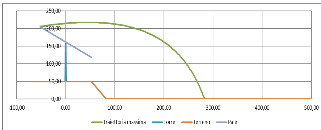
Figura 7 - Traiettoria del moto di un frammento di 1 m, a seguito di rottura
