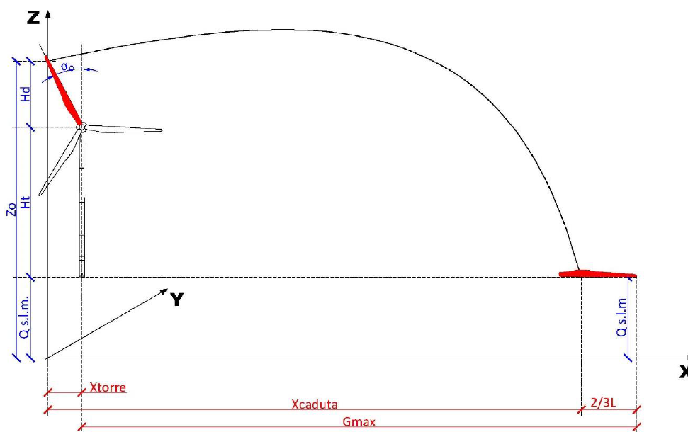
Figura 2 - Modello geometrico del distacco della pala intera
