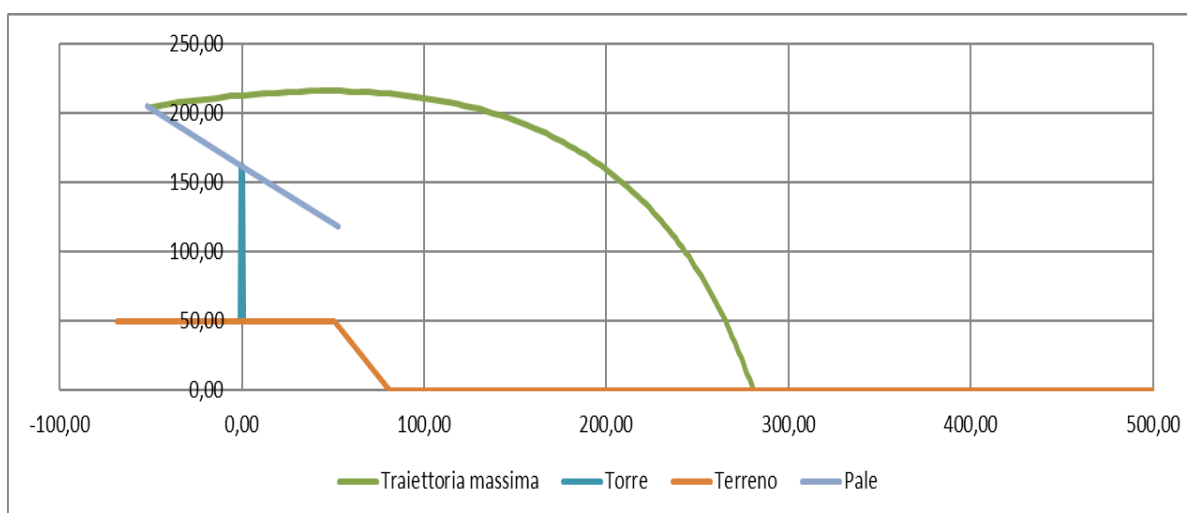
Figura 6 - Traiettoria del moto di un frammento di 5 m, a seguito di rottura
