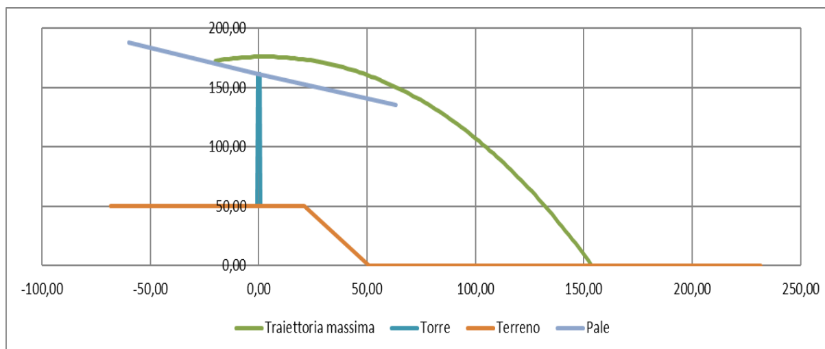
Figura 4 - Traiettoria del moto della pala intera, a seguito del distacco
