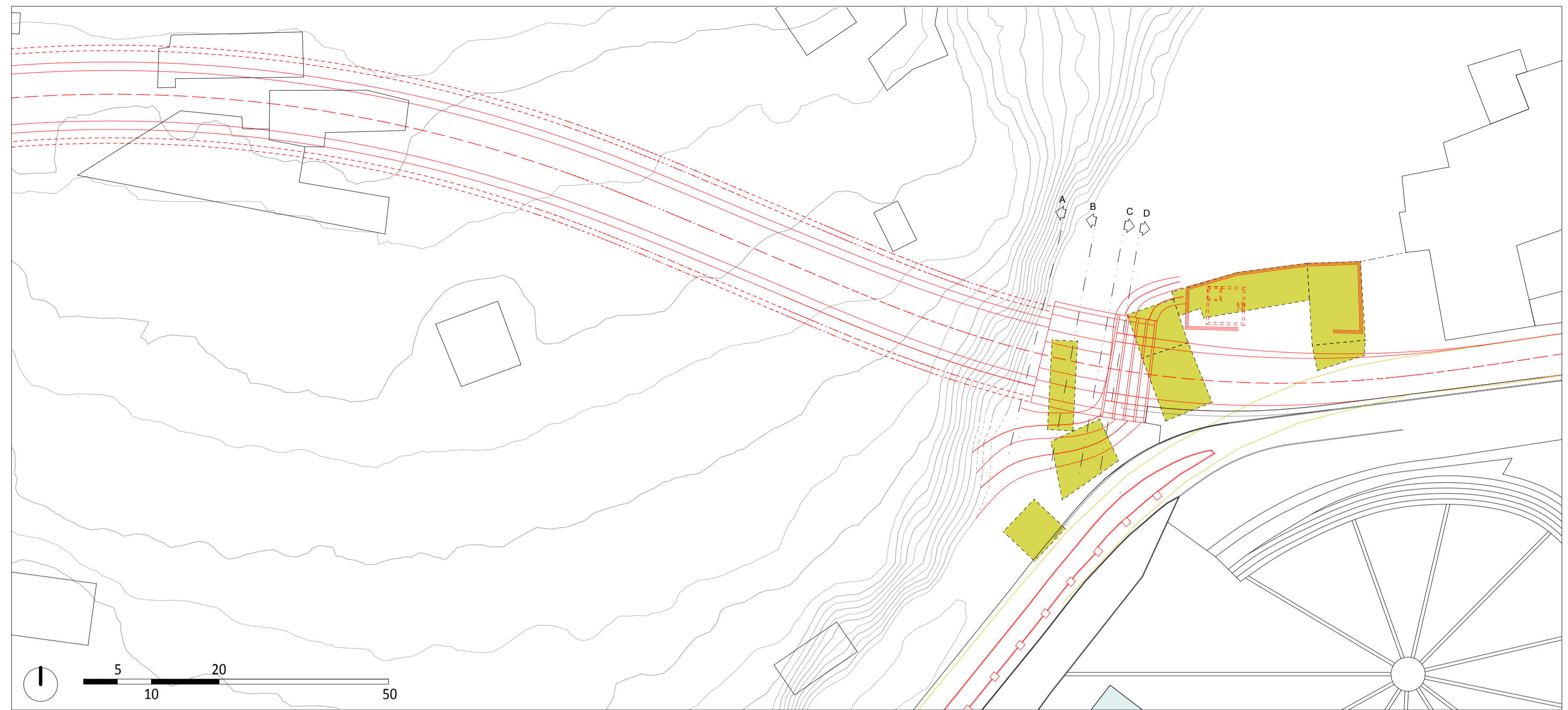
PLANIMETRIA DI CONFRONTO IMBOCCO GALLERIA MAIORI - SCALA 1:500
