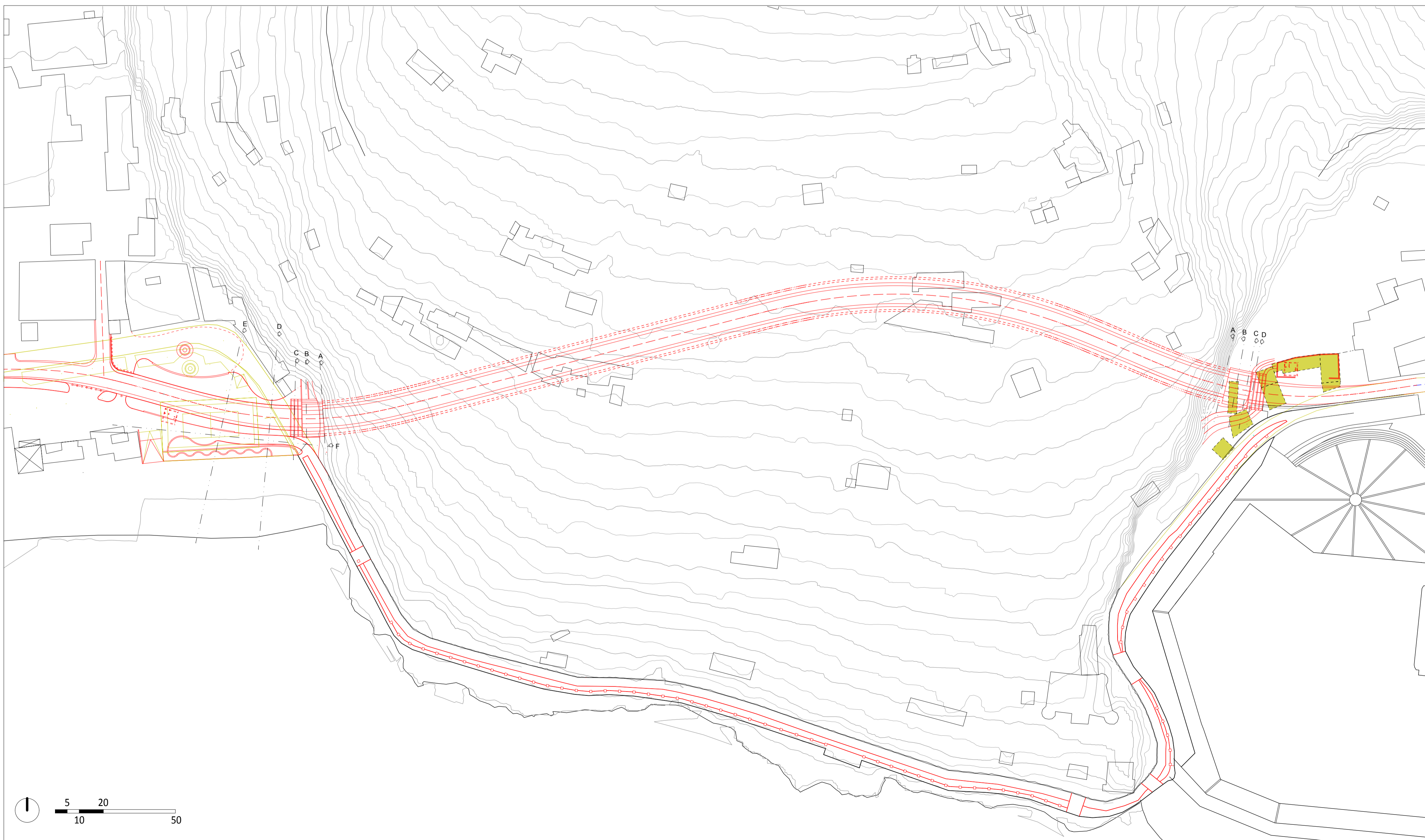
PLANIMETRIA GENERALE DI CONFRONTO - SCALA 1:1000
