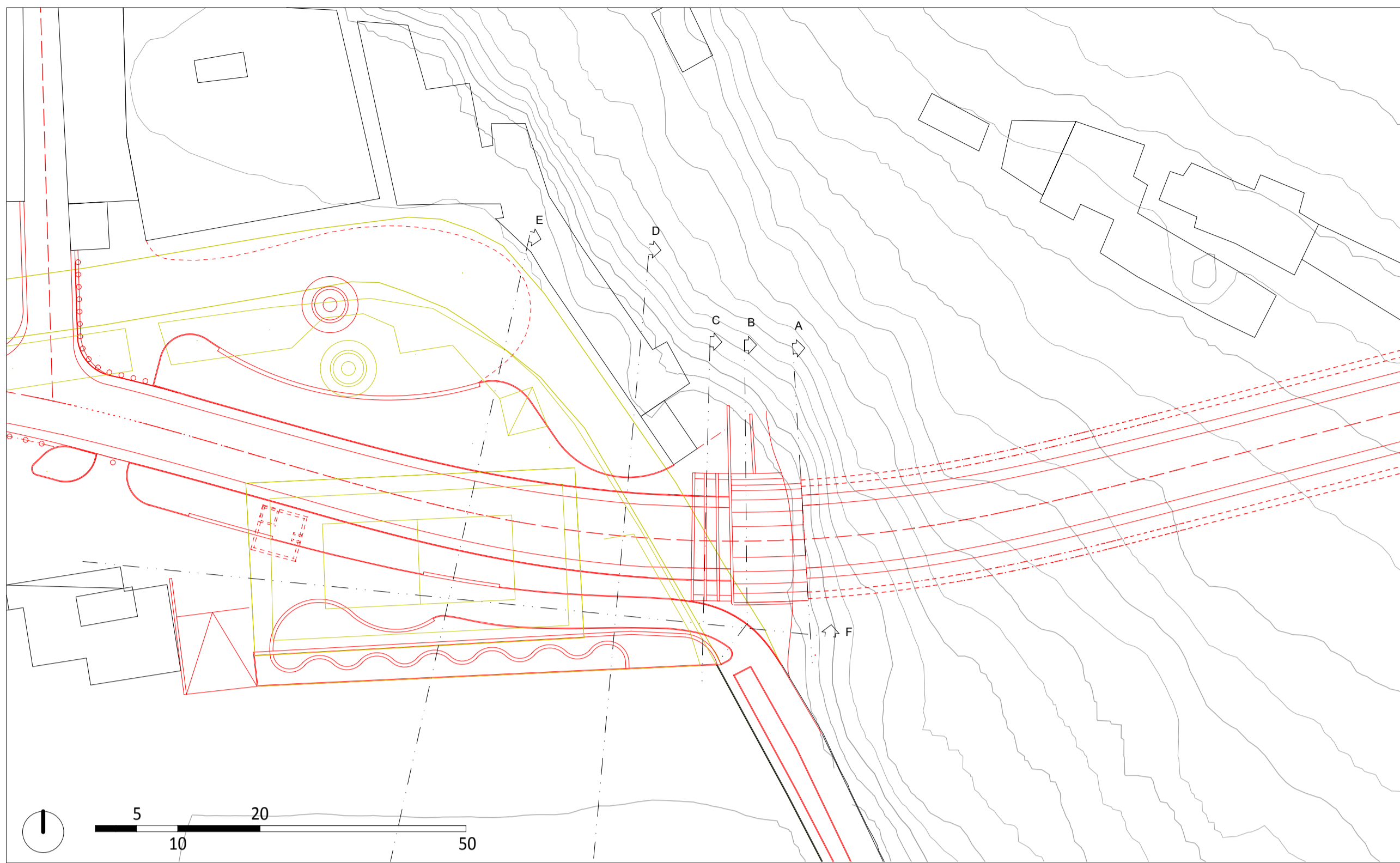
PLANIMETRIA DI CONFRONTO IMBOCCO GALLERIA MINORI - SCALA 1:500
