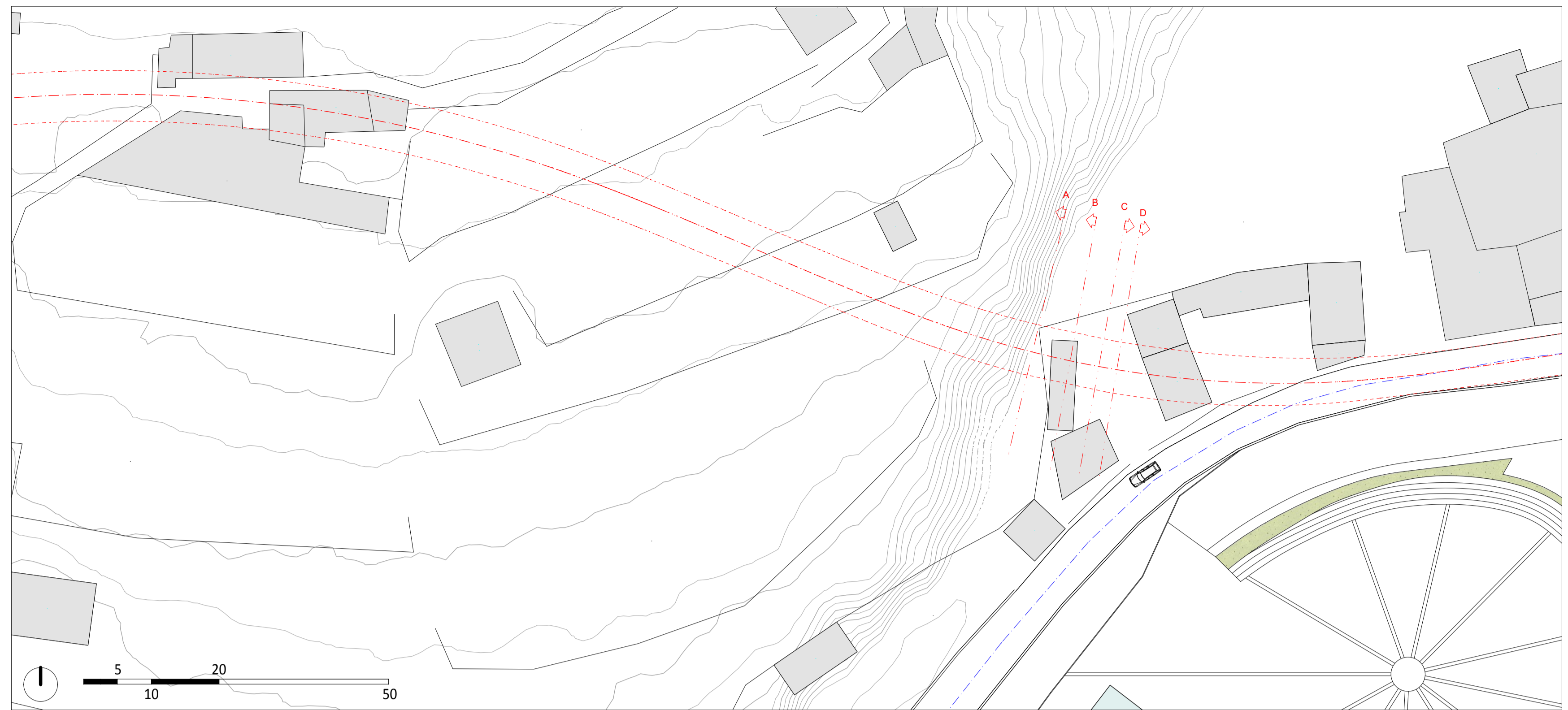
PLANIMETRIA STATO DI FATTO IMBOCCO GALLERIA MAIORI - SCALA 1:500
