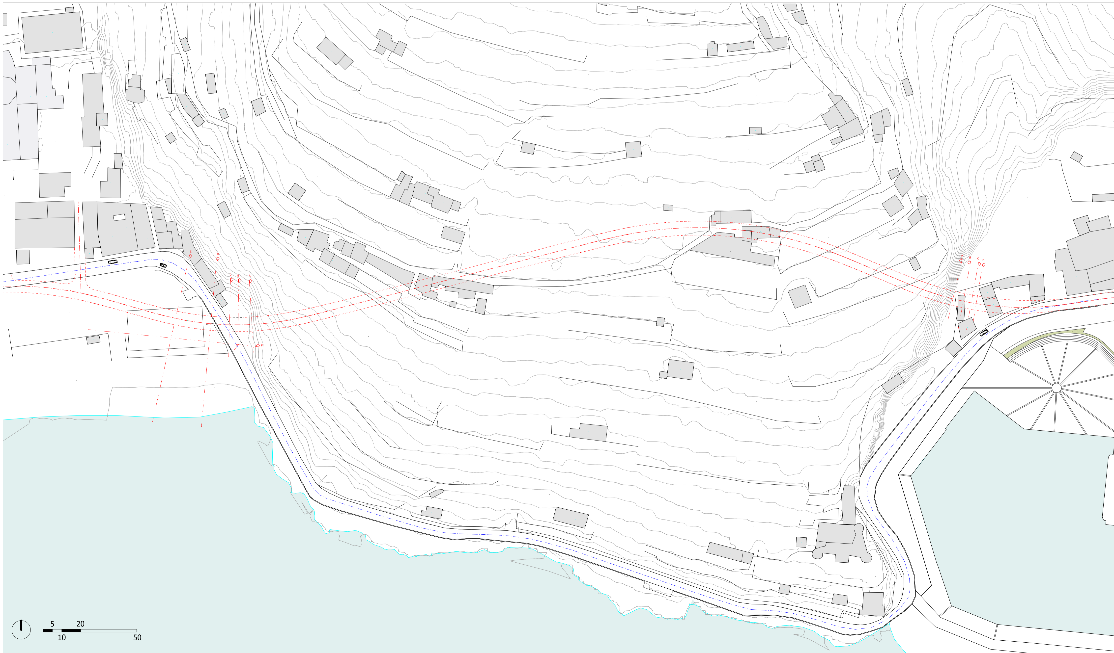
PLANIMETRIA GENERALE STATO DI FATTO - SCALA 1:1000
