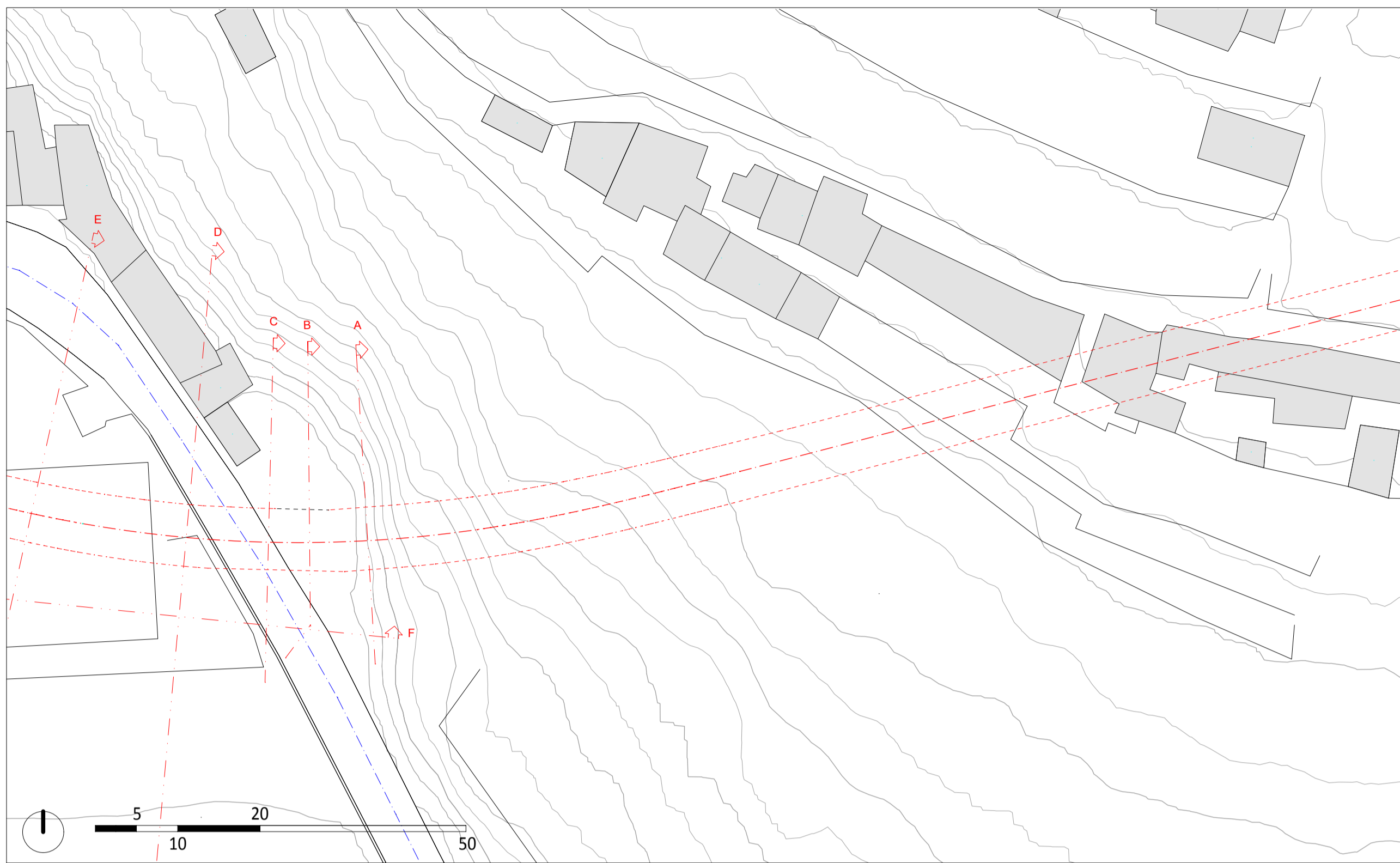
PLANIMETRIA STATO DI FATTO IMBOCCO GALLERIA MINORI - SCALA 1:500
