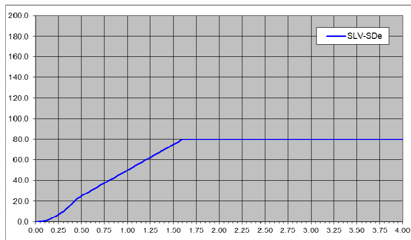
Figura 15.1. Spettro in spostamento SLV
