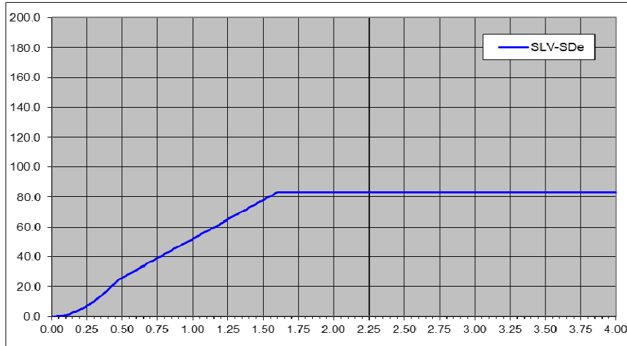
Figura 15.2. Spettro in spostamento SLC
