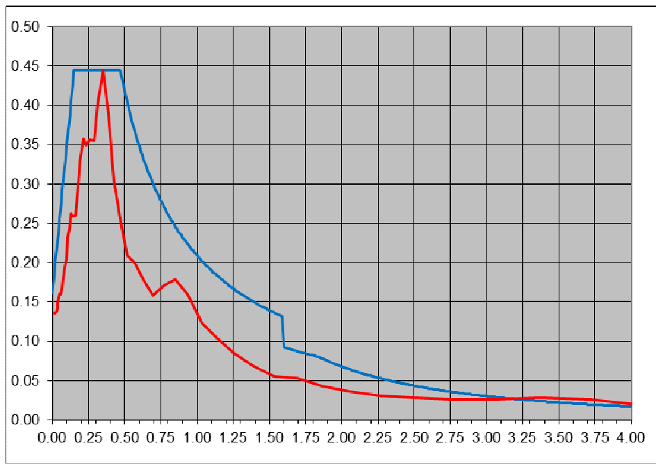
Figura 4.2. Spettro SLC
