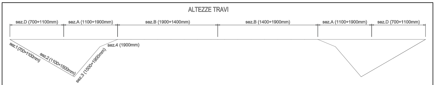
Figura 6.1: Distribuzione e altezze delle sezioni tipo
