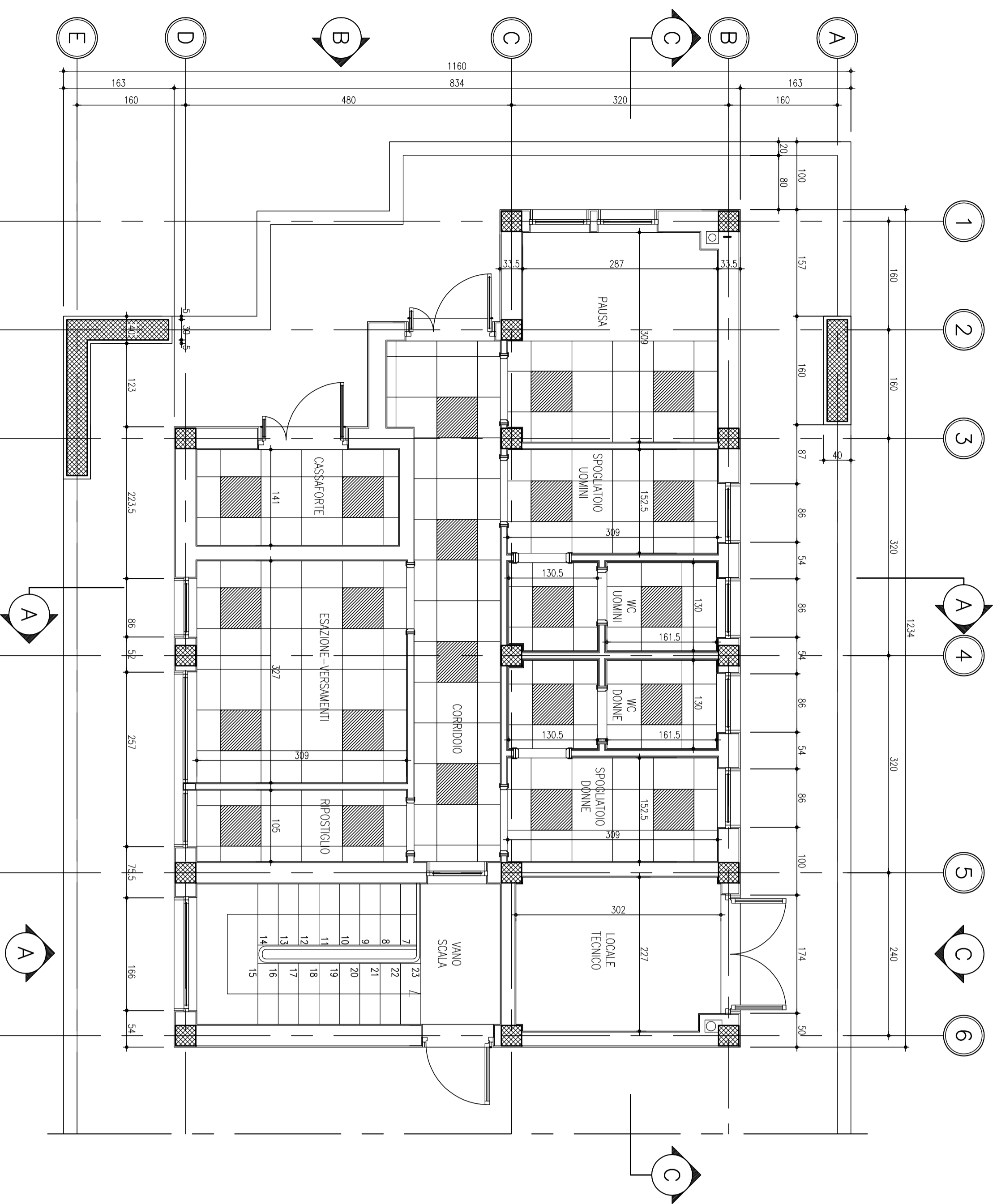
PIANTA DEI CONTROSOFFITTI Rapp. 1:50
