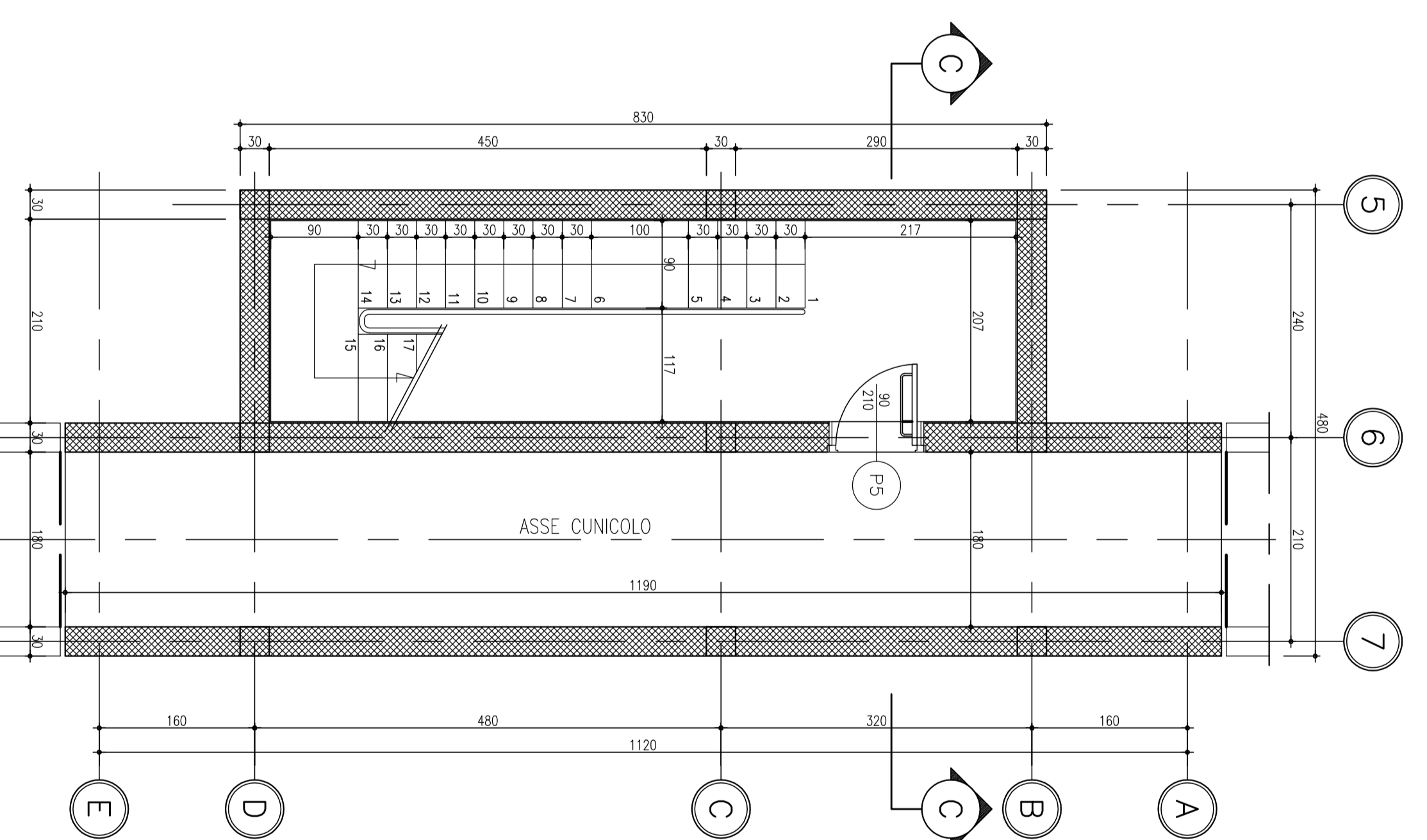
PIANTA PIANO INTERRATO Rapp. 1:50
