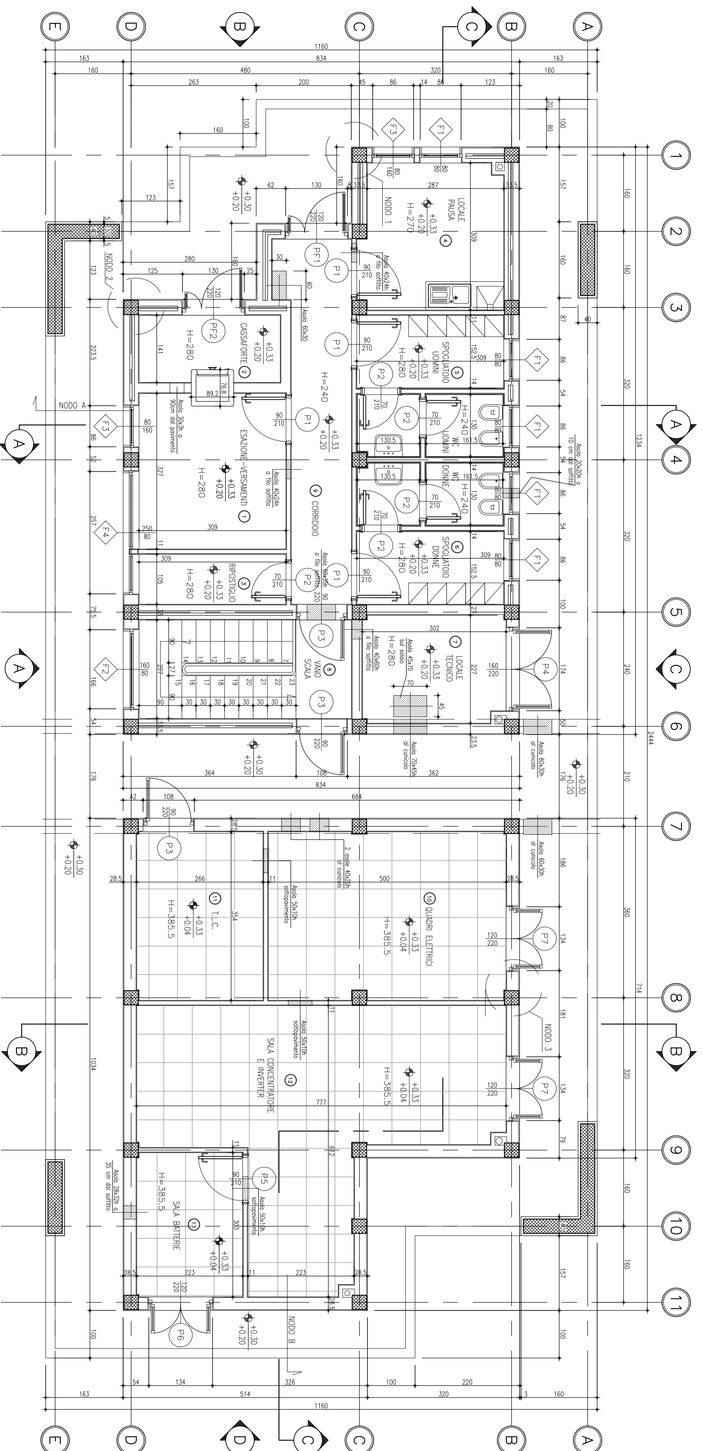
PIANTA PIANO TERRA Rapp. 1:50
