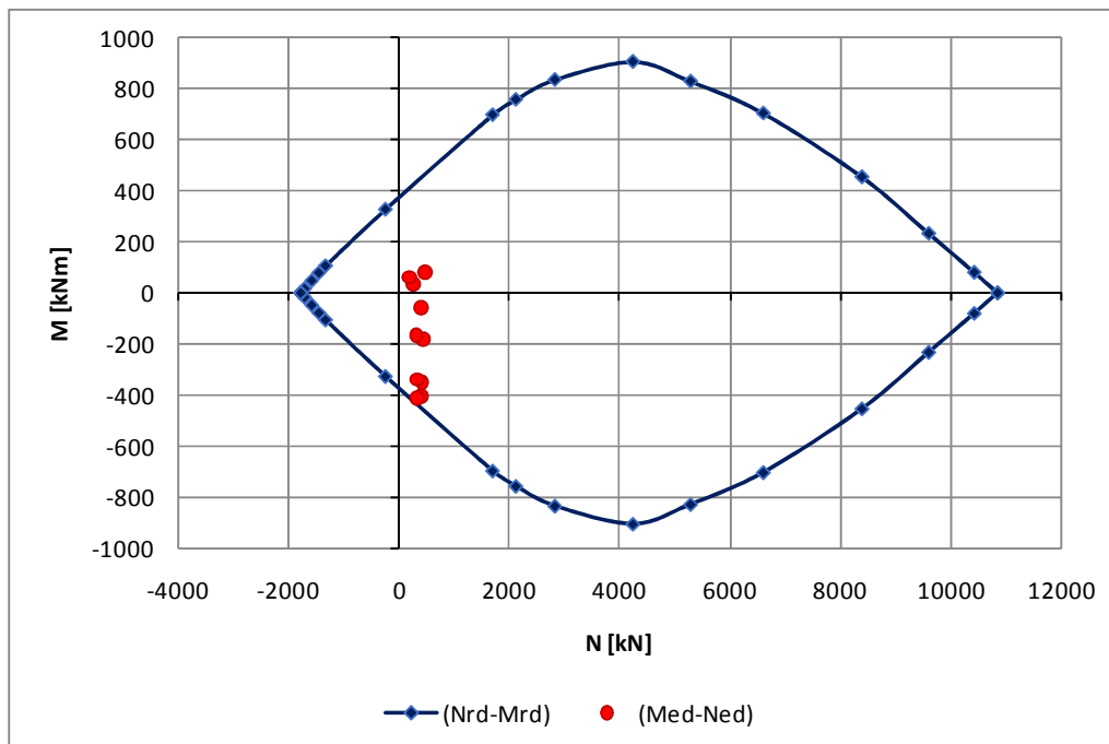
Figura 19 – Dominio ultimo della sezione
