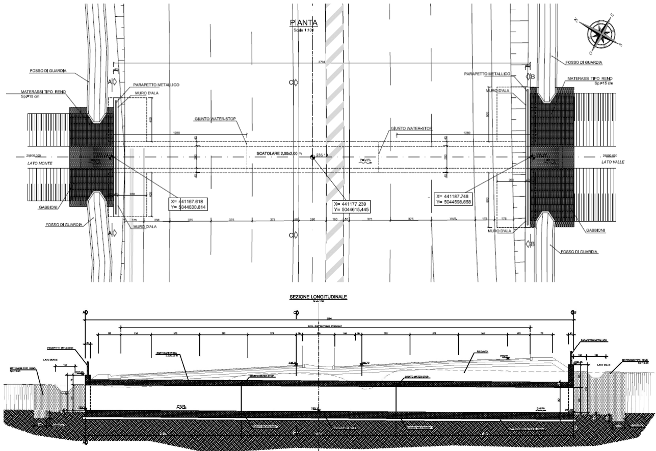
Figura 1 TM03, pianta e sezione longitudinale
