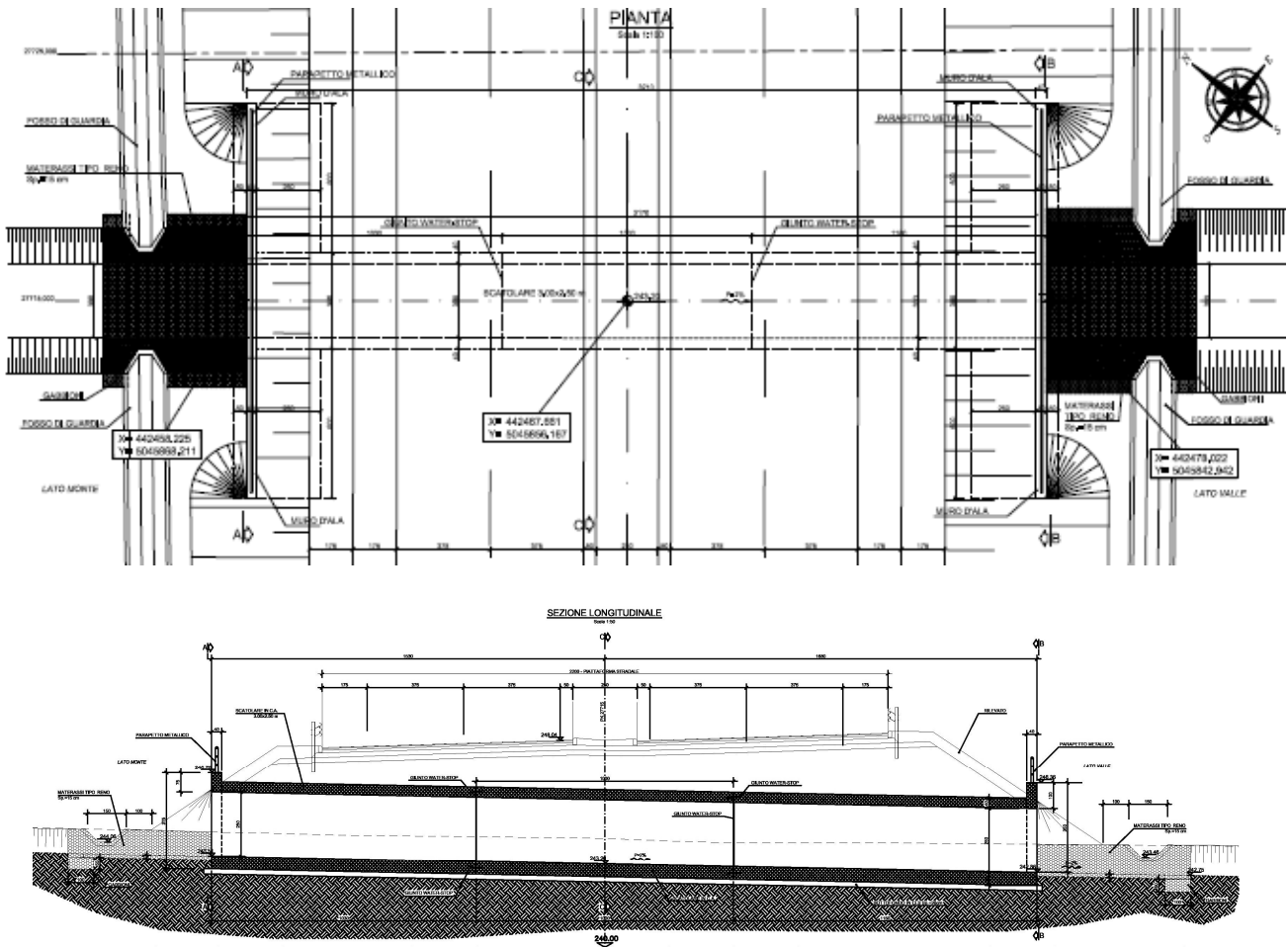
Figura 1 TM08, pianta e sezione longitudinale
