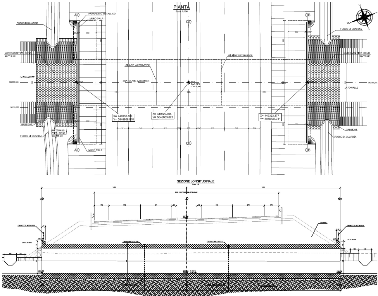
Figura 1 TM31, pianta e sezione longitudinale
