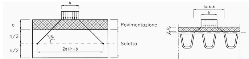
Figura 5.1.3a – Diffusione dei carichi concentrati nelle solette
