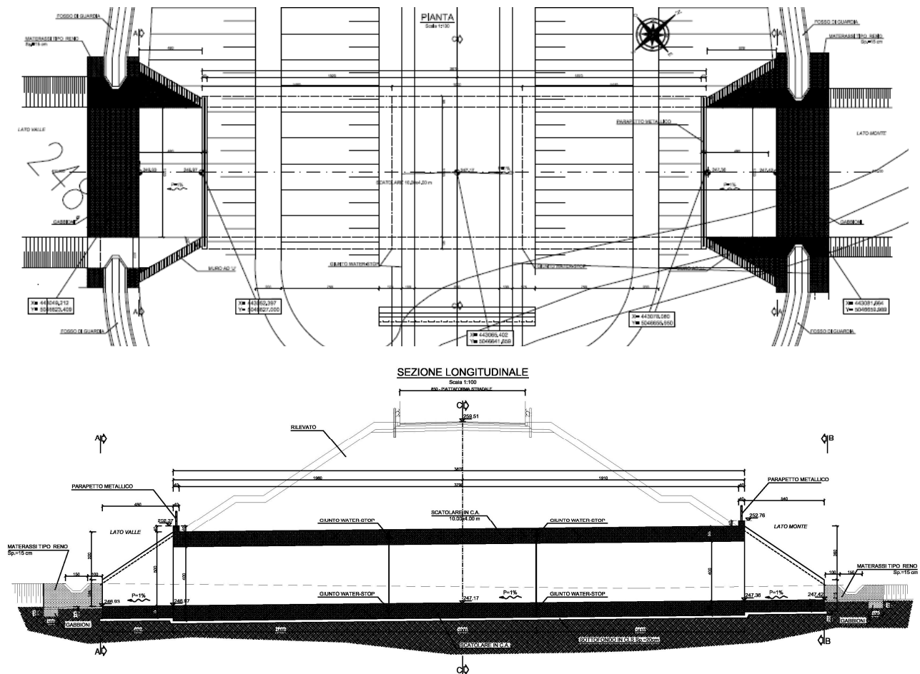
Figura 1 TM47, pianta e sezione longitudinale
