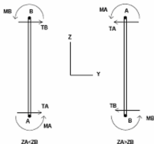
Figura 11-1: convenzioni di segno per l'elemento BEAM
