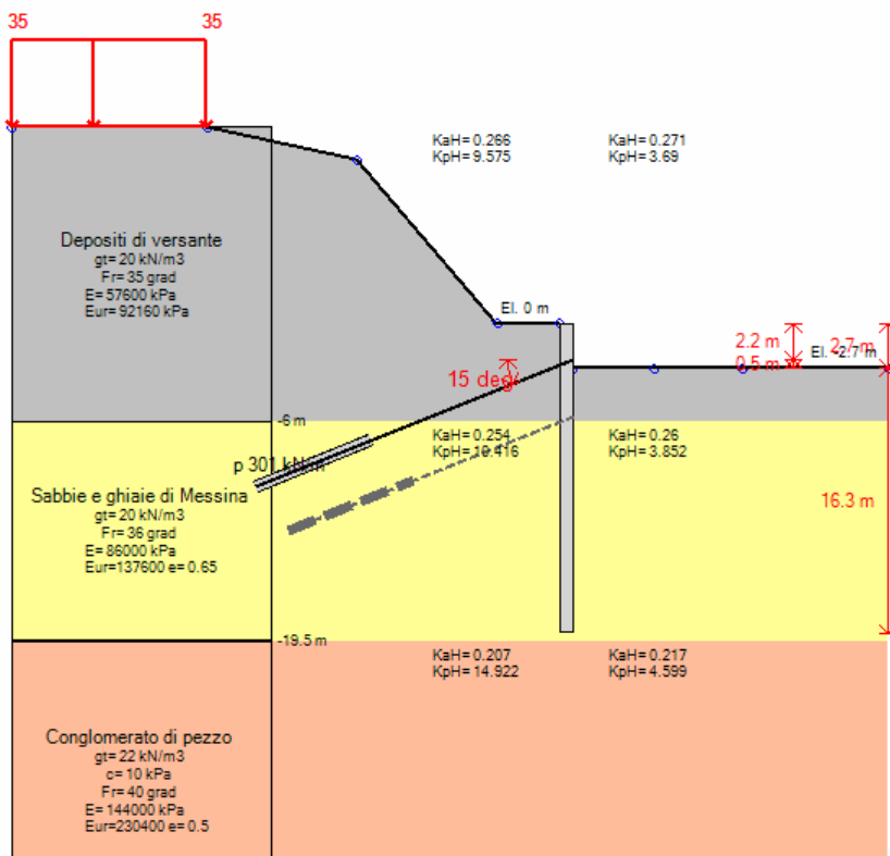
Stage 2 – Inserimento tirante a quota -2.70 m
