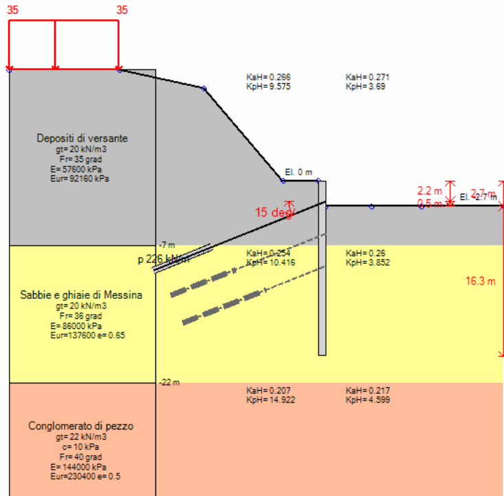
Stage 2 – Inserimento tirante a quota -2.20 m
