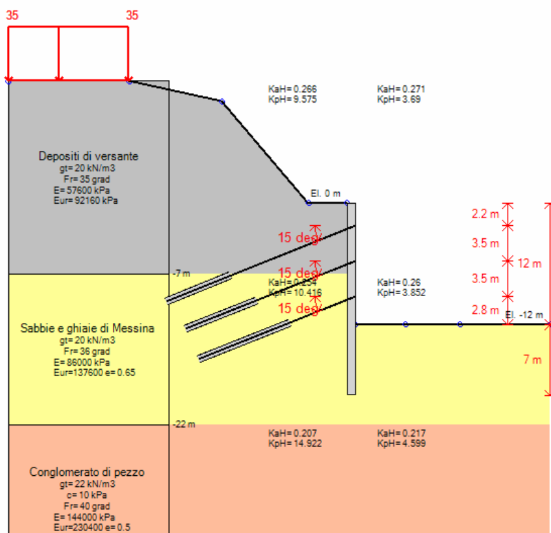
Stage 6 – Inserimento tirante a quota -9.20 m
