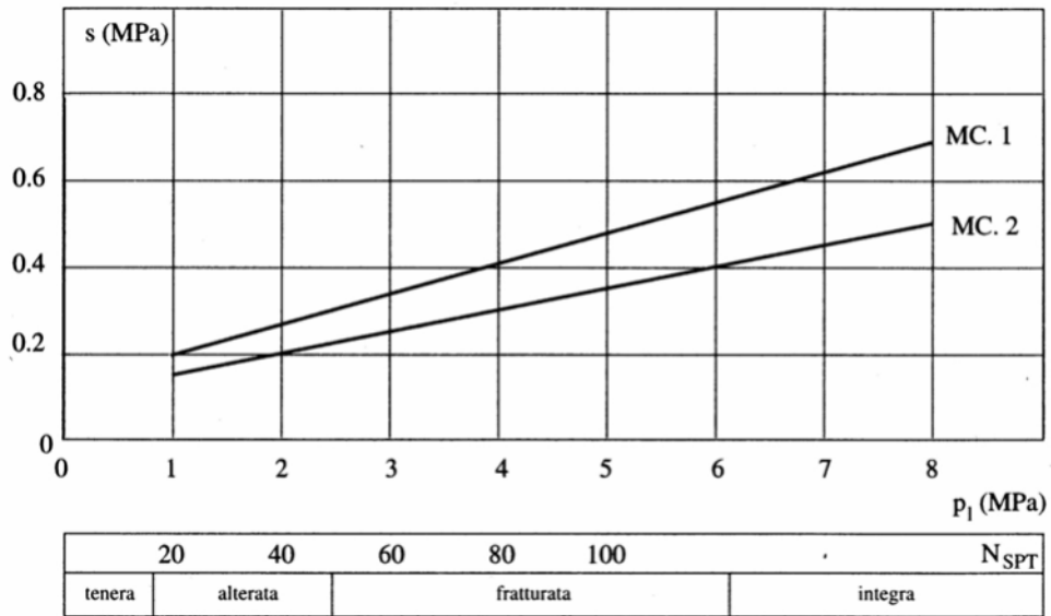
Figura 8.7: Gessi, marne, marne calcaree
