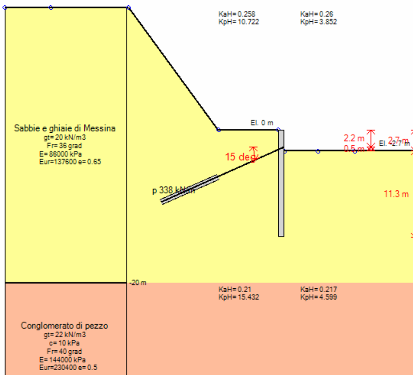
Stage 2 – Inserimento tirante a quota -2.20 m
