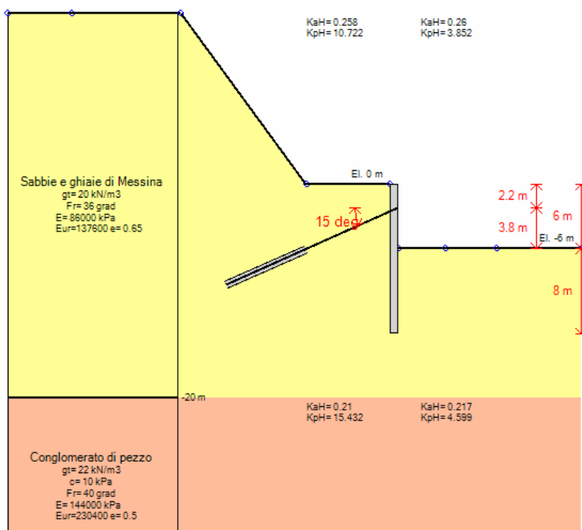
Stage 3 – Scavo a quota -6.00 m
