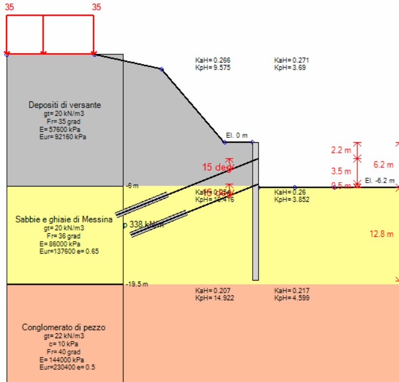
Stage 4 – Inserimento tirante a quota -5.70 m
