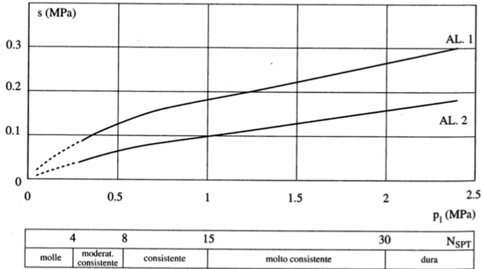
Figura 8.6: Argille e limi
