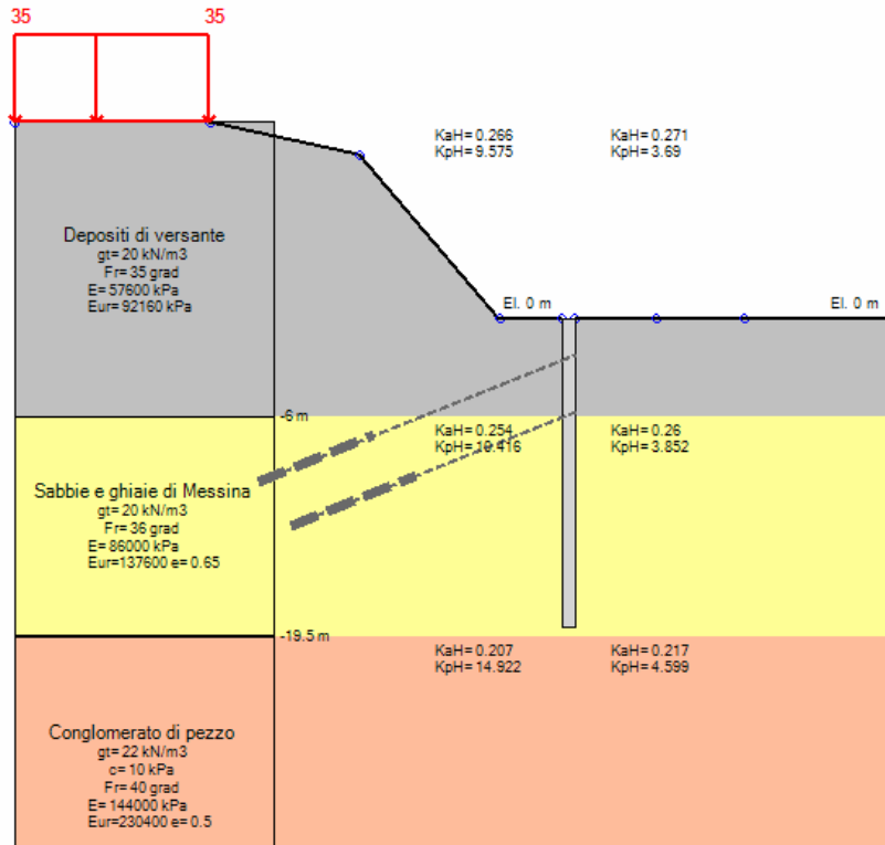
Stage 0 – Infissione
