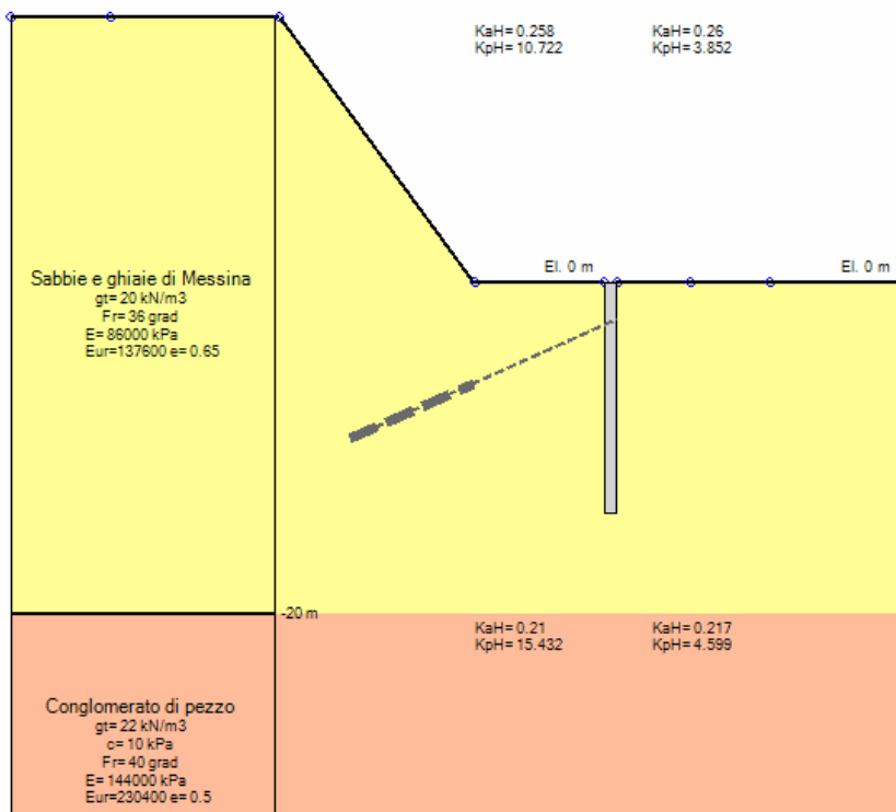
Stage 0 – Infissione
