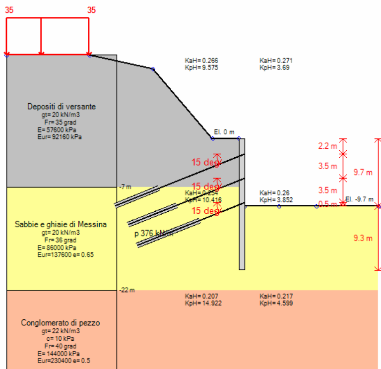
Stage 6 – Inserimento tirante a quota -9.20 m
