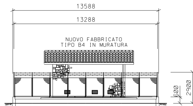
PROSPETTO B
