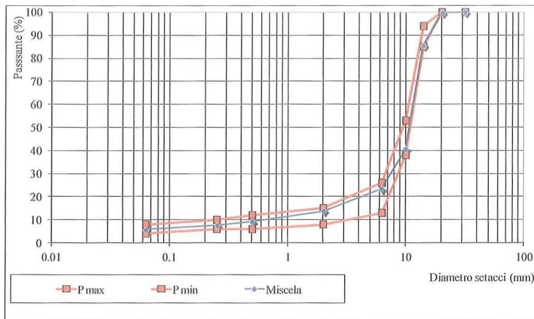
Graf. 5.1 – Curva granulometrica e fuso di riferimento del tappeto drenante steso nella zona del campo prove
