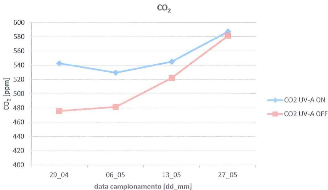
Graf. 2.20 - Sovrapposizione valori di CO 2 tra condizioni di lampade UV-A accese e spente
