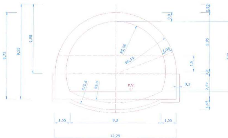
Fig. 2.1 – Pianta e sezione della galleria, carreggiata nord
