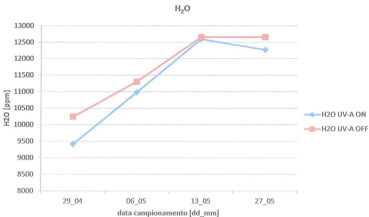
Graf. 2.21 - Sovrapposizione valori di H 2 O tra condizioni di lampade UV-A accese e spente
