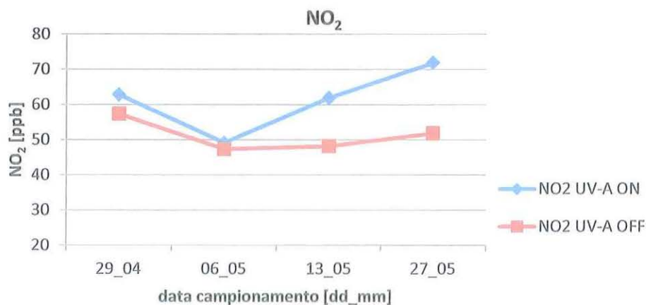
Graf. 2.5 – Sovrapposizione NO 2 in condizioni di lampade UV-A accese e spente
