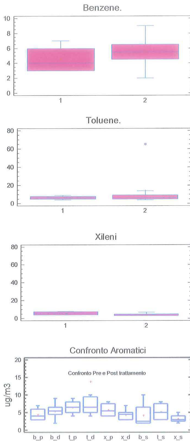
Graf. 2.4 – Analisi di acetati, cloruri, nitriti, nitrati, ossalati, solfati, benzene, toluene, xileni e aromatici
