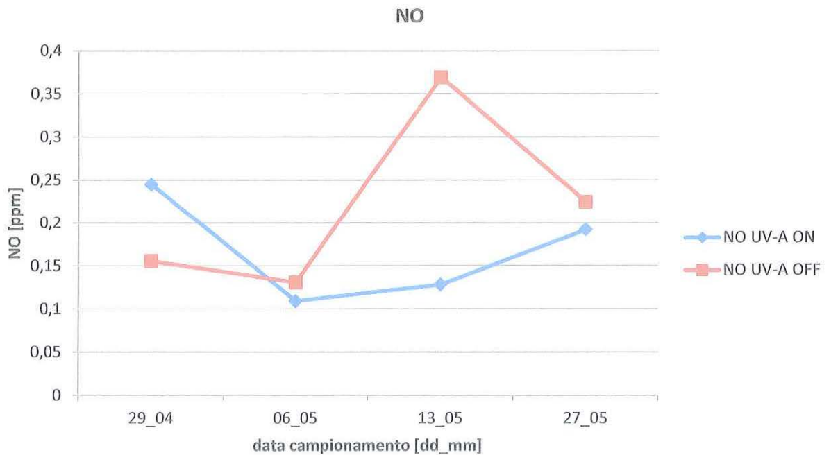
Graf. 2.18 - Sovrapposizione valori di NO tra condizioni di lampade UV-A accese e spente
