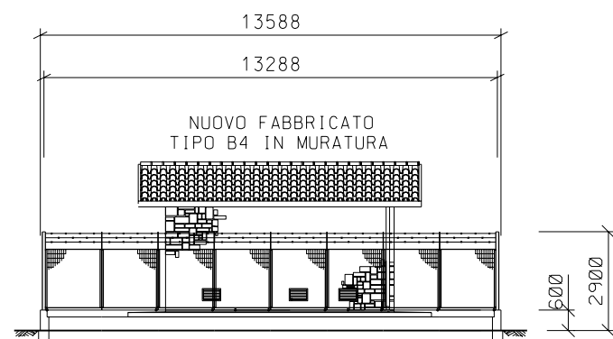
PROSPETTO B
