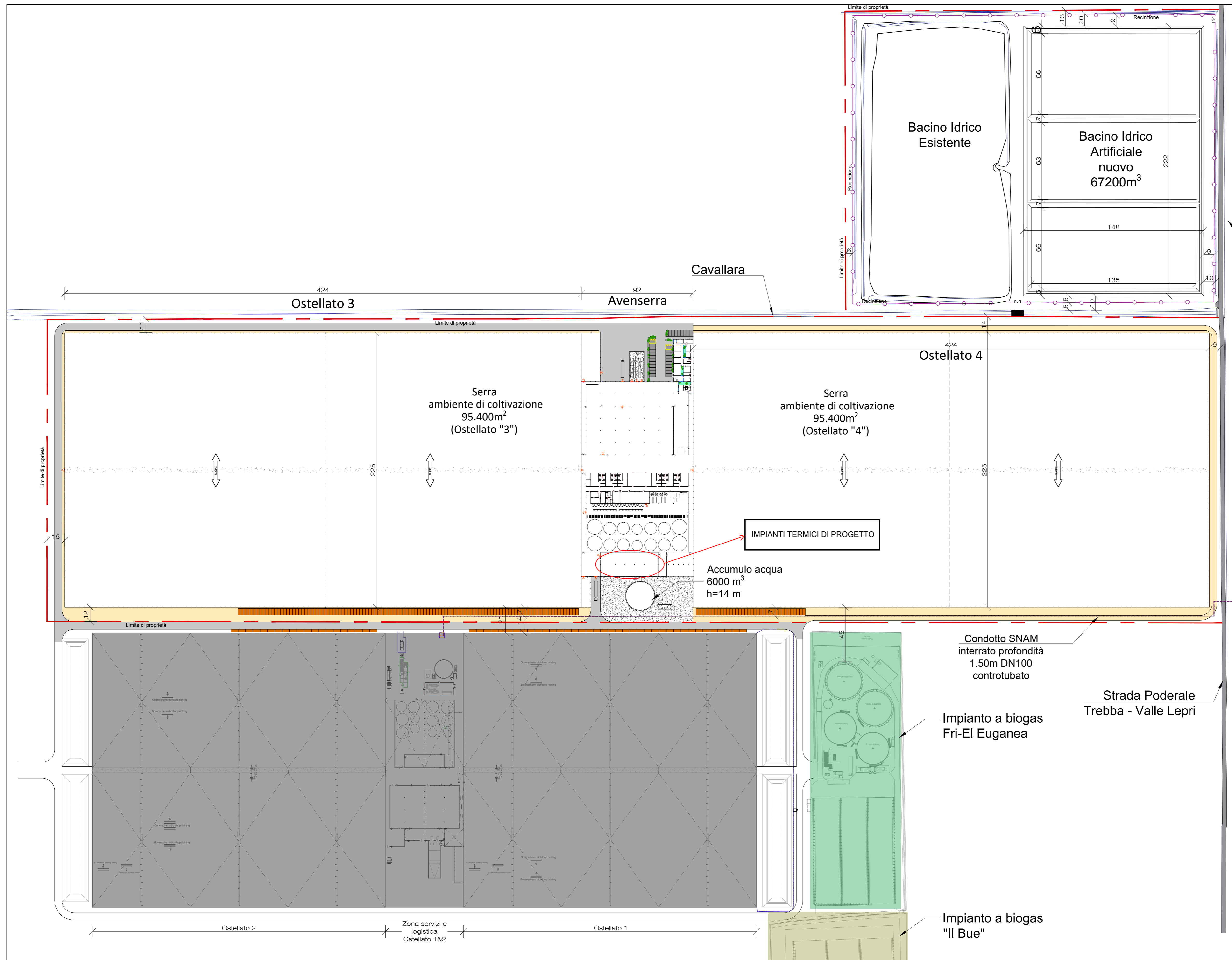
PLANIMETRIA GENERALE STATO DI PROGETTO Scala 1:1500
