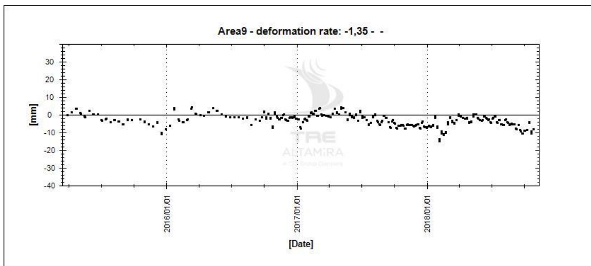
Figura 27: Serie storica media (componente orizzontale) dei punti di misura evidenziati in Figura 25 e Figura 26.
