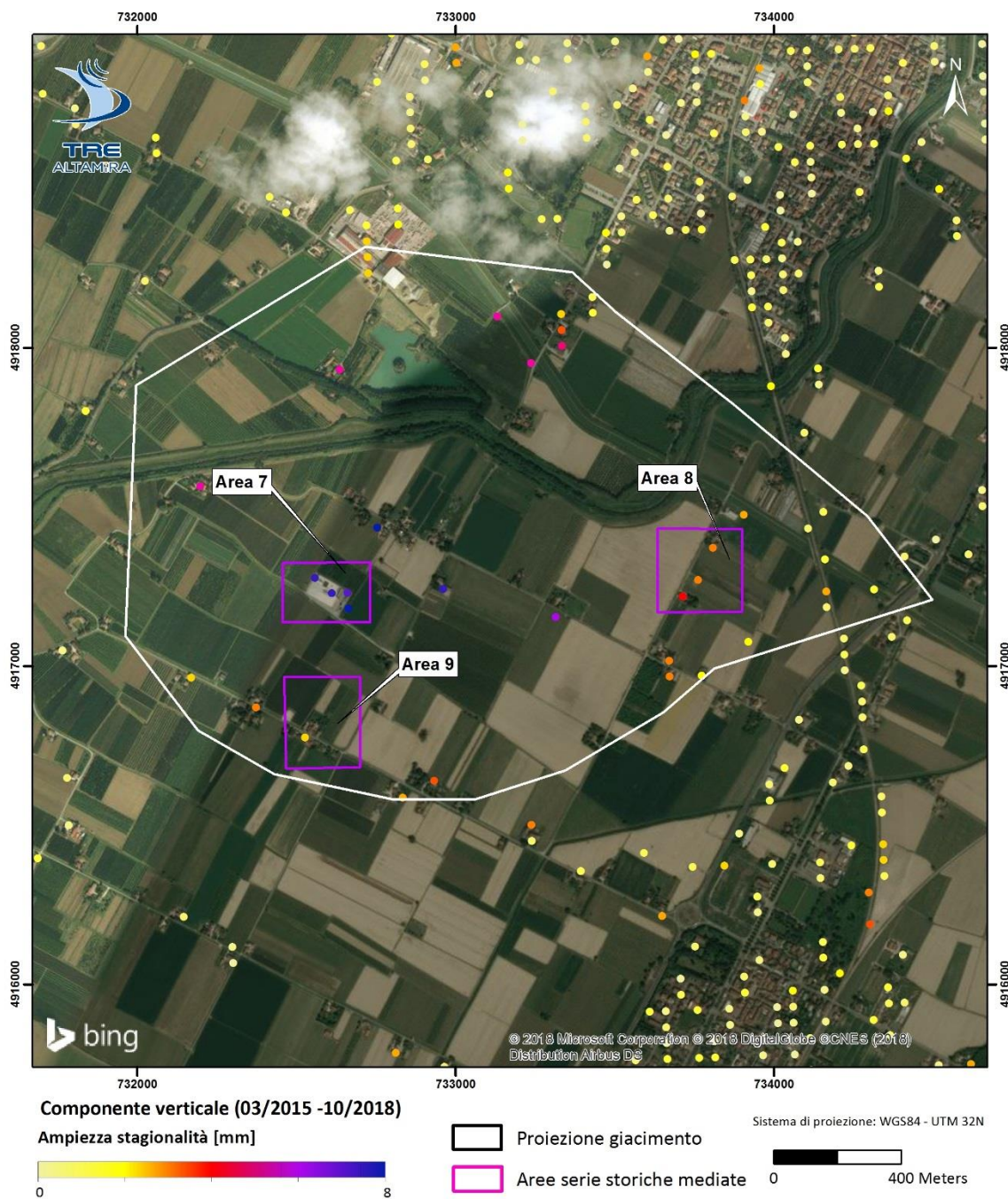
Figura 23: Dettaglio della ampiezza media della stagionalità per la componente verticale sull'area del Pool C. Le serie storiche dei punti all'interno delle aree viola sono stati mediati per ottenere le serie storiche medie mostrate in Figura 24
