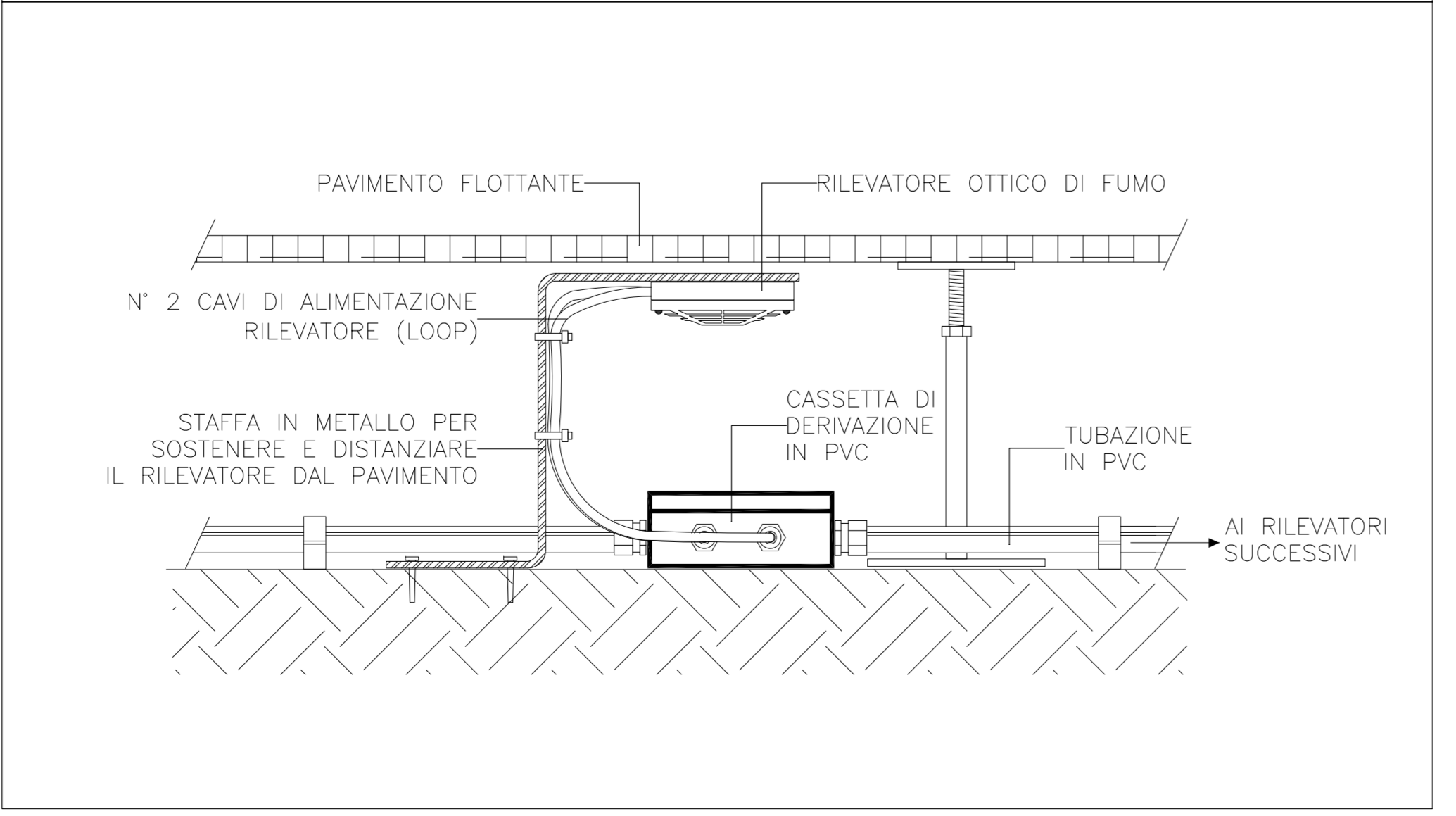
RILEVATORE DI FUMO SOTTO PAVIMENTO
