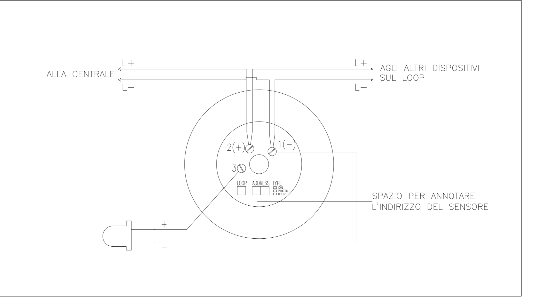
RILEVATORE DI FUMO A SOFFITTO SCHEMA DI COLLEGAMENTO
