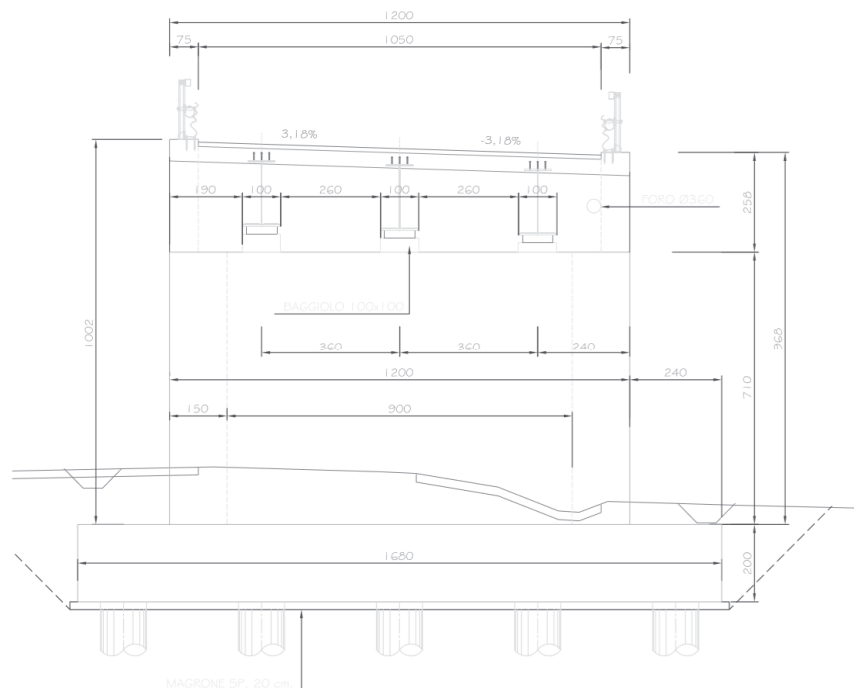
Figura 6: Prospetto trasversale Spalla SP1
