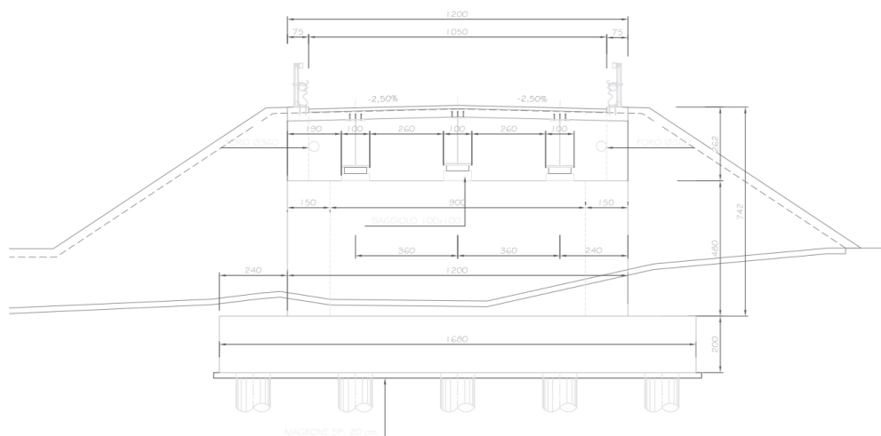
Figura 7: Prospetto trasversale Spalla SP2
