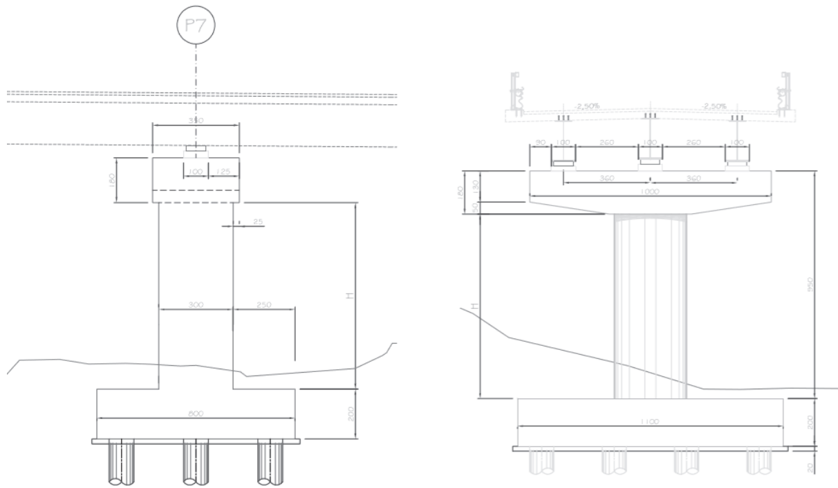
Figura 8: Carpenteria pile
