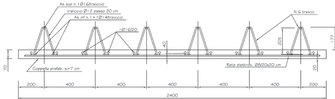
Figura 23: Coppella prefabbricata
