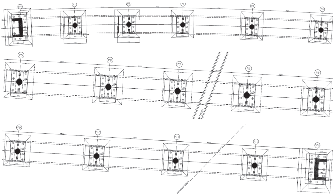
Figura 4: Pianta delle fondazioni
