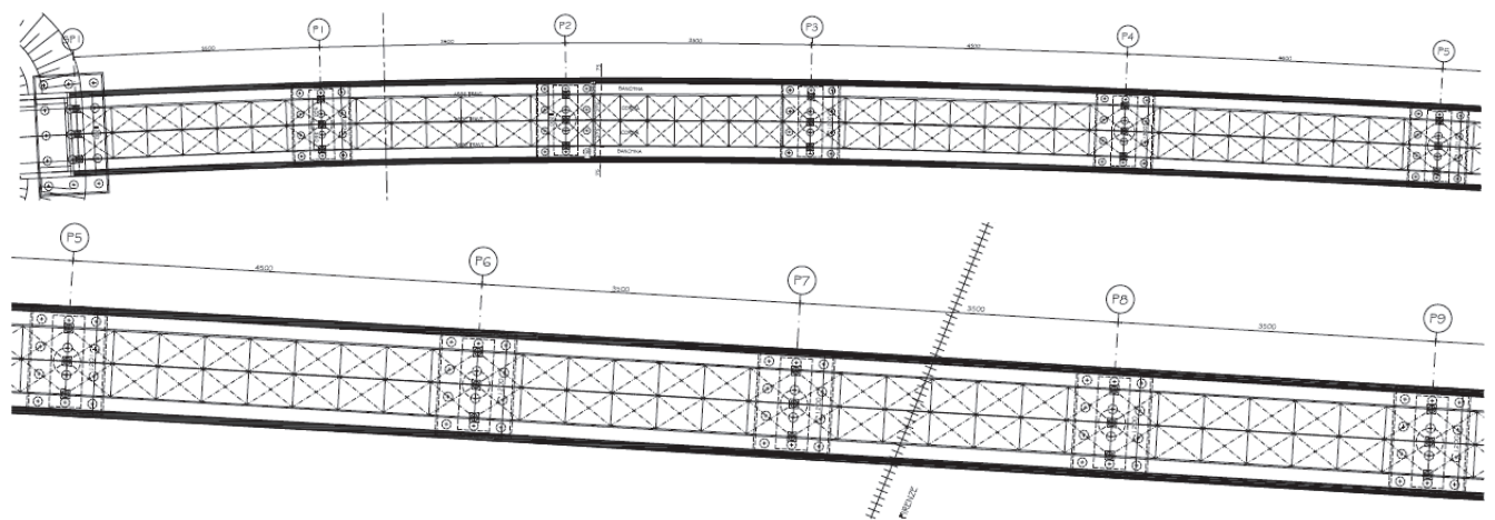
Figura 2: Pianta impalcato (Parte 1)
