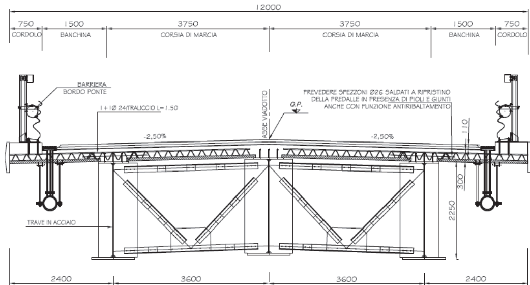
Figura 5: Sezione trasversale dell'impalcato – Sezione corrente trave H=2.25m
