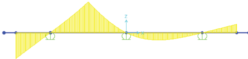
Figura 27: Linea di influenza del momento flettente – Sezione in campata
