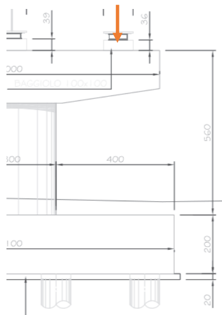
Figura 40: Schematizzazione della mensola
