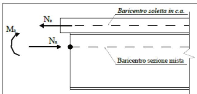
Figura 9: Azioni equivalenti al ritiro
