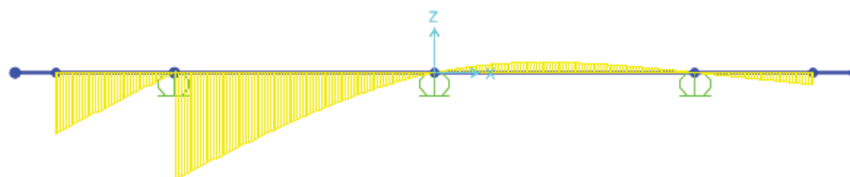
Figura 36: Linea di influenza del taglio – Sezione all'appoggio esterno
