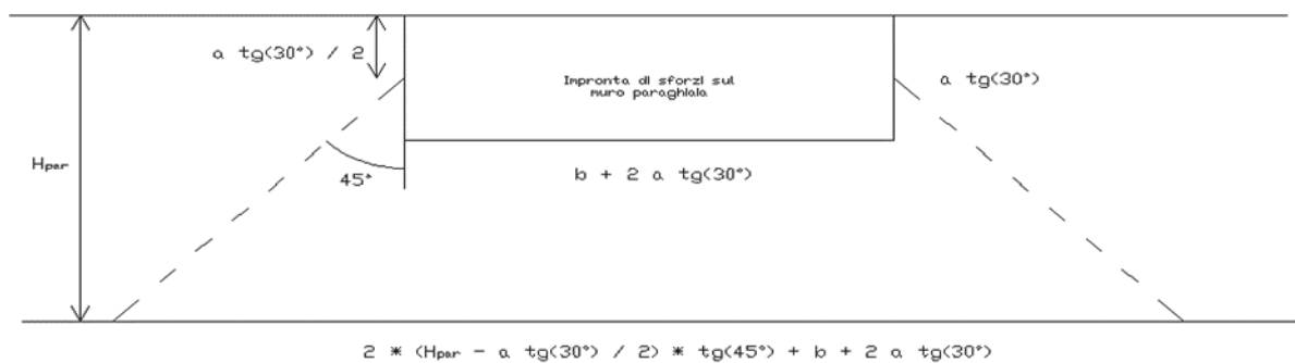
Prospetto del muro paraghiaia
