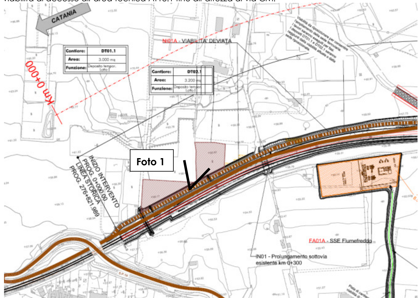
Stralcio Planimetrico ubicazione cantiere DT01.1 e DT02.1
