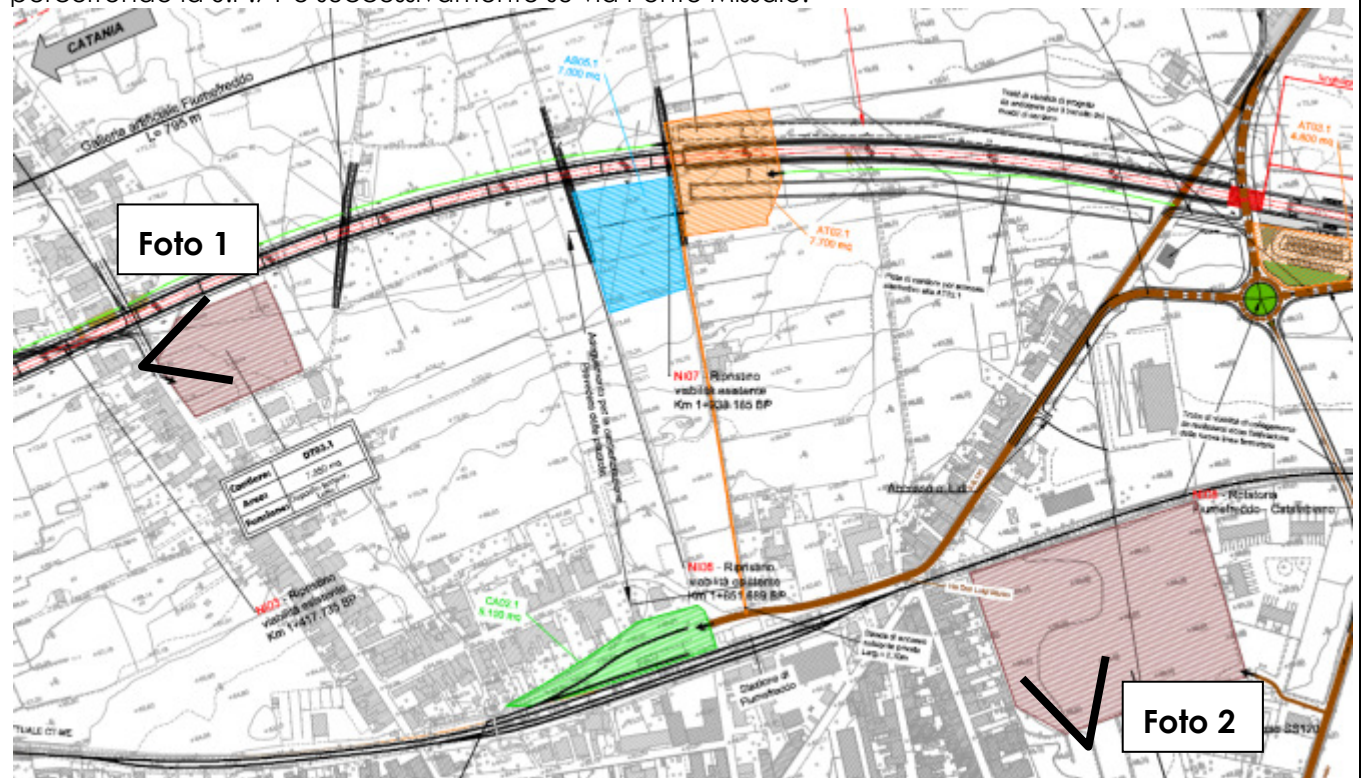
Stralcio Planimetrico ubicazione cantiere DT03.1 - DT04.1
