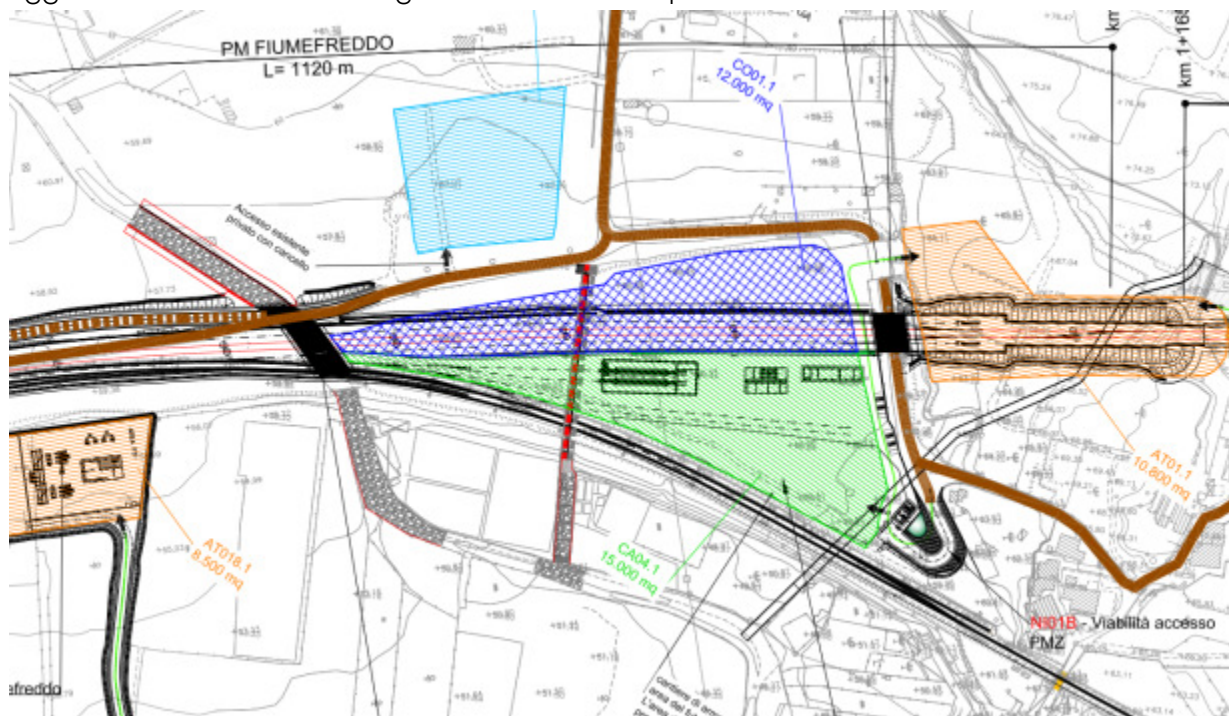
Stralcio Planimetrico ubicazione cantiere CO01.1
