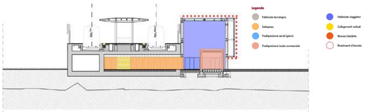
Figura 13 - Schema funzionale fermata di Nizza-Alì_ sezione
