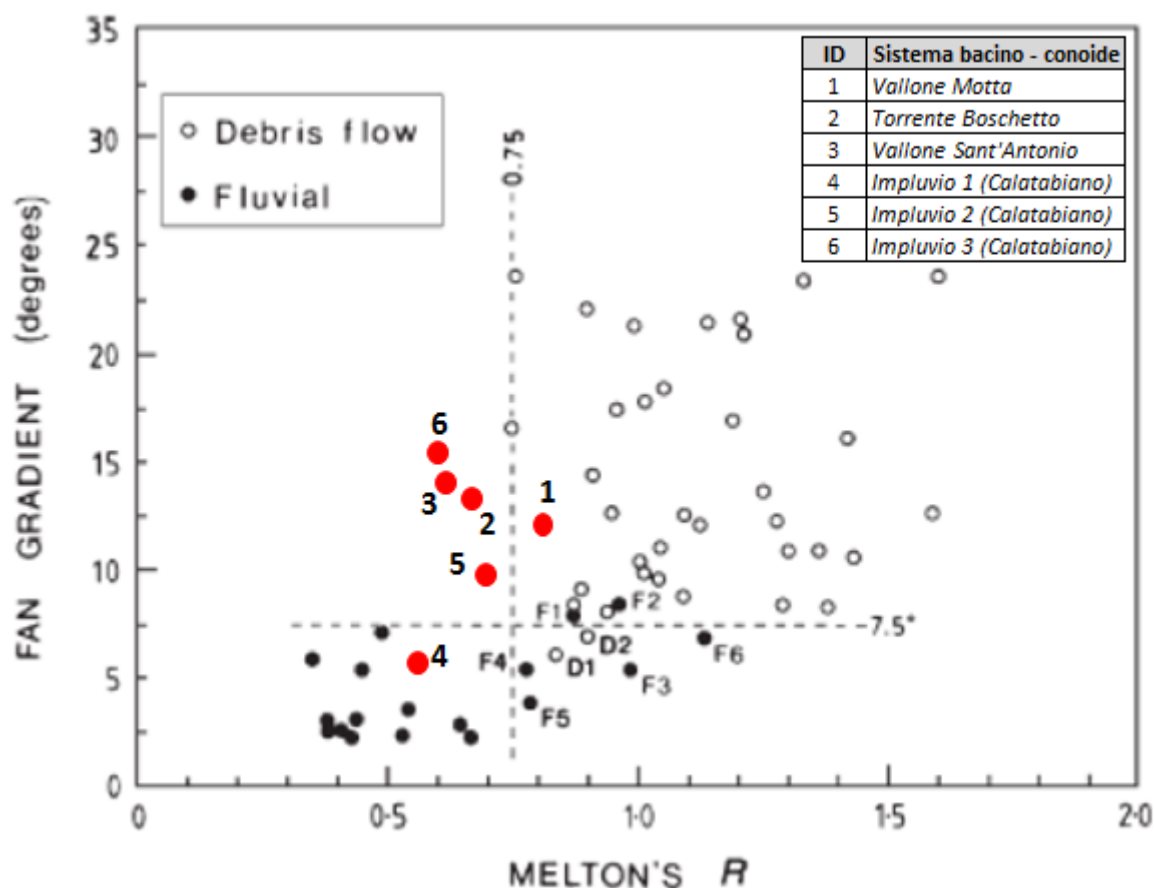
Figura 4-8: Pendenza conoide vs indice di Melton (DeSclally & Owens, 2004).
