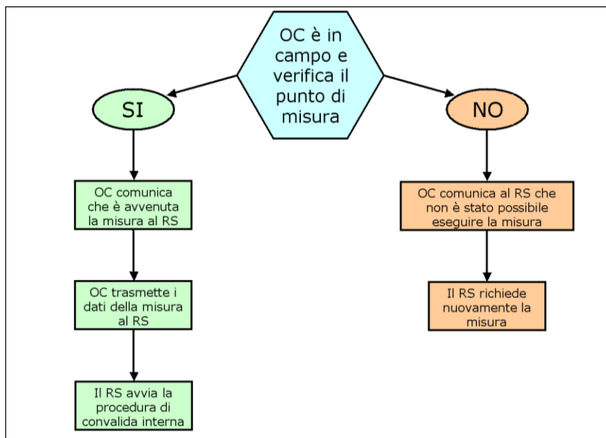
FIGURA 2-1 PROCEDURA RELATIVA ALLO SVOLGIMENTO DEI RILIEVI E ALLA TRASMISSIONE DEI DATI
