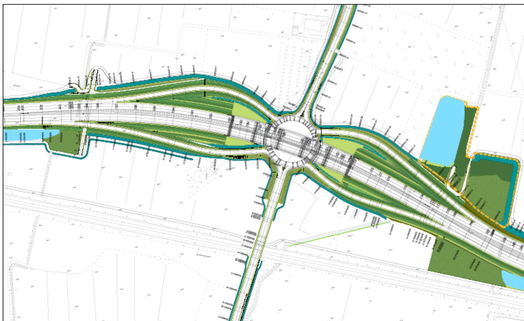
FIGURA 1-4 – SVINCOLO DI PIEVE MODOLENA
