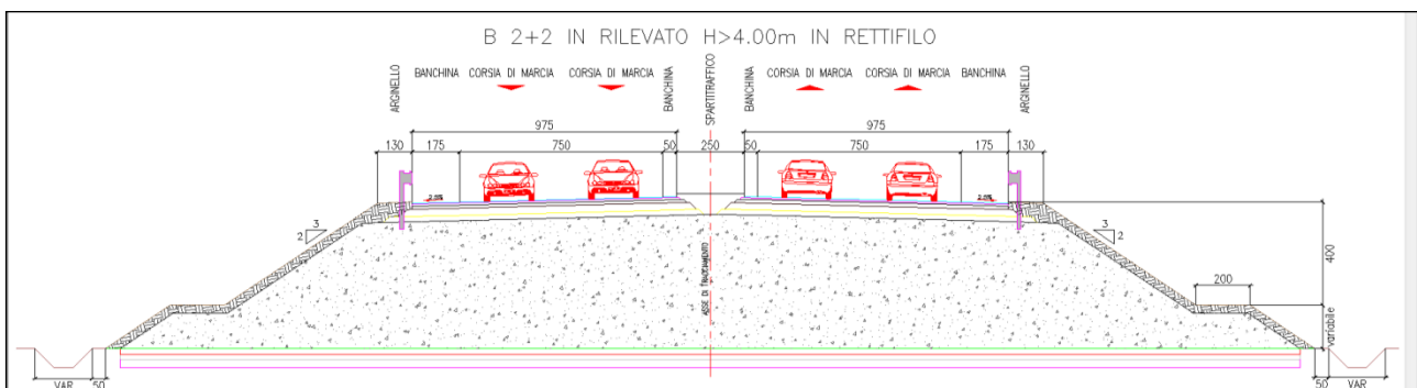
FIGURA 1-7 - SEZIONE TIPO CATEGORIA B
