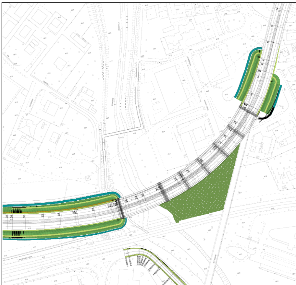
FIGURA 1-2 - ATTRAVERSAMENTO DEL TORRENTE CROSTOLO
