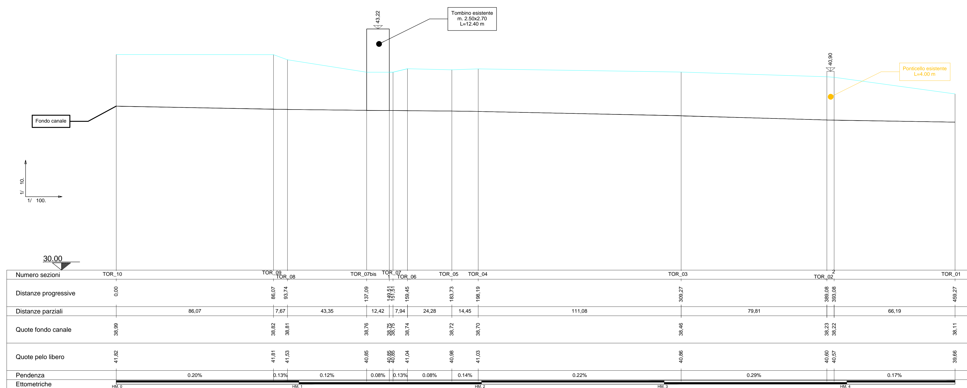
FOSSETTA DELLA TORRETTA - profilo asse (esistente)
