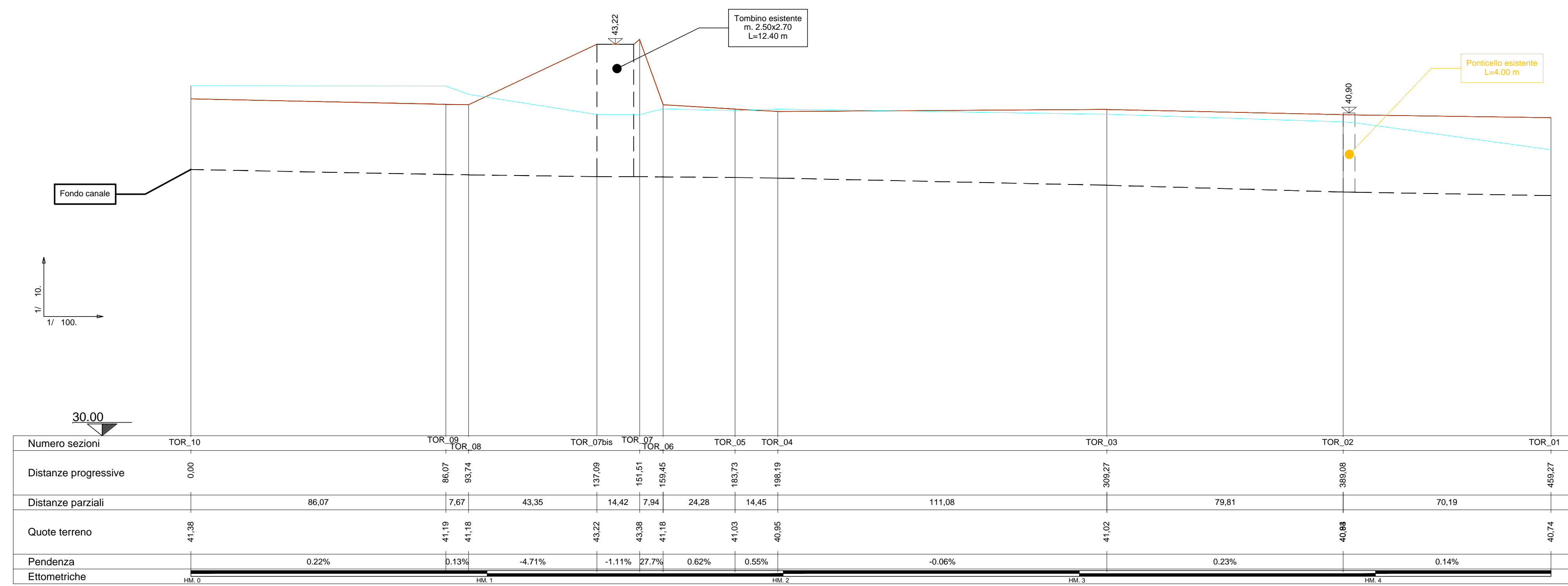
FOSSETTA DELLA TORRETTA - profilo sponda destra (esistente)
