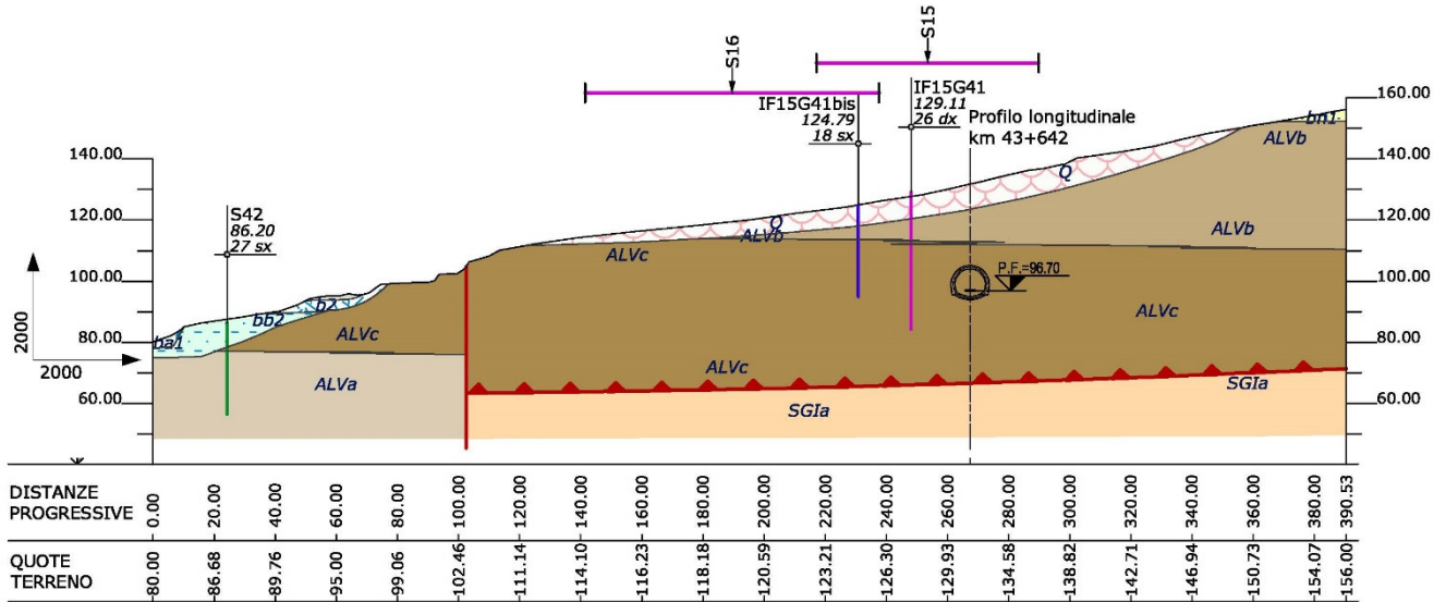
Figura 51 - Sezione geologica trasversale al tracciato di progetto al km 43+600 circa, ricostruita lungo il versante in frana, con indicazione schematica dell'opera in sotterraneo.
