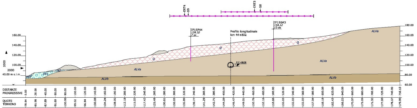
Figura 54 - Sezione geologica trasversale 6 al tracciato di progetto al km 44+800 circa, ricostruita lungo il versante in frana, con indicazione schematica dell'opera in sotterraneo.
