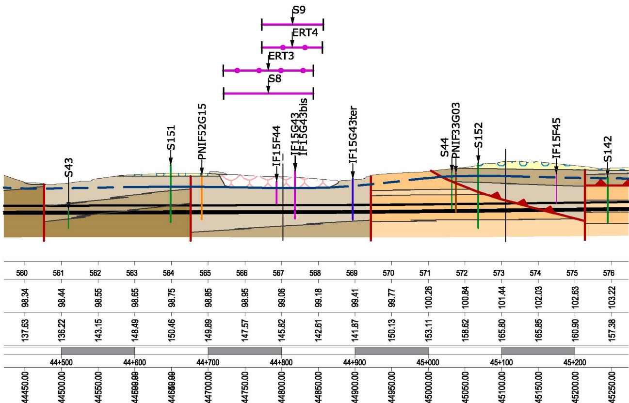
Figura 55 – Sezione geologica del versante su cui insiste la frana complessa con stato quiescente al km 44+800 circa.
