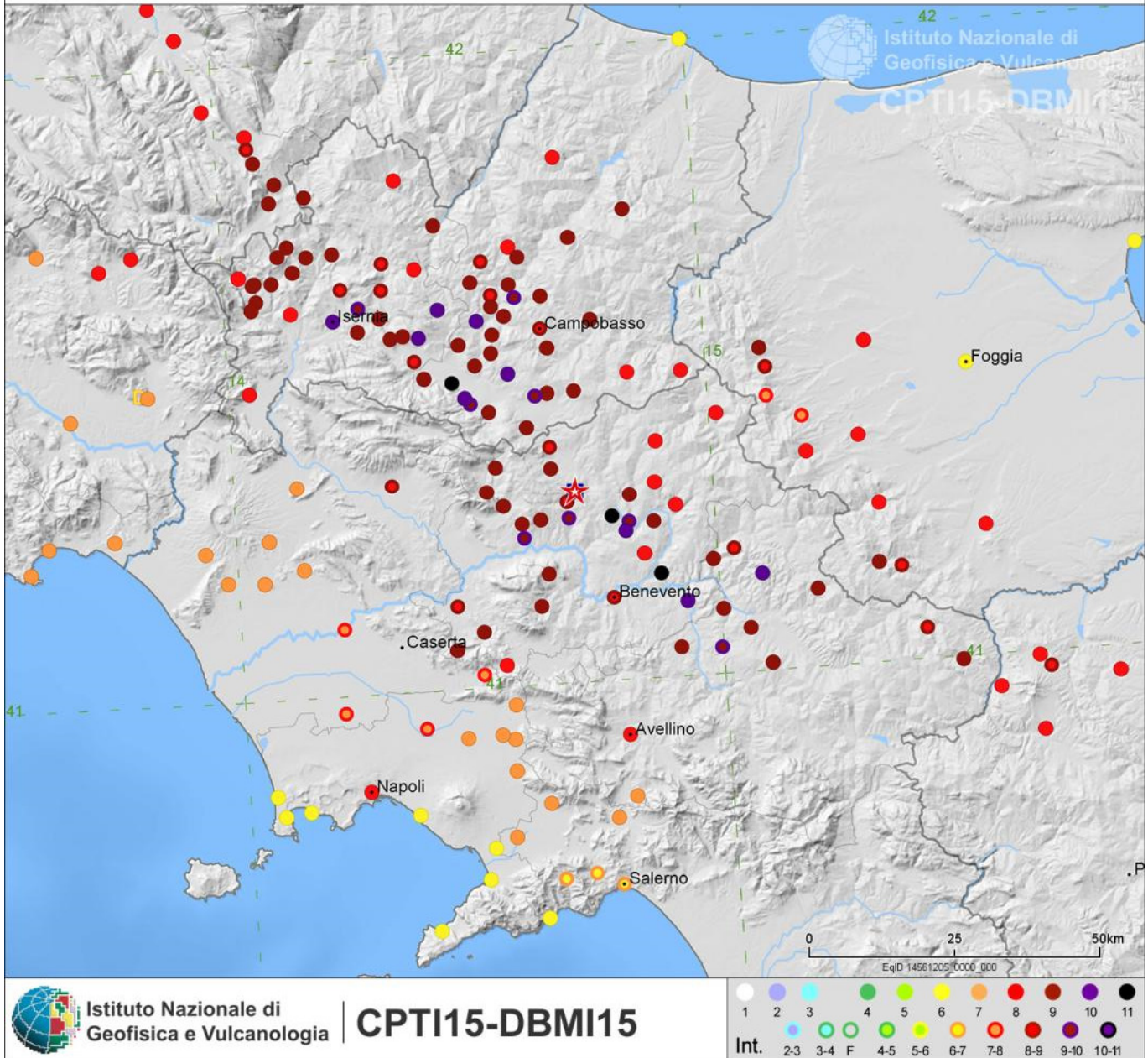
Figura 19 - Distribuzione del danneggiamento prodotto dal terremoto del 1456 nell'area di studio ( http://emidius.mi.ingv.it/ CPTI15-DBMI15).
