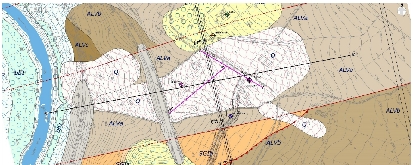
Figura 53 – Stralcio della carta geologica con elementi di geomorfologia km 44+800.
