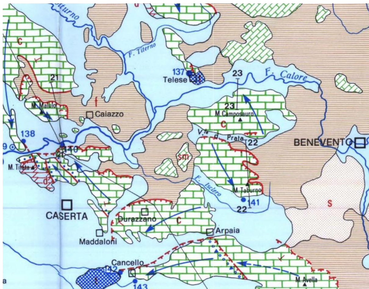
Figura 14 – Stralcio dello schema idrogeologico dell'Appennino carbonatico centro-meridionale (da Celico 1978).
