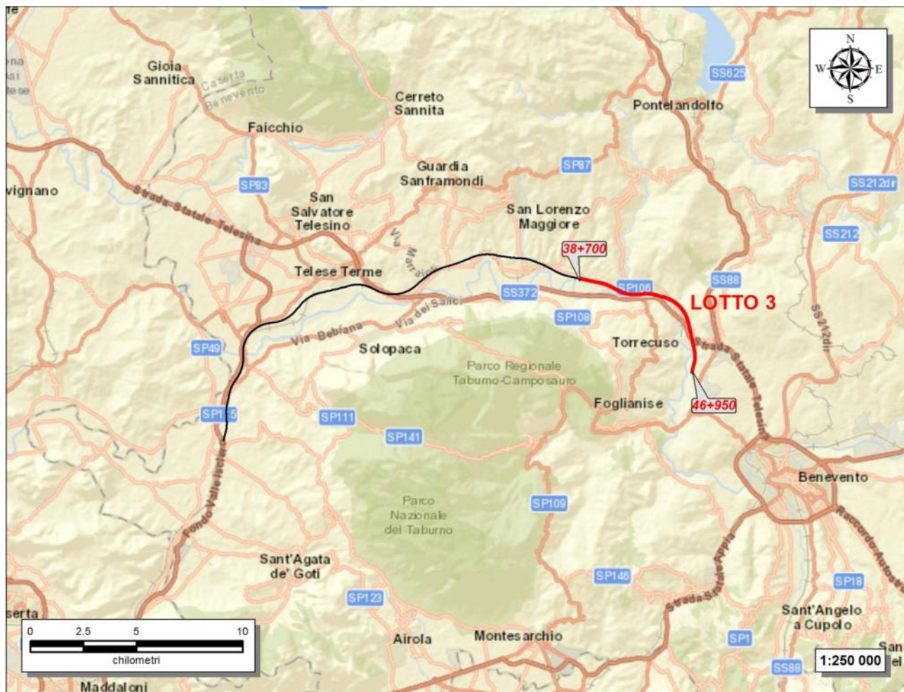
Figura 1 – Corografia in scala 1:250000 dell’area in cui si colloca lo studio geologico con individuazione, in colore rosso, del tracciato di stretto interesse progettuale relativo al Lotto 3.
