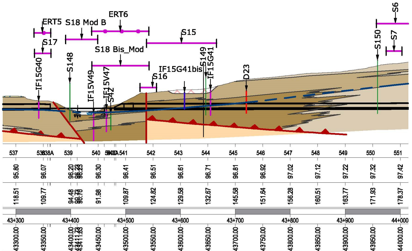
Figura 52 - Sezione geologica in asse al tracciato di progetto al km 43+600 circa.
