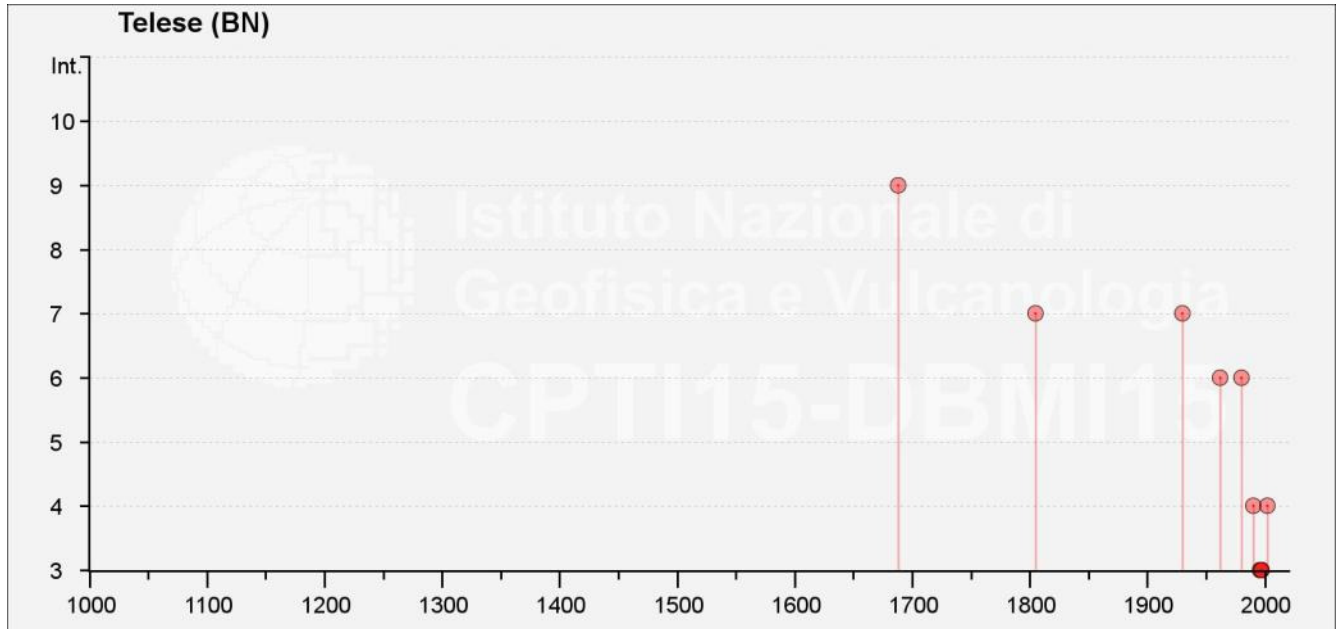
Figura 40– Grafico illustrante la storia sismica di Telese. Sulle ascisse sono riportati i riferimenti temporali espressi in anni, sulle ordinate le intensità sismiche (I) degli eventi rilevati (da http://emidius.mi.ingv.it/CPT115-DBMI15/ ).
