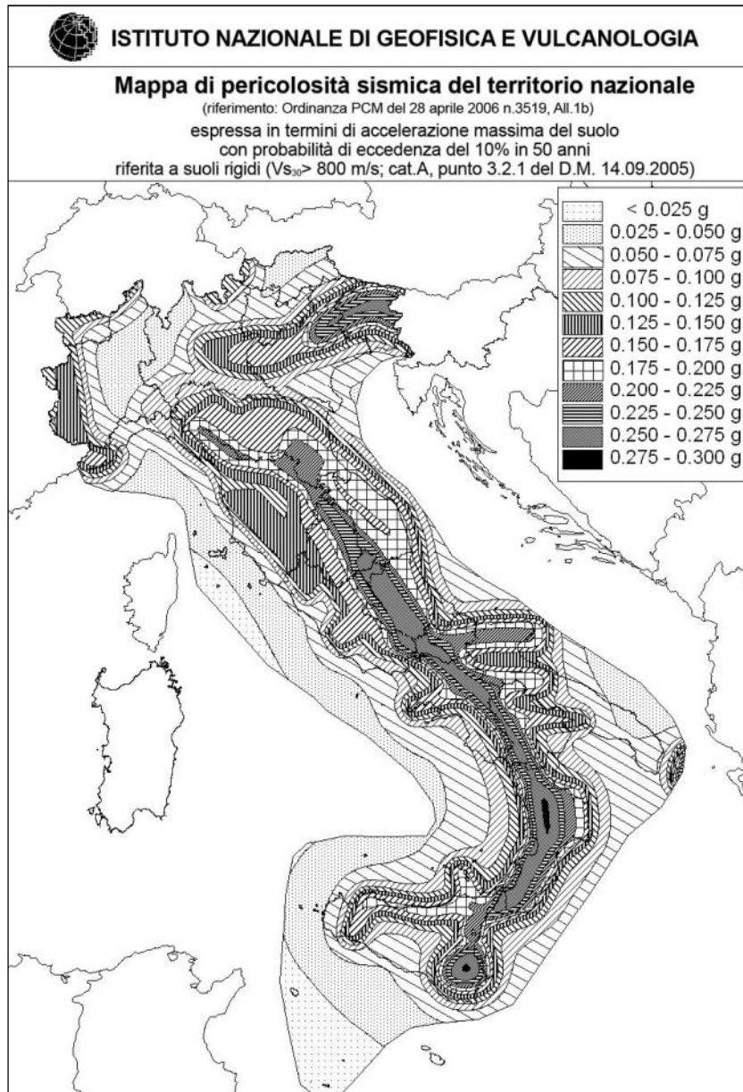
Figura 46 – Mappa di pericolosità sismica del territorio nazionale, espressa in termini di accelerazione massima del suolo con probabilità di eccedenza del 10% in 50 anni (da INGV 2006).
