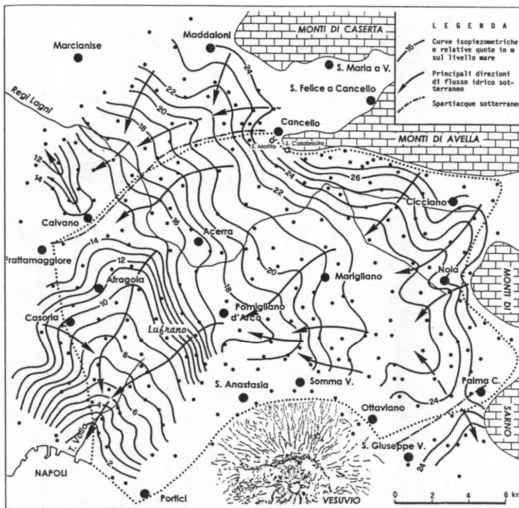
Figura 15 – Ricostruzione delle curve isopiezometriche e dei principali assi di drenaggio e spartiacque sotterranei del settore orientale della Piana Campana (Esposito 1996).
