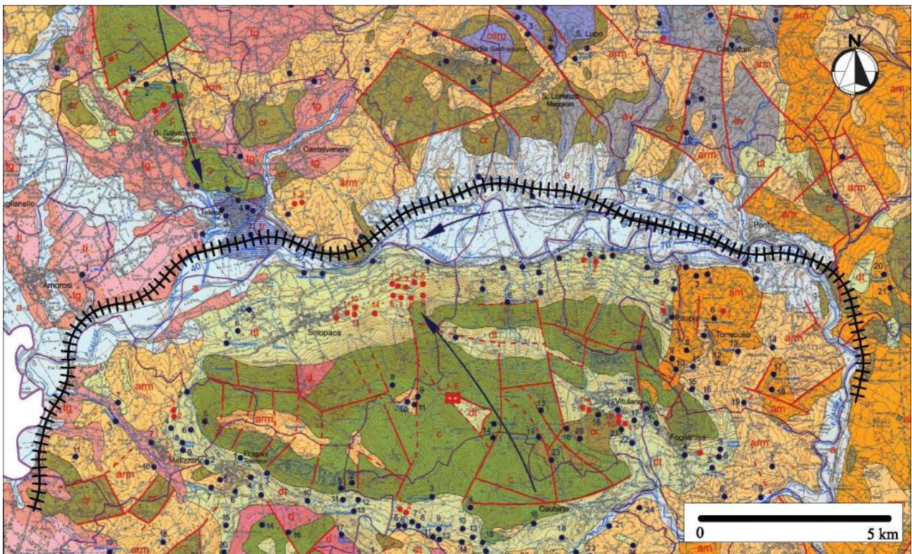
Figura 57 – Stralcio della Carta idrogeologica della Provincia di Benevento, con sovrapposizione del tracciato di progetto (da L. Esposito, P. Celico, F.M. Guadagno e S Aquino); con puntino rosso sono indicati i pozzi di interesse e con quelli blu le sorgenti.
