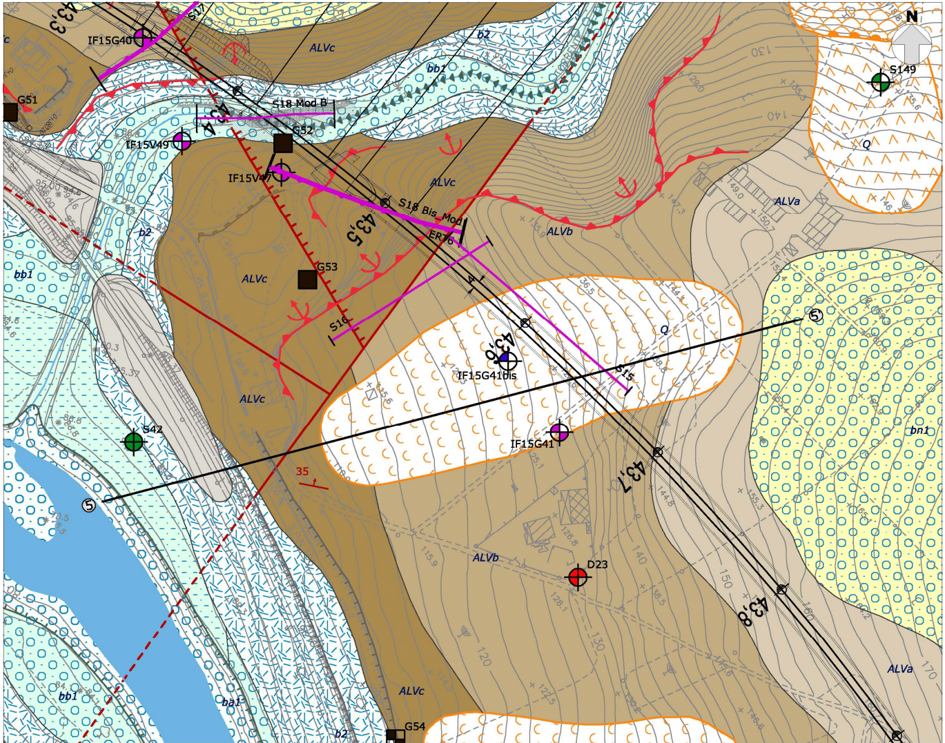
Figura 50 – Stralcio della carta geologica con elementi di geomorfologia km 43+600.
