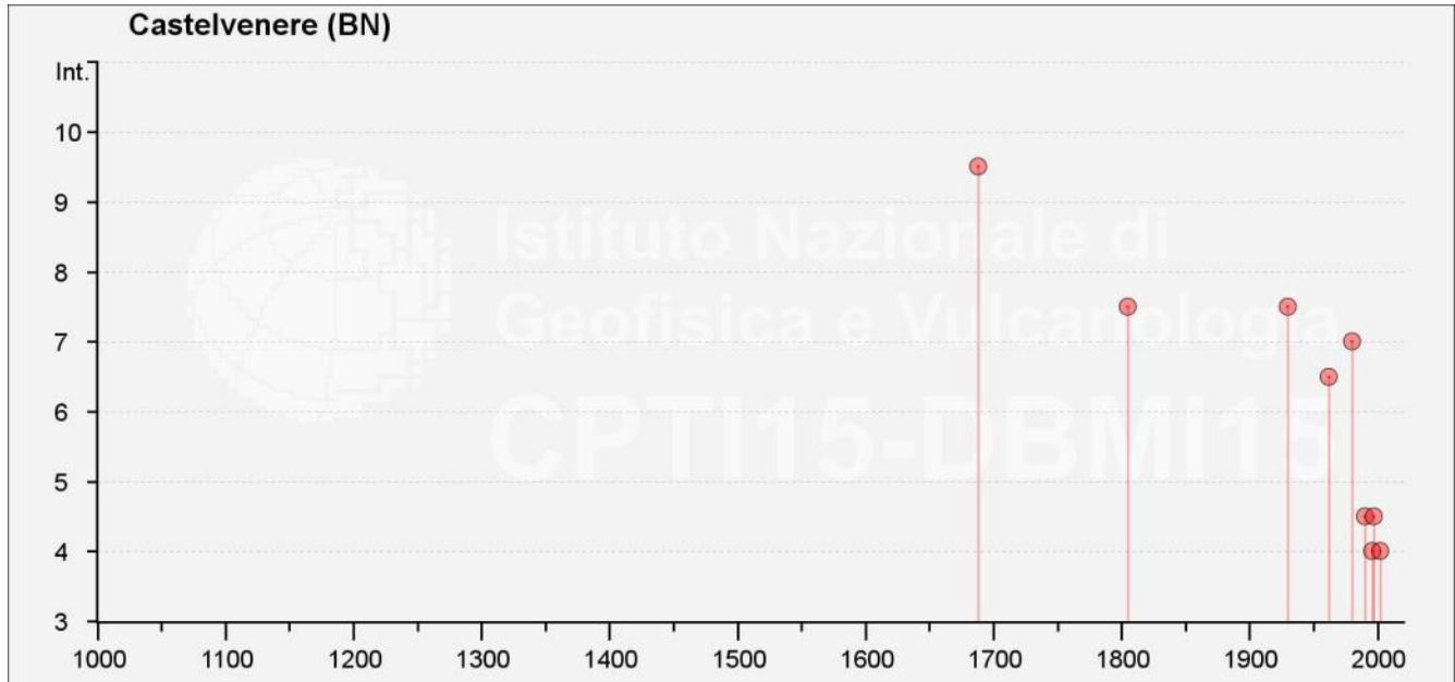
Figura 26– Grafico illustrante la storia sismica di Castelvenere (BN). Sulle ascisse sono riportati i riferimenti temporali espressi in anni, sulle ordinate le intensità sismiche (I) degli eventi rilevati (da http://emidius.mi.ingv.it/CPT115-DBMI15/ ).
