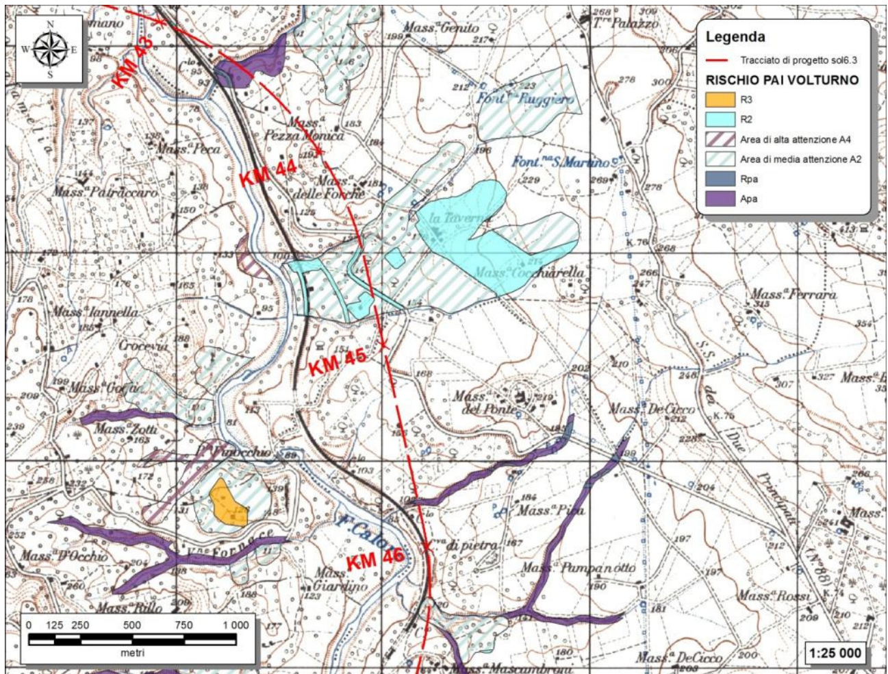
Figura 56 – Stralcio della carta del Rischio tratta dal Piano stralcio di Assetto Idrogeologico dei Fiumi Liri Garigliano e Volturno, tratto km 43+000÷46+500 circa.
