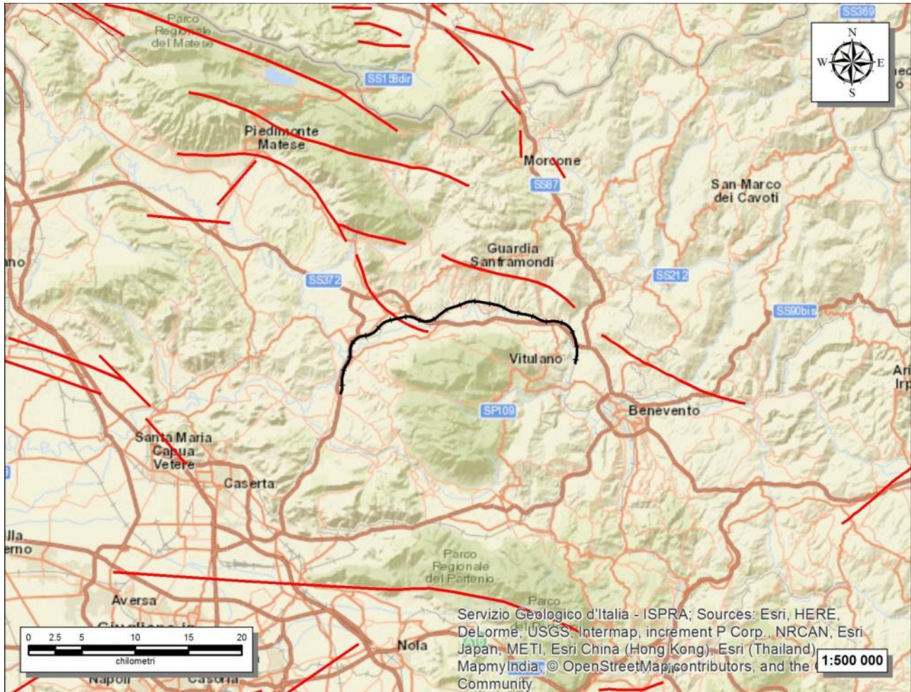
Figura 45 – Stralcio cartografico dell'area di studio con indicazione della tratta ferroviaria di progetto (in nero) e delle faglie capaci (in rosso) ( http://sgi.isprambiente.it/ArcGIS/rest/services/servizi/ithaca/MapServer ).
