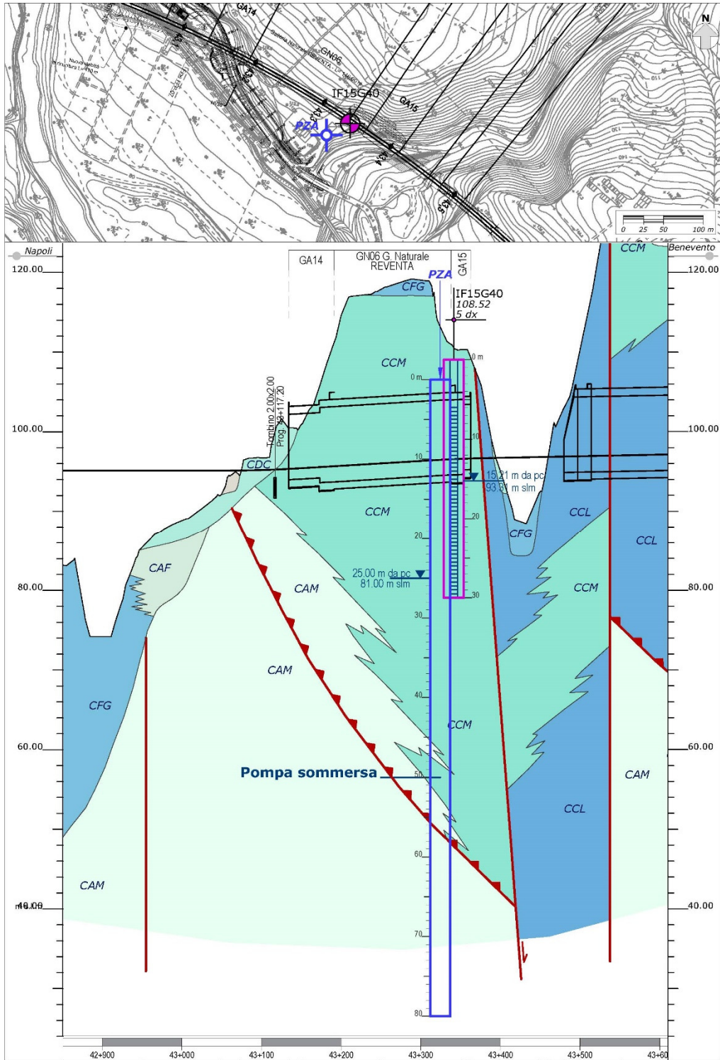
Figura 59 – planimetria di ubicazione del piezometro IF15G40 e del PZA e sezione idrogeologica con indicazione del pozzo e dei livelli di falda registrati.
